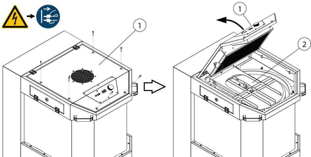
Bild 27: Filterbyte – Åtkomst till filterpatronen
