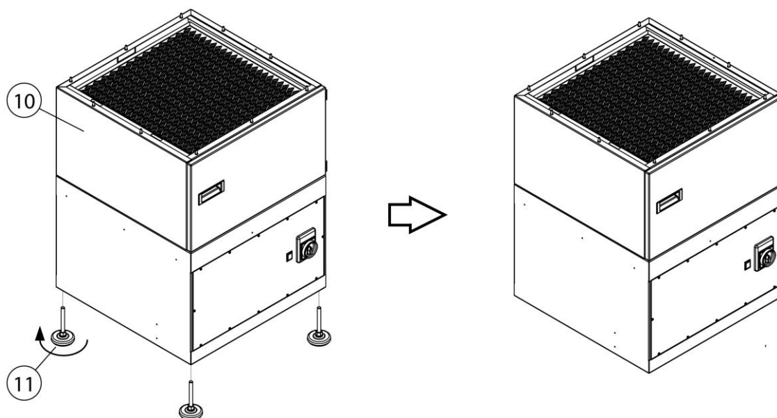
Rys. 139: Montaż – demontaż nóg maszyny
