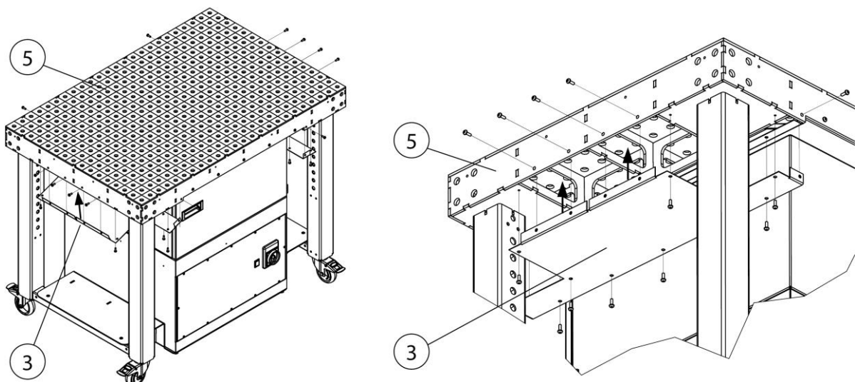
Afb. 59: Montage – stofkuiplaat
