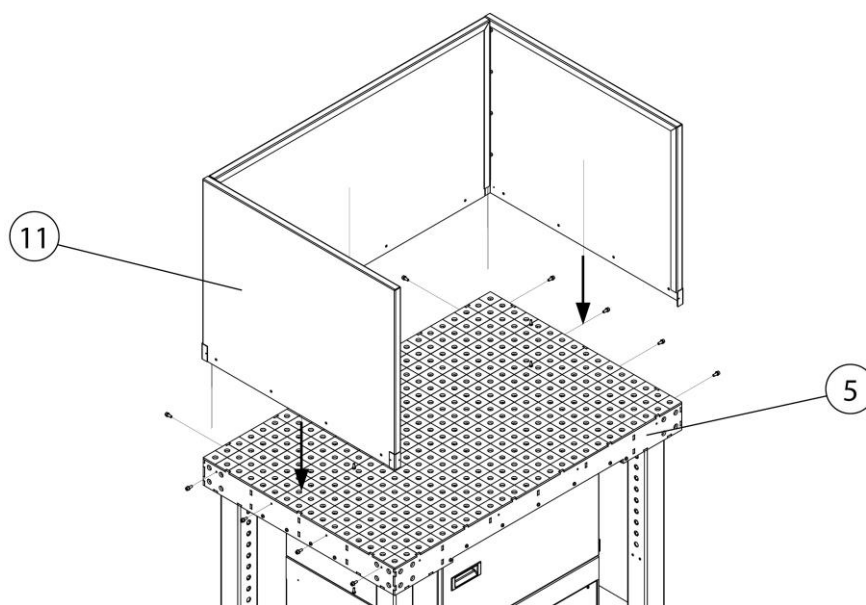
Fig. 43: Montage – Paroi latérale (en option)
