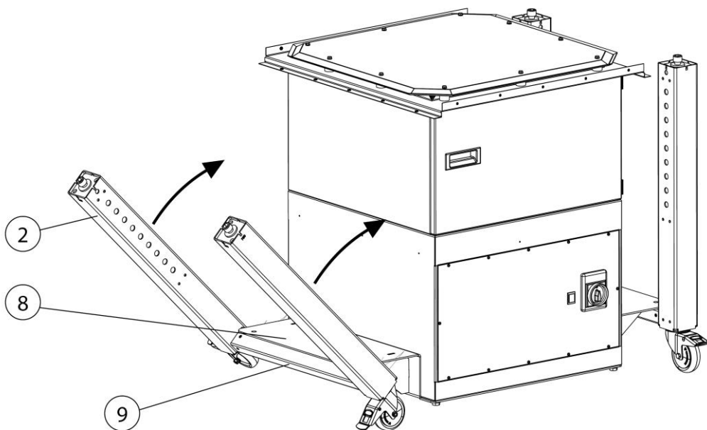
Abb. 6: Montage - Tischbeine
