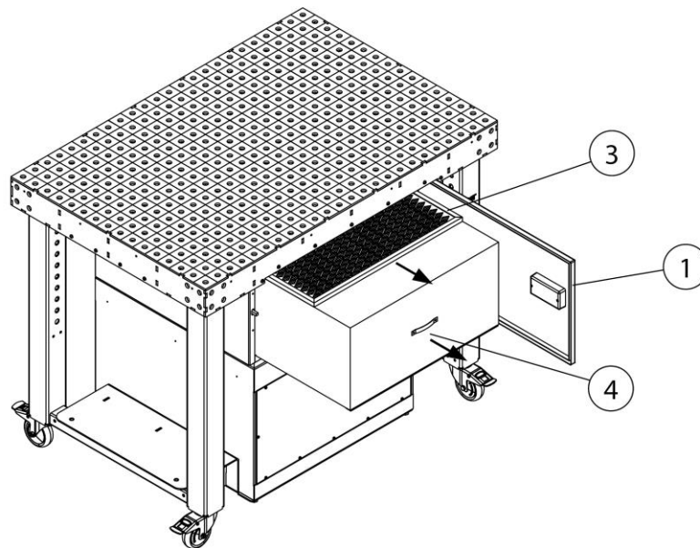
183. ábra: Szűrőcsere - Előszűrő + Főszűrő
