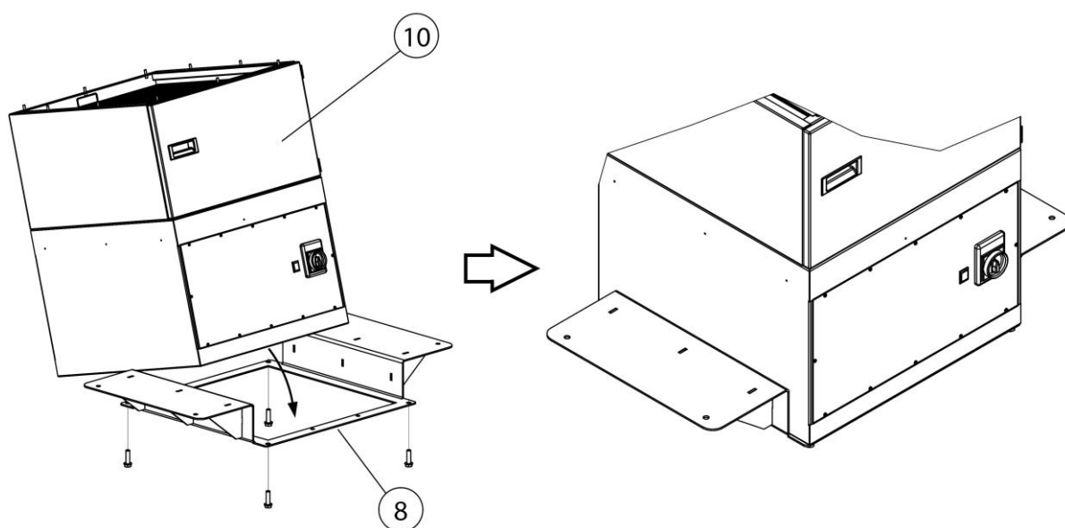
Fig. 72: Montaje – Montar el equipo de filtro sobre el bastidor portante
