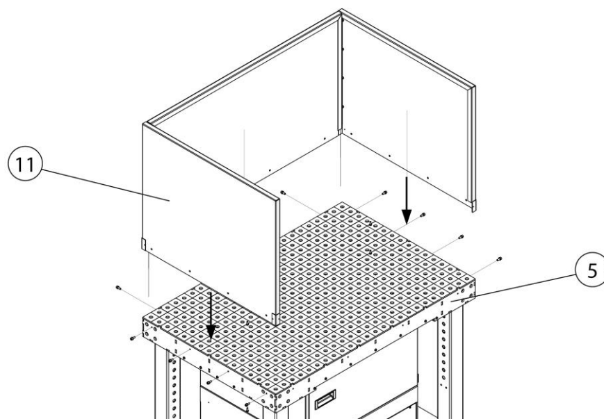
Sl. 196: Montaža – Stranska stena (izbirno)
