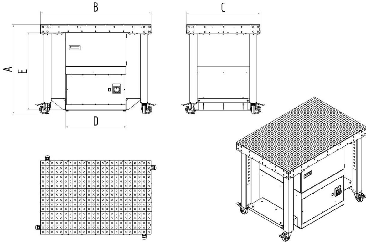
186. ábra: Méretlap
