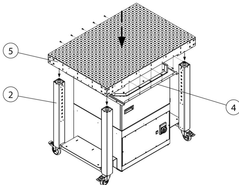
Obr. 126: Montáž – deska stolu
