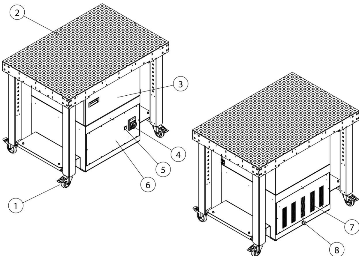
Obr. 120: Pozice na výrobku
