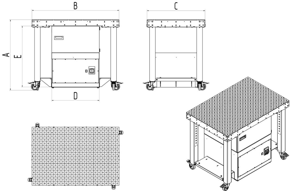
Afb. 67: Maatblad
