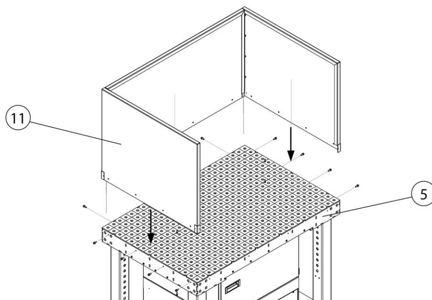
Fig. 111: Montaggio – Parete laterale (opzionale)
