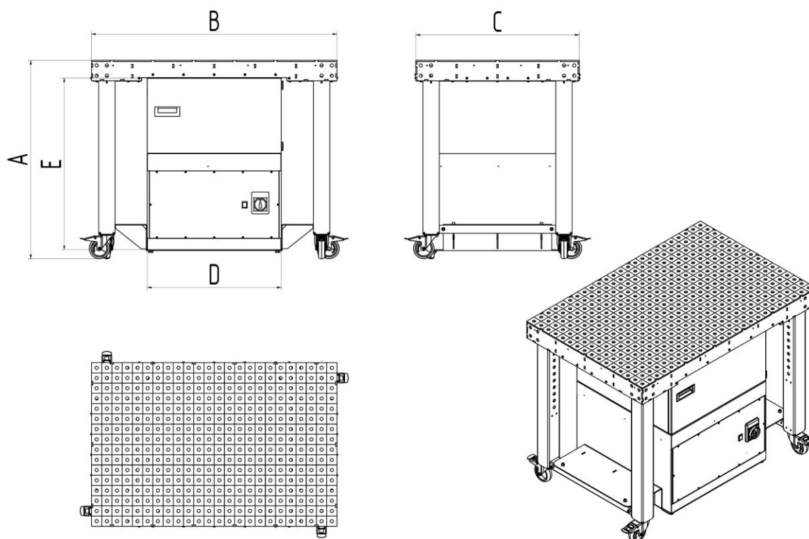
Рис. 169: Габаритный чертеж
