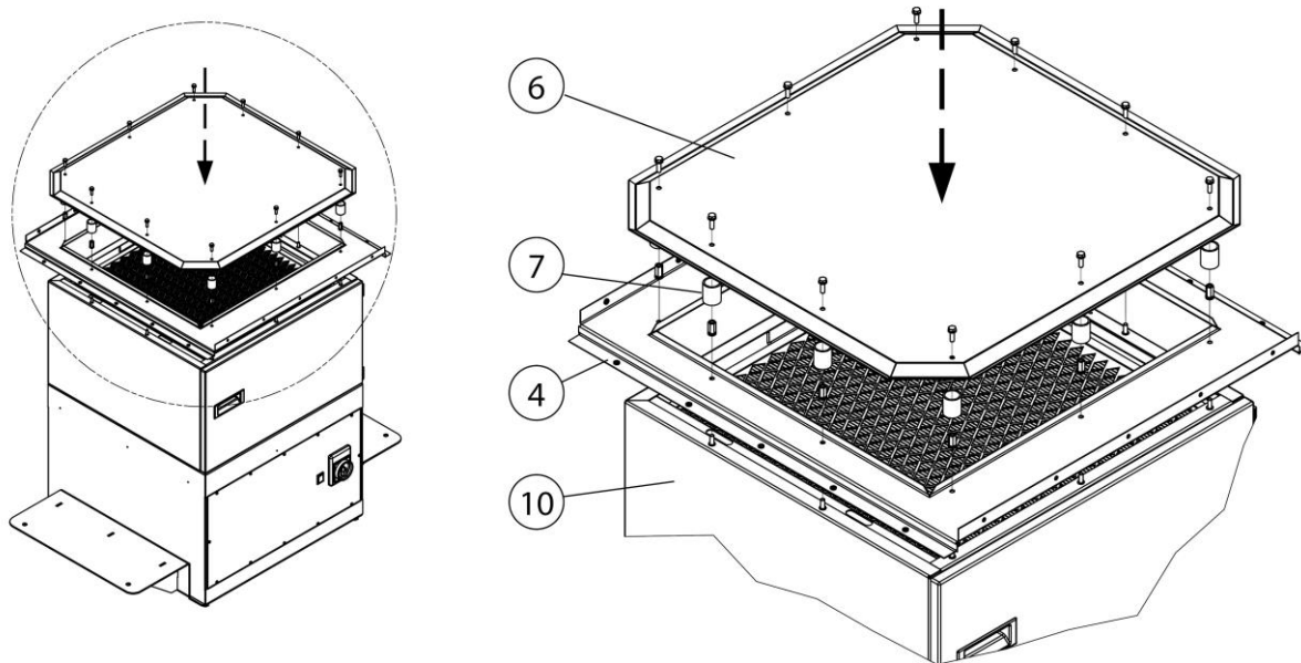
Afb. 56: Montage – steunframe en vonkplaat
