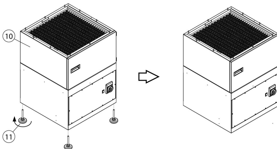
Рис. 156: Монтаж – демонтаж опор машины
