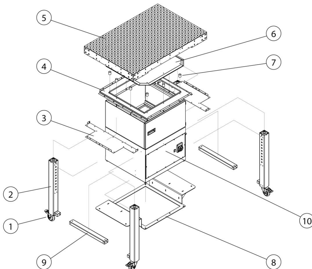
Fig. 87: Montagem – Vista geral dos componentes
