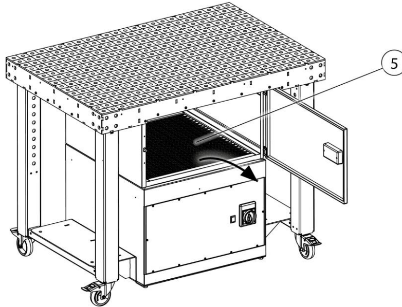
184. ábra: Szűrőcsere - Aktívszén-szűrő (opcionális)
