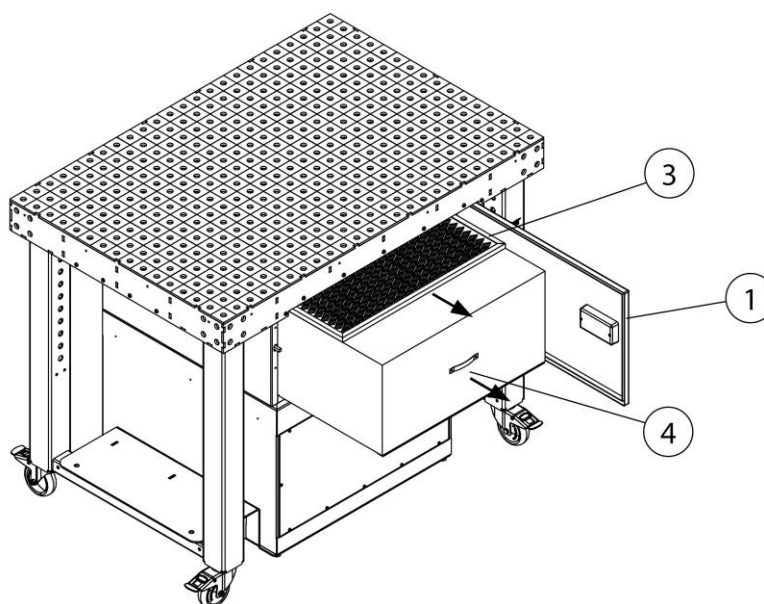
Рис. 166: Замена фильтра – фильтра предварительной очистки + основного фильтра
