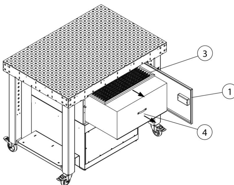
Fig. 98: Substituição dos filtros – Pré-filtro + filtro principal
