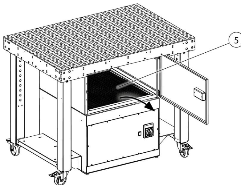
Fig. 116: Sostituzione filtro – filtro a carbone attivo (opzionale)
