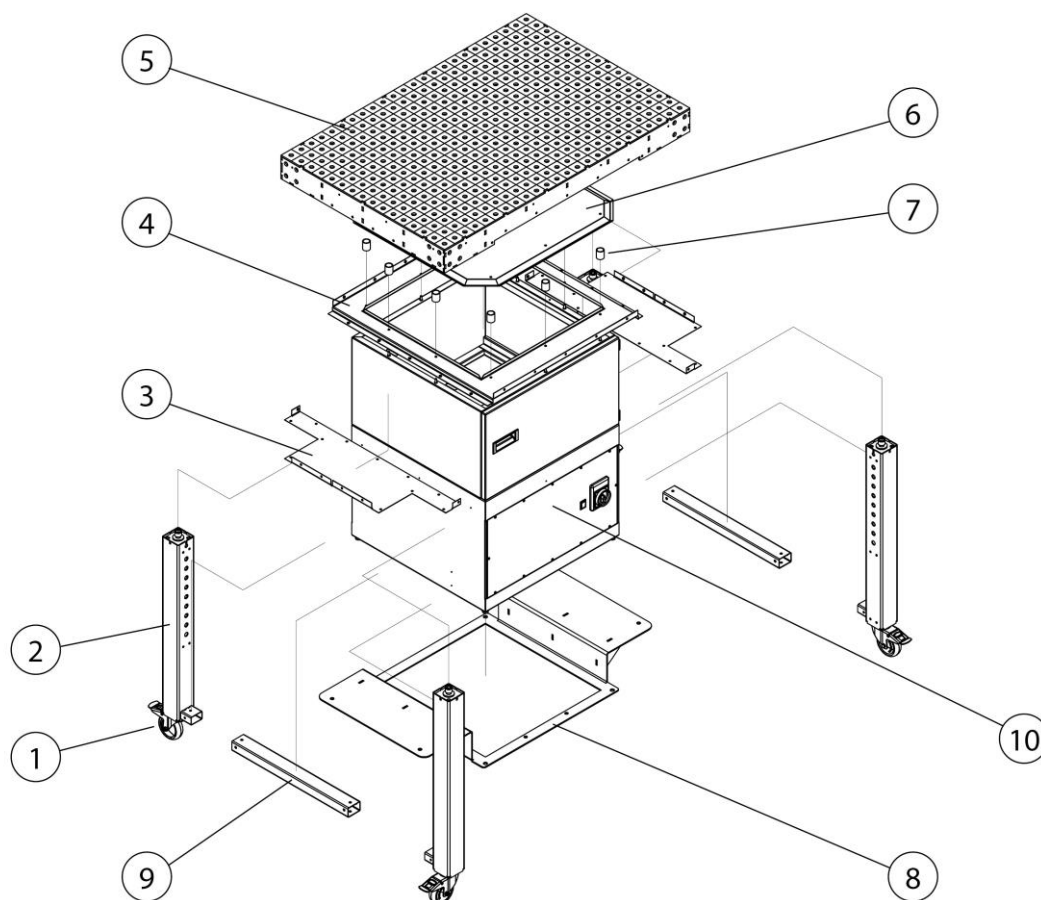
172. ábra: Szerelés – Az alkatrészek áttekintése
