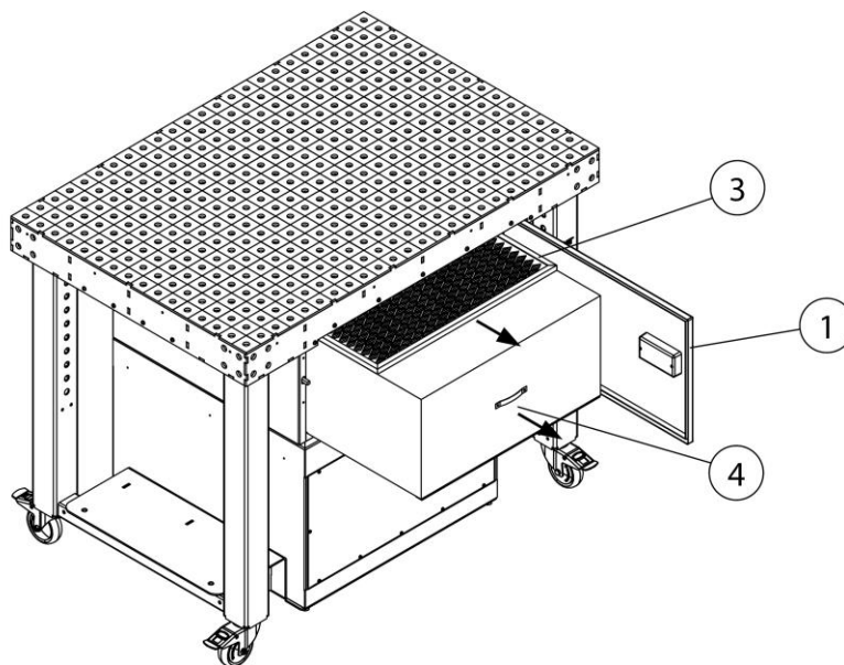
Sl. 200: Menjava filtra – Prefilter + glavni filter
