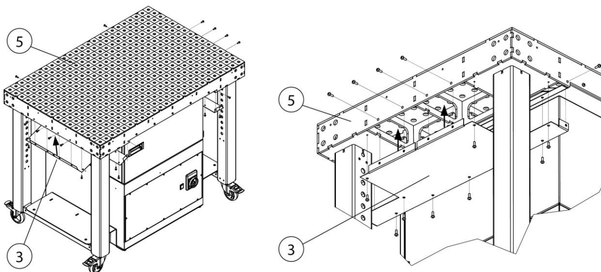
Fig. 76: Montaje - Chapa de bandeja recogepolvo
