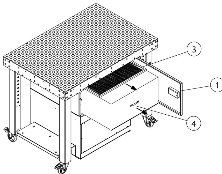
Afb. 64: Filtervervanging – voorfilter + hoofdfilter
