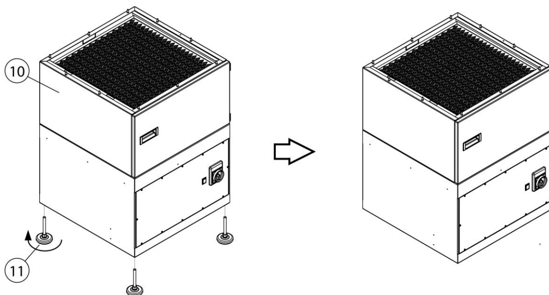
Obr. 122: Montáž – demontáž noh stroje
