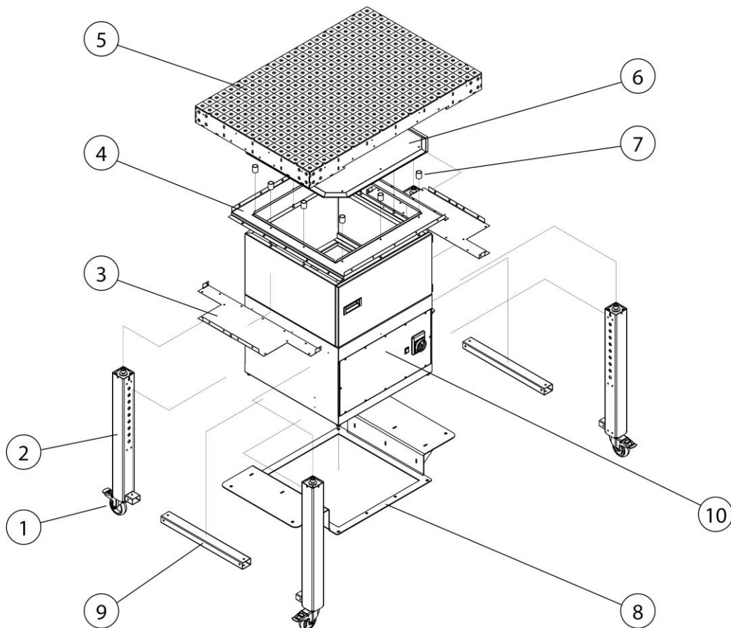
Afb. 53: Montage – Overzicht van de onderdelen
