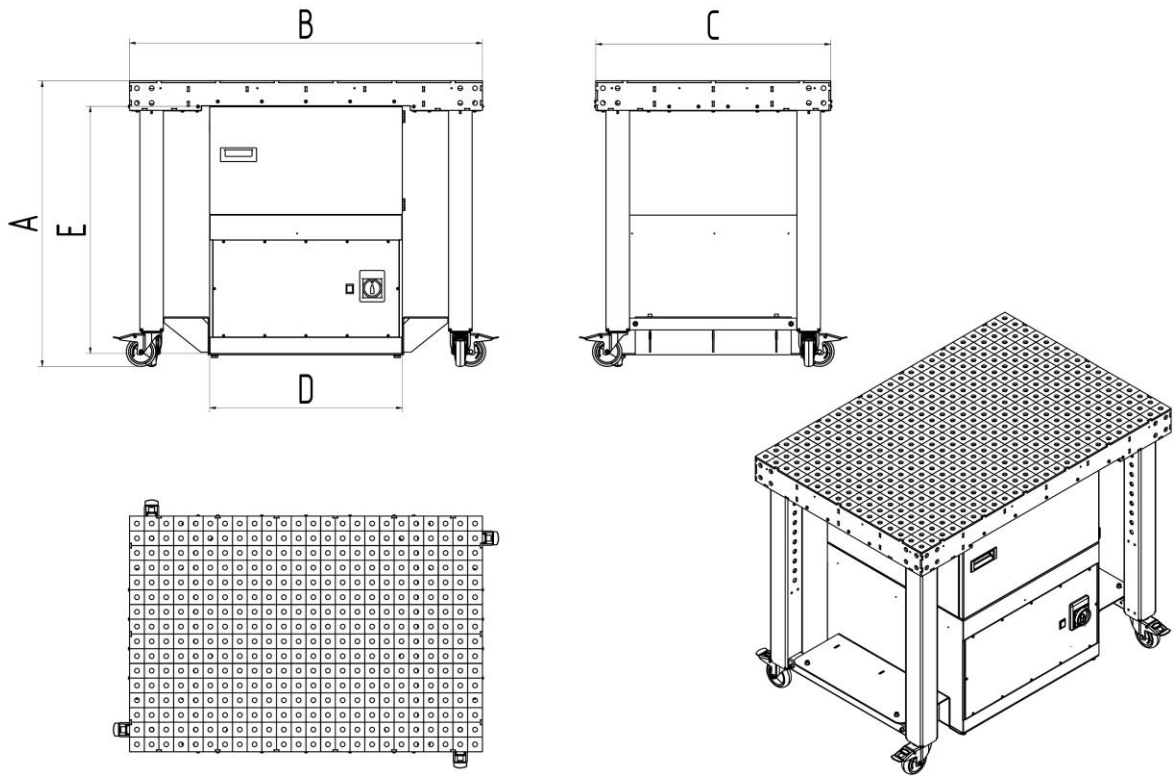
Fig. 50 : Fiche dimensionnelle
