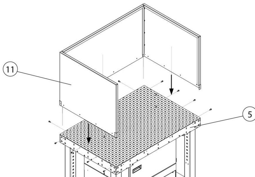
Рис. 162: Монтаж – боковая стенка (опция)
