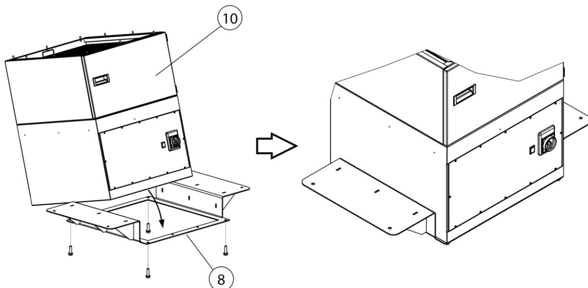
Fig. 38 : Montage – Montage de l'appareil de filtration sur le cadre porteur
