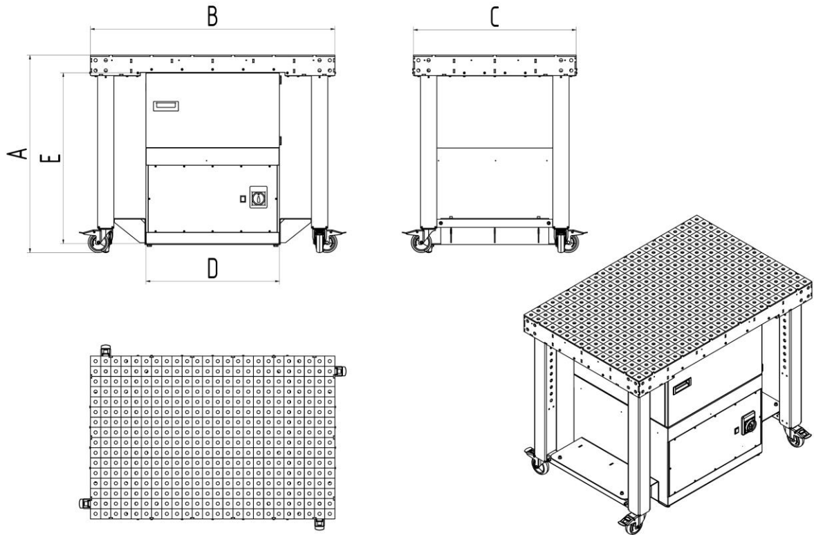
Abb. 16: Maßblatt
