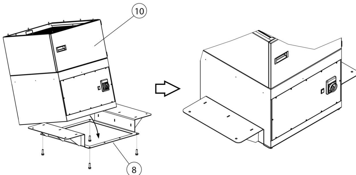
Fig. 89: Montagem – Montar aparelho de filtragem sobre armação portadora
