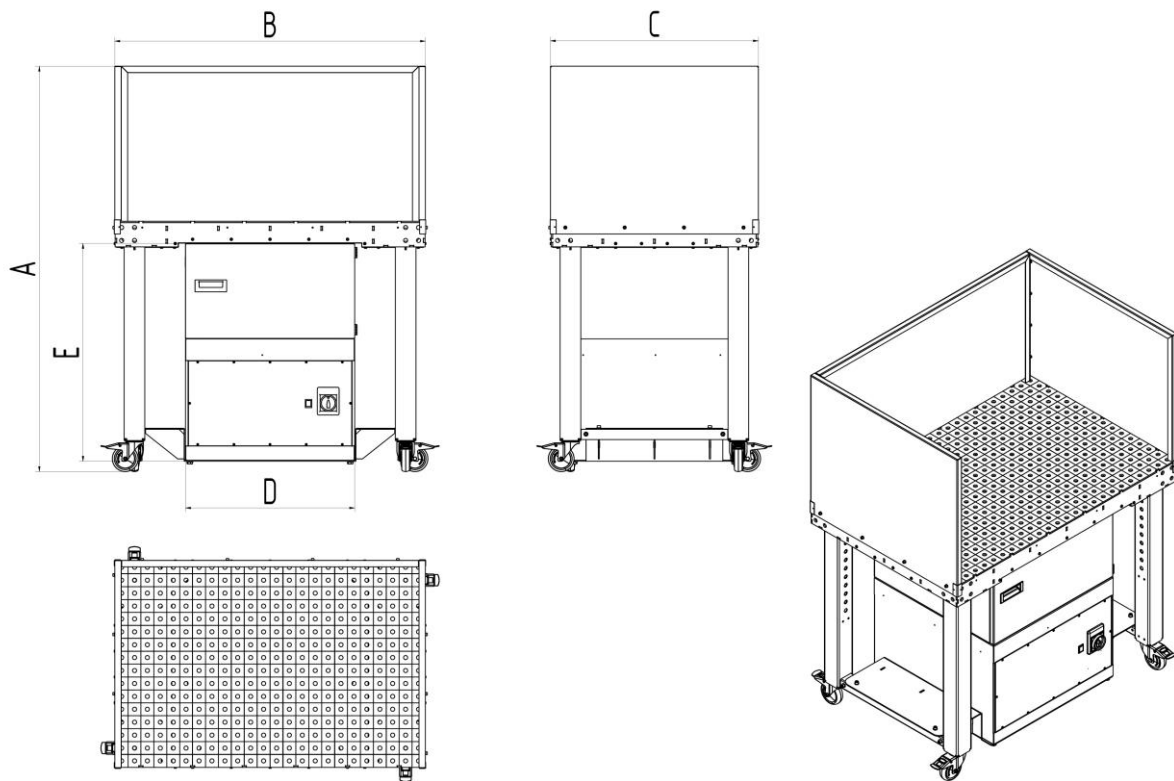
Abb. 17: Maßblatt mit Seitenwand
