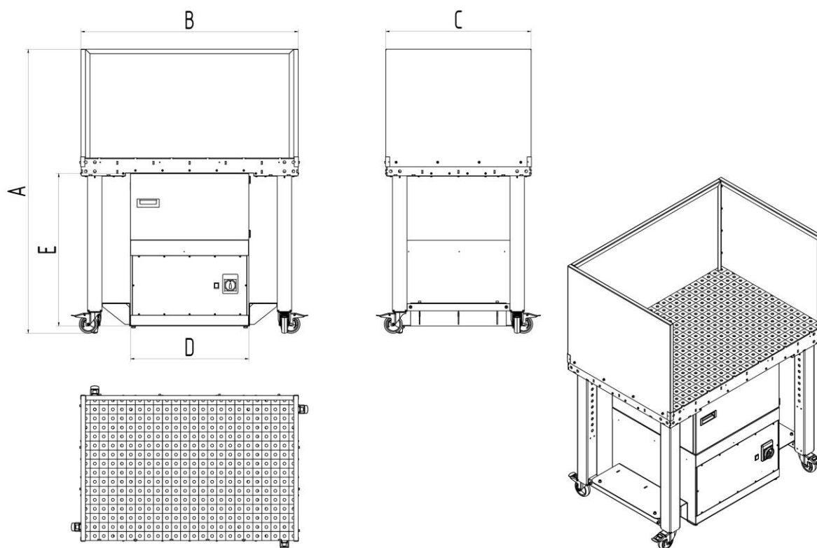
Fig. 85: Hoja de medidas con pared lateral
