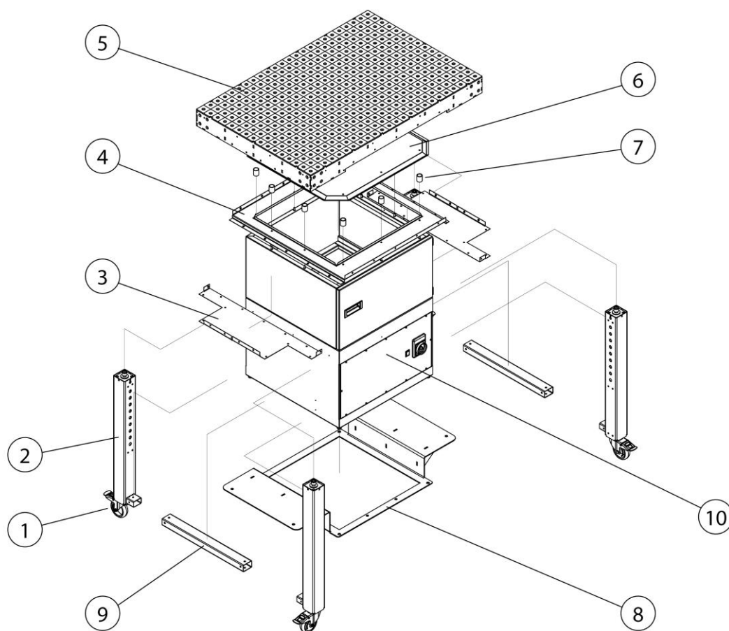
Fig. 104: Montaggio – Panoramica dei componenti
