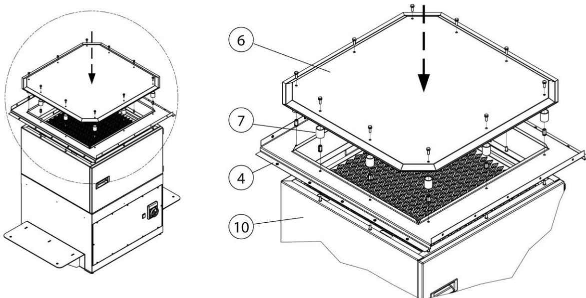
Рис. 158: Монтаж – опорная рама и искрозащитный экран
