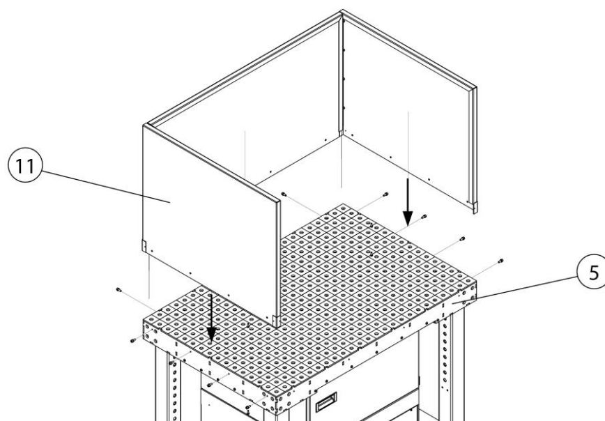
Afb. 60: Montage – zijwand (optioneel)
