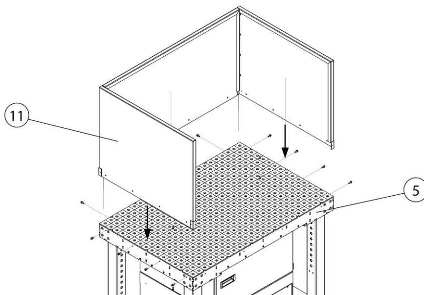
Obr. 128: Montáž – bočnice (volitelně)
