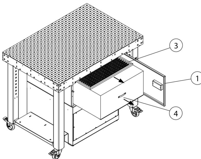
Рис. 163: Контроль направления вращения вентилятора
