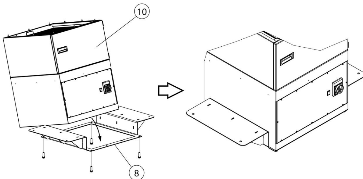
174. ábra: Szerelés – A szűrőkészülék felszerelése a tartókeretre
