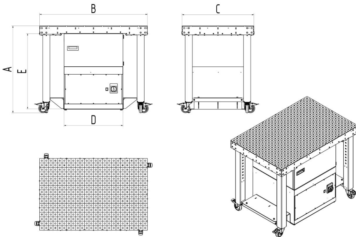
Fig. 118: Disegno quotato
