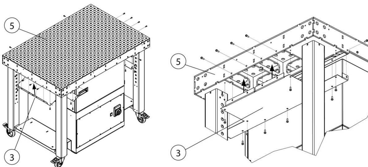
Fig. 93: Montagem - Chapa de tina para pó
