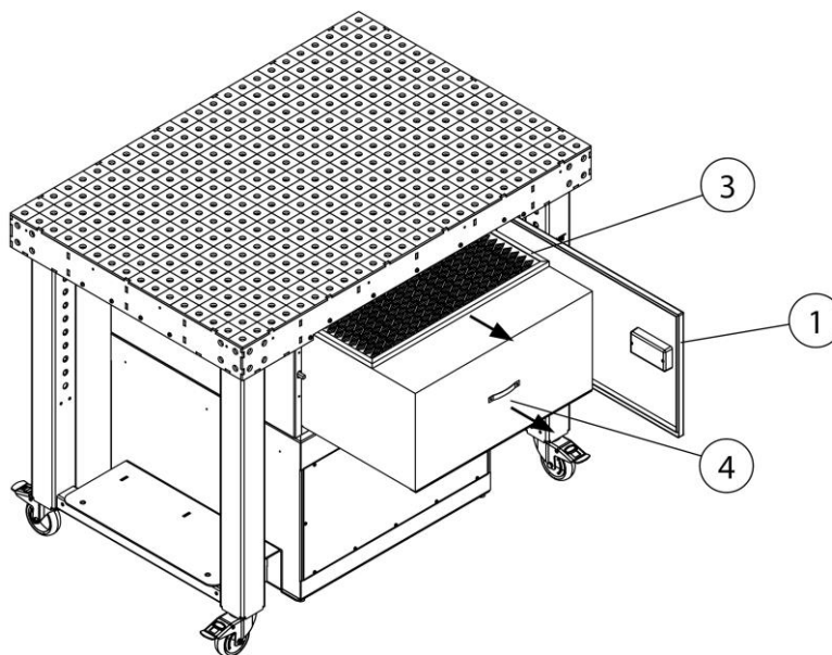
Obr. 129: Kontrola směru otáčení ventilátoru
