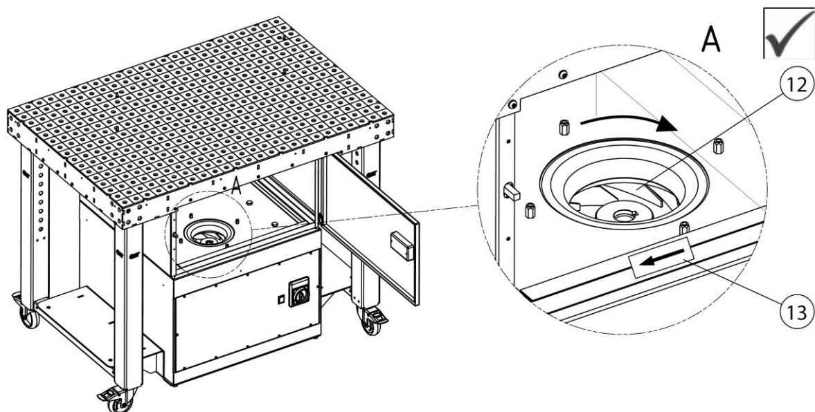
Afb. 62: Draairichting van het ventilator-schoepenwiel controleren
