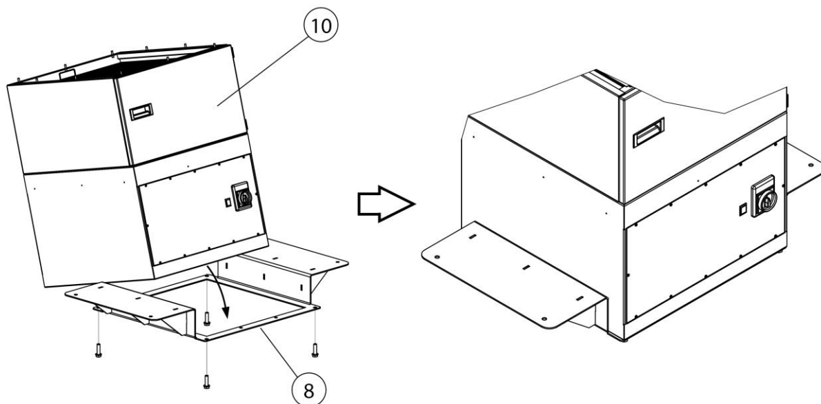
Fig. 106: Montaggio – Montaggio del dispositivo di filtraggio sul telaio di supporto
