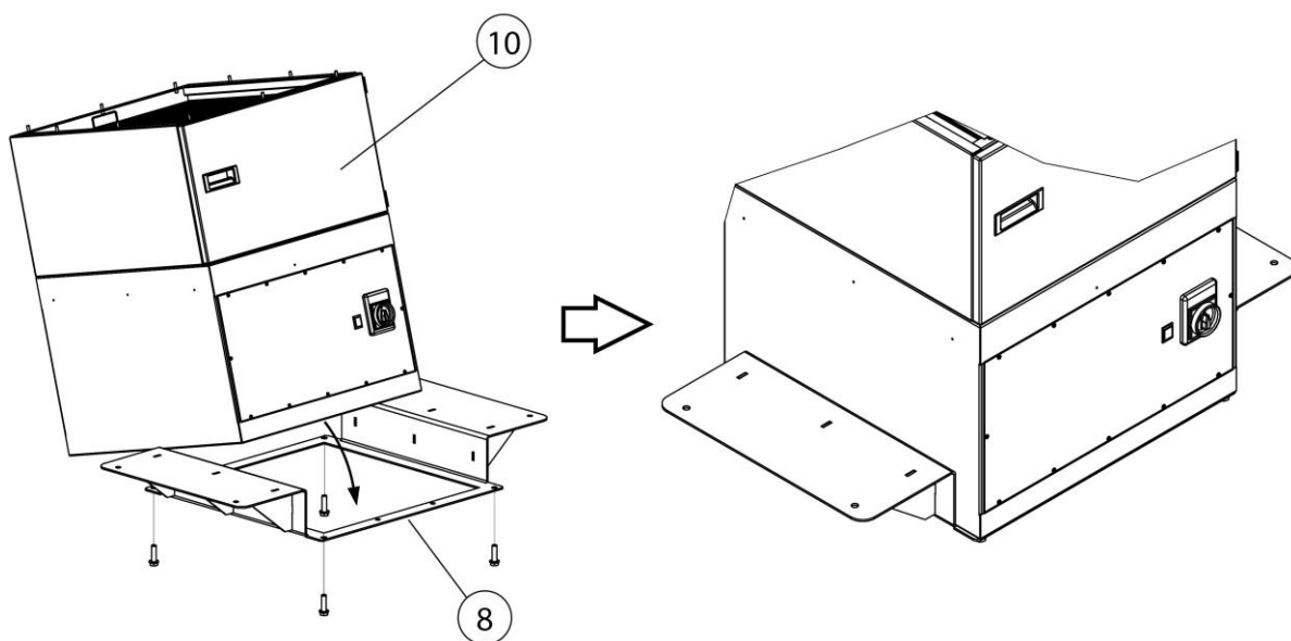
Рис. 157: Монтаж – установка фильтровального устройства на опорной раме
