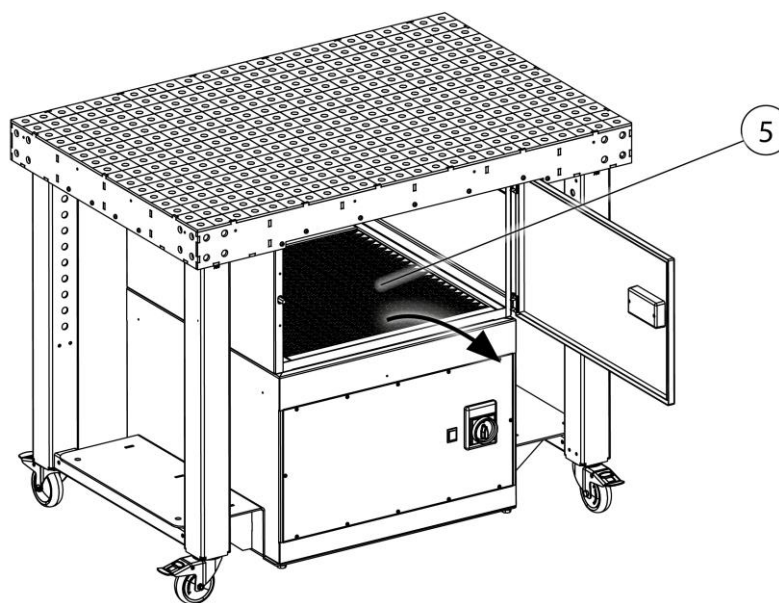
Sl. 201: Menjava filtra – Filter z aktivnim ogljem (izbirno)
