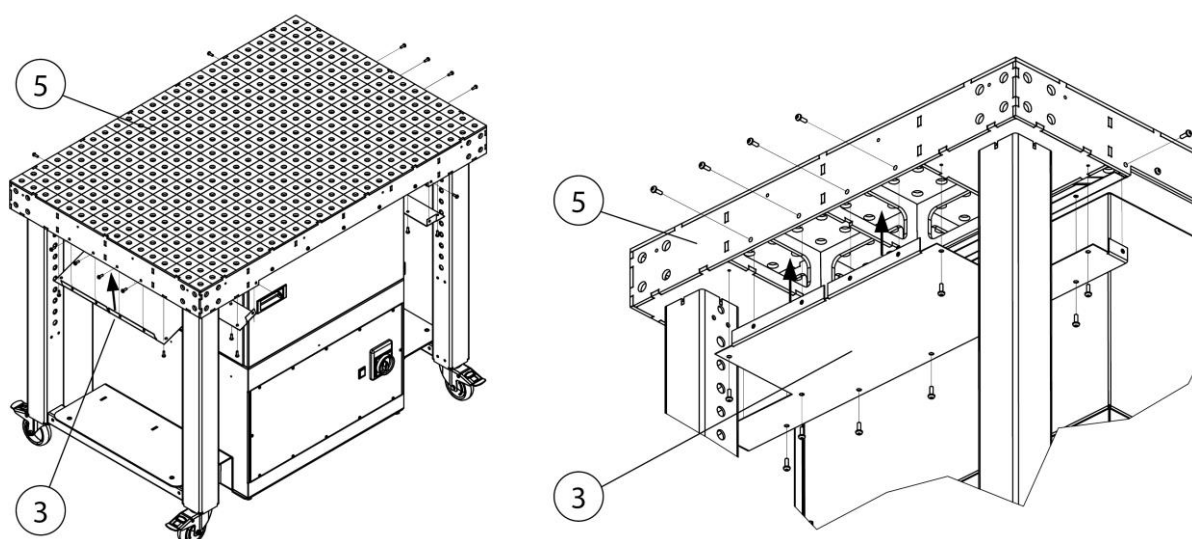
Fig. 110: Montaggio - Lamiera raccoglitrice polvere
