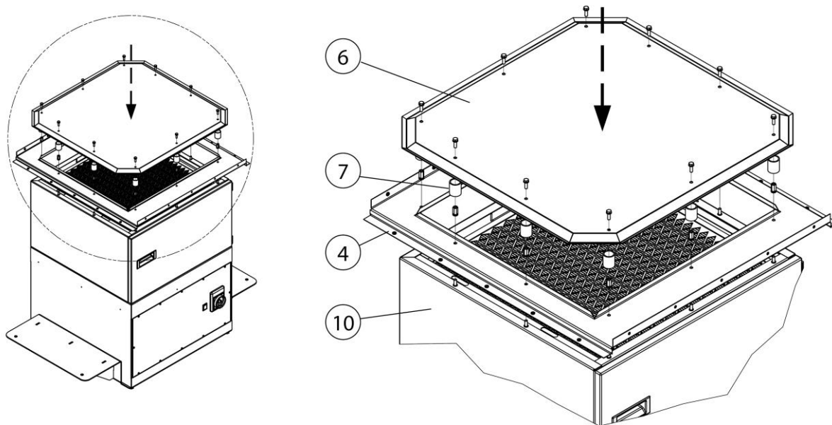
Fig. 90: Montagem -Armação de suporte + chapa de proteção contra faíscas
