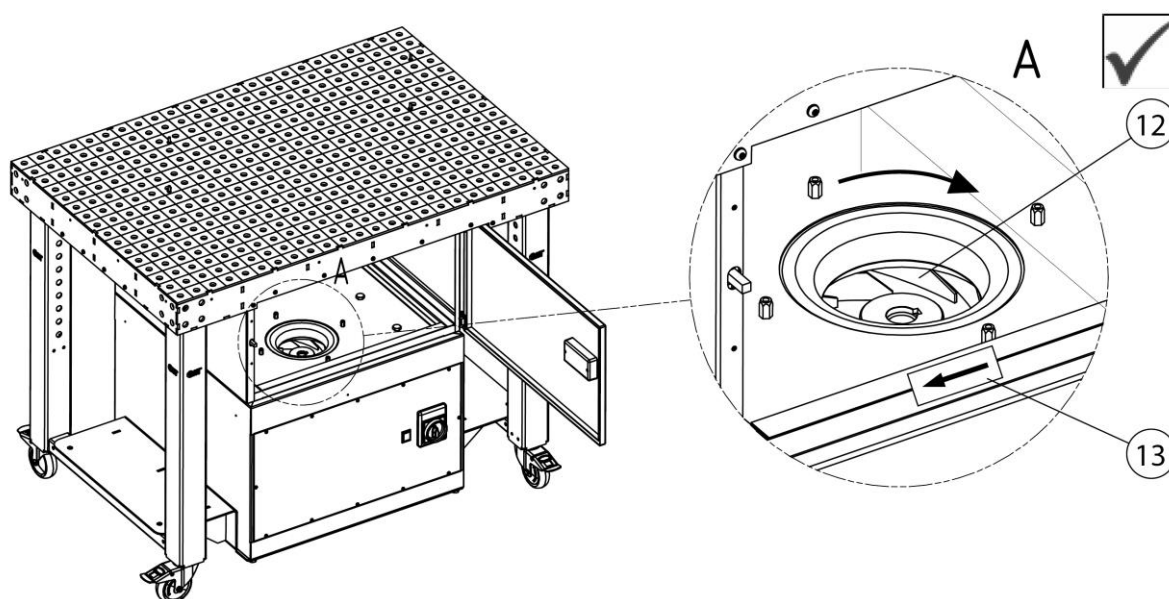
Obr. 130: Kontrola směru otáčení oběžného kola ventilátoru
