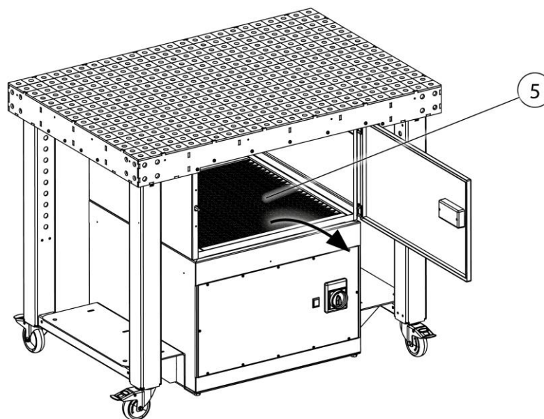
Fig. 82: Cambio de filtro– filtro de carbón activo (opcional)
