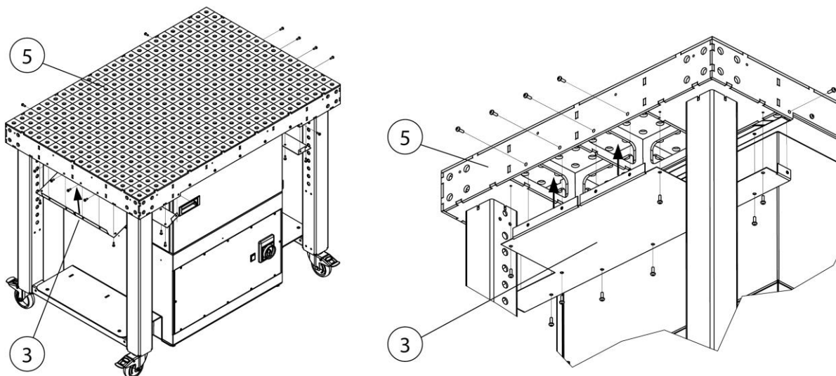
Obr. 127: Montáž – plech prachové vany
