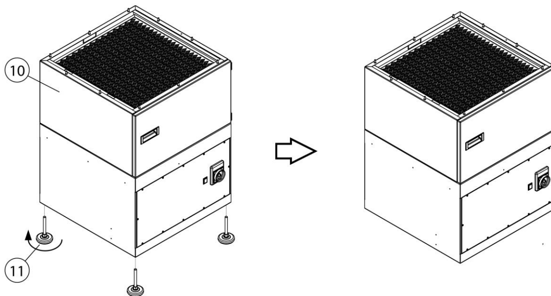
Fig. 88: Montagem – Desmontar os pés da máquina
