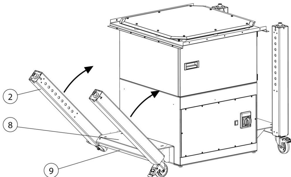
Рис. 159: Монтаж – ножки стола
