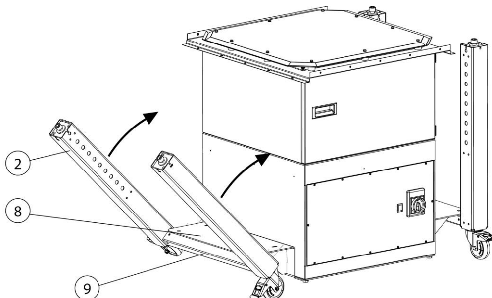
Fig. 40 : Montage - Pieds de la table
