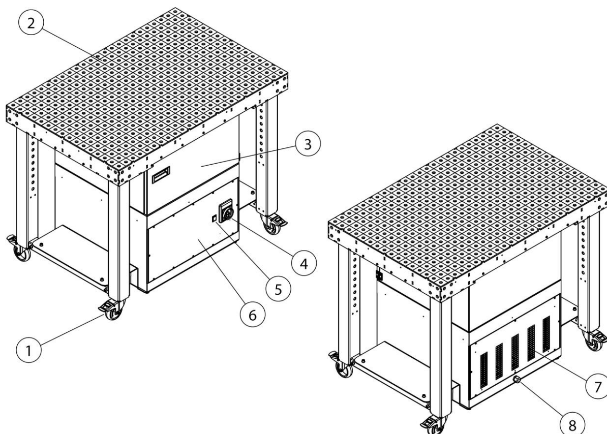
Sl. 188: Položaji na izdelku
