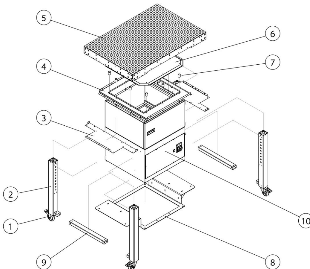
Fig. 36 : Montage – Aperçu des composants
