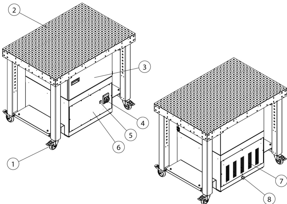
Afb. 52: Posities op het product
