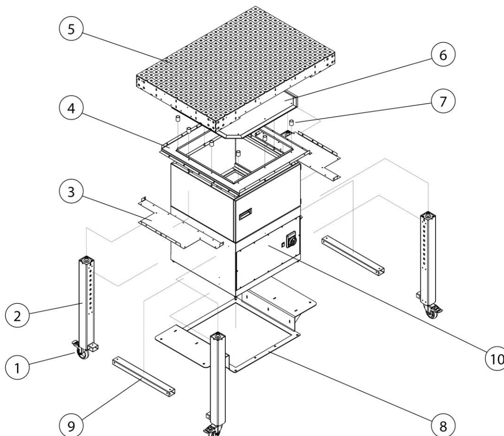
Fig. 70: Montaje - Visión general de los componentes
