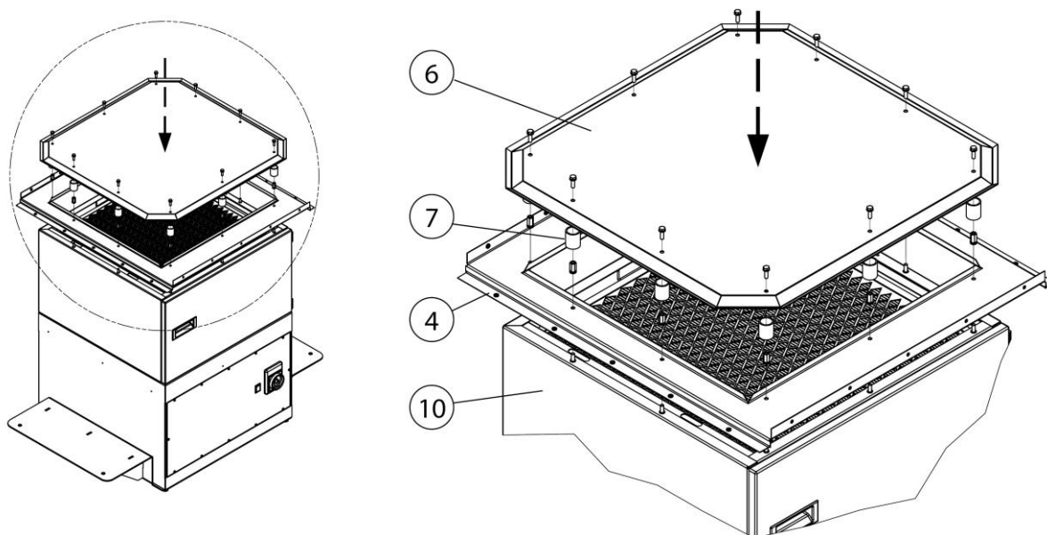
Obr. 124: Montáž – podpěrný rám a jiskrový plech
