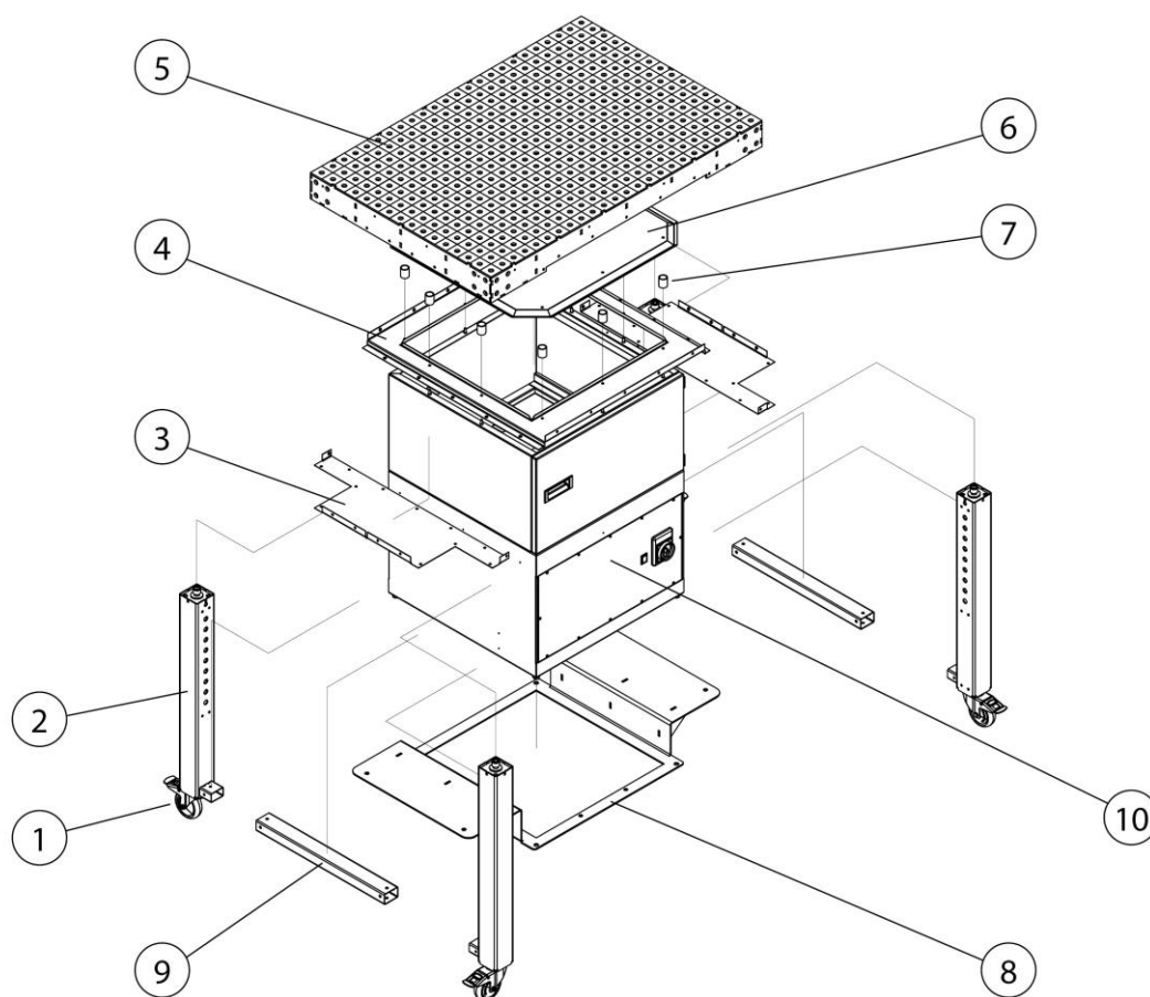
Rys. 138: Montaż – specyfikacja części
