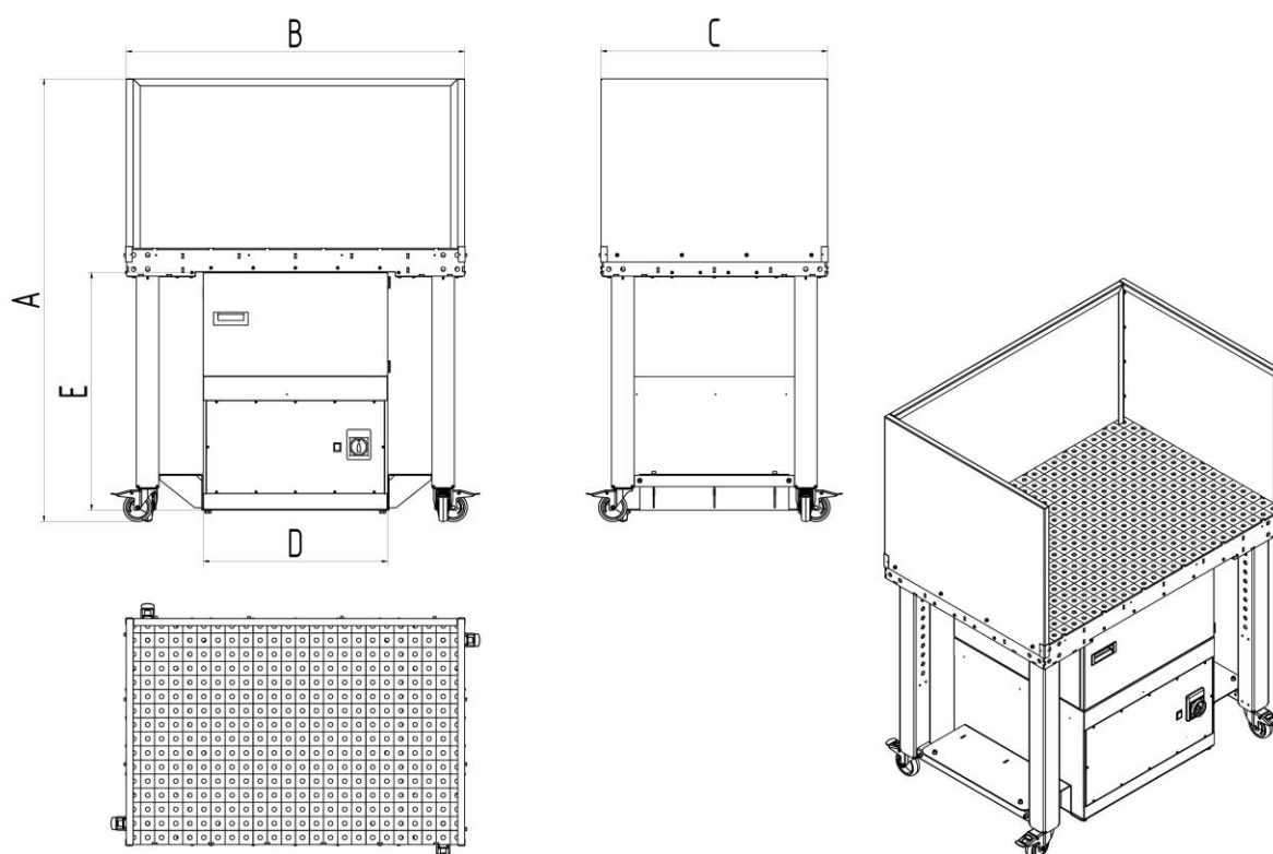
Fig. 51 : Fiche dimensionnelle avec paroi latérale
