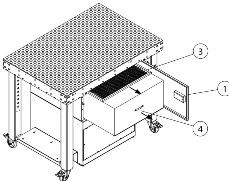
Obr. 132: Výměna filtrů – předřazený filtr + hlavní filtr
