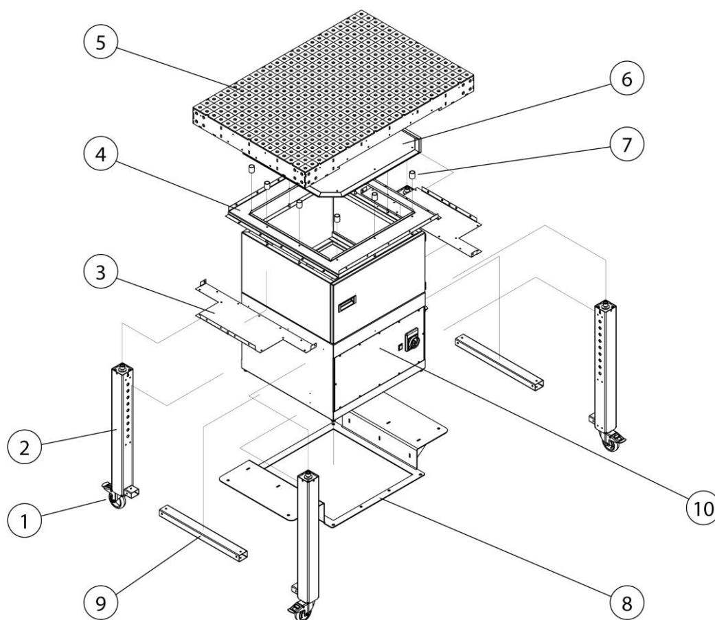
Sl. 189: Montaža – Pregled sestavnih delov
