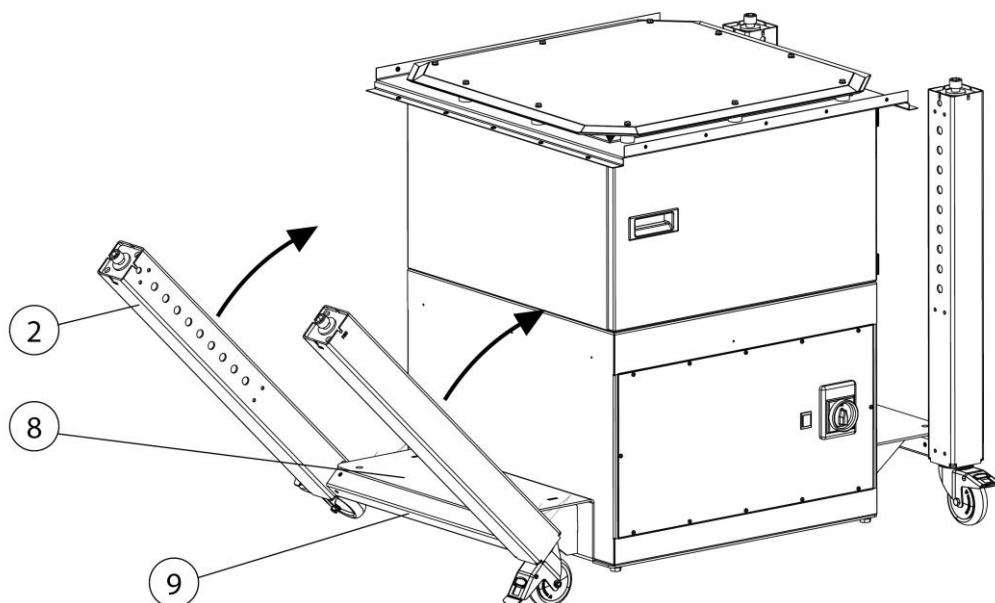
176. ábra: Szerelés – Asztallábak
