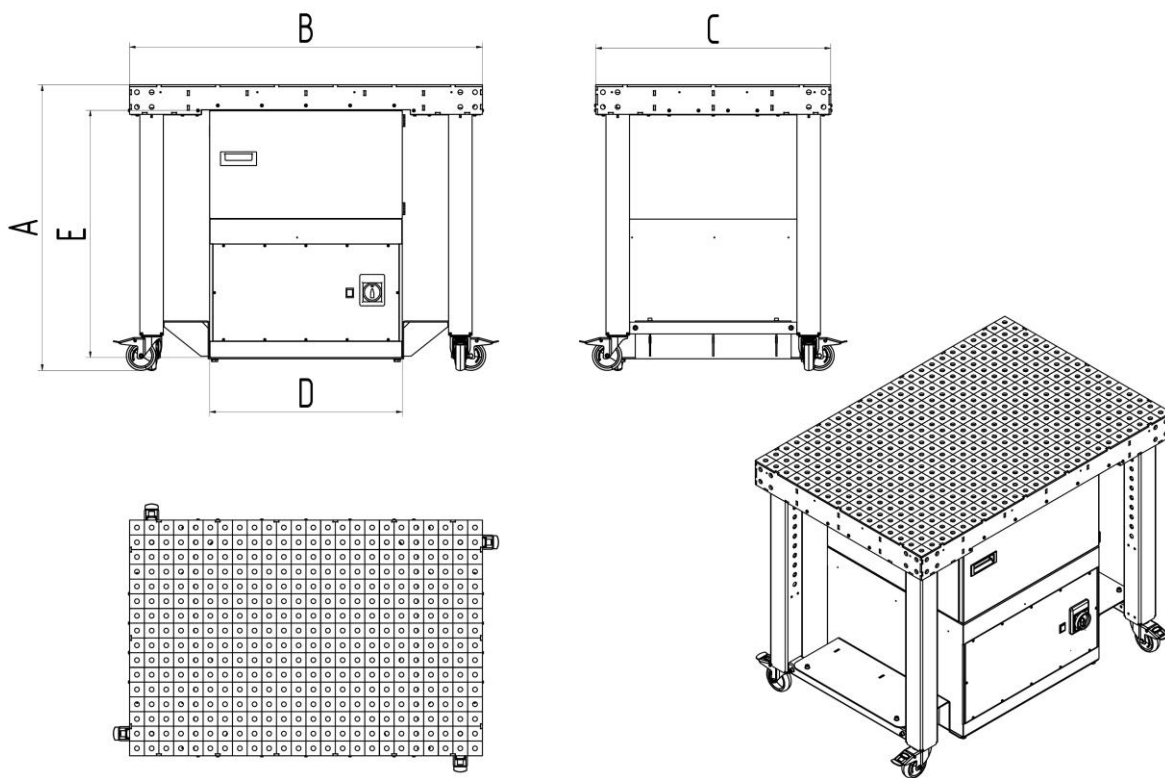
Fig. 84: Hoja de medidas
