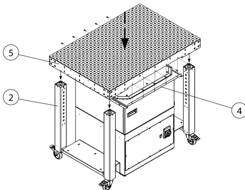
Fig. 92: Montagem - Tampo da mesa
