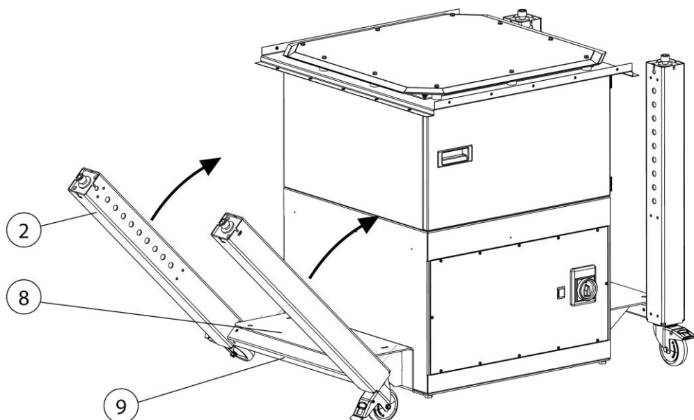
Afb. 57: Montage – tafelpoten
