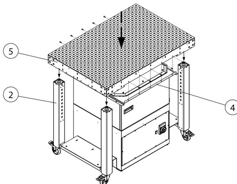
Рис. 160: Монтаж – столешница
