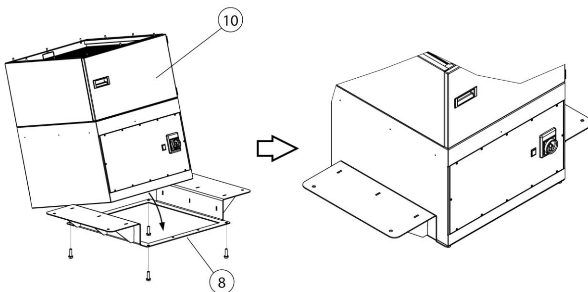
Rys. 140: Montaż – montaż urządzenia filtrującego na ramie nośnej
