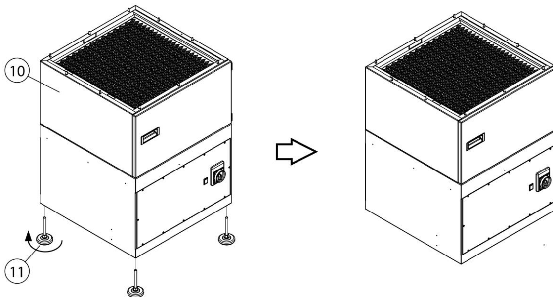
Sl. 190: Montaža – Odstranitev nog naprave
