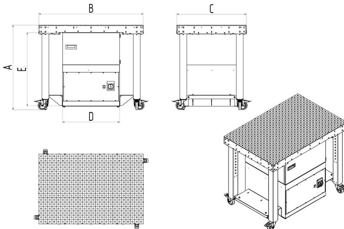
Rys. 152: Karta wymiarów
