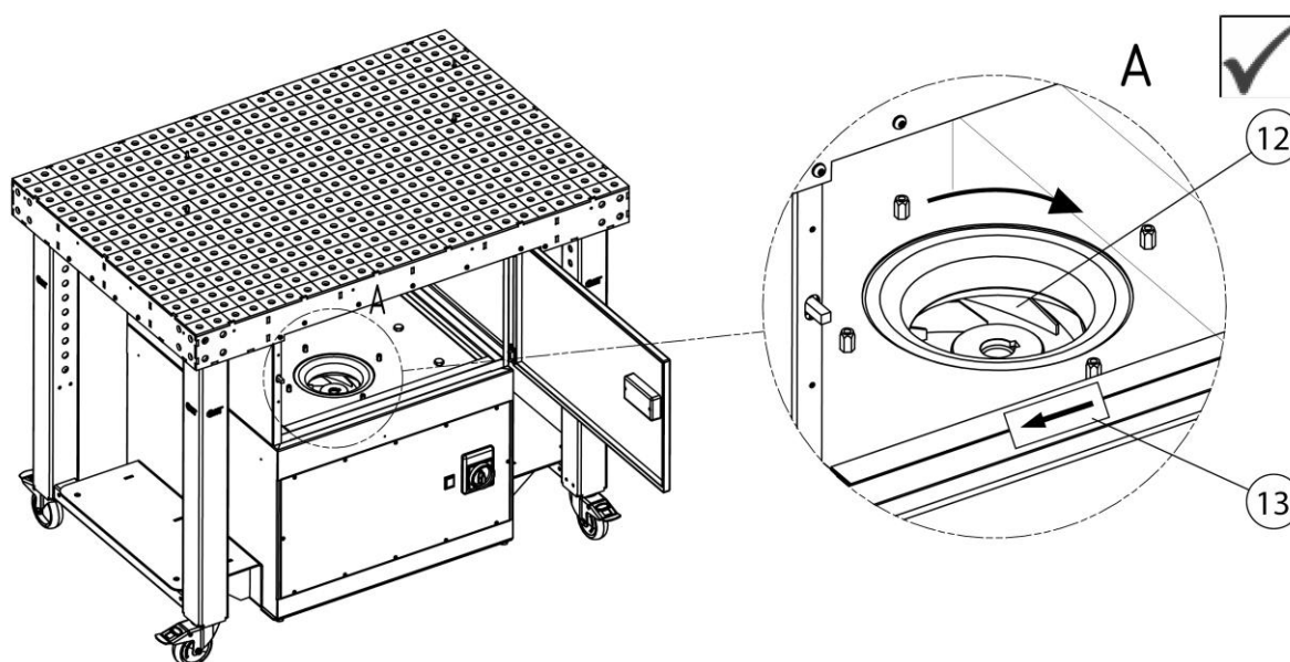
Fig. 45 : Contrôle du sens de rotation de la roue à ailettes du ventilateur
