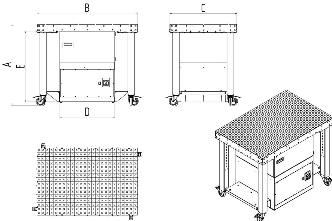
Obr. 135: Rozměrový výkres
