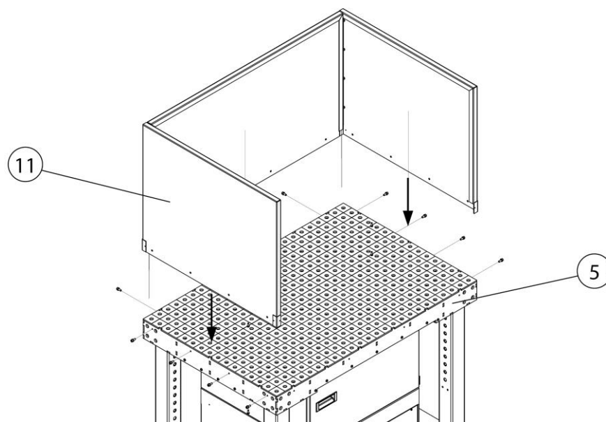
Rys. 145: Montaż – ścianka boczna (opcja)
