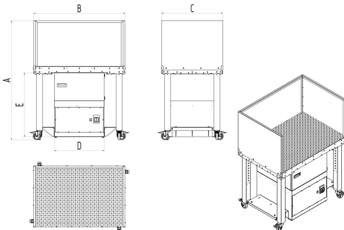
Рис. 170: Габаритный чертеж с боковой стенкой
