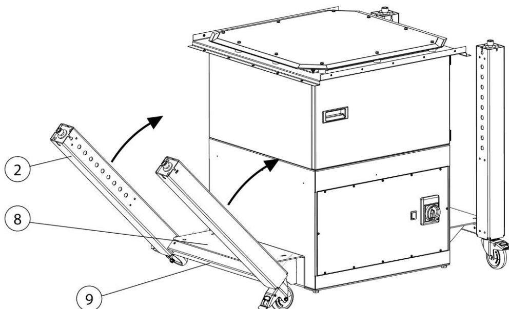
Rys. 142: Montaż – nogi stołu
