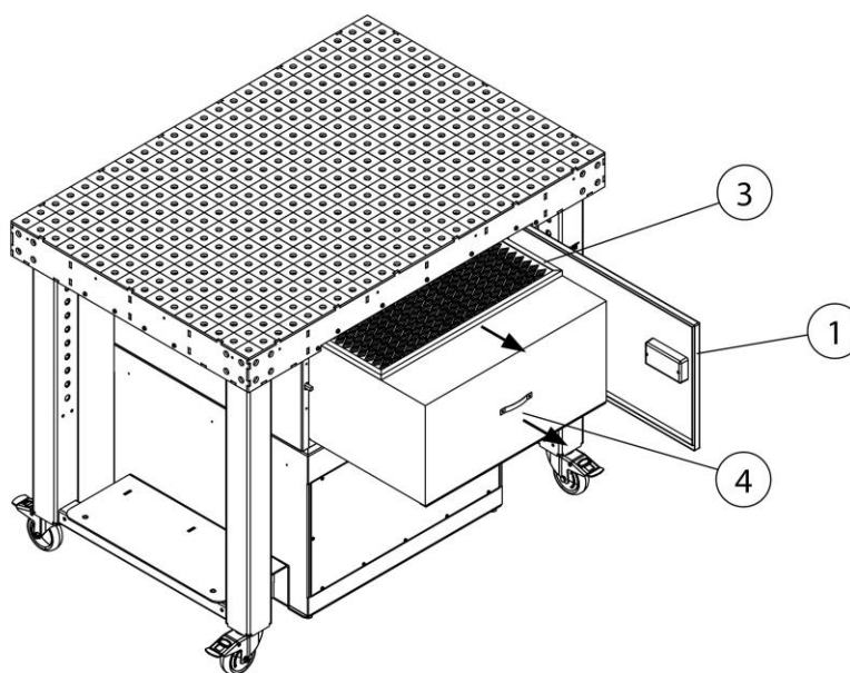
Fig. 115: Sostituzione filtro - prefiltro + filtro principale
