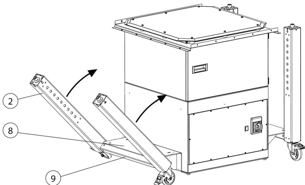
Fig. 108: Montaggio - Gambe del tavolo
