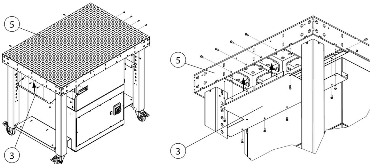
Abb. 8: Montage - Staubwanneblech
