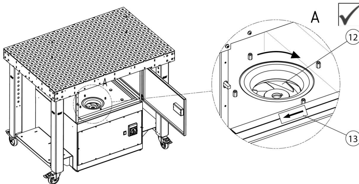
Рис. 164: Проверка направления вращения крыльчатки вентилятора
