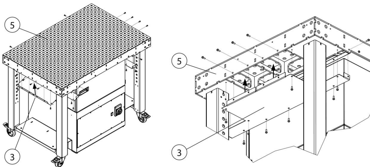
Рис. 161: Монтаж – ванна для пыли
