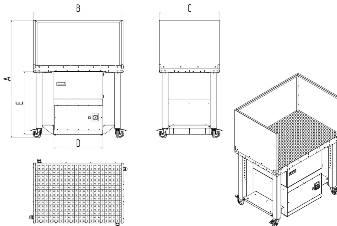
Rys. 153: Karta wymiarów ze ścianką boczną
