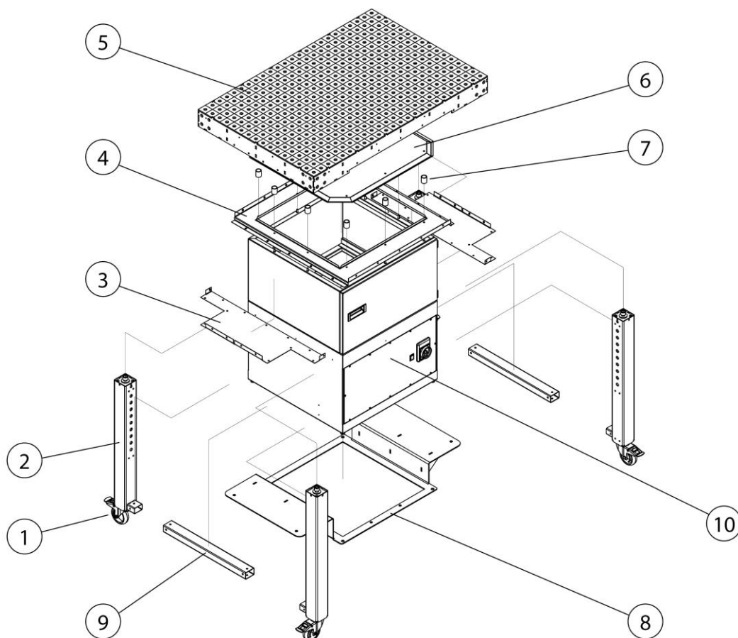
Рис. 155: Монтаж – обзор компонентов
