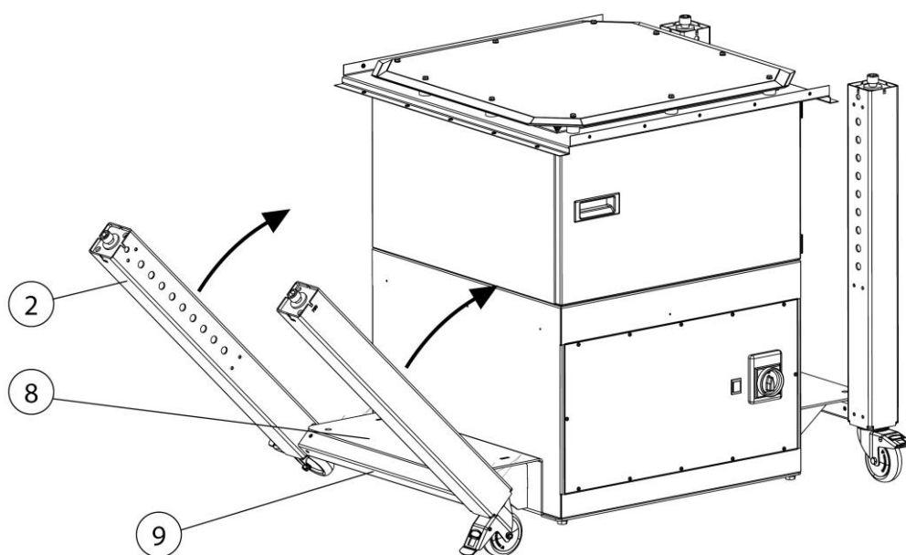
Obr. 125: Montáž – nohy stolu
