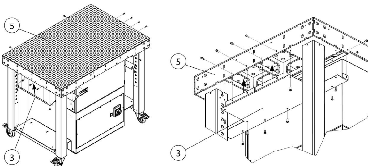
Fig. 42 : Montage - Plaque de récupération des poussières
