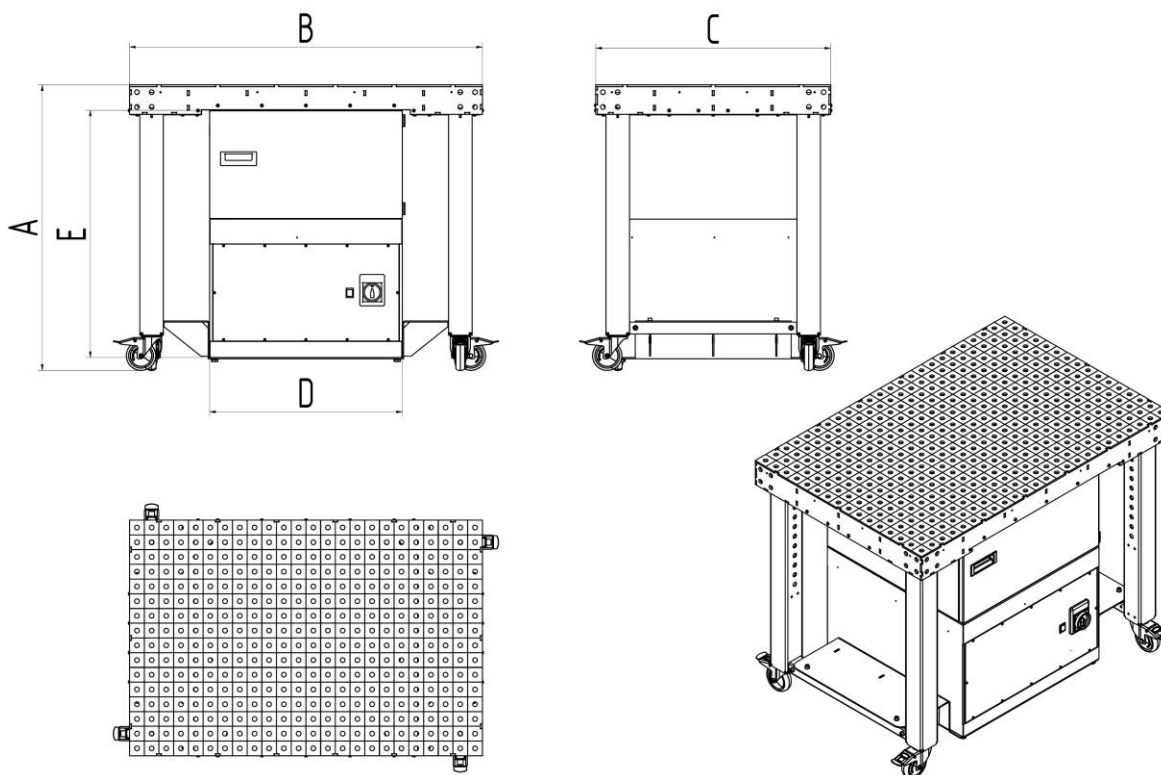
Fig. 101: Folha de dimensões
