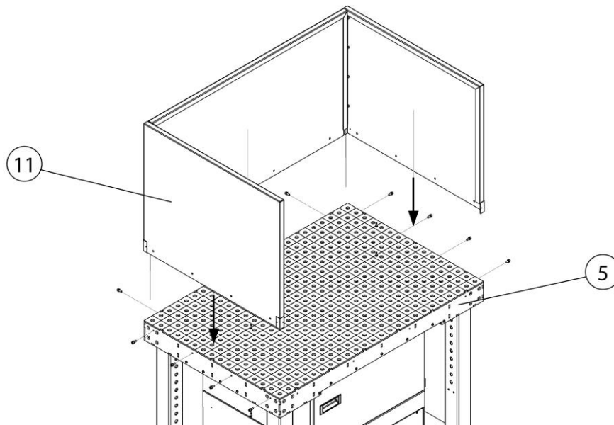
Fig. 94: Montagem – Parede lateral (opcional)
