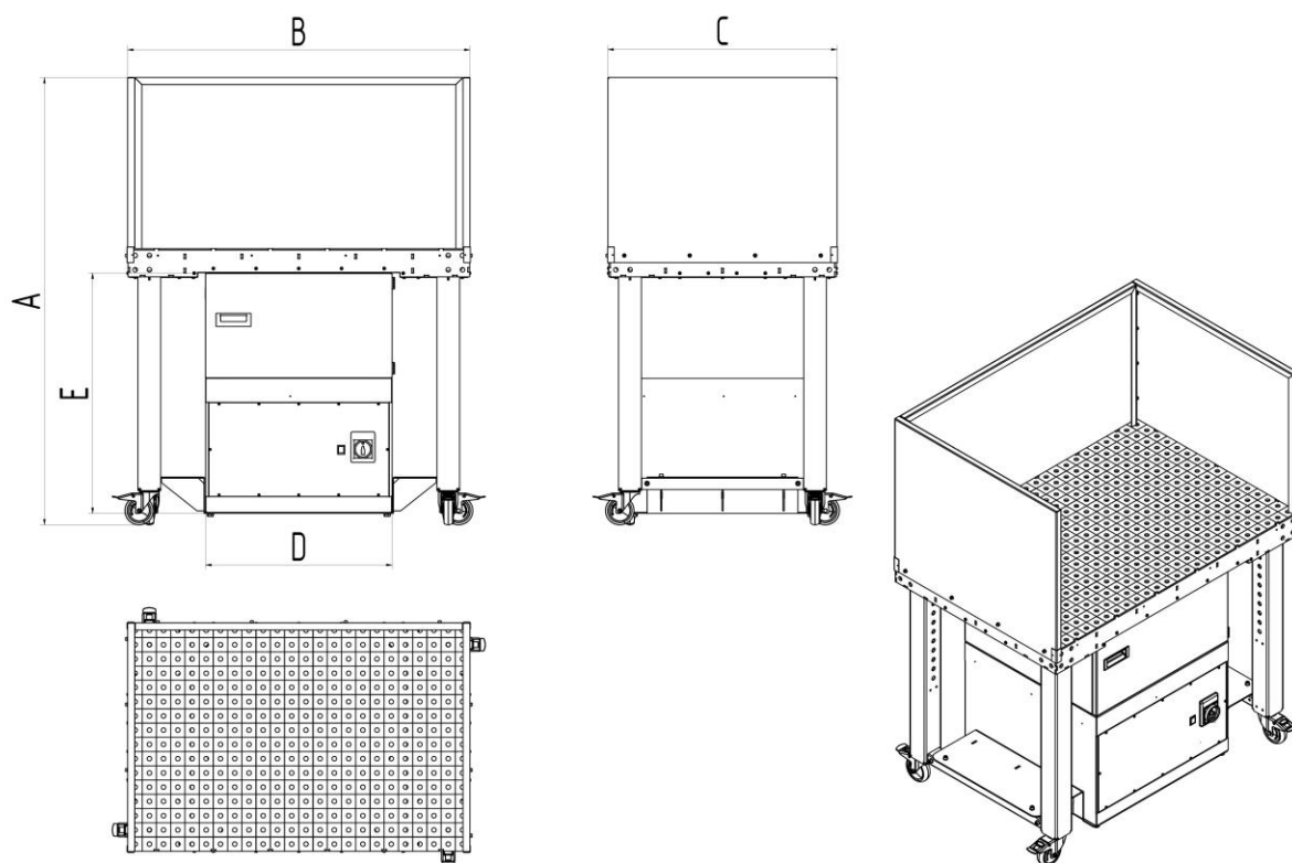
Fig. 119: Disegno quotato con parete laterale
