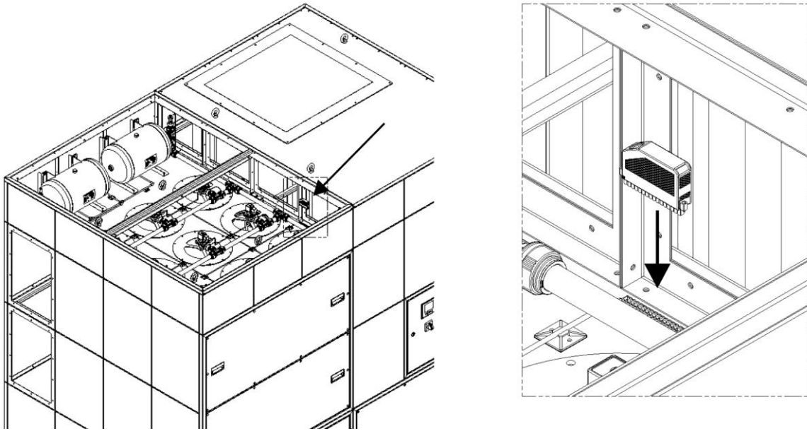
Afb. 96: Montage groene stekker
