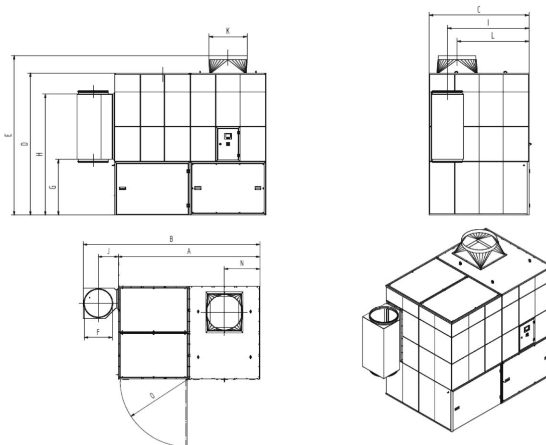
Fig. 365: Disegno quotato 34110
