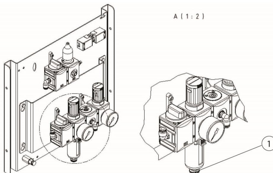
Fig. 286: Válvula de drenagem de condensado da unidade de manutenção de ar comprimido
