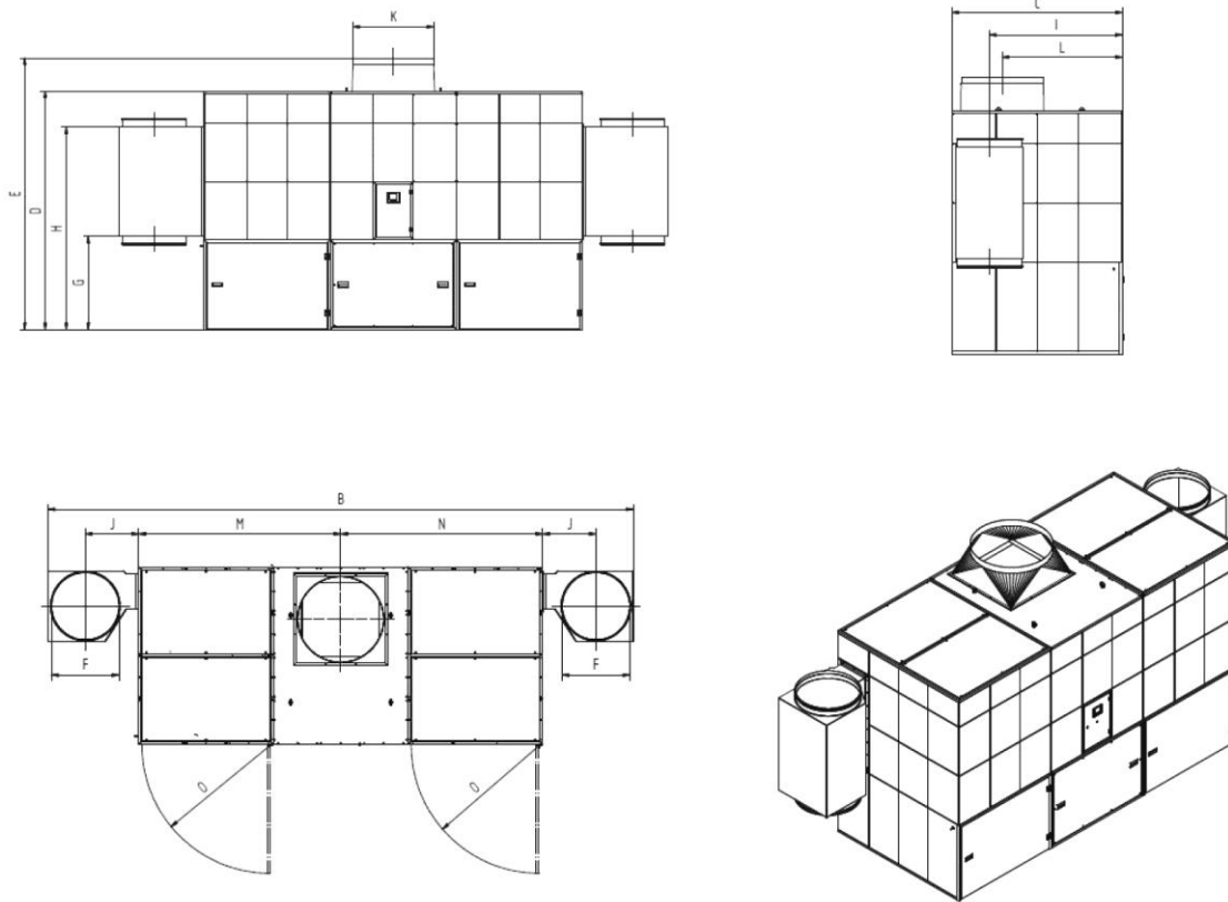
Afb. 146: Maatblad 34180
