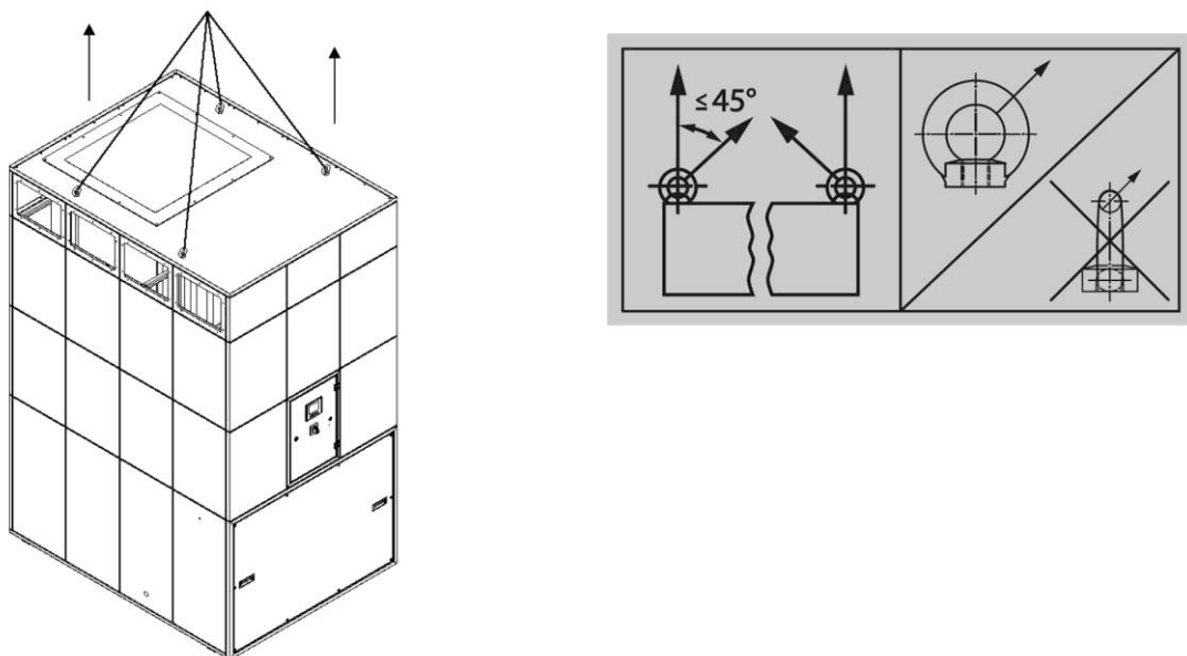
Fig. 158: Elevación del ventilador con grúa
