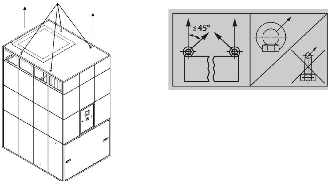
Fig. 306: Sollevamento gruppo ventilatore con gru
