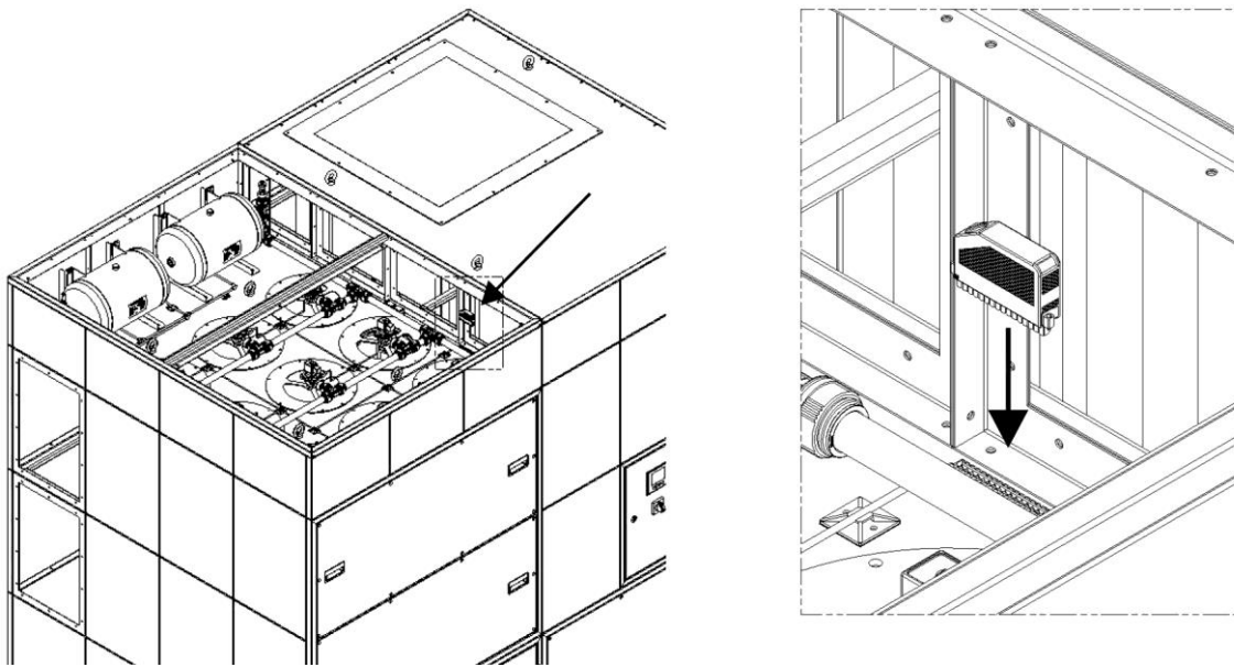
Fig. 318: Montaggio spina verde
