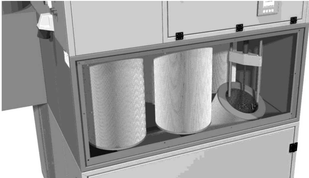
Fig. 284: Substituição do filtro - retirar os cartuchos filtrantes
