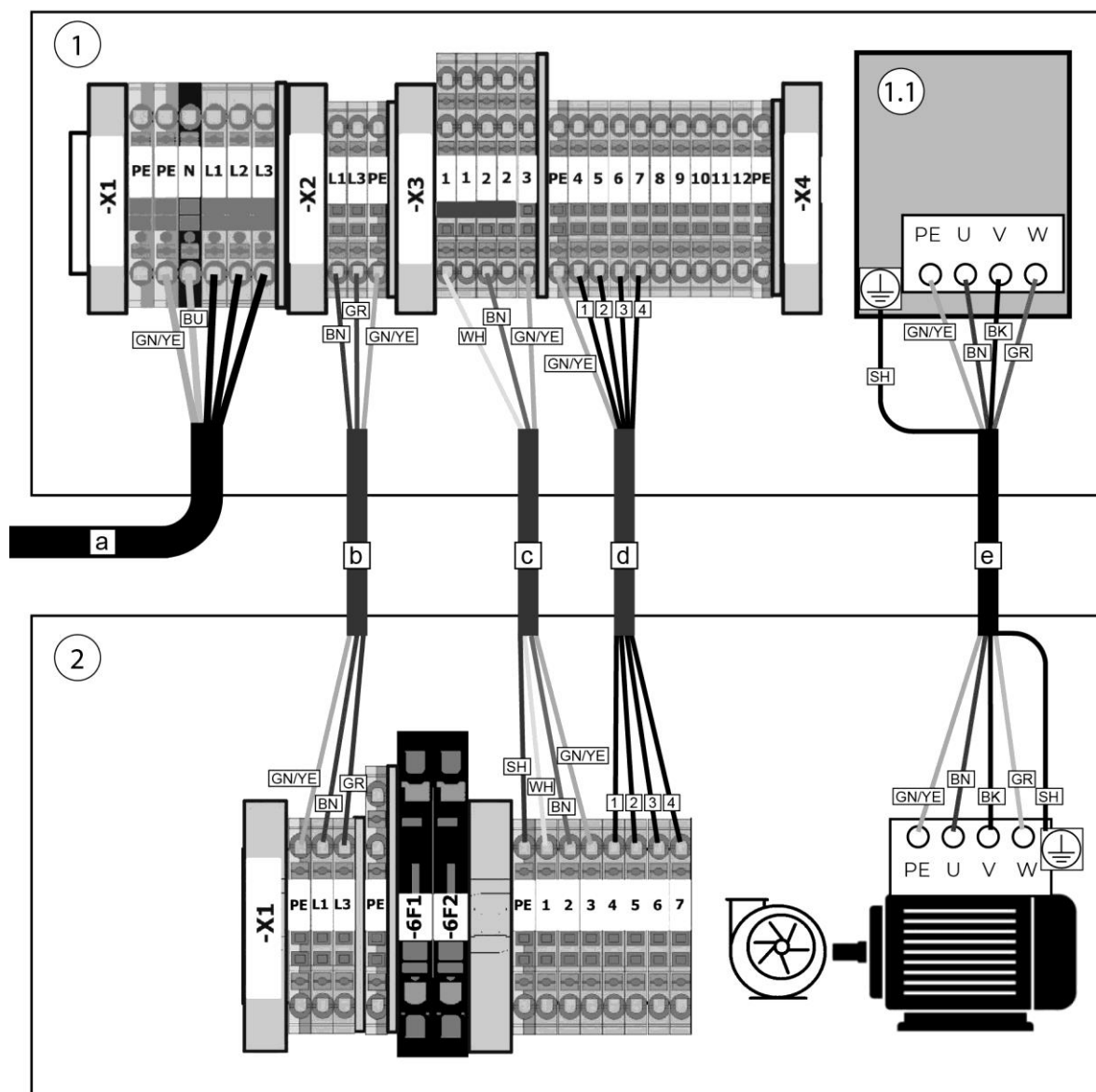
Fig. 183: Esquema de cableado regulación de la potencia de aspiración con producto
