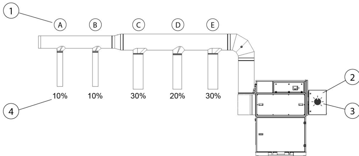
Fig. 350: Impostazione della regolazione della potenza di aspirazione
