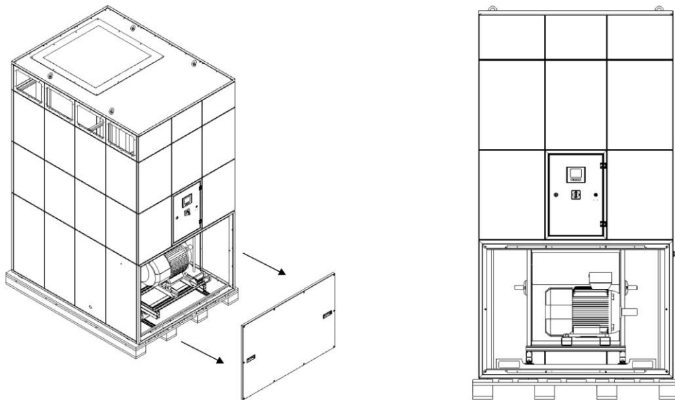
Afb. 83: Onderhoudsdeur van het ventilatordeel openen
