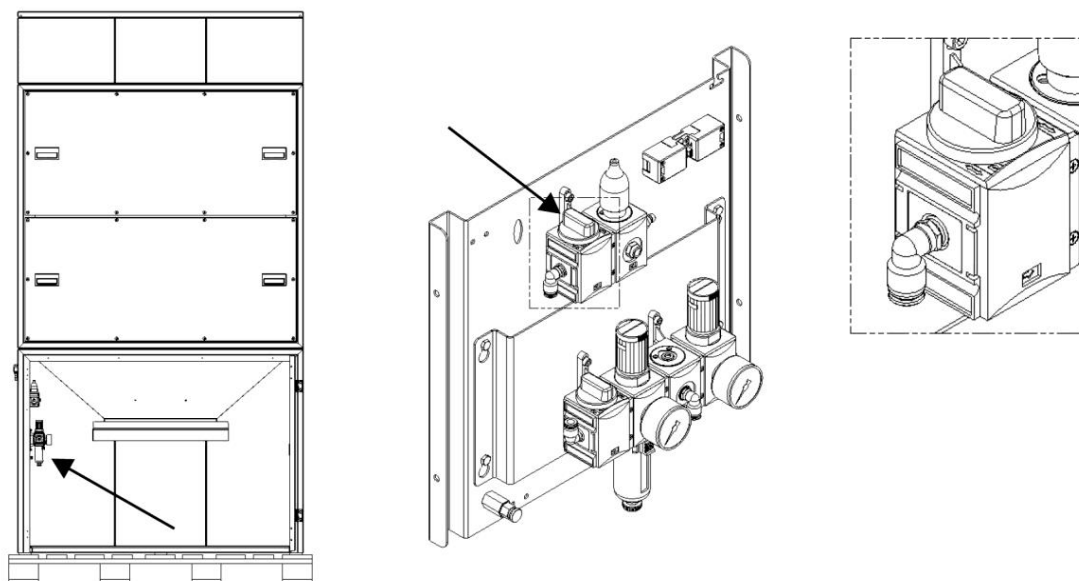
Fig. 236: Válvula de abaixamento recipiente coletor de pó
