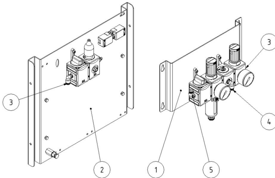
Fig. 179: Unidad de aire comprimido
