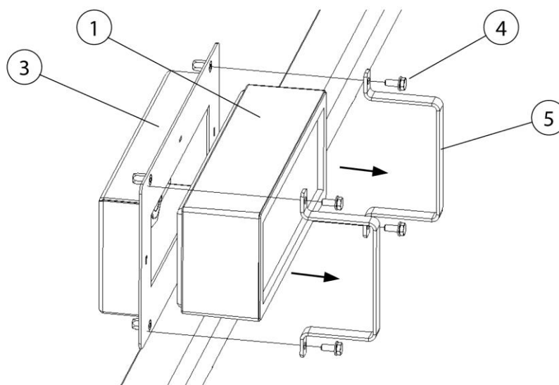
Fig. 281: Substituição do filtro de segurança
