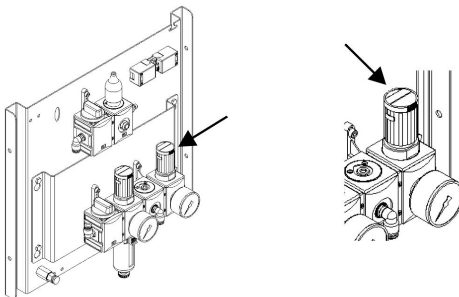
Fig. 326: Regolazione pressione dispositivo di sollevamento/collettore di polvere
