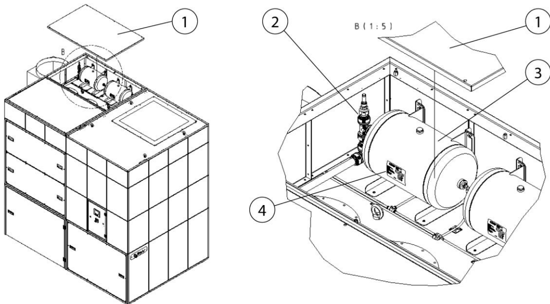
Afb. 141: Toegang tot persluchtreservoir + veiligheidsklep
