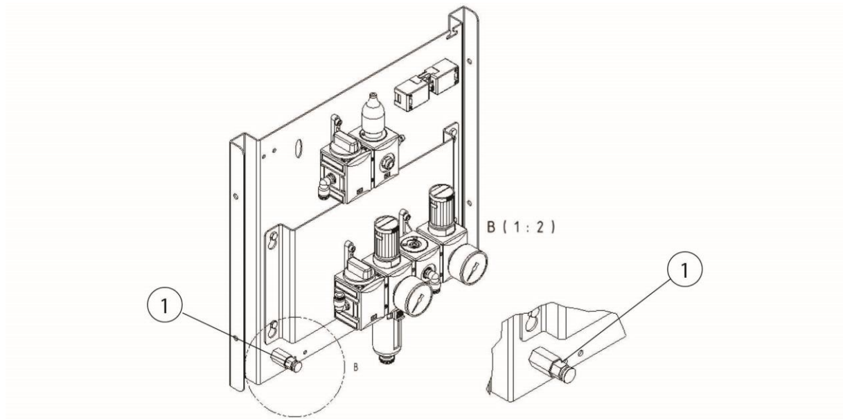
Fig. 63 : soupape de vidange des condensats réservoir d'air comprimé
