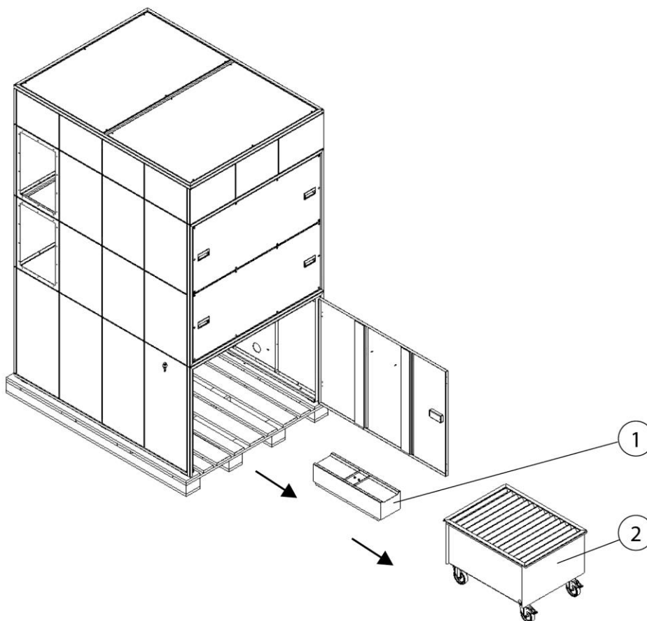
Afb. 90: Verwijder het stofopvangreservoir en de hijsinstallatie
