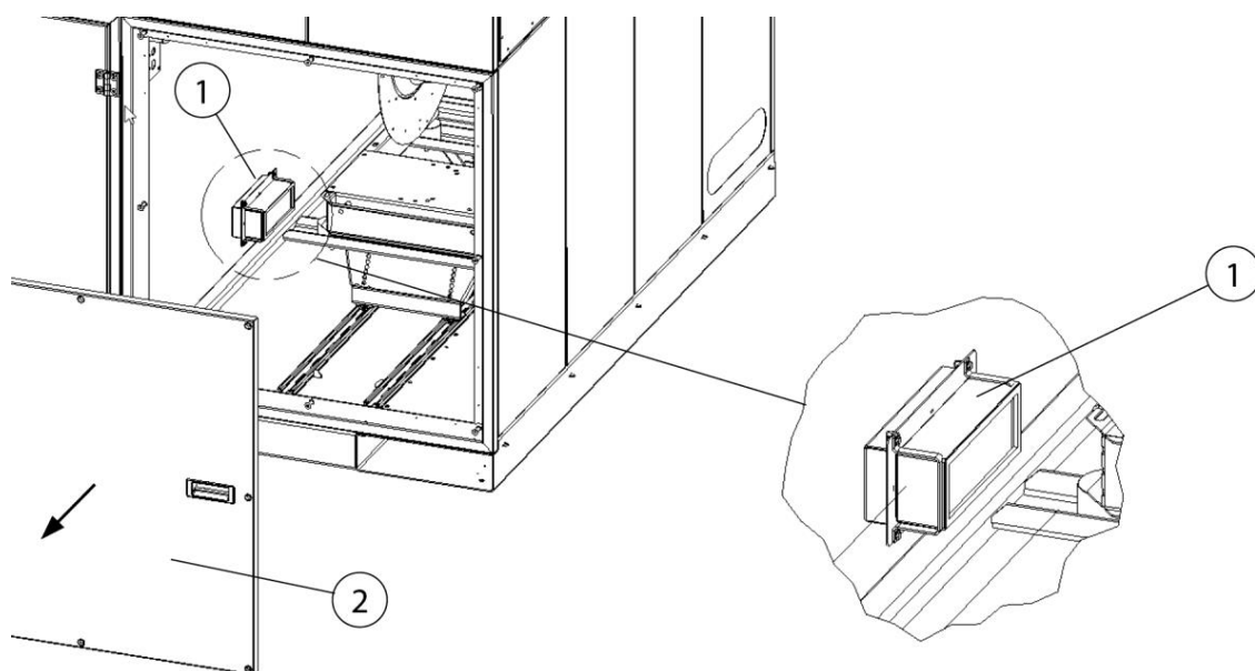
Fig. 206: Acceso al filtro de seguridad
