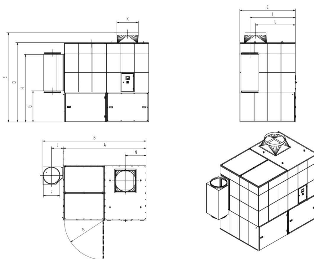
Fig. 70 : fiche dimensionnelle 34130
