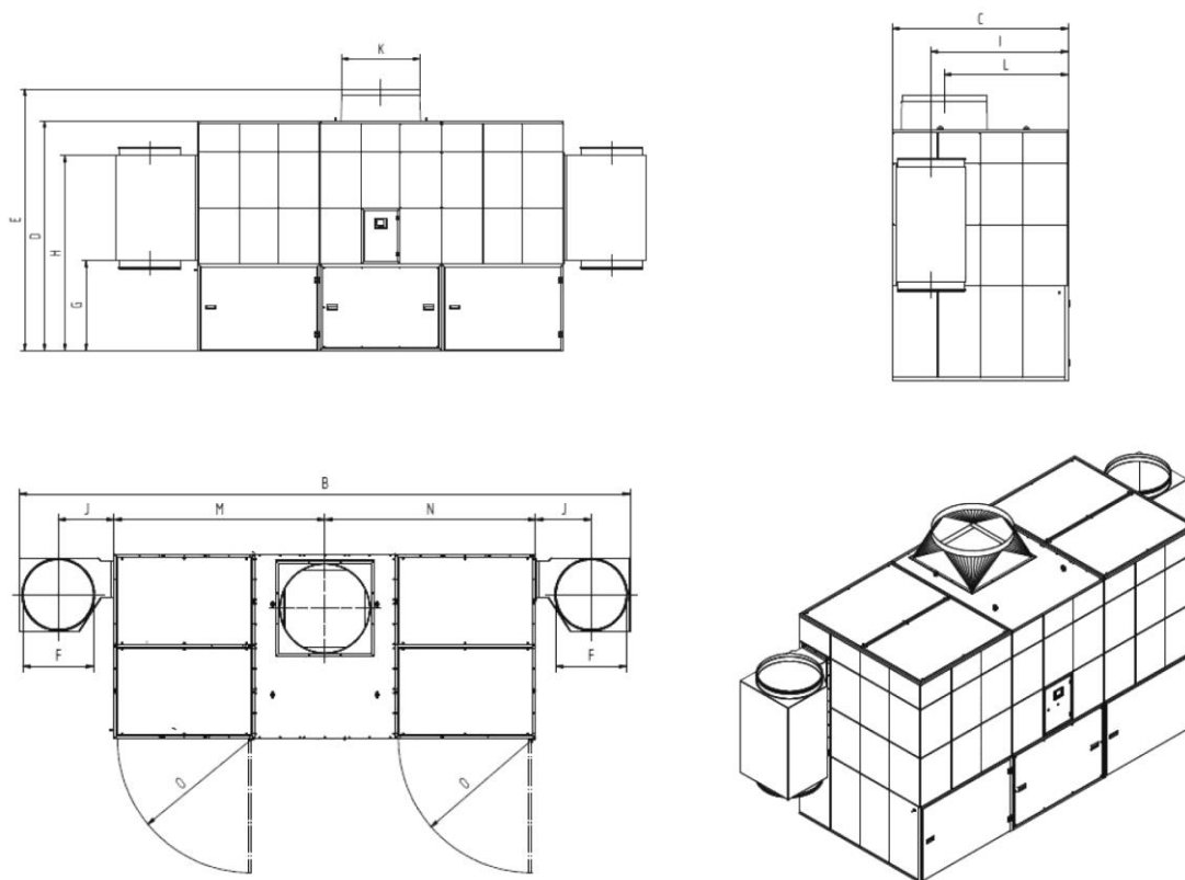
Fig. 293: Folha de dimensões 34160
