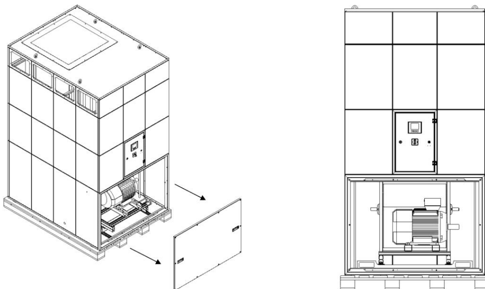
Fig. 305: Apertura porta di manutenzione del gruppo ventilatore
