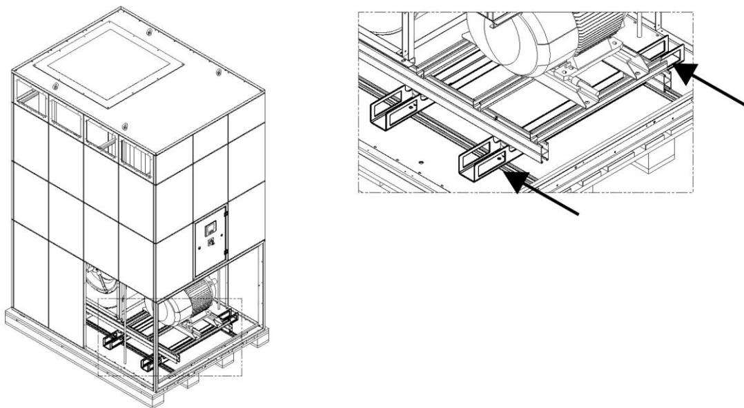
Fig. 307: Sollevamento gruppo ventilatore con carrello elevatore a forche
