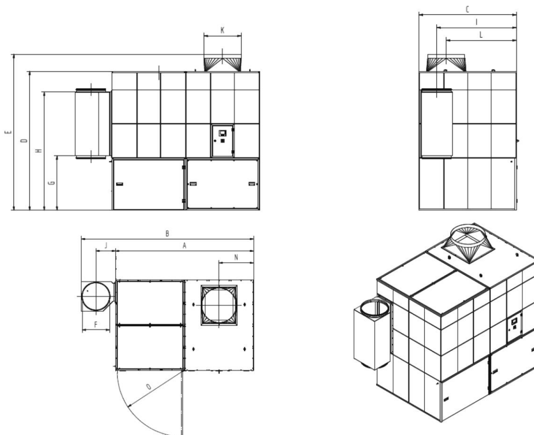
Fig. 291: Folha de dimensões 34110
