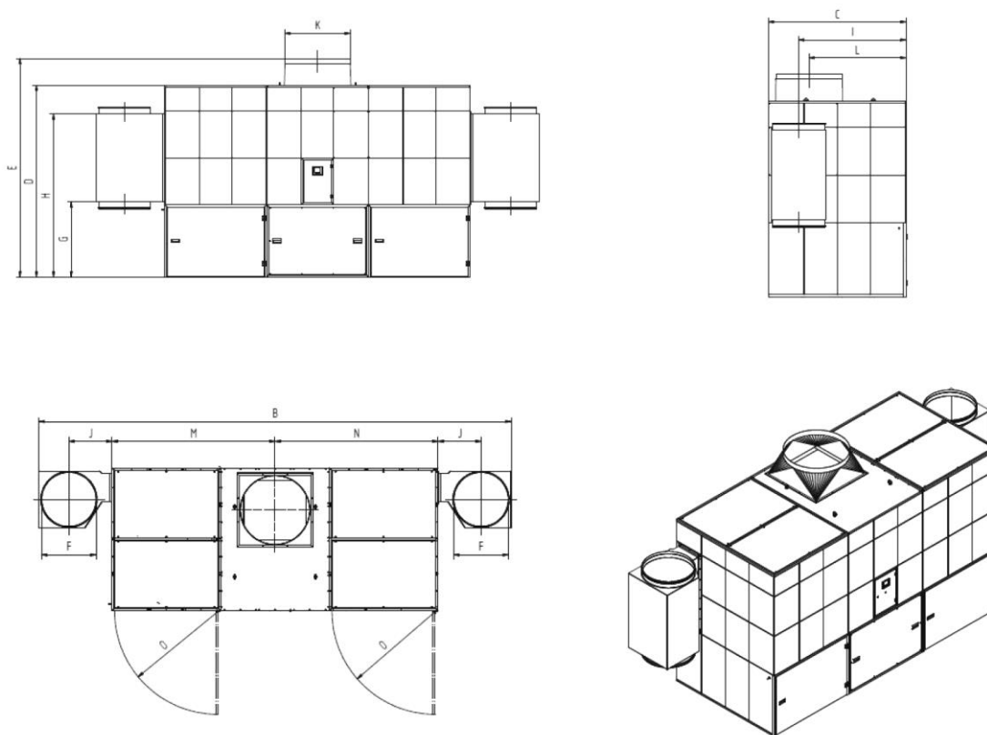
Fig. 72 : fiche dimensionnelle 34180
