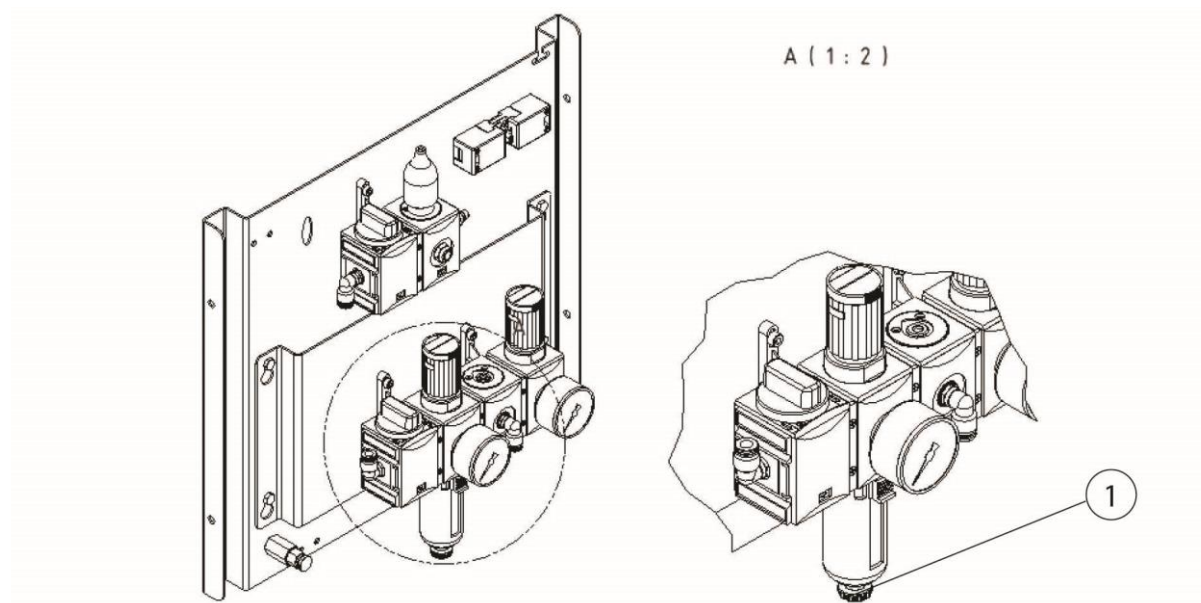
Fig. 64 : soupape de vidange des condensats unité de maintenance d'air comprimé
