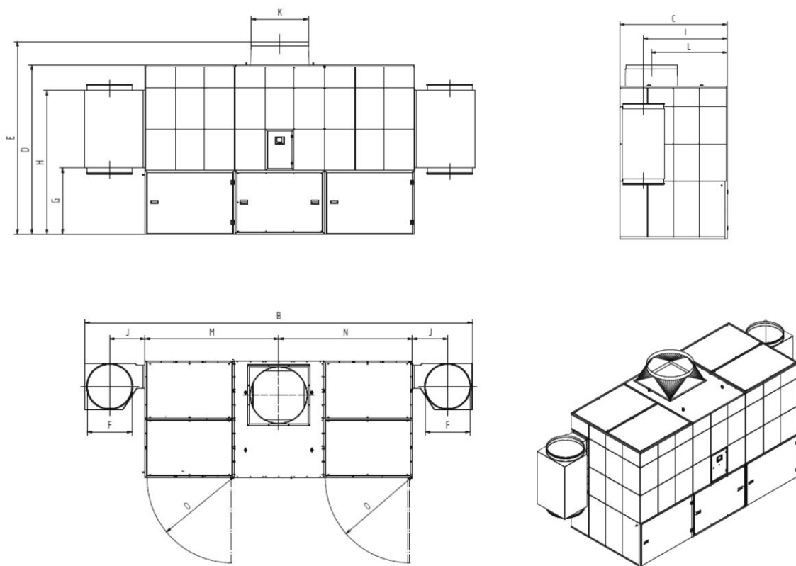
Fig. 369: Disegno quotato 34200 + 34220
