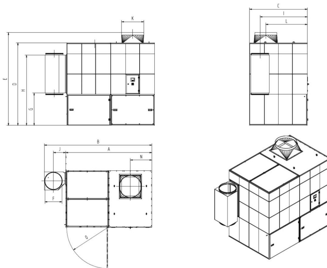
Afb. 144: Maatblad 34130
