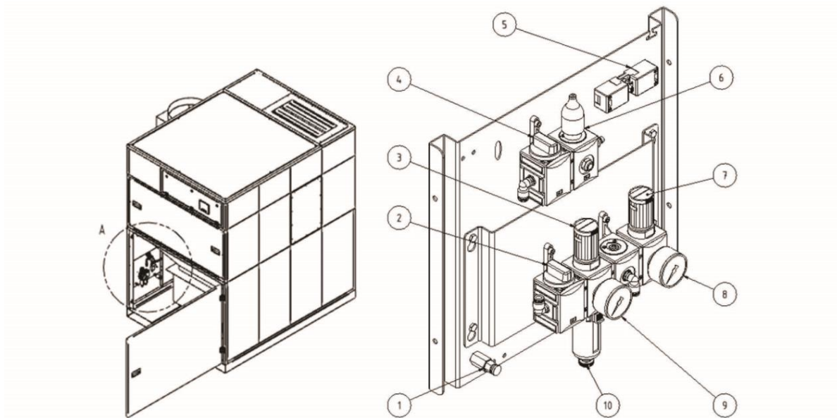
Fig. 175: Unidad de aire comprimido
