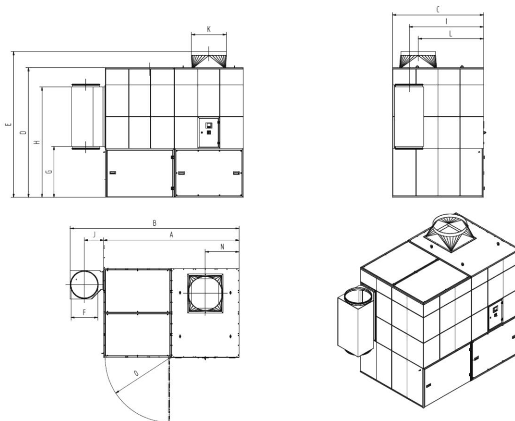
Fig. 366: Disegno quotato 34130
