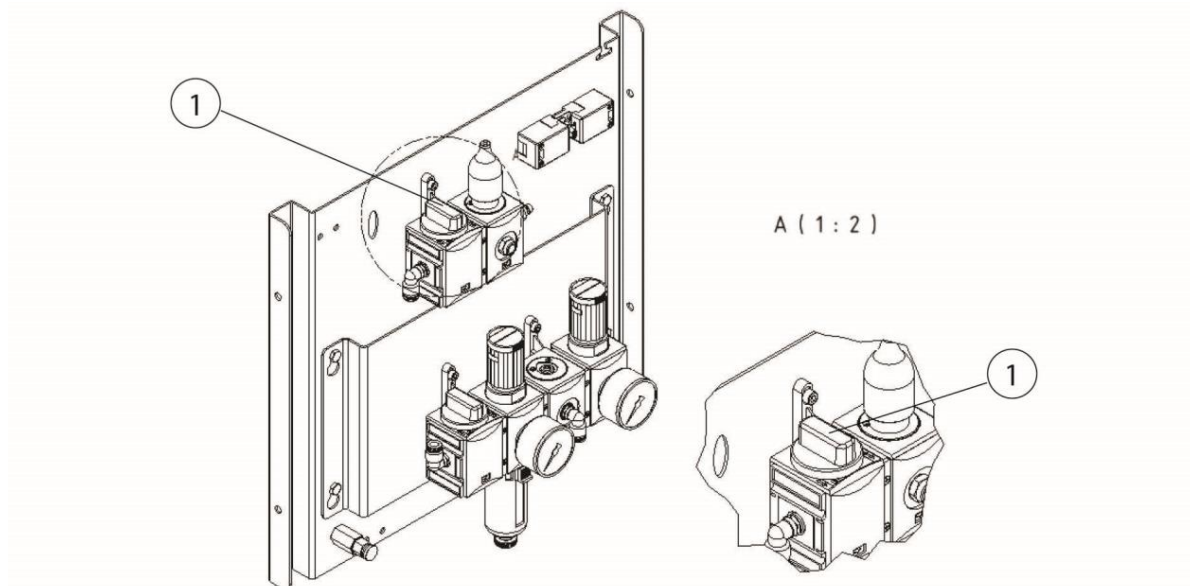
Fig. 351: Valvola pneumatica collettore di polvere
