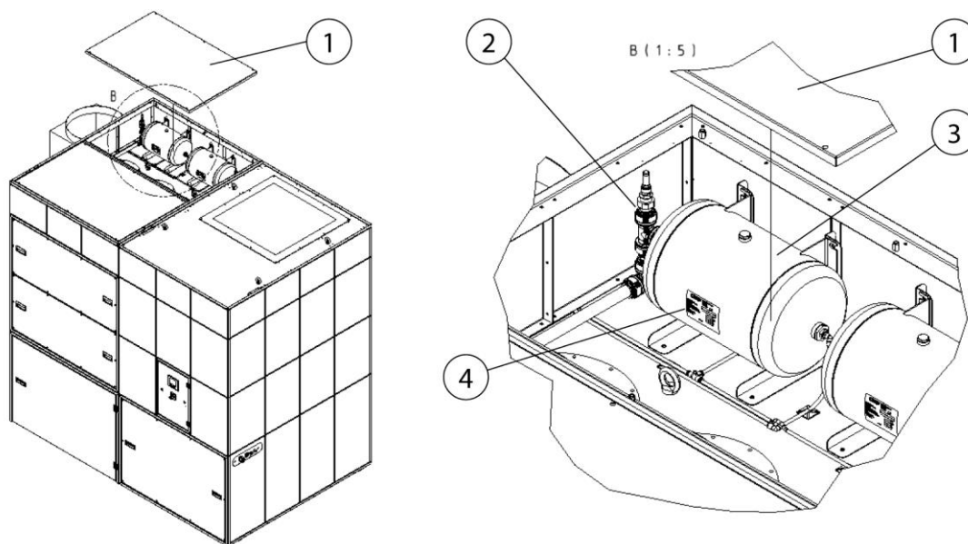
Fig. 67 : Accès au réservoir d'air comprimé + vanne de sécurité
