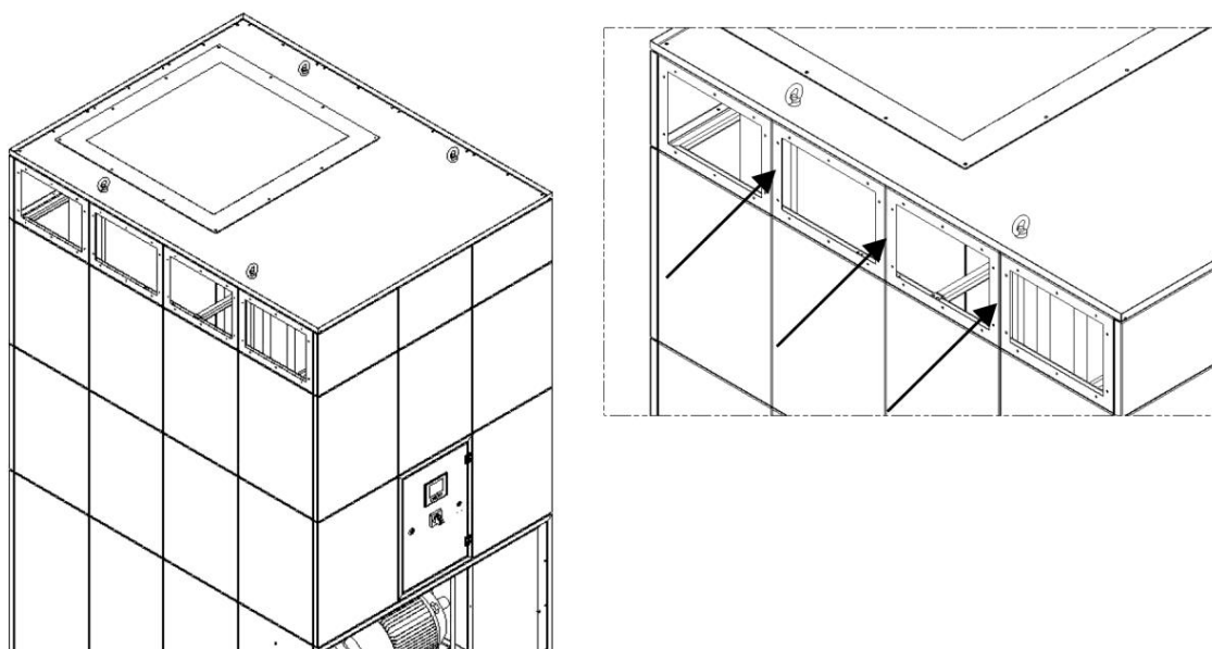
Fig. 160: Paso del aire limpio
