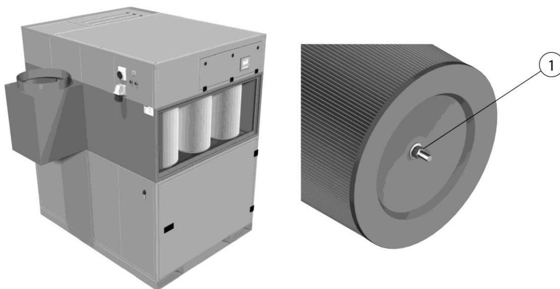
Fig. 356: Sostituzione del filtro – Coperchio di manutenzione
