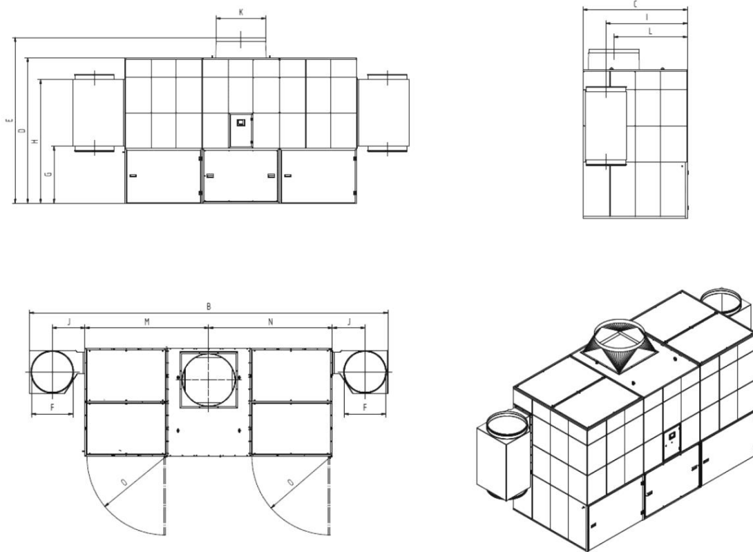
Fig. 220: Hoja de dimensiones 34180
