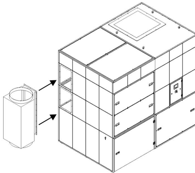
Afb. 100: Montage aansluitkast aan zuigzijde
