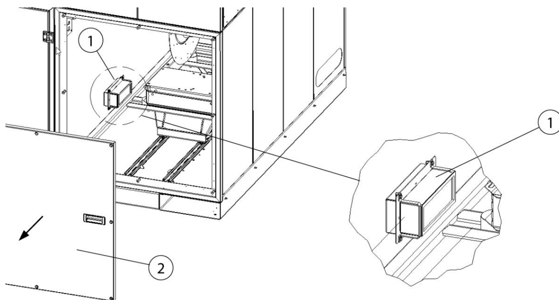
Fig. 280: Acesso ao filtro de segurança
