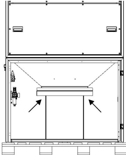
Fig. 167: Elevación del módulo del filtro con una carretilla elevadora
