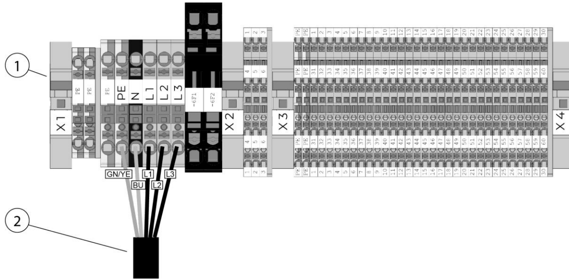
Afb. 106: Aansluitklemmenstrook schakelkast product
