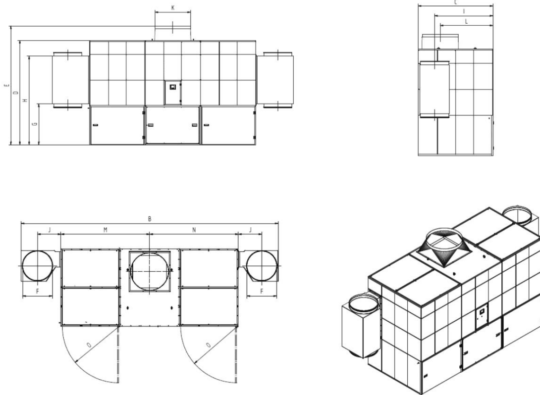
Fig. 368: Disegno quotato 34180
