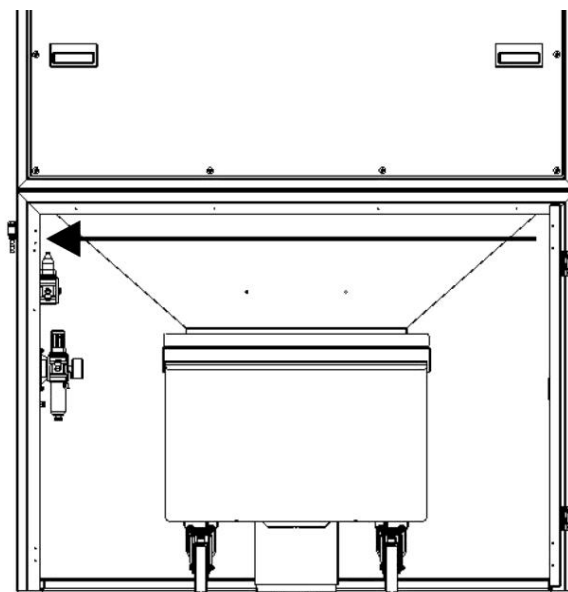
Fig. 247: Colocação de cabos por calha técnica
