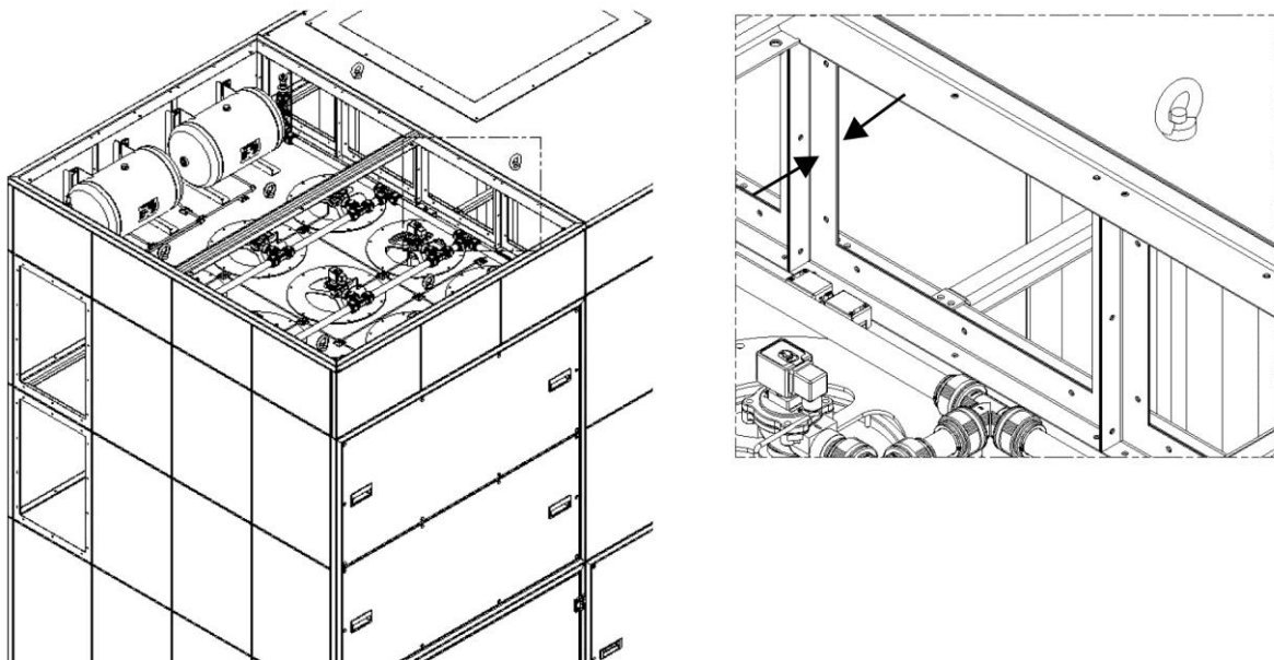
Afb. 95: Ventilatordeel met filterdeel verbinden
