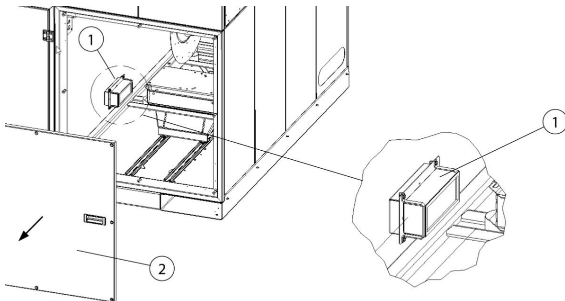
Fig. 354: Accesso al filtro di sicurezza
