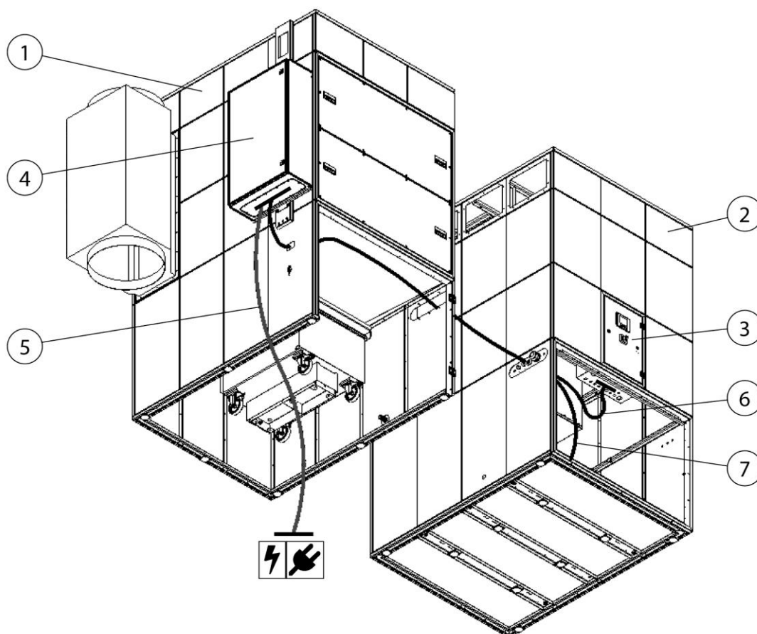
Fig. 181: Ejemplo: Cableado regulación de la potencia de aspiración
