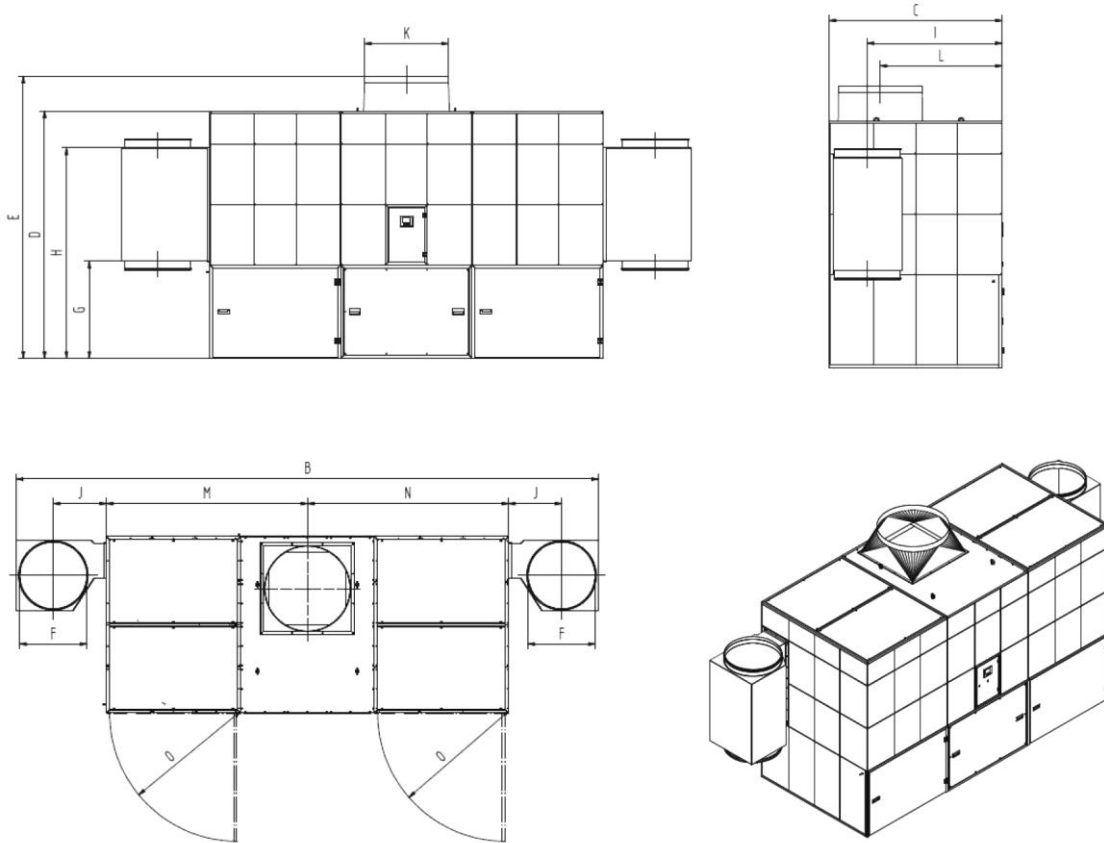
Afb. 148: Maatblad 34240 + 34270
