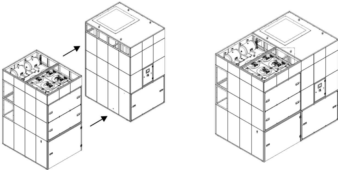
Afb. 94: Filterdeel met ventilatordeel verbinden
