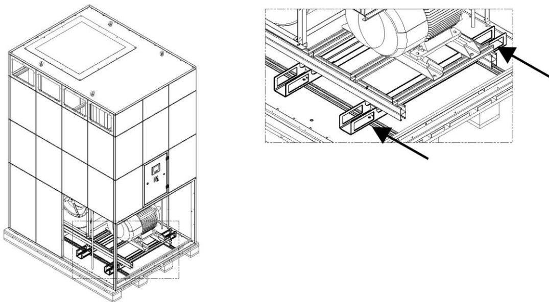
Fig. 233: Elevação do ventilador com empilhadora
