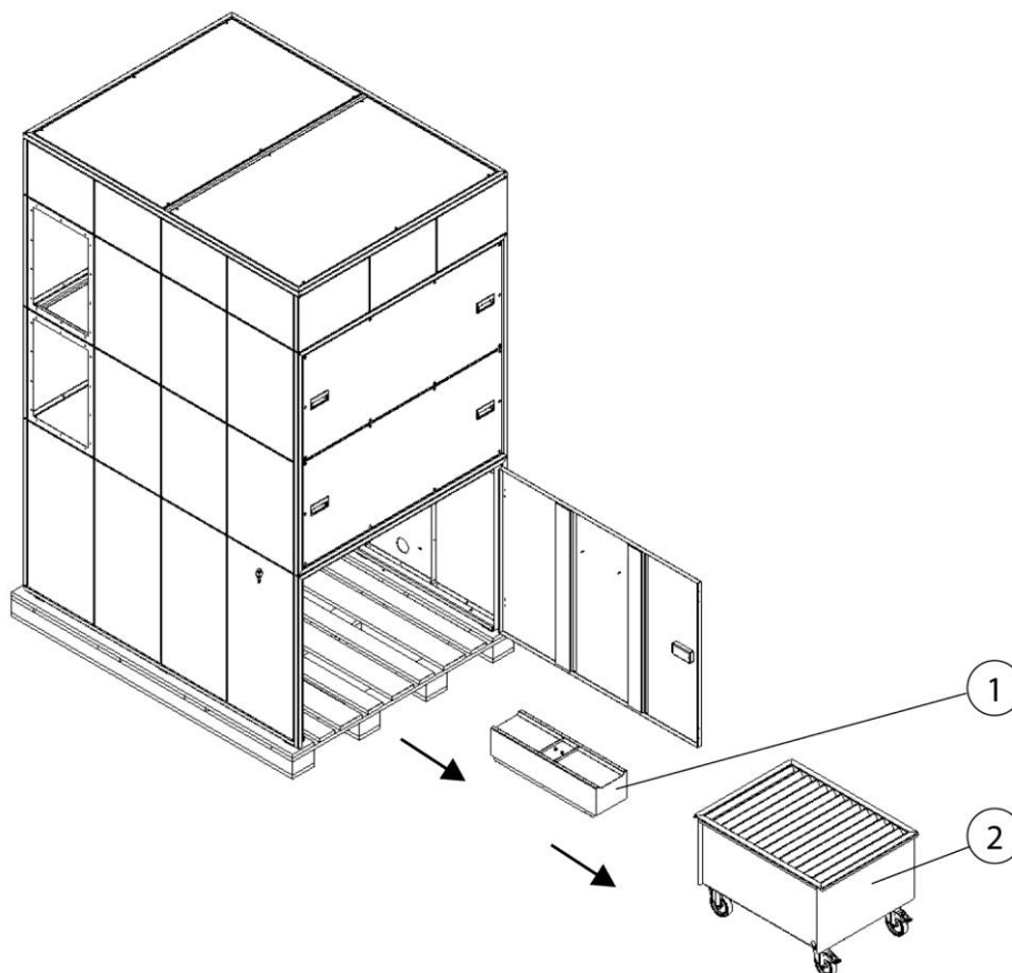
Fig. 312: Rimozione del collettore di polvere e del dispositivo di sollevamento
