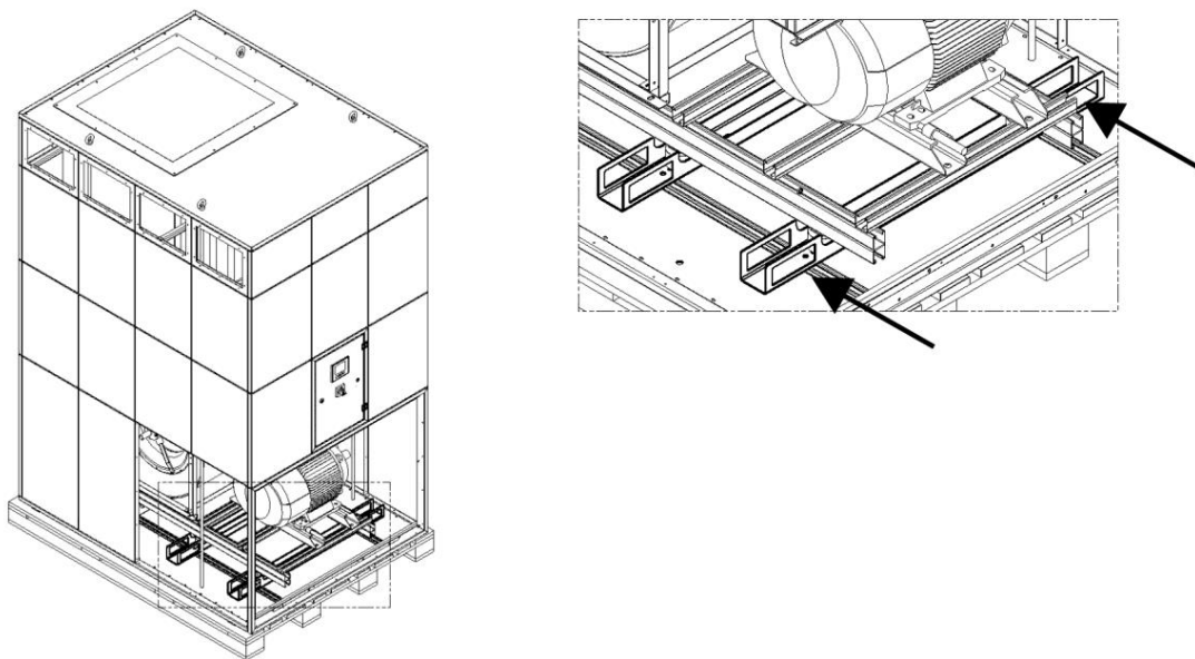
Fig. 159: Elevación del módulo del ventilador con una carretilla elevadora
