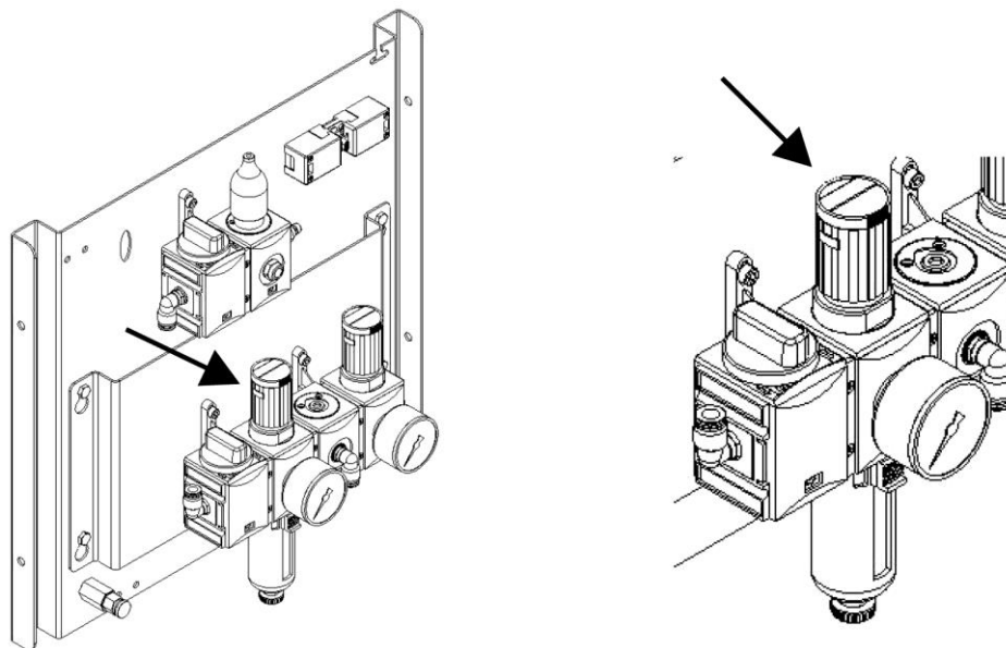
Fig. 177: Ajuste de la presión de servicio
