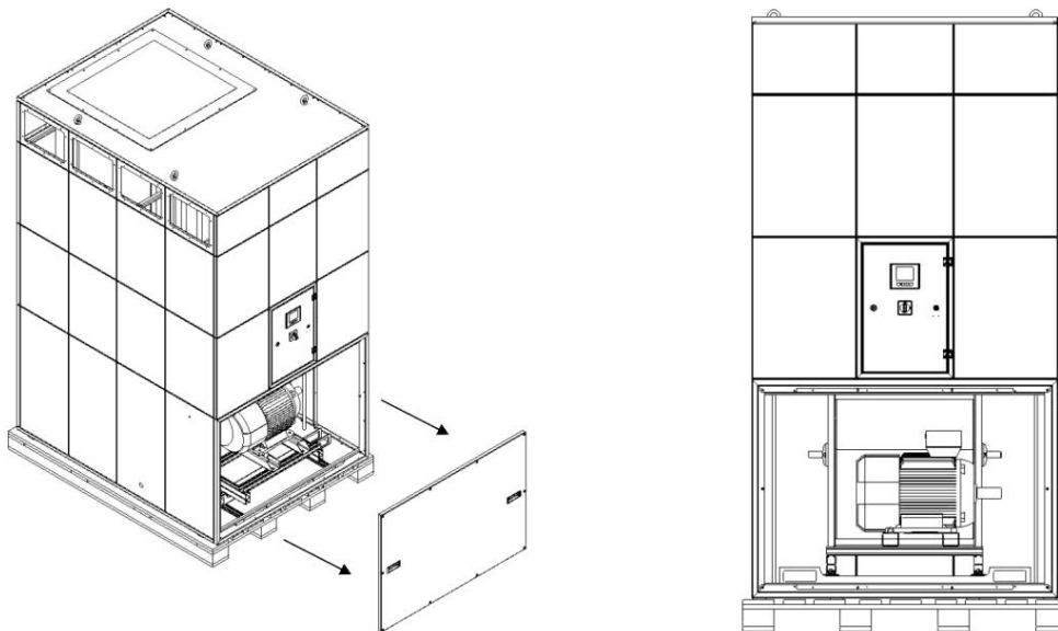
Fig. 157: Abra la puerta de mantenimiento del ventilador
