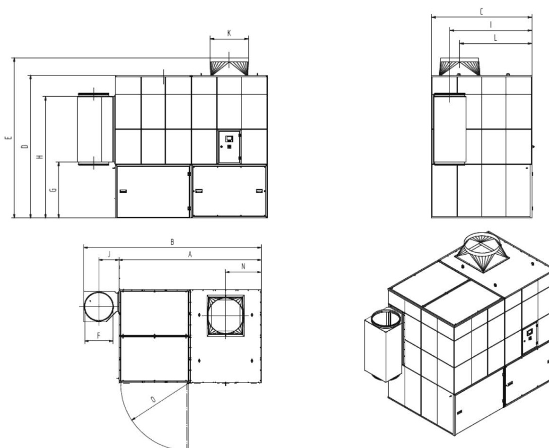
Fig. 69 : fiche dimensionnelle 34110
