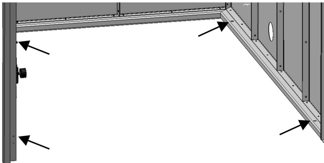
Fig. 171: Fijación del módulo del filtro al suelo
