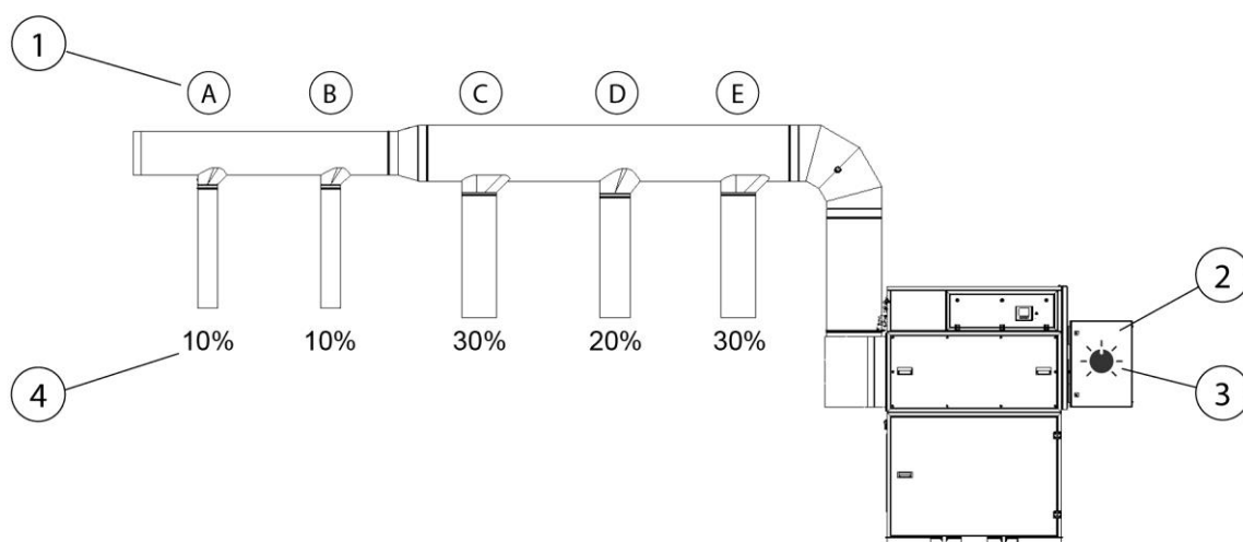
Afb. 128: Instellen van de zuigvermogensregeling
