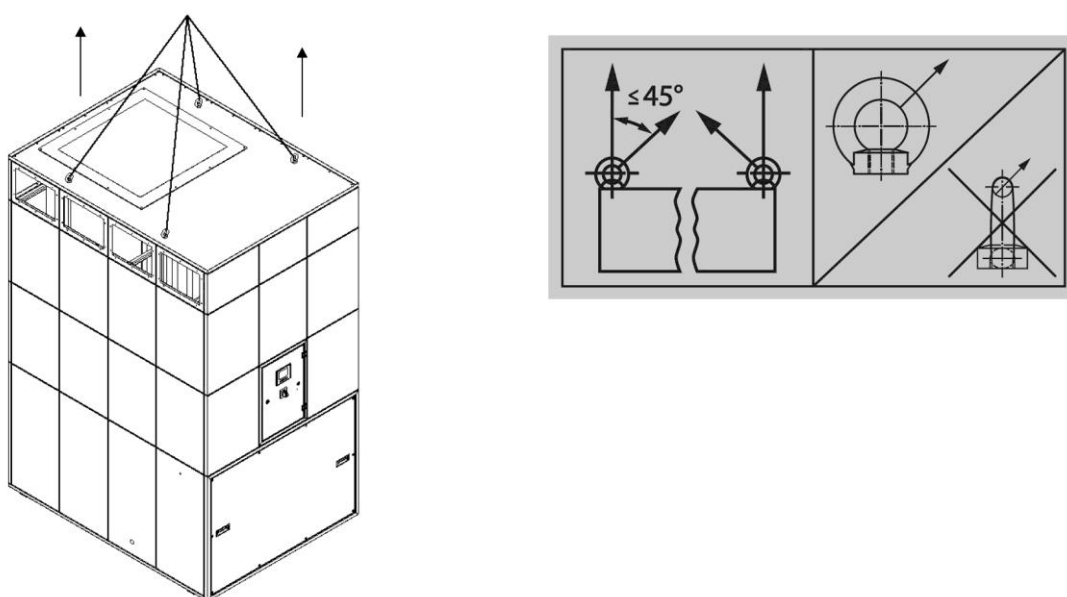
Fig. 314: Sollevamento gruppo filtro con gru
