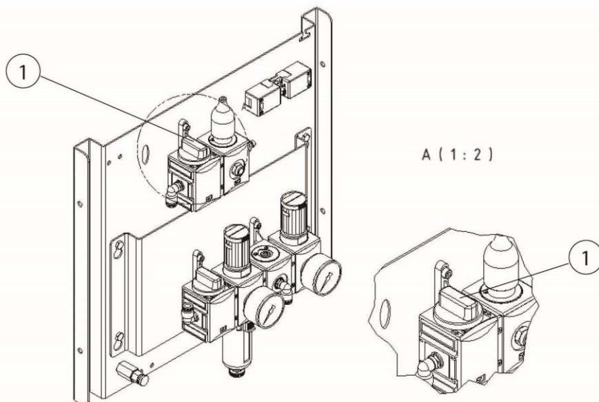
Fig. 203: Válvula de aire comprimido depósito colector de polvo
