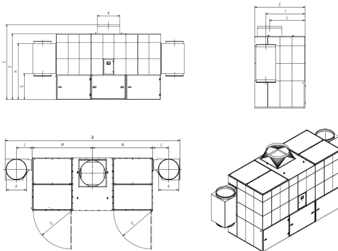
Afb. 145: Maatblad 34160
