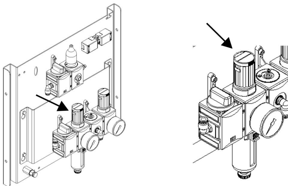
Fig. 251: Ajuste da pressão de serviço
