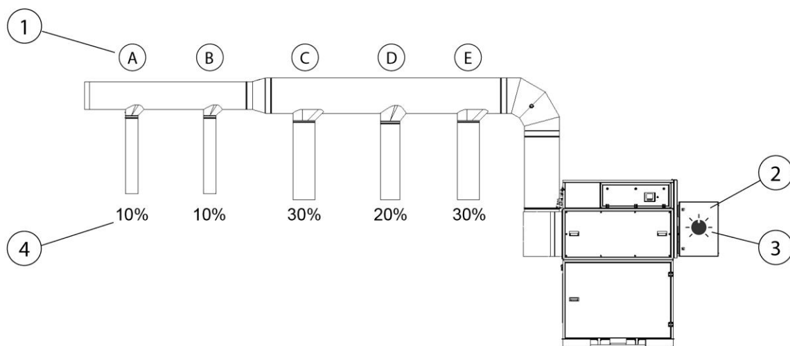
Fig. 202: Ajuste de la regulación de la potencia de aspiración
