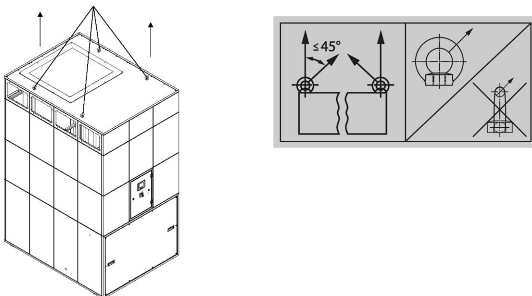
Fig. 232: Elevação do ventilador com grua
