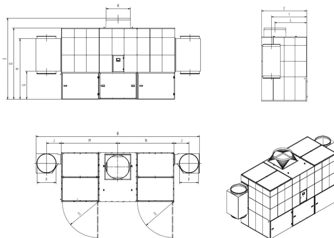
Fig. 295: Folha de dimensões 34200 + 34220
