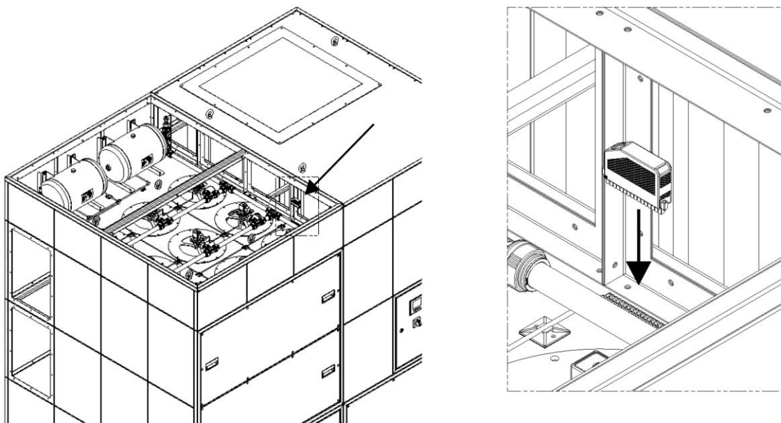
Fig. 170: Montaje de clavija verde
