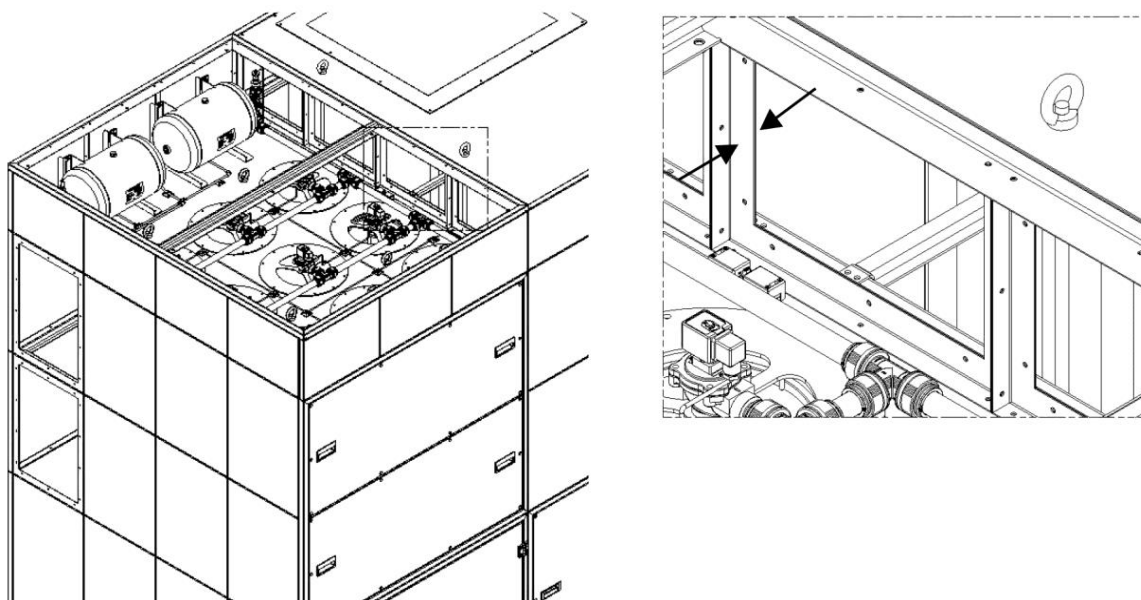
Fig. 243: Unir o ventilador ao filtro
