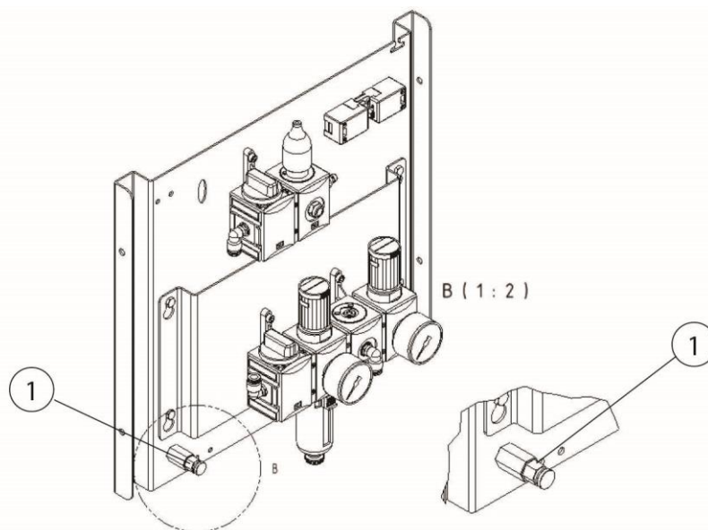
Fig. 285: Válvula de drenagem de condensado do reservatório de ar comprimido
