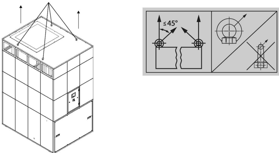
Afb. 84: Ventilatordeel met kraan hijsen
