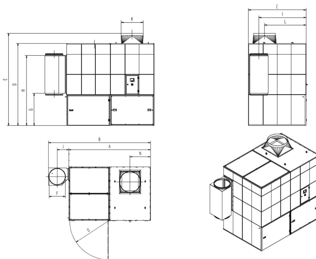
Afb. 143: Maatblad 34110
