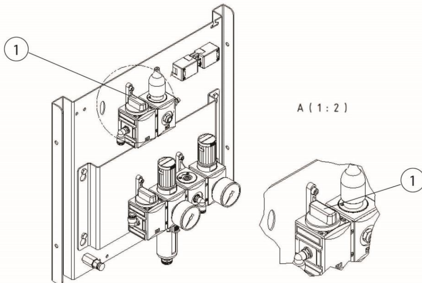
Fig. 277: Válvula de ar comprimido do recipiente coletor de pó
