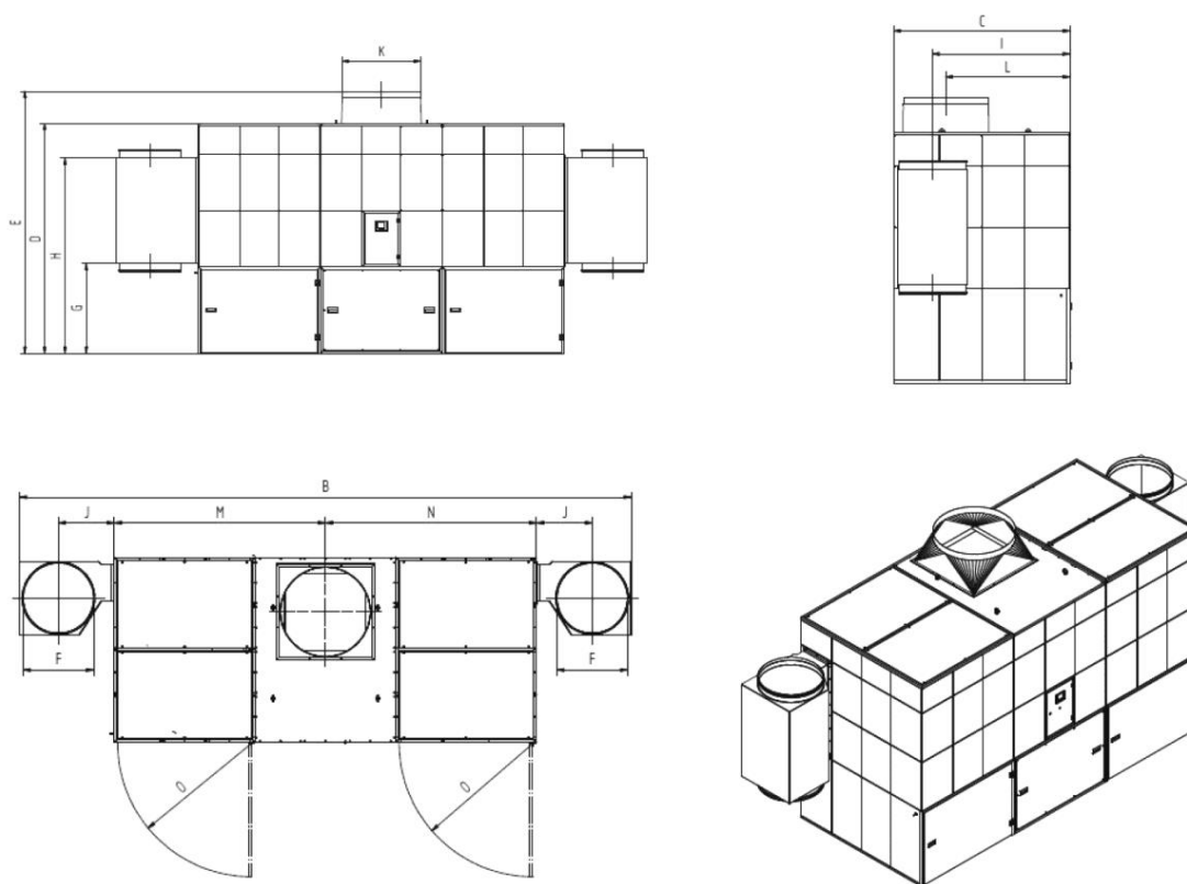
Fig. 71 : fiche dimensionnelle 34160
