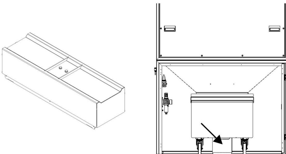
Fig. 172: Fijación del dispositivo de elevación al suelo
