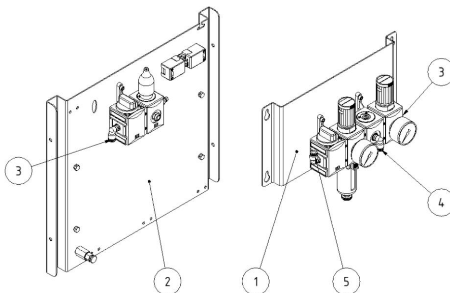
Fig. 253: Unidade de ar comprimido
