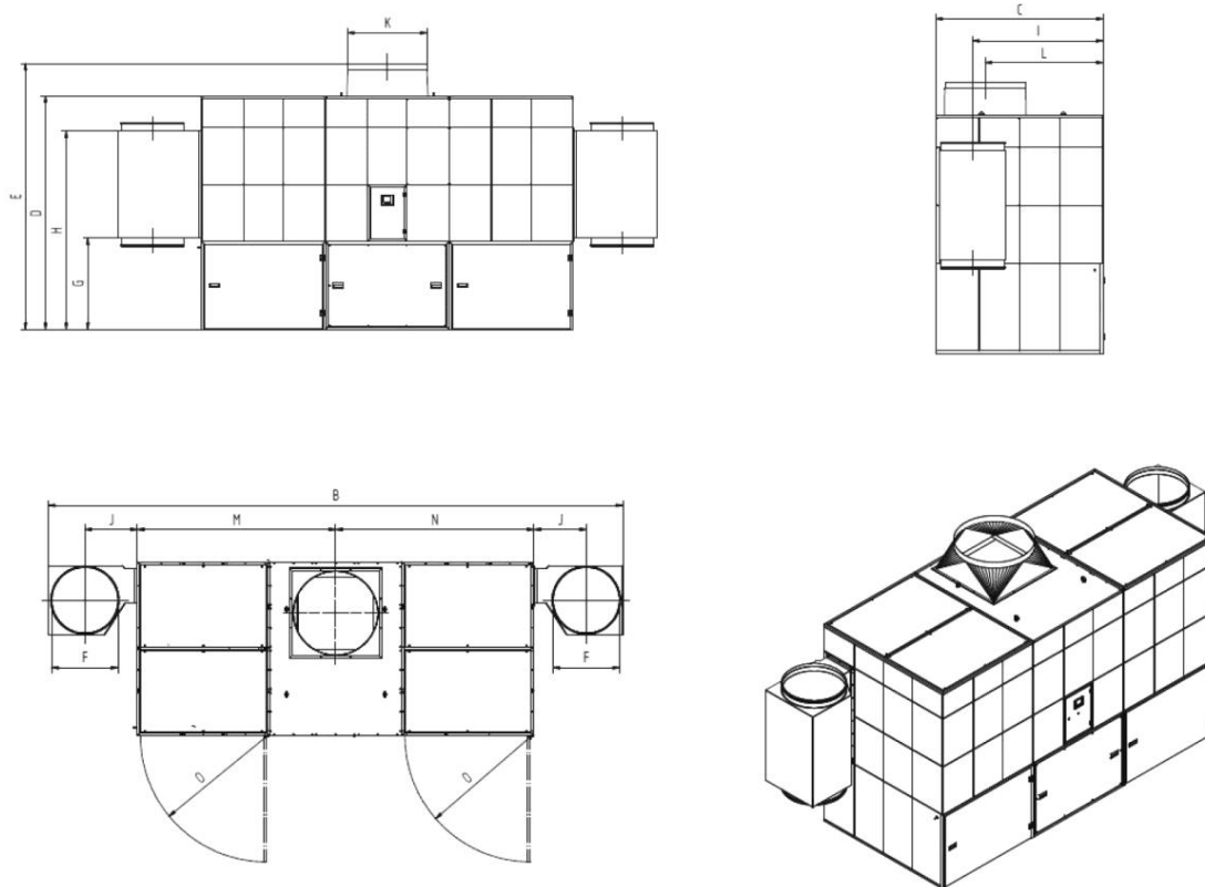
Fig. 294: Folha de dimensões 34180
