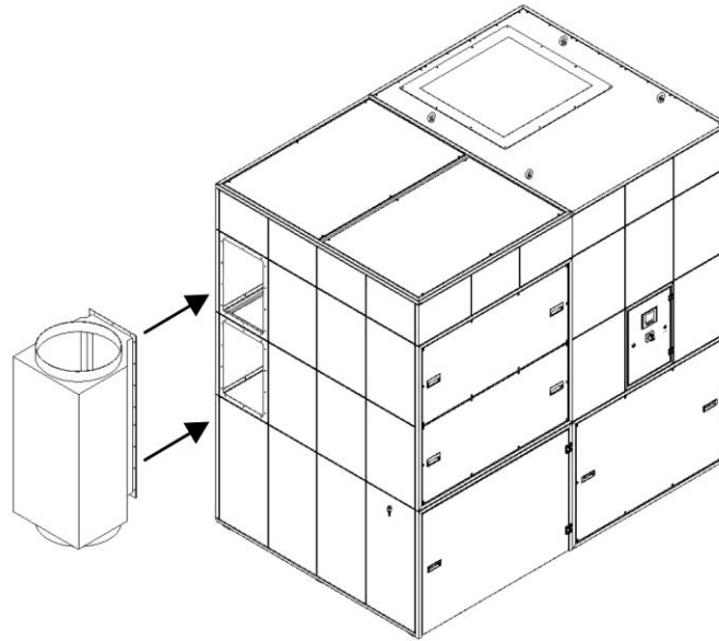
Fig. 322: Montaggio scatola di connessione lato aspirazione
