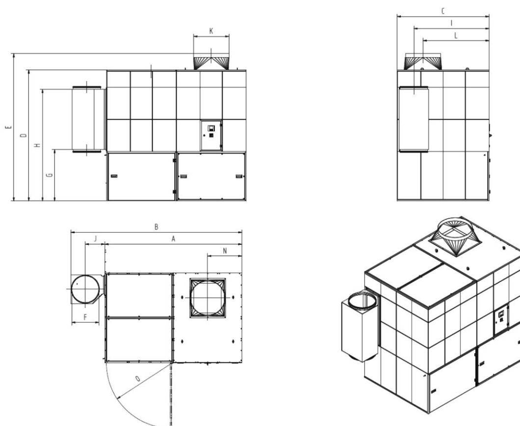
Fig. 292: Folha de dimensões 34130
