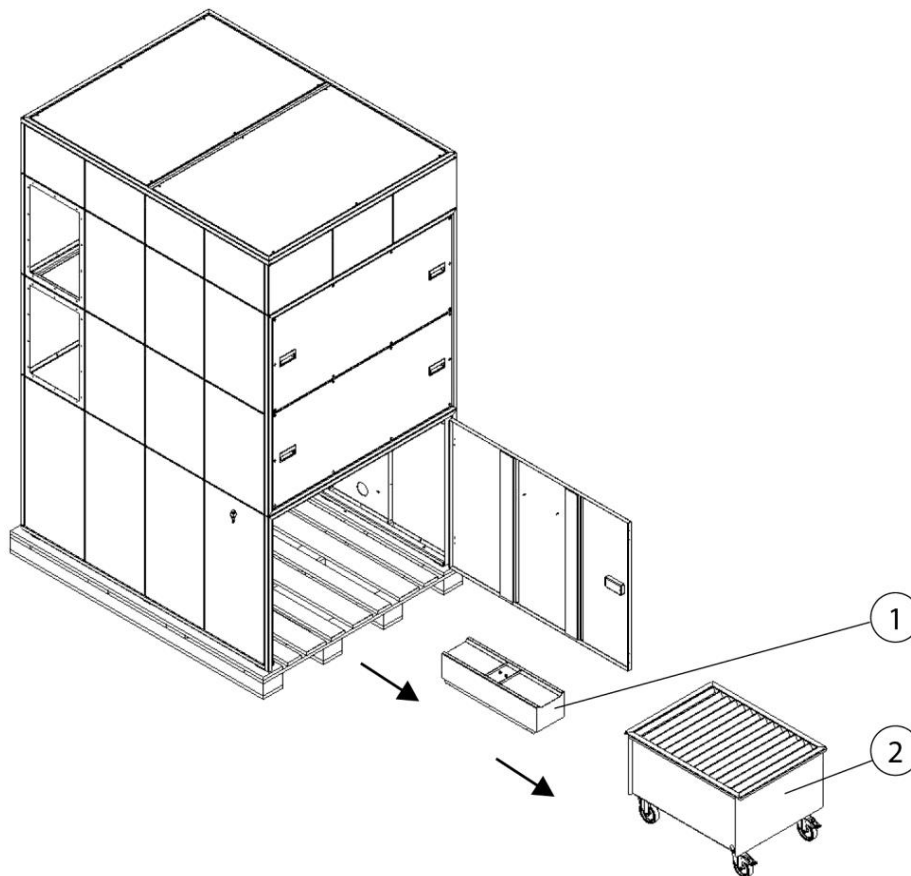
Fig. 164: Retirar el dispositivo colector de polvo y el dispositivo de elevación
