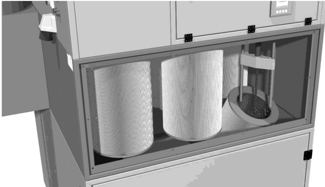
Afb. 136: Filtervervanging – filterpatronen verwijderen
