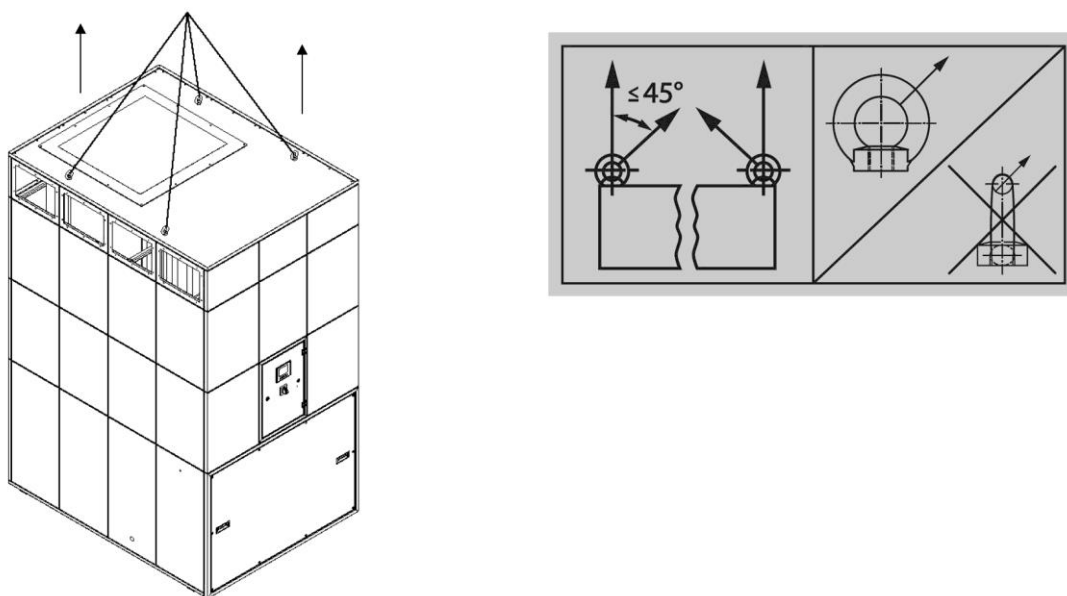
Fig. 166: Elevación del módulo del filtro con grúa
