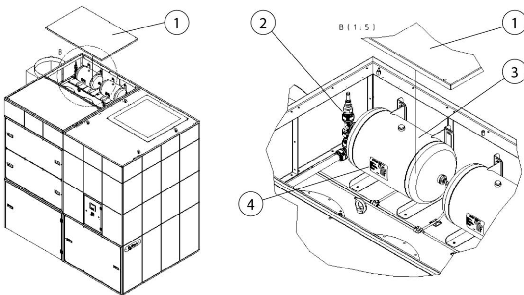
Fig. 289: Acesso ao reservatório de ar comprimido + válvula de segurança
