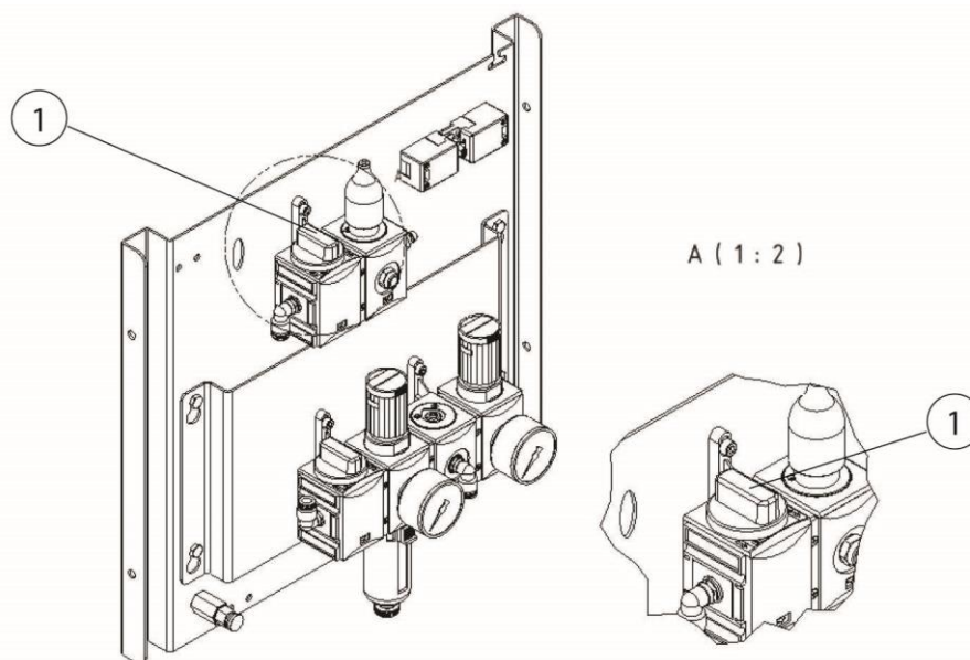
Fig. 55 : soupape pneumatique bac collecteur de poussières
