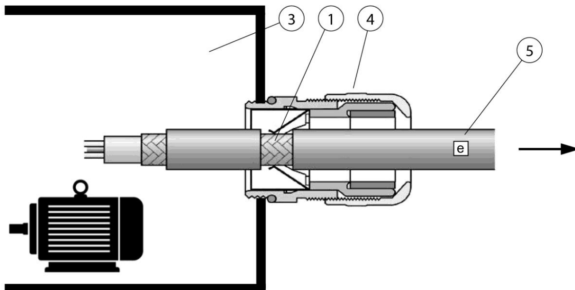
Fig. 185: Conectar pantalla del cable de motor
