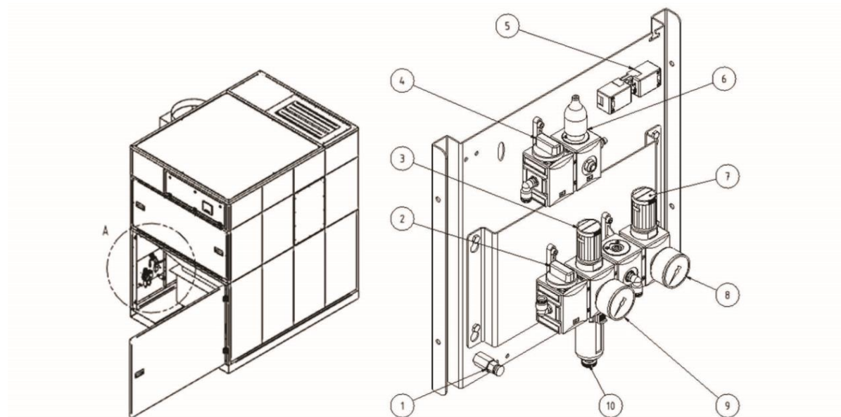
Fig. 27 : l'unité d'air comprimé
