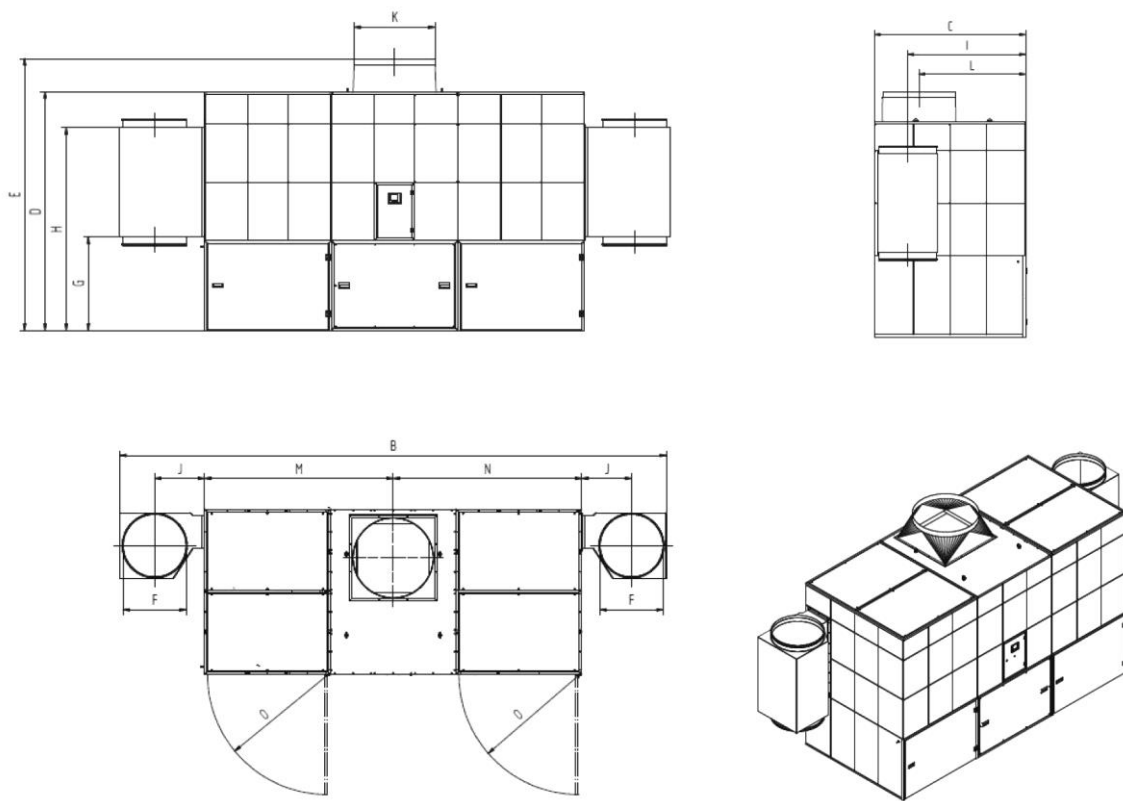
Fig. 73 : fiche dimensionnelle 34200 + 34220
