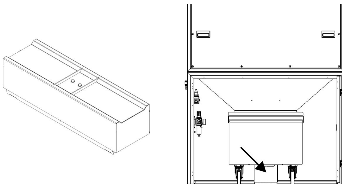
Fig. 320: Fissaggio del dispositivo di sollevamento sul pavimento
