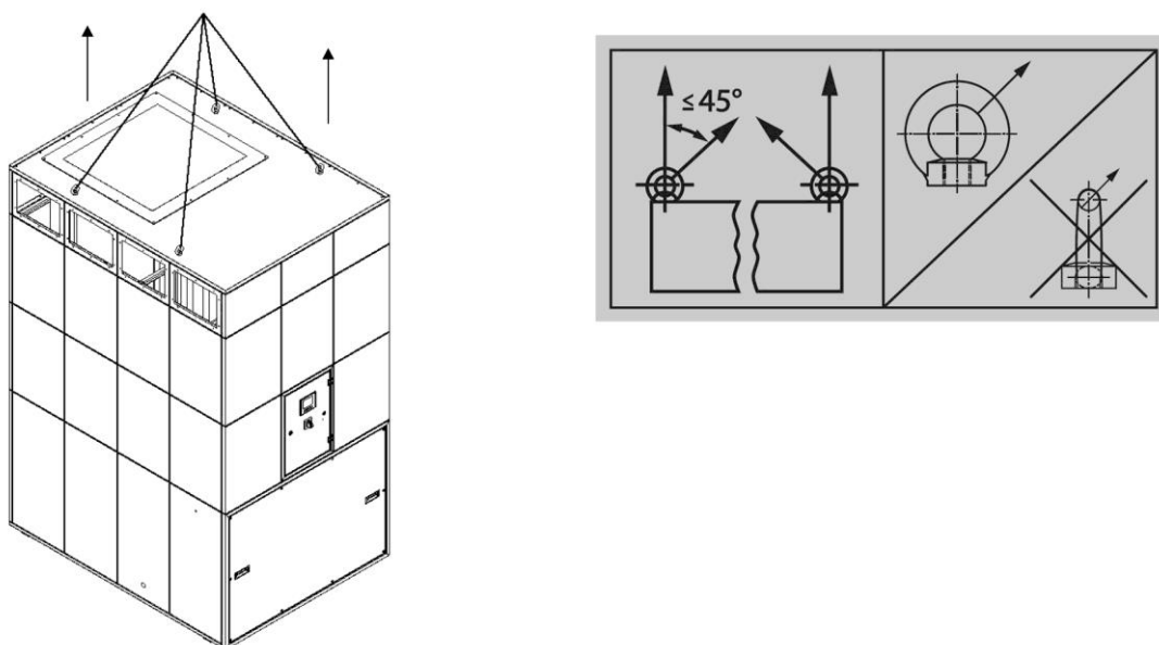
Fig. 240: Elevação do filtro com grua
