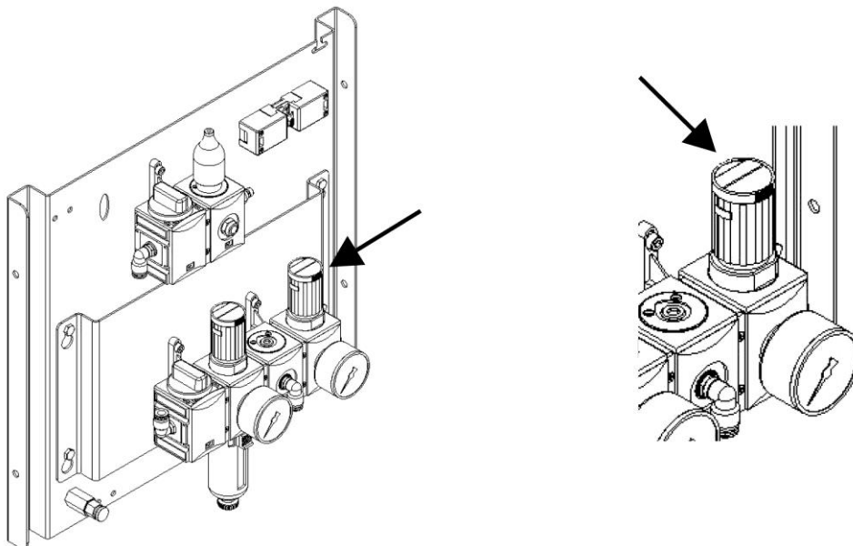
Afb. 104: Instellen van de druk voor hefinrichting/stofopvangreservoir
