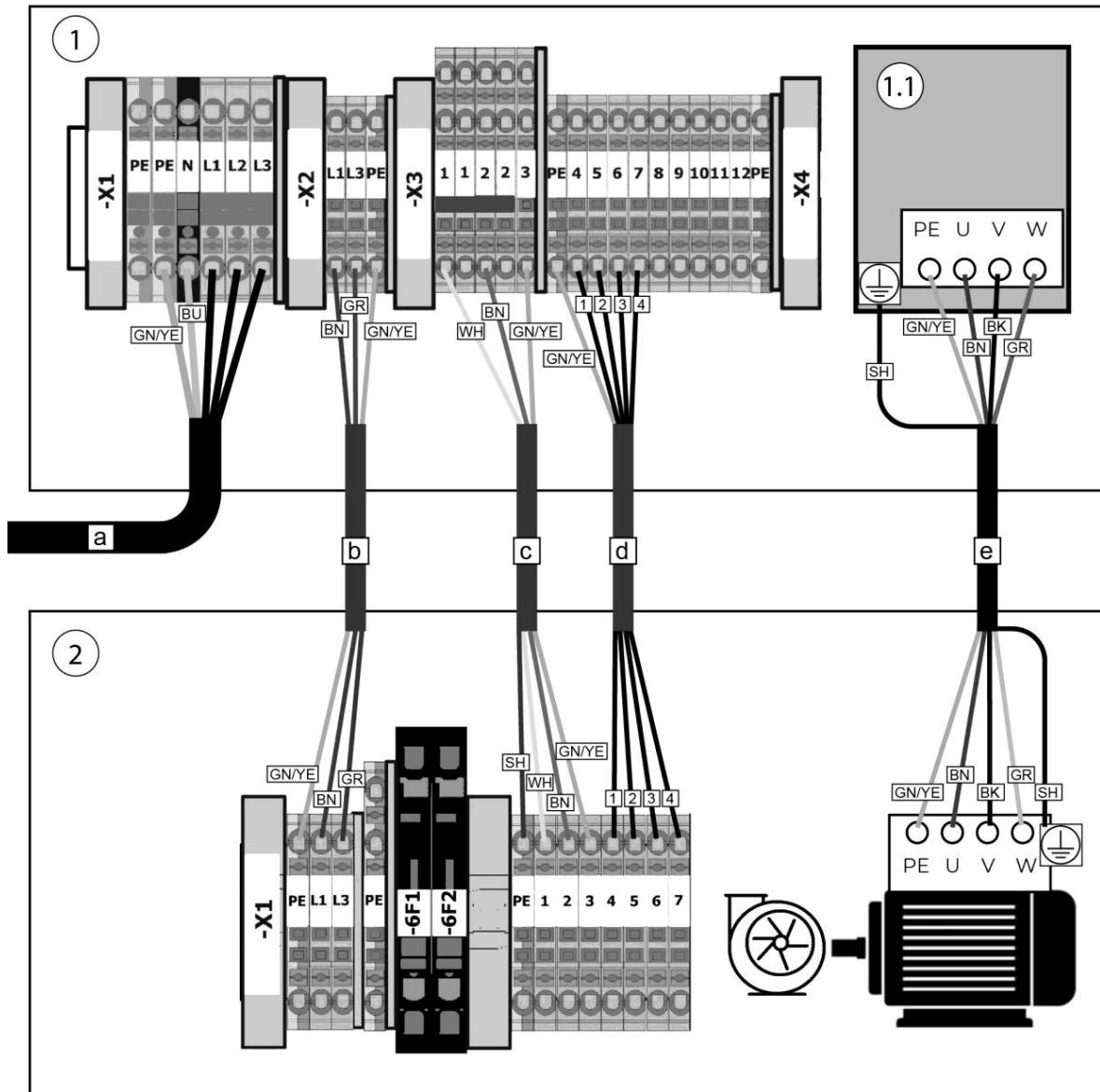
Fig. 331: Schema di cablaggio regolazione della potenza di aspirazione con prodotto
