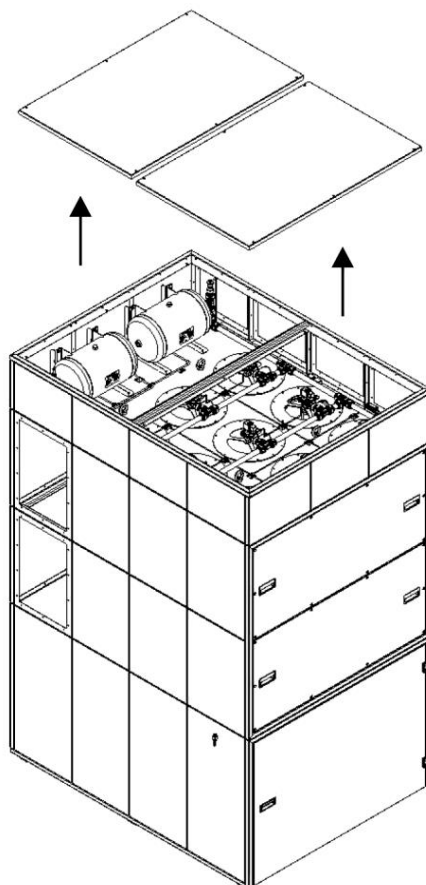
Fig. 313: Rimozione lamiera di copertura
