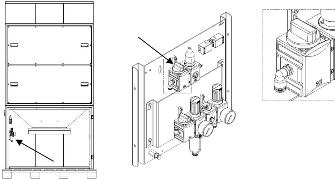
Fig. 14 : Soupape d'abaissement collecteur de poussières
