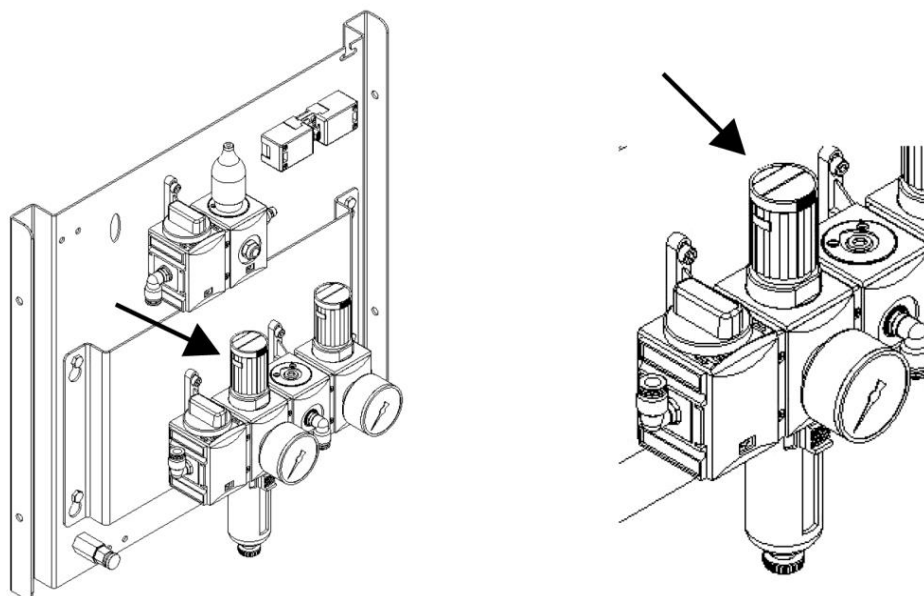
Fig. 325: Regolazione della pressione di esercizio
