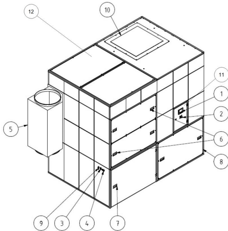
Fig. 149: 34110 - 34130
