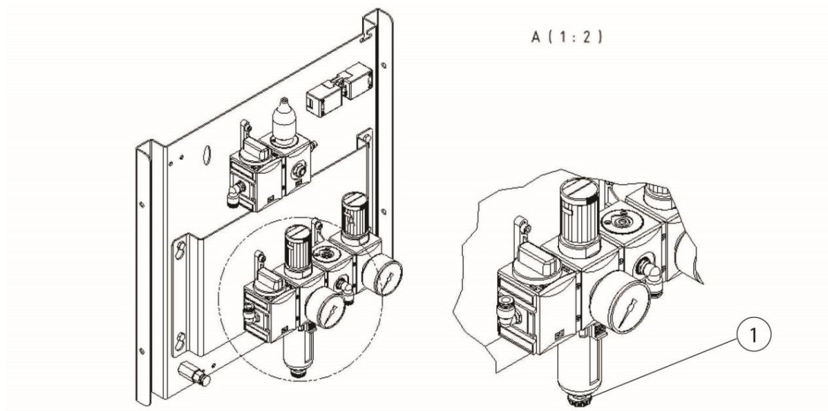
Fig. 212: Válvula de descarga de condensado unidad de mantenimiento de aire comprimido
