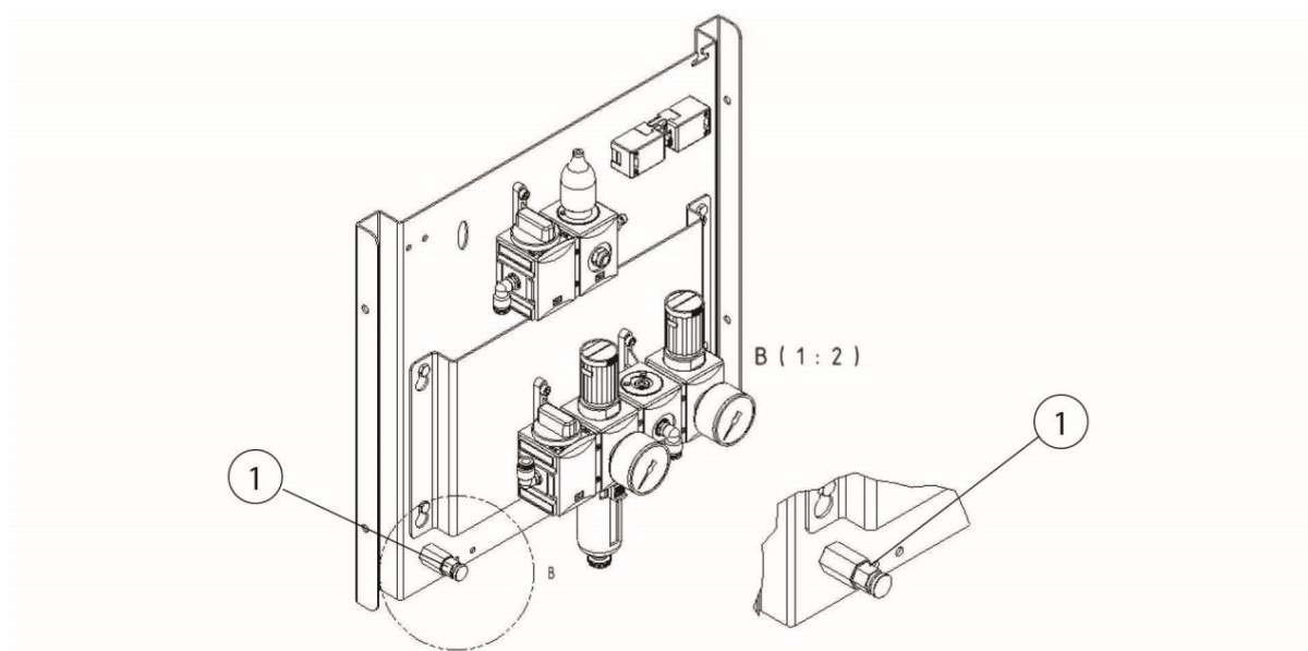
Fig. 211: Válvula de descarga de condensado depósito de aire comprimido
