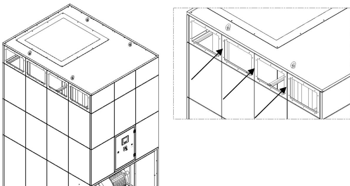
Fig. 12 : passage de l'air pur
