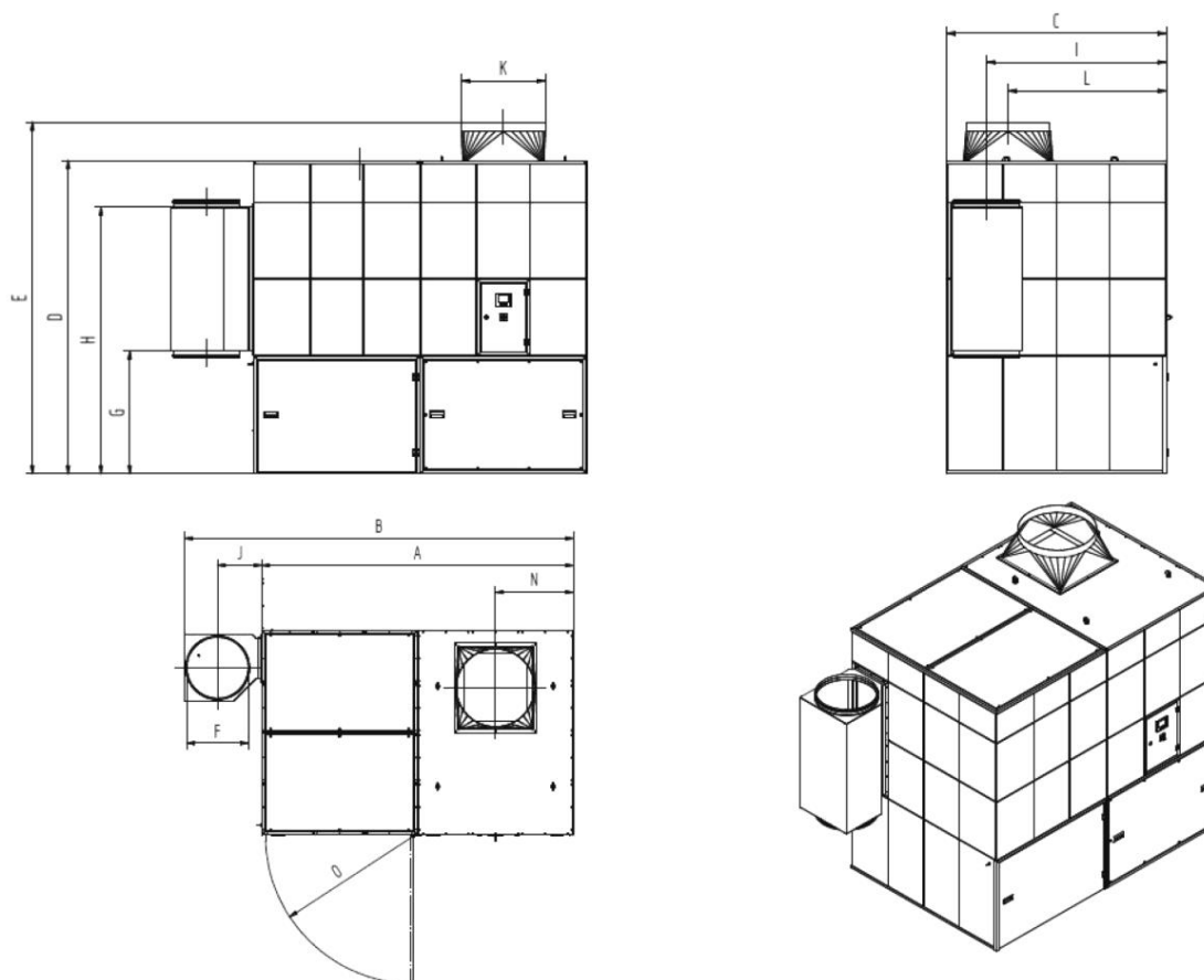
Fig. 217: Hoja de dimensiones 34110
