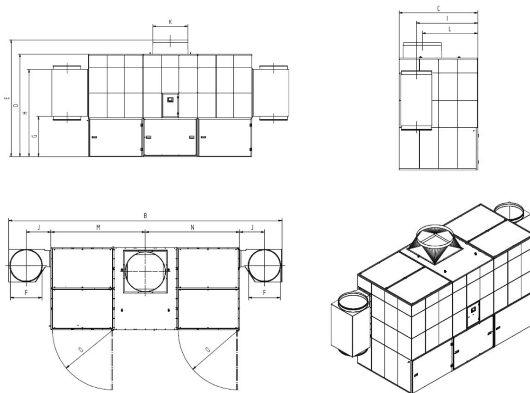
Fig. 219: Hoja de dimensiones 34160
