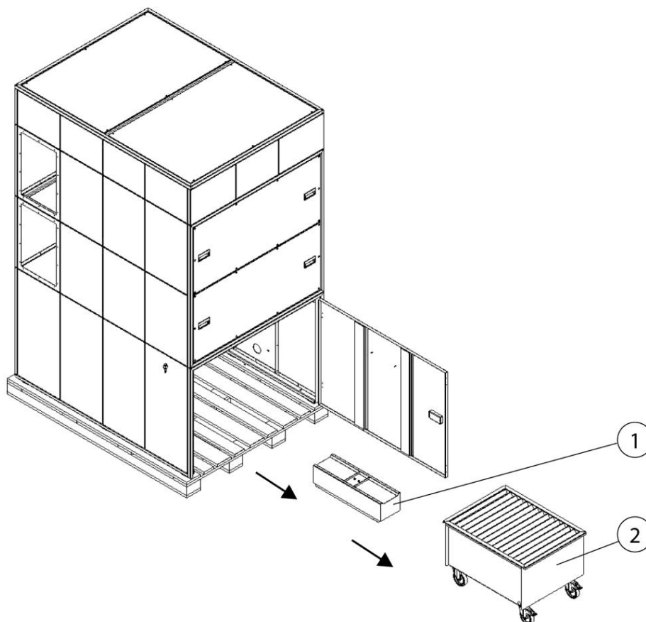
Fig. 238: Remover o recipiente coletor de pó e o dispositivo de elevação
