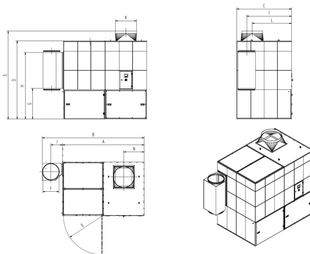
Fig. 218: Hoja de dimensiones 34130
