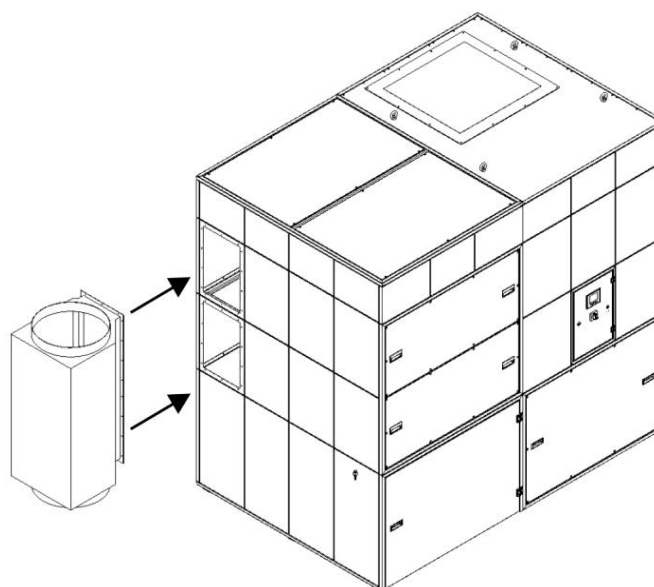
Fig. 248: Montagem da caixa de ligação do lado da aspiração
