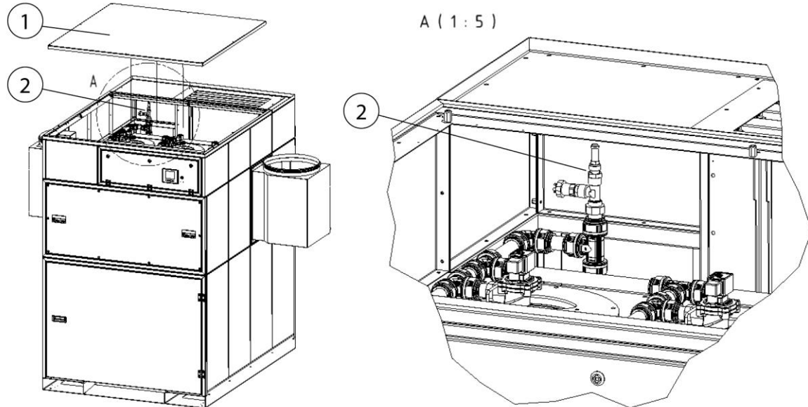
221. ábra: Hozzáférés a sűrített levegő biztonsági szelephez
