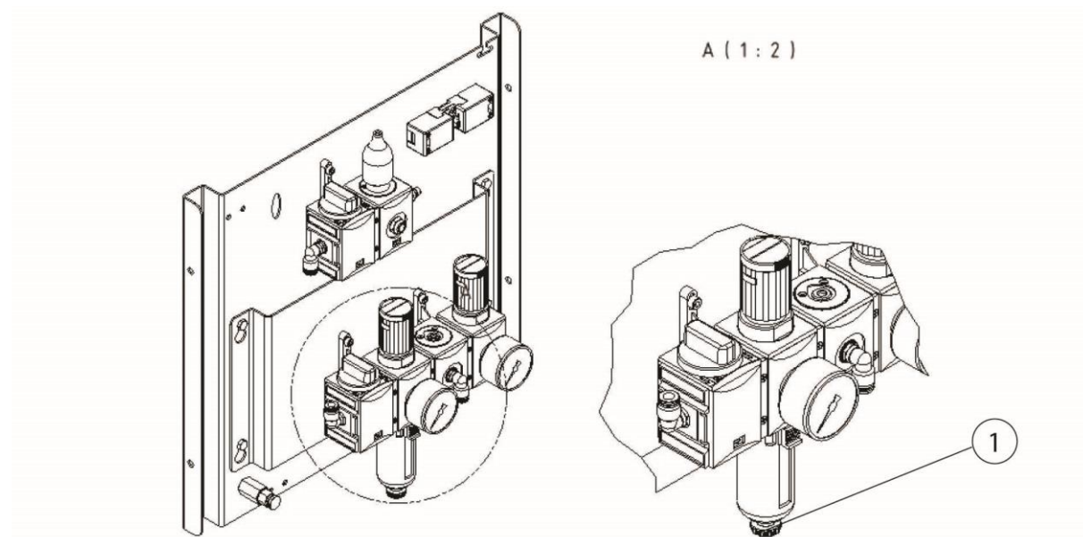
Rys. 103: Zawór spustowy skroplin jednostki uzdatniania sprężonego powietrza
