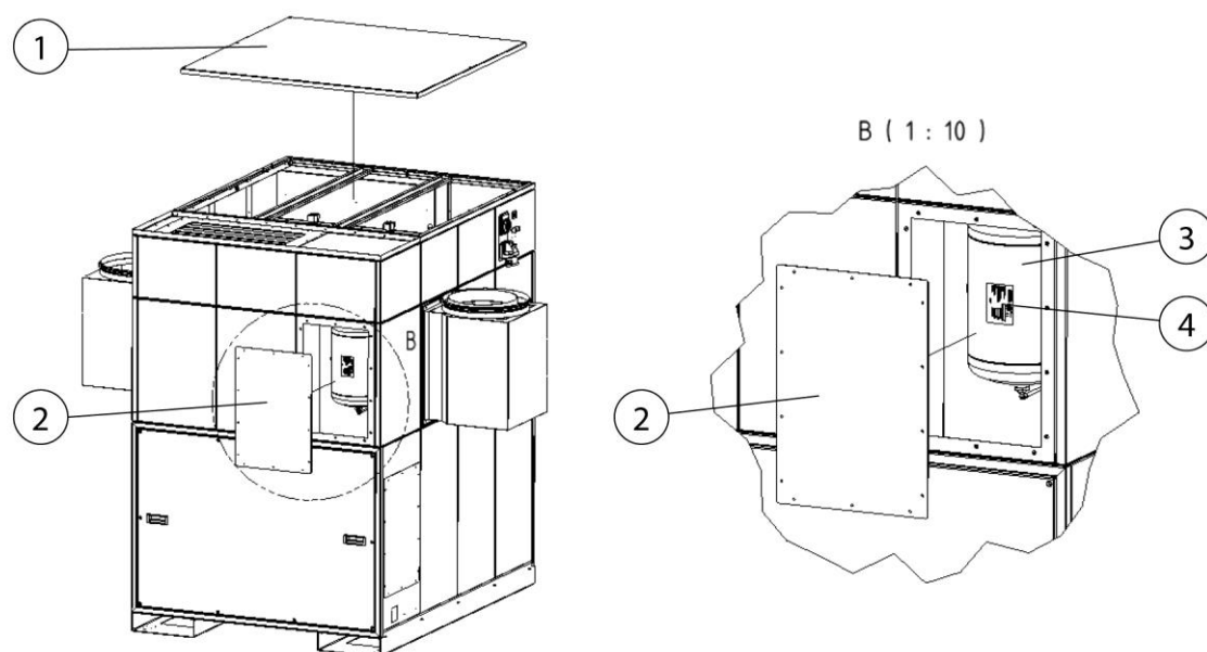
Rys. 106: Dostęp do zbiornika sprężonego powietrza
