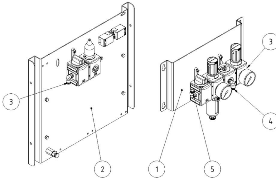
Sl. 241: Enota s stisnjnim zrakom (zunanja različica)
