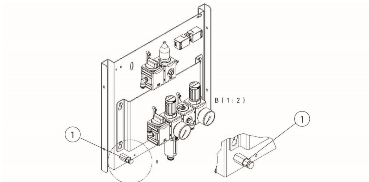
Sl. 273: Ventil izpusta kondenzata iz posode stisnjenega zraka
