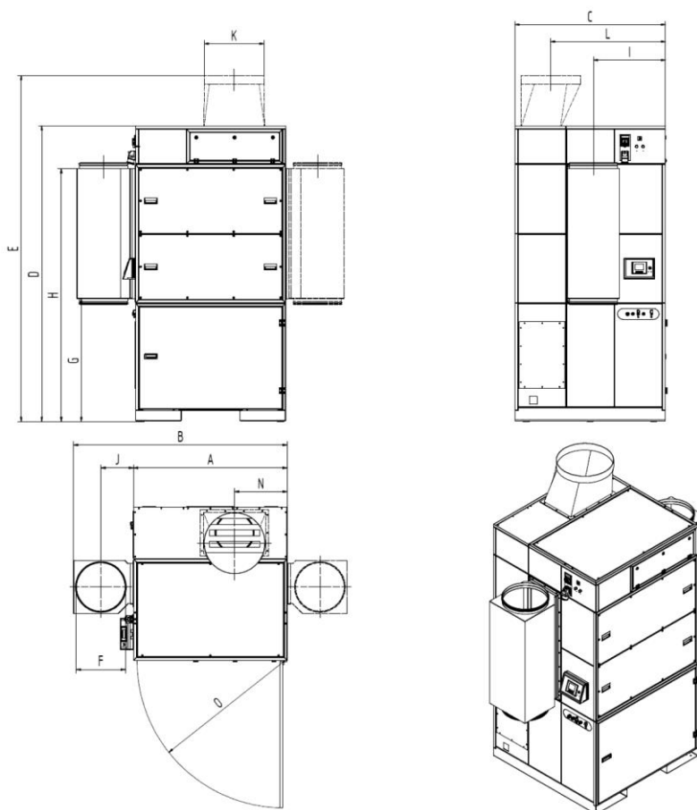
Rys. 113: Karta wymiarowa 3475
