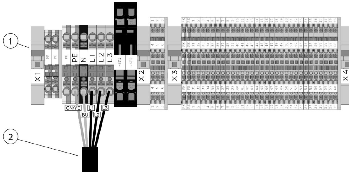
Рис. 128: Рейка с присоединительными зажимами в распределительном шкафу изделия
