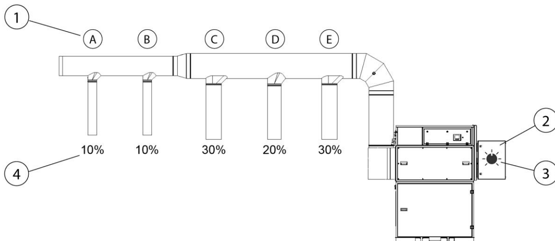
Sl. 264: Nastavitev upravljanja zmogljivosti odsesavanja
