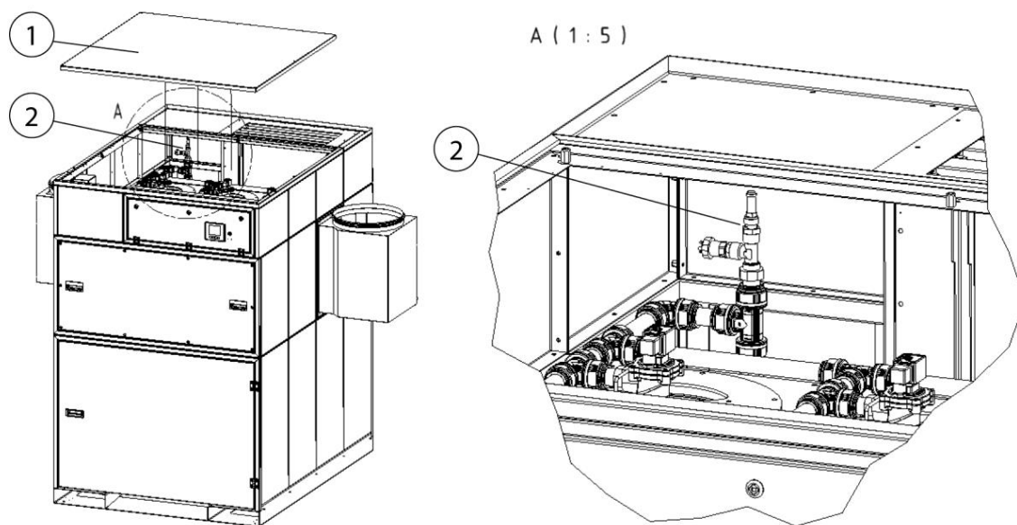
Рис. 164: Доступ к предохранительному клапану сжатого воздуха
