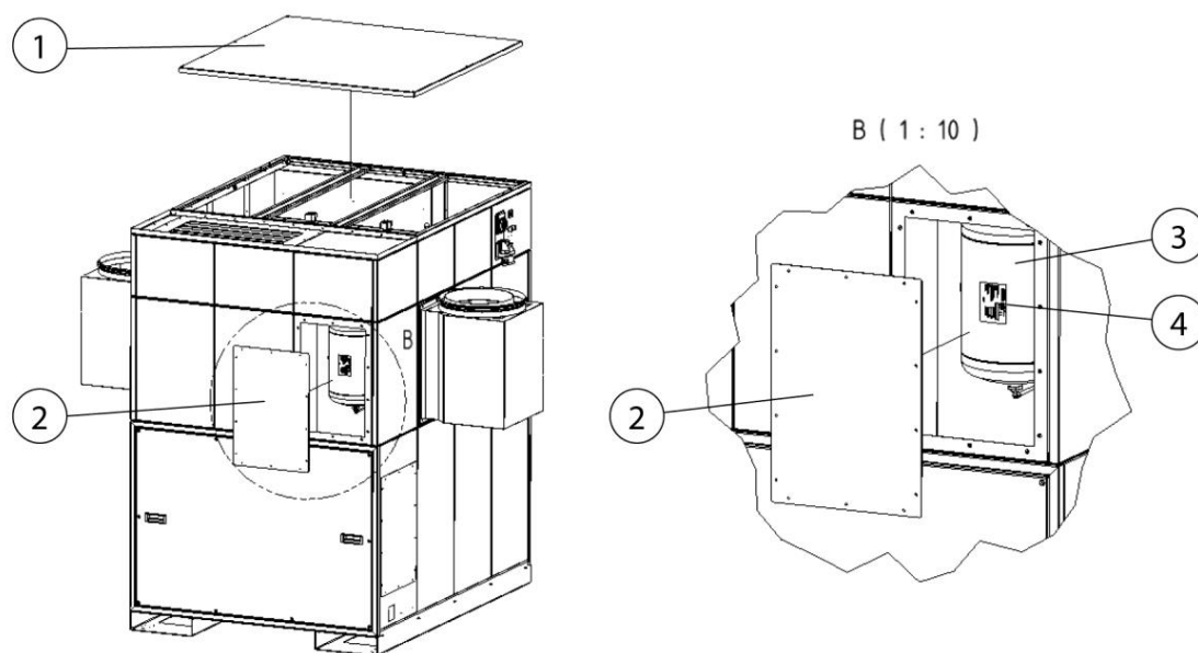
Sl. 277: Dostop do posode s stisnjenim zrakom
