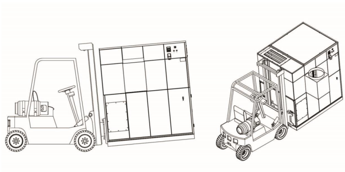
Рис. 124: Транспортировка изделия
