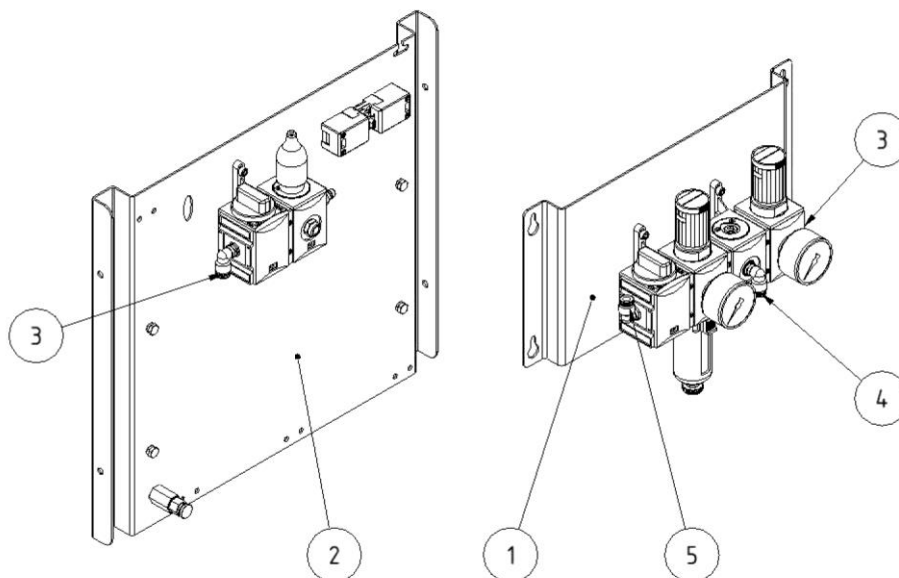
184. ábra: Sűrített levegős egység (kültéri változat)
