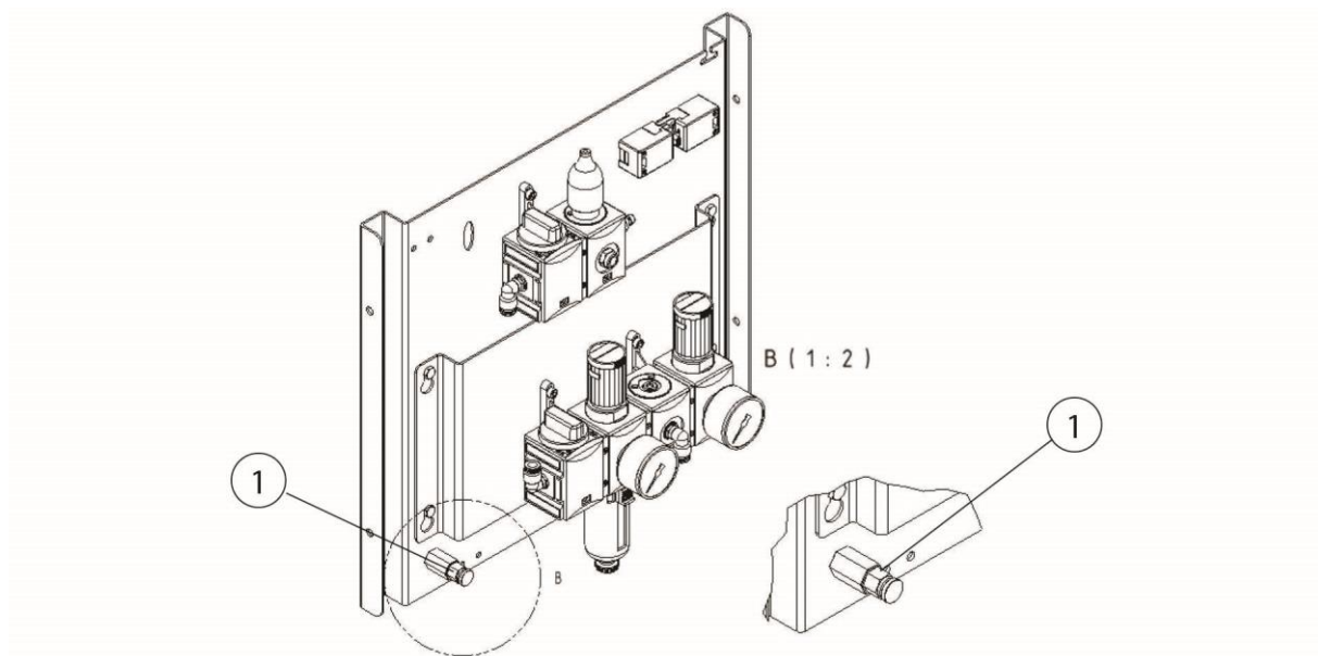
216. ábra: Sűrítettlevegő-tartály kondenzvíz leeresztőszelepe
