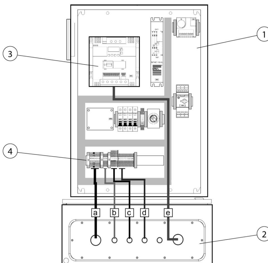
Sl. 244: Nadzorna omarica upravljanja zmogljivosti odsesavanja
