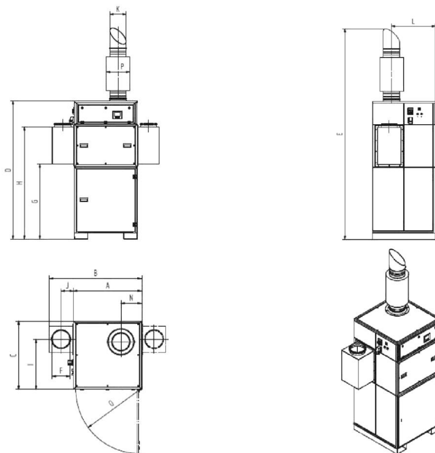
Рис. 166: Габаритный чертеж 3420
