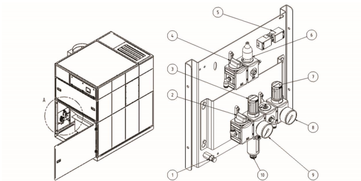
Rys. 69: Jednostka sprężonego powietrza
