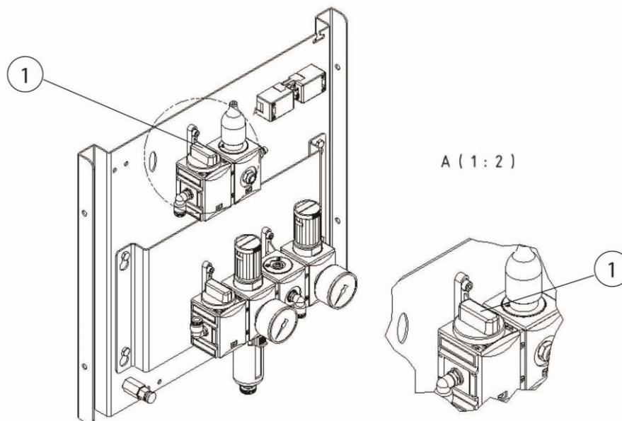
208. ábra: Porgyűjtő tartály pneumatikus szelepe
