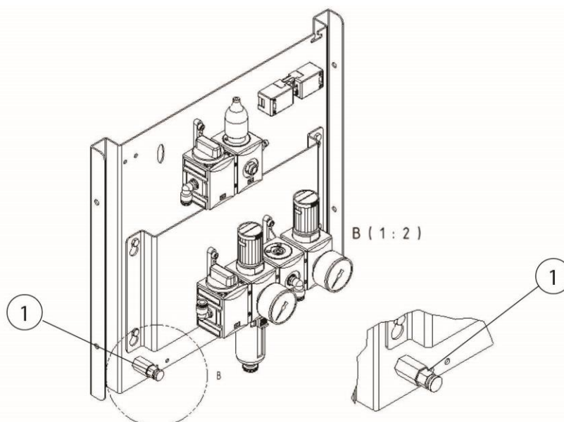
Rys. 102: Zawór spustowy skroplin zbiornika sprężonego powietrza
