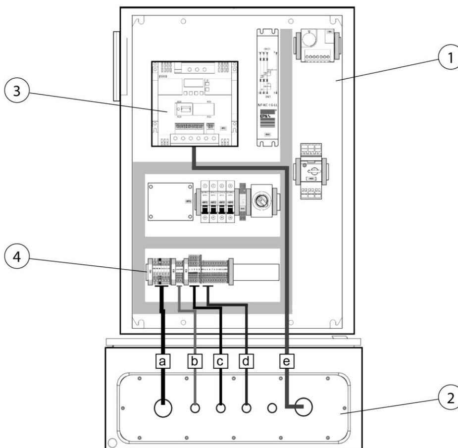
Rys. 73: Szafa rozdzielcza, układ regulacji mocy ssącej
