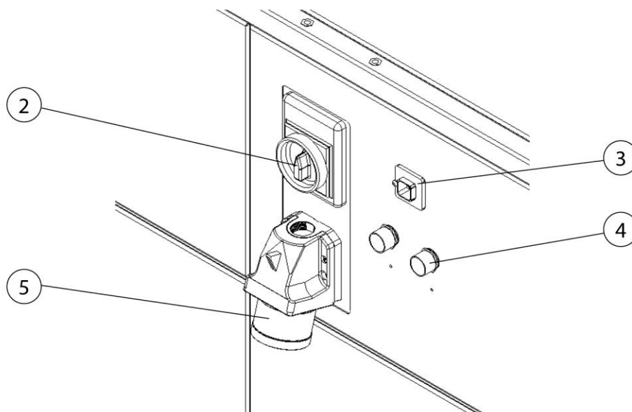
178. ábra: Csatlakozópanelek
