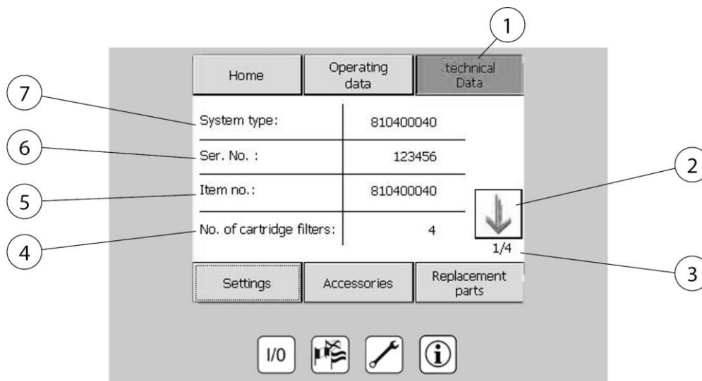
Rys. 79: Dane techniczne
