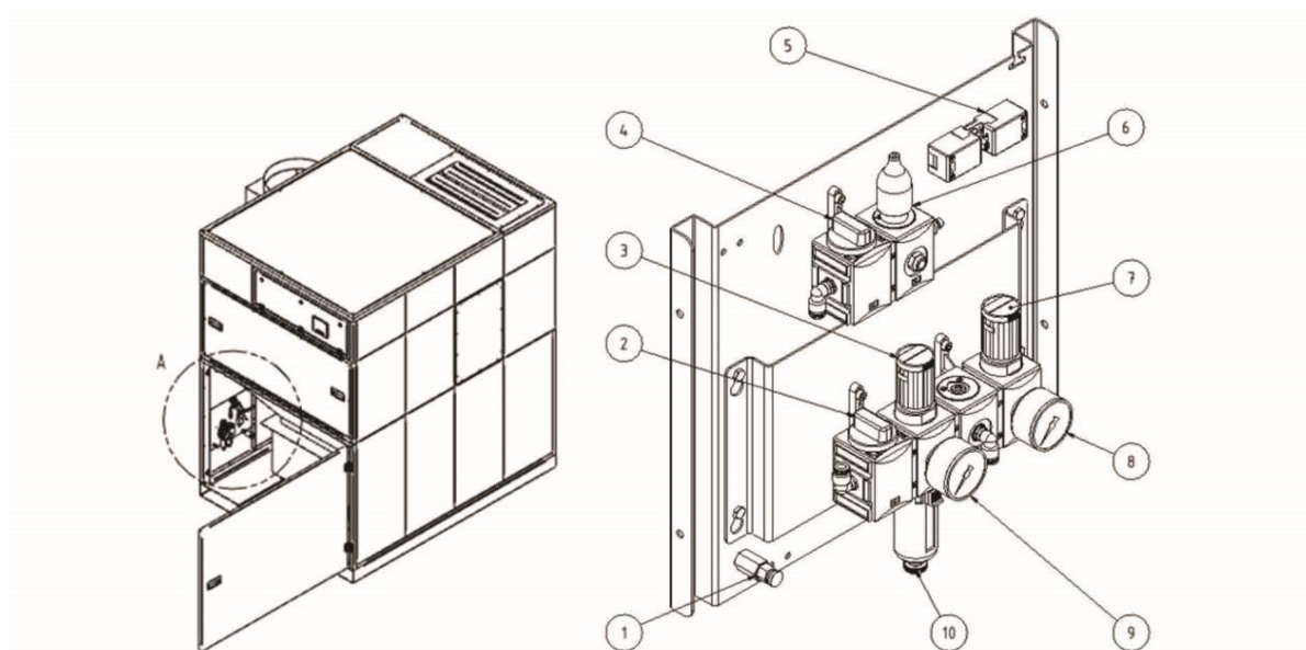
Рис. 126: Узел пневмосистемы
