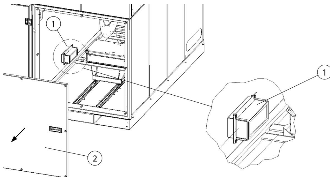
211. ábra: Hozzáférés a biztonsági szűrőhöz
