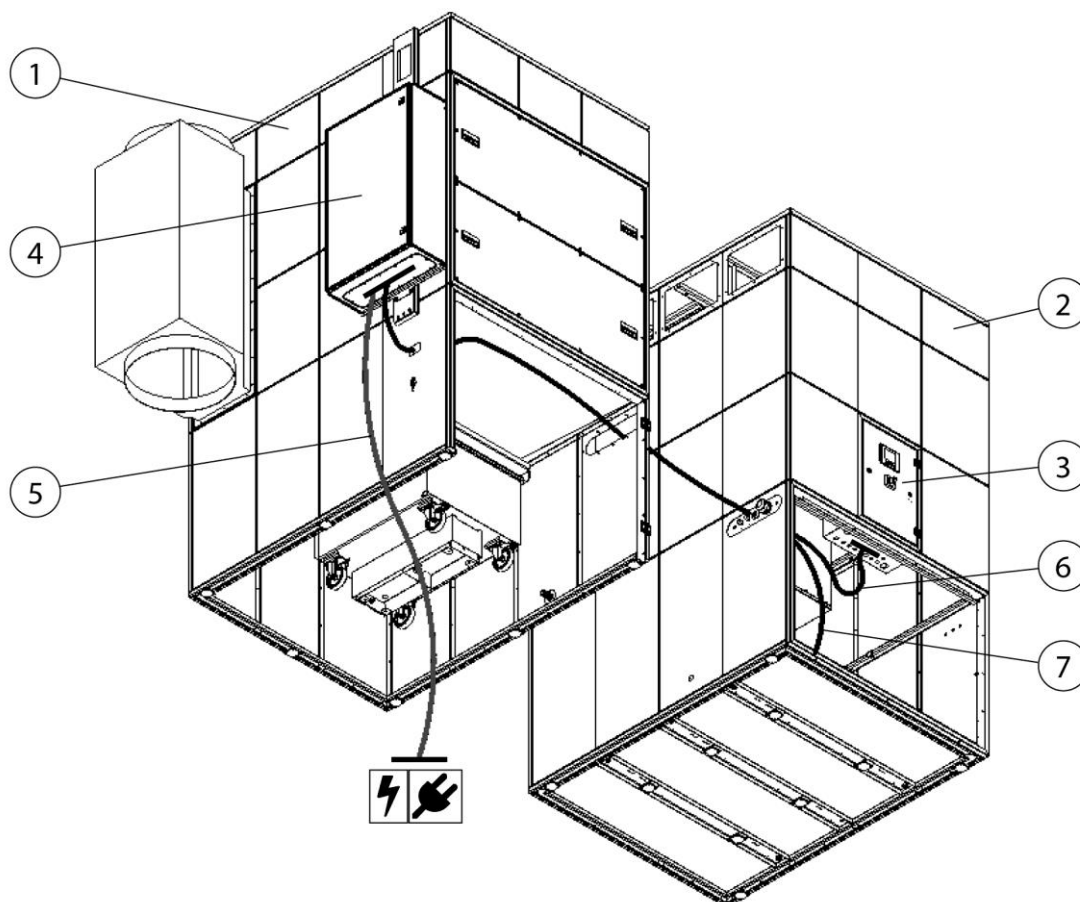
Obr. 15: Příklad: Pokládání kabelů regulace odsávacího výkonu
