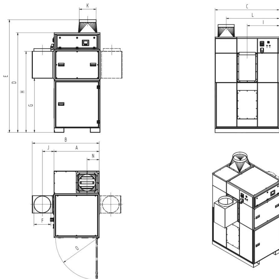
Рис. 167: Габаритный чертеж 3430
