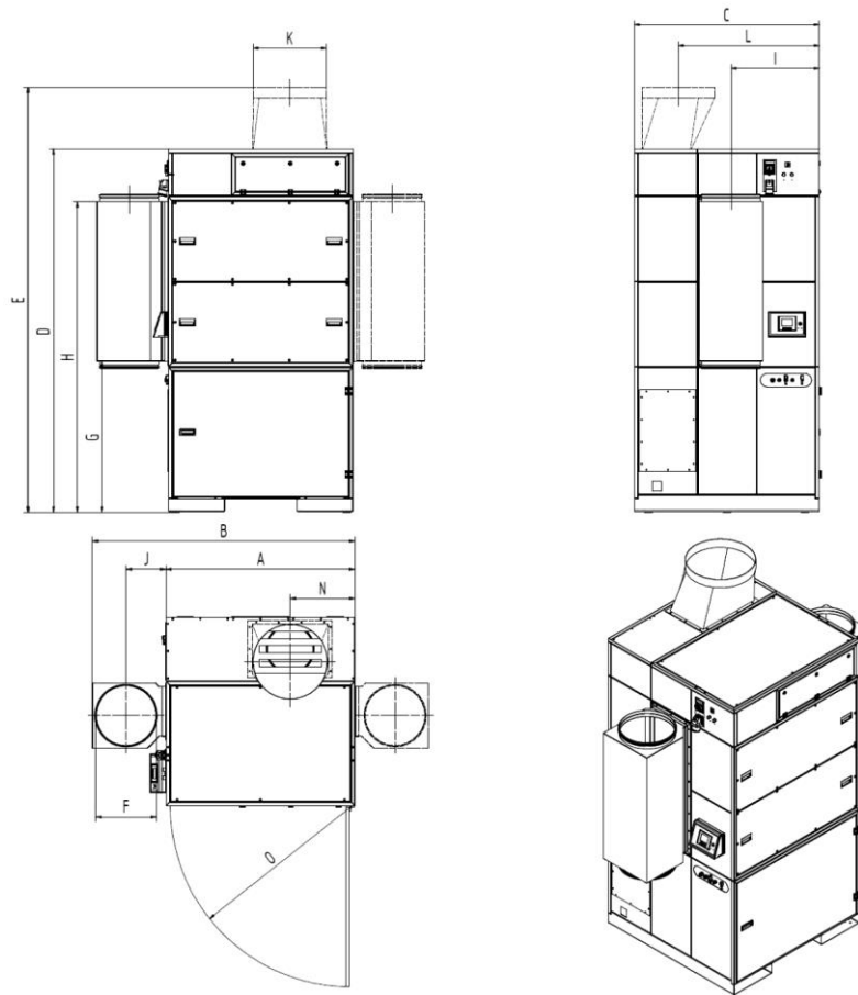
Obr. 56: Rozměrový výkres 3475
