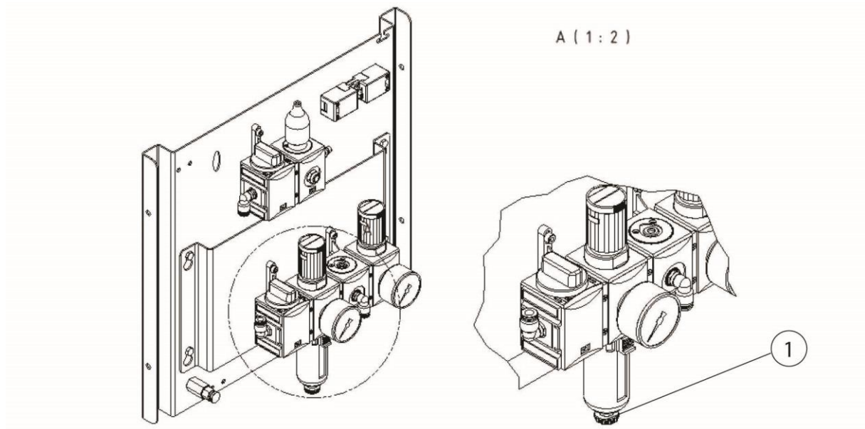
217. ábra: A sűrített levegős karbantartó egység kondenzvíz leeresztőszelepe
