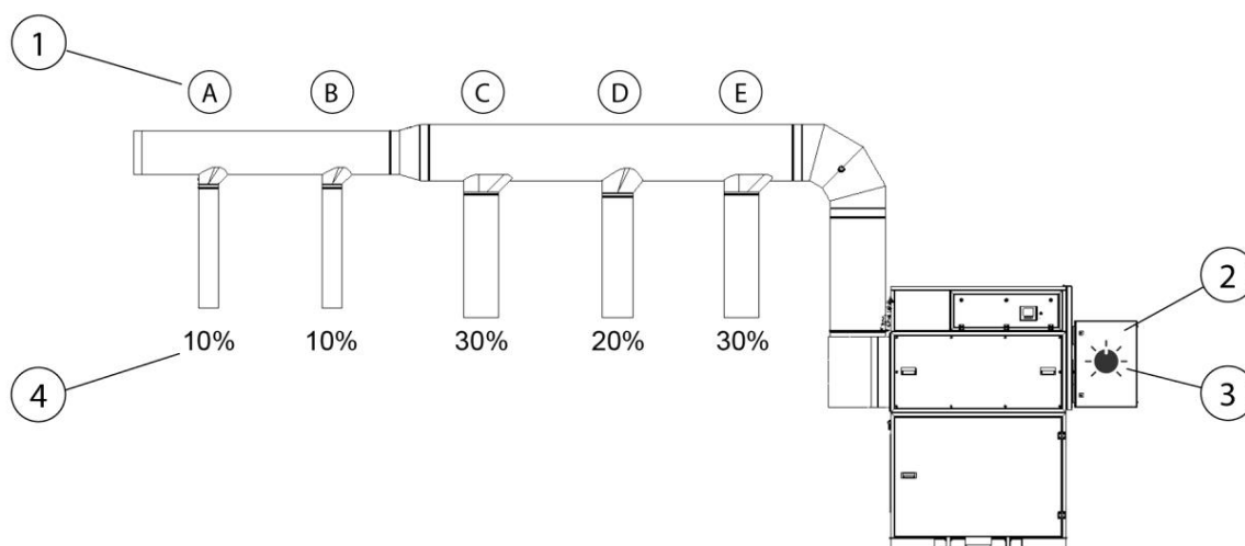
Рис. 150: Регулировка производительности вытяжки
