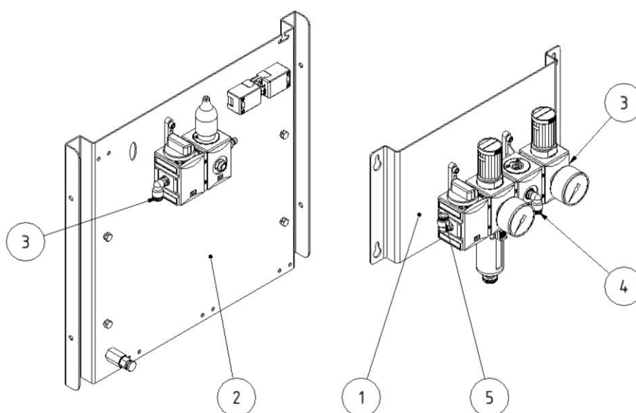
Rys. 70: Jednostka sprężonego powietrza ( Wersja Zewnętrzna)
