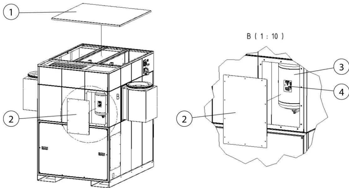
220. ábra: Hozzáférés a sűrítettlevegő-tartályhoz
