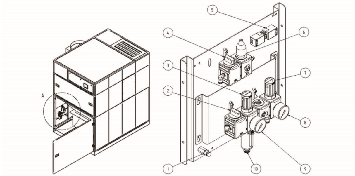
183. ábra: Sűrített levegős egység
