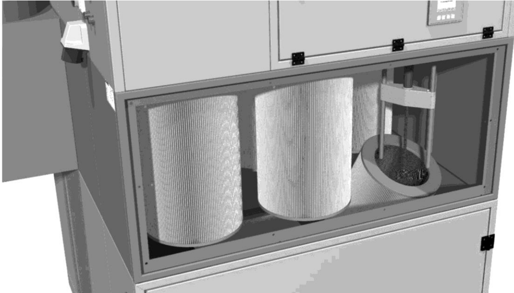
Rys. 101: Wymiana filtra- wymiana wkładu filtra
