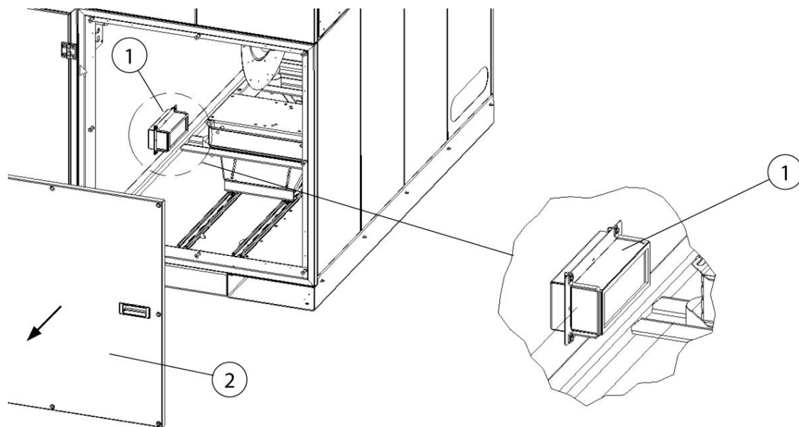
Рис. 154: Доступ к защитному фильтру
