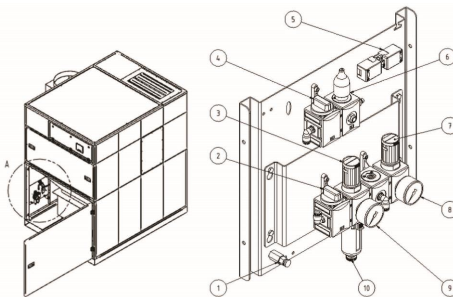
Sl. 240: Enota s stisnjnim zrakom
