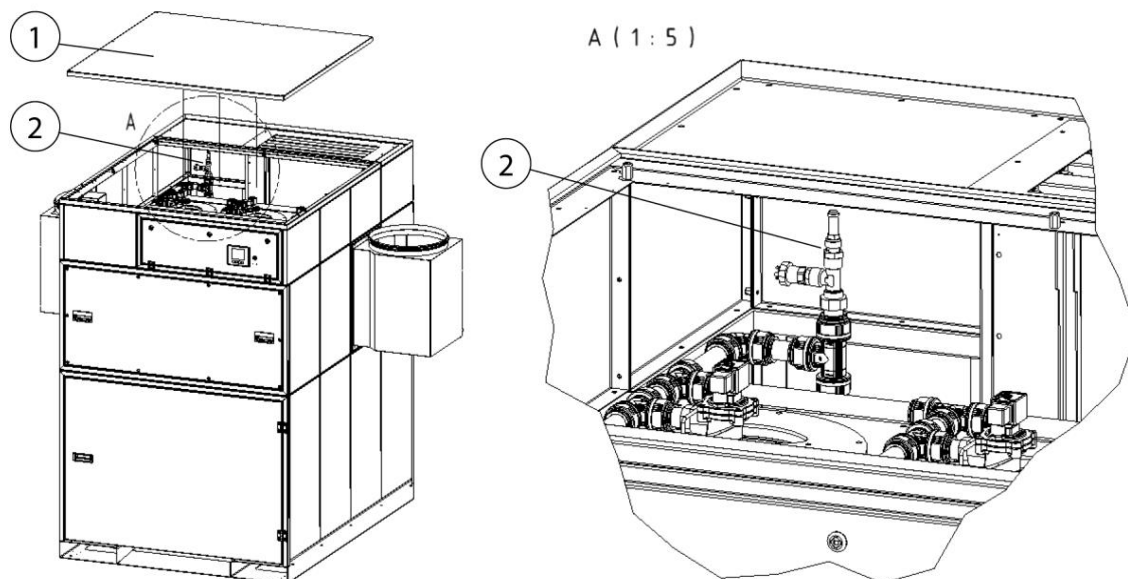
Sl. 278: Dostop do varnostnega ventila stisnjenega zraka
