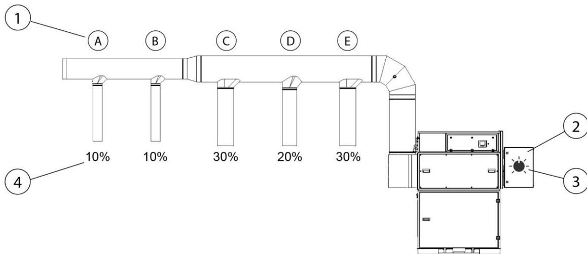
207. ábra: Az elszívási teljesítmény-szabályozó beállítása
