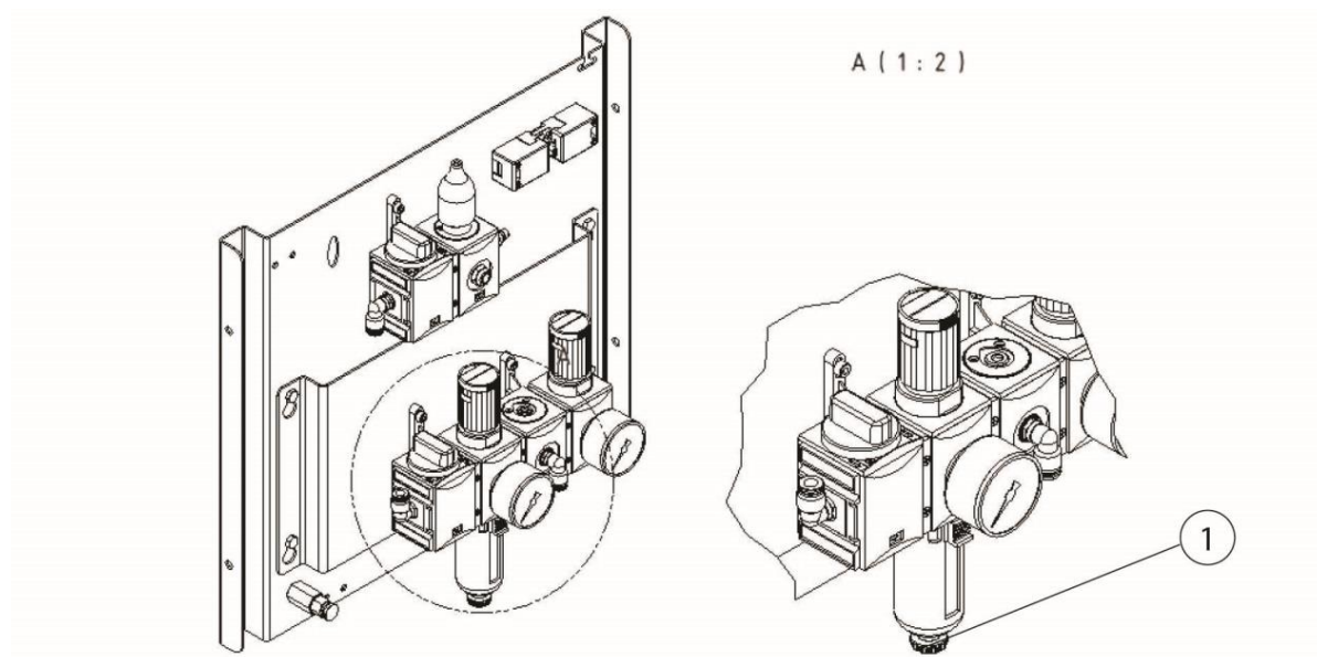
Sl. 274: Ventil odtoka kondenzata vzdrževalne enote s stisnjenim zrakom
