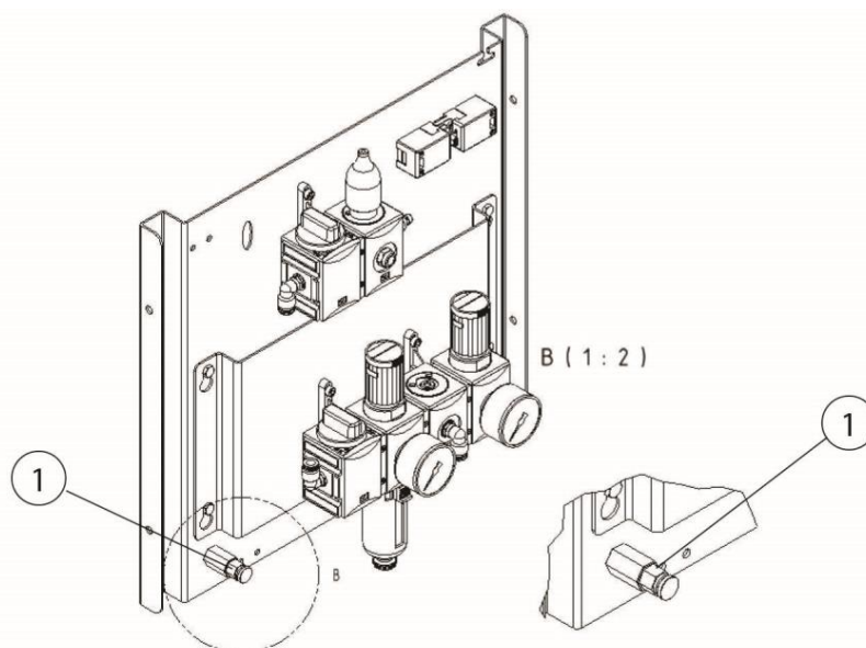
Рис. 159: Вентиль слива конденсата из ресивера
