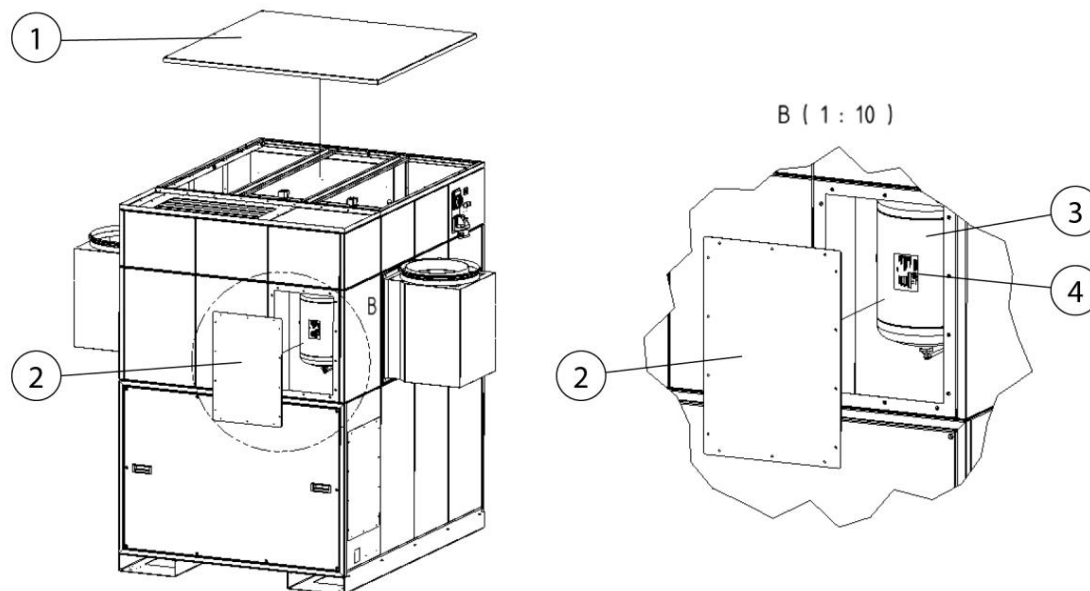
Рис. 163: Доступ к резервуару для сжатого воздуха
