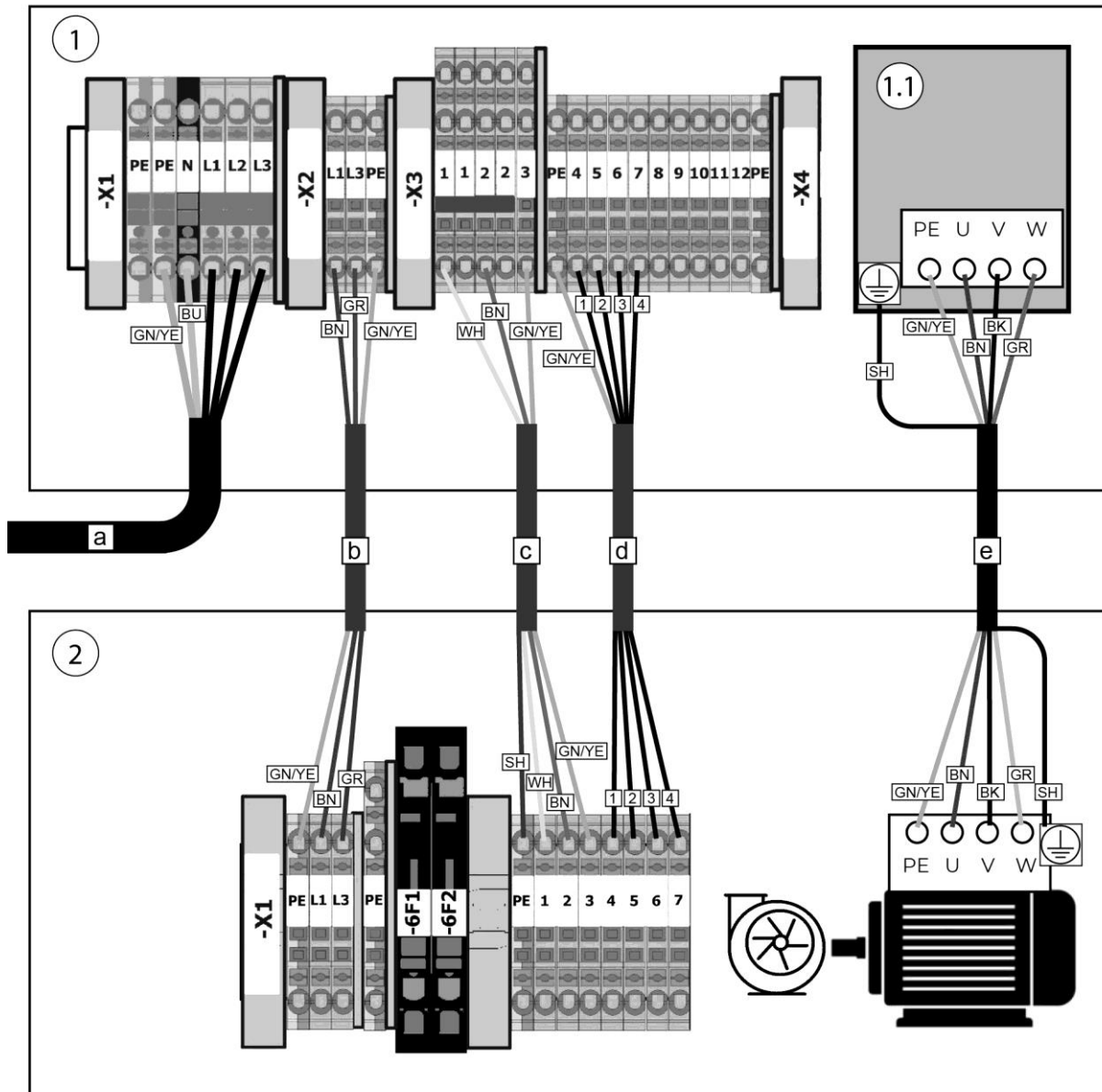
188. ábra: Huzalozási terv - elszívási teljesítmény-szabályozó és termék
