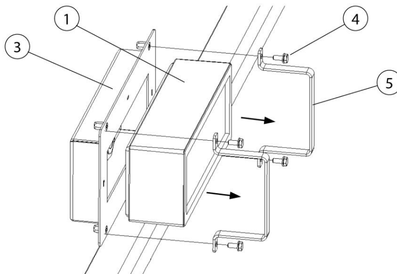
Рис. 155: Замена защитного фильтра
