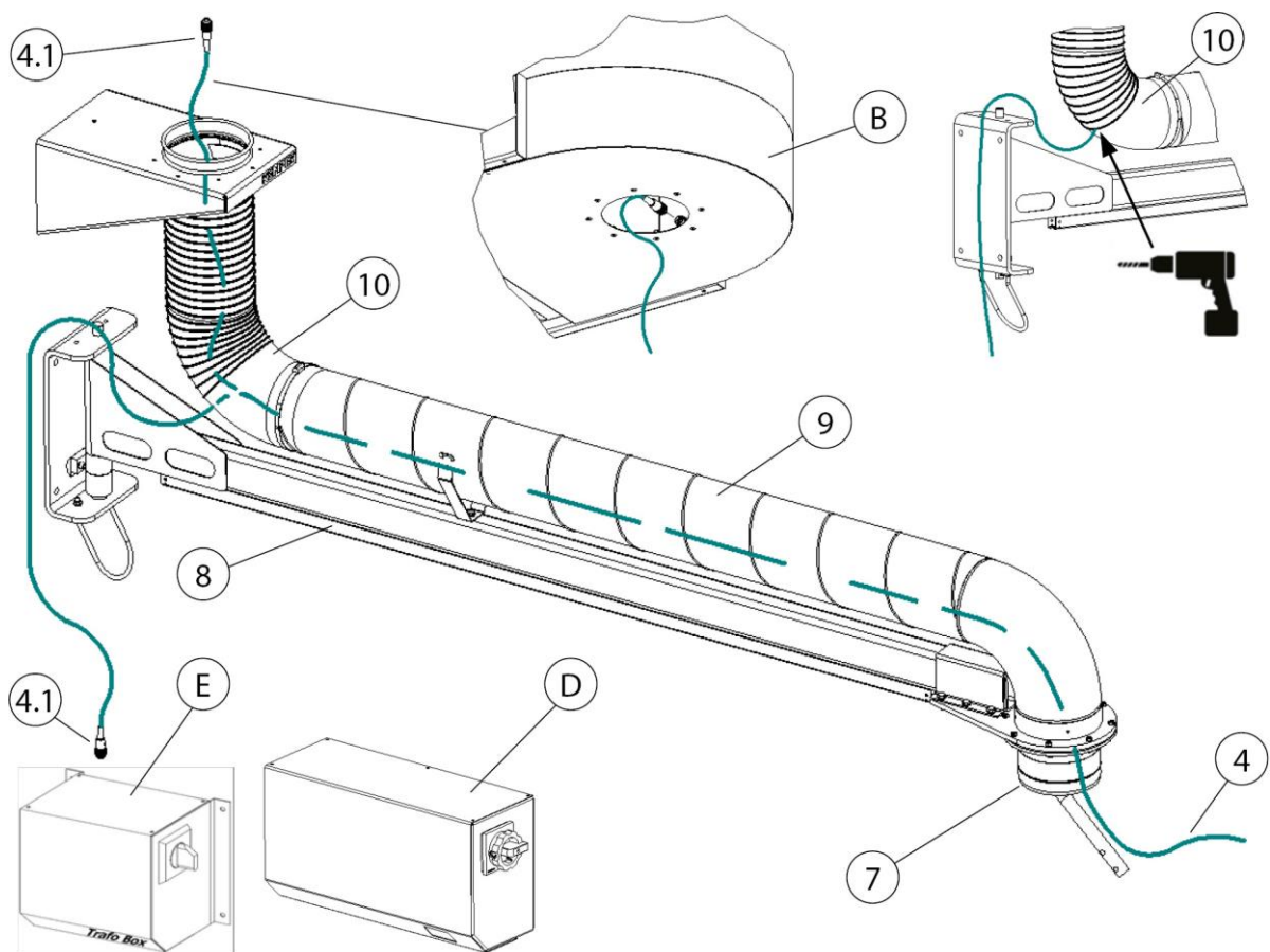
Afb. 83: Kabel leggen – afzuigarmen met kraangiek
