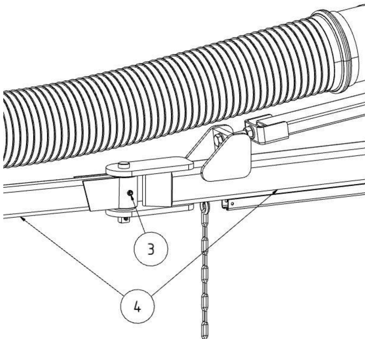
Rys. 192: Hamulec
