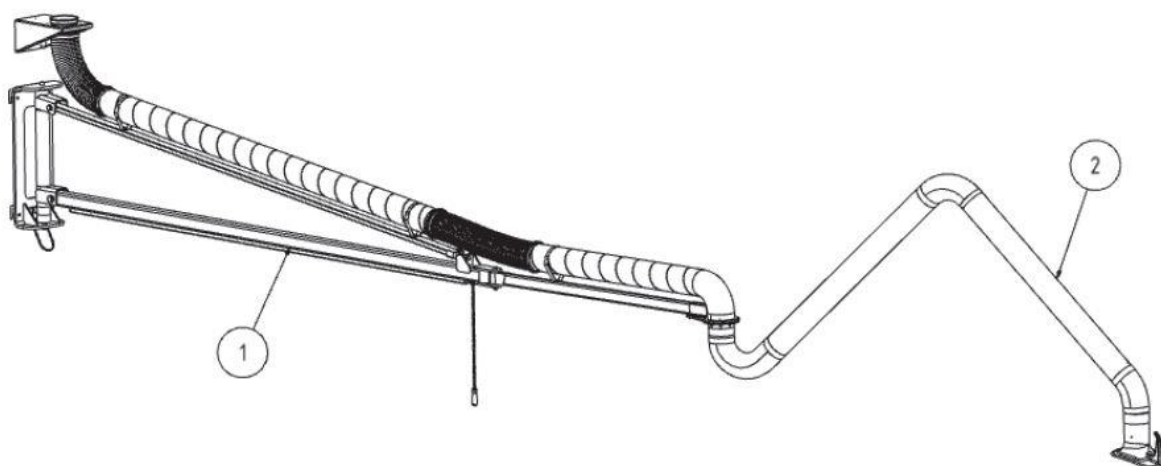
Rys. 177: Ramię odciągowe z ramieniem wysięgnika wychylnego
