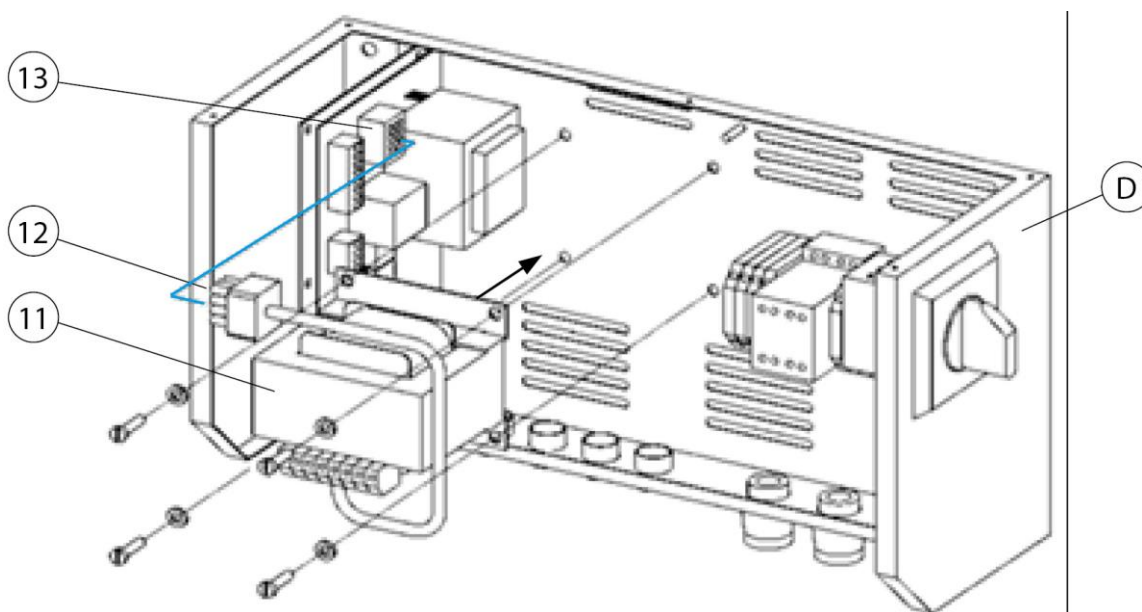
Рис. 216: Блок управления – дооснащение трансформатором
