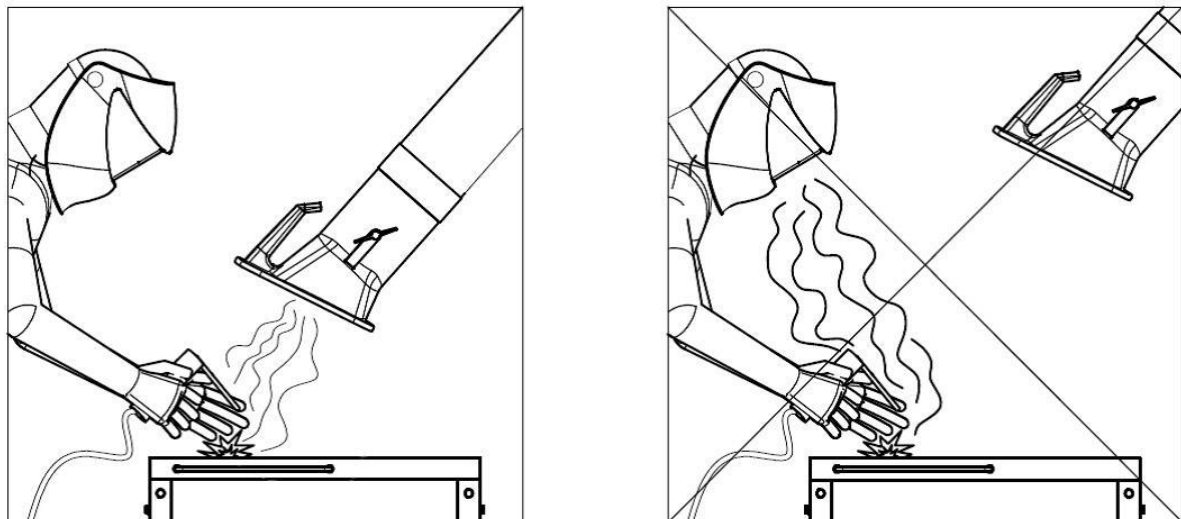
Afb. 87: Positionering van de afzuigkap
