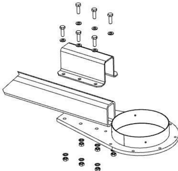
230. ábra: Az elszívókartartó felszerelése
