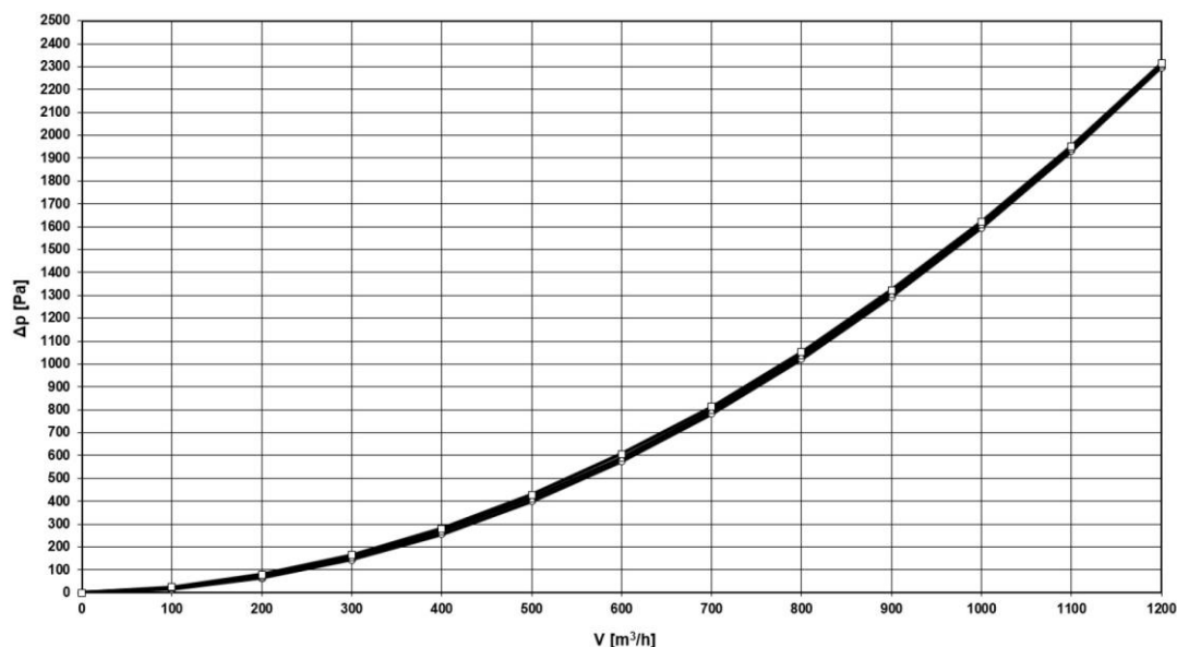
Afb. 88: Drukverliesschema
