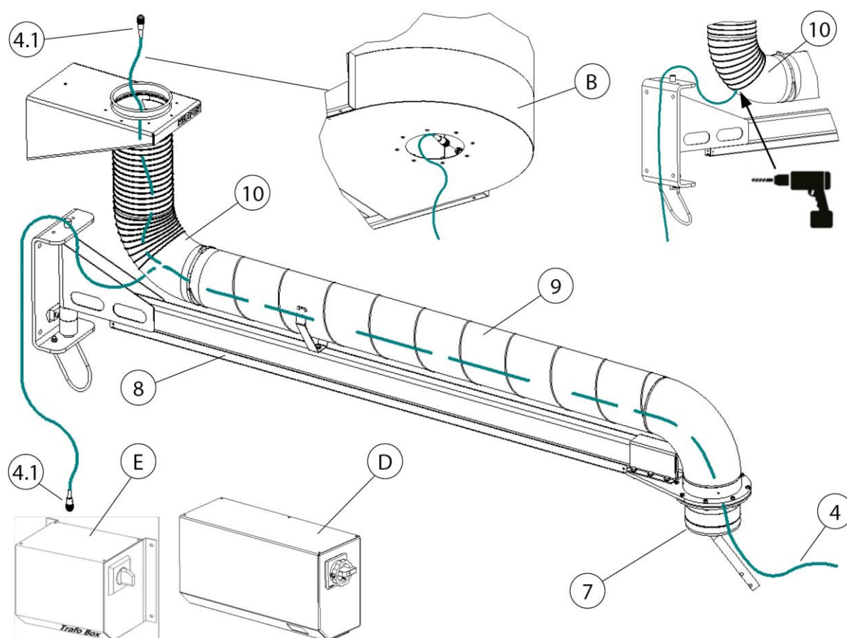
Rys. 193: Układanie kabla – ramiona odciągowe z wysięgnikiem
