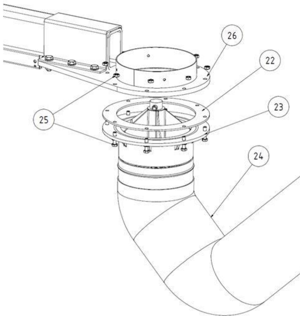
232. ábra: Elszívókar a hosszabbítókaron
