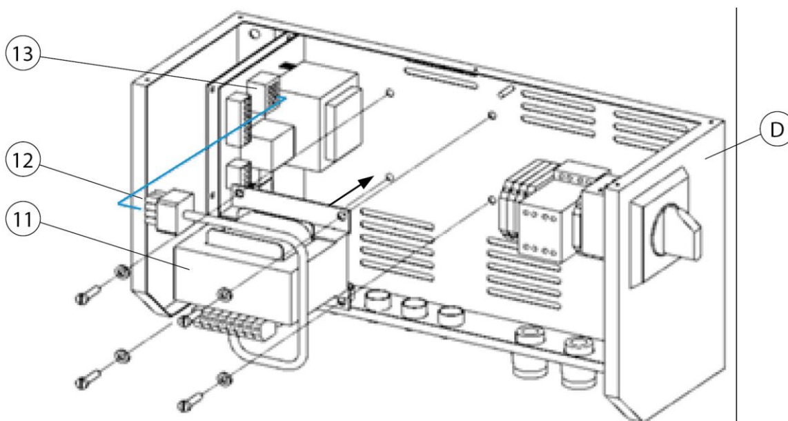
Fig. 62 : Rééquipement du transformateur dans le Control-Box (boîtier de commande)
