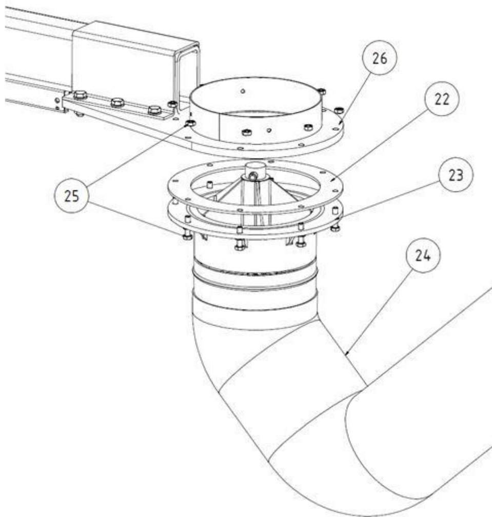
Afb. 78: Afzuigarm op de giekarm
