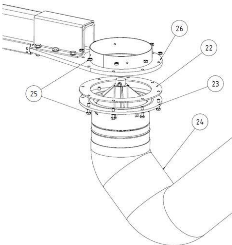
Рис. 210: Вытяжной рукав на консоли
