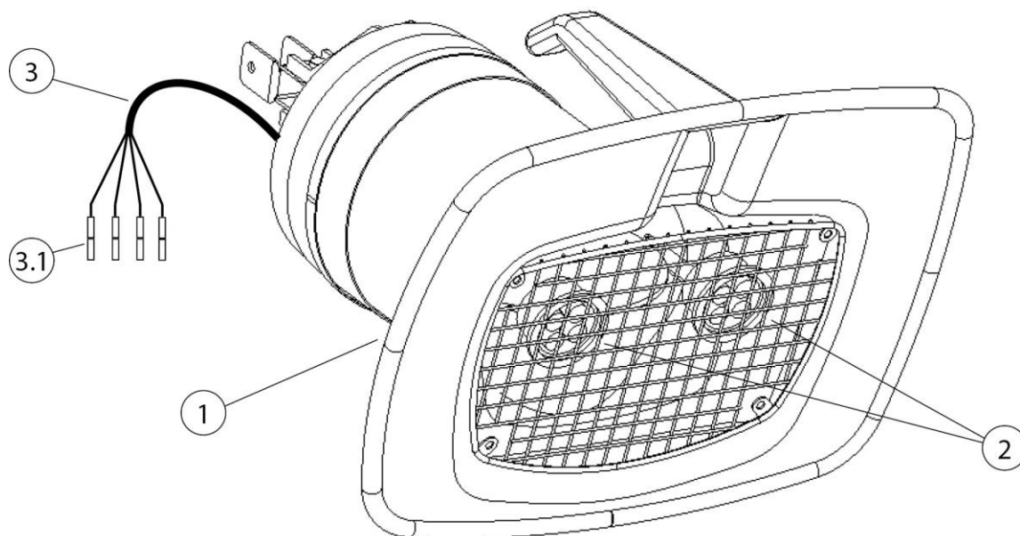
239. ábra: Világítással ellátott szívóbúra
