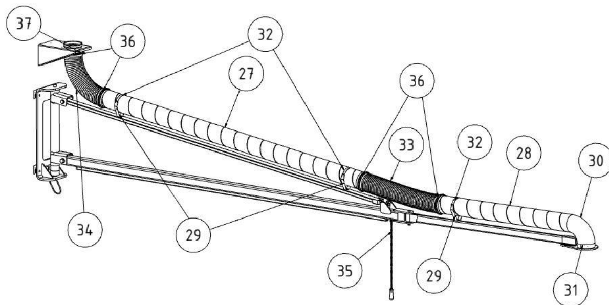
Fig. 58 : montage du tuyau agrafé
