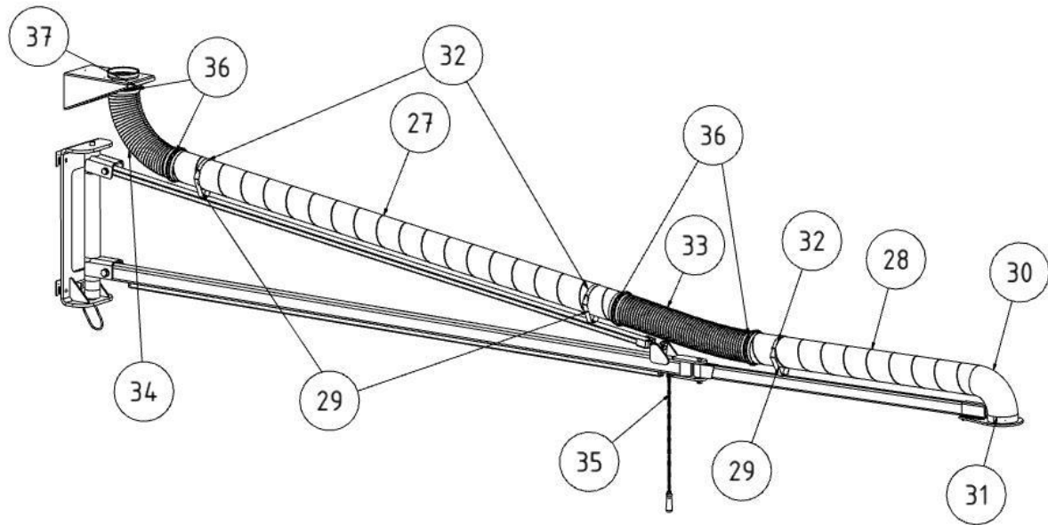
Abb. 14: Wickelfalzrohr montieren
