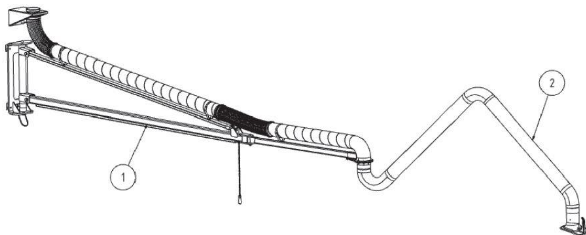
Obr. 155: Odsávací rameno s výkyvnou konzolou
