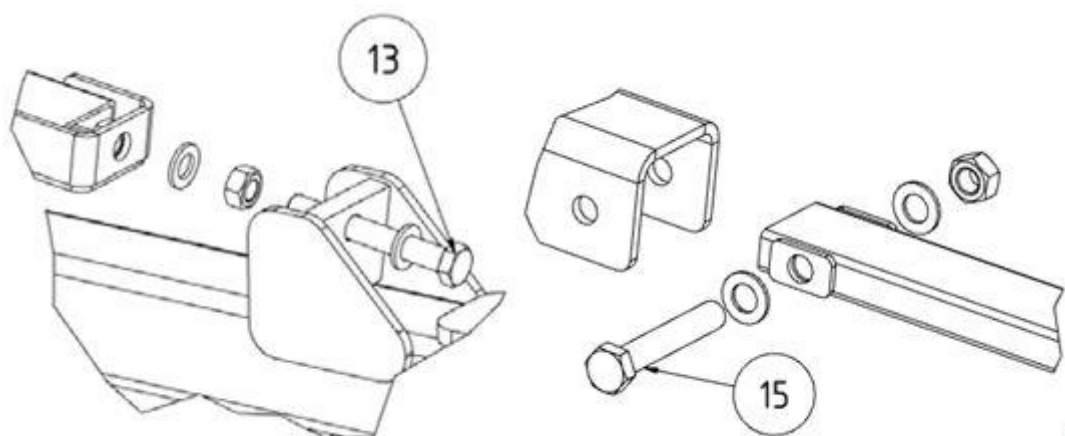
Abb. 8: Auslegerarm
