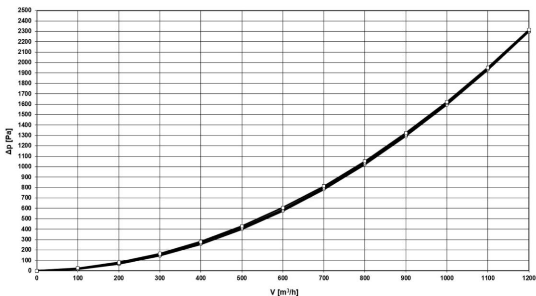
Fig. 154: Diagramma della perdita di pressione
