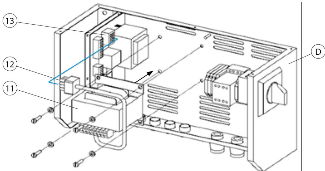
Abb. 18: Control-Box – Transformator nachrüsten
