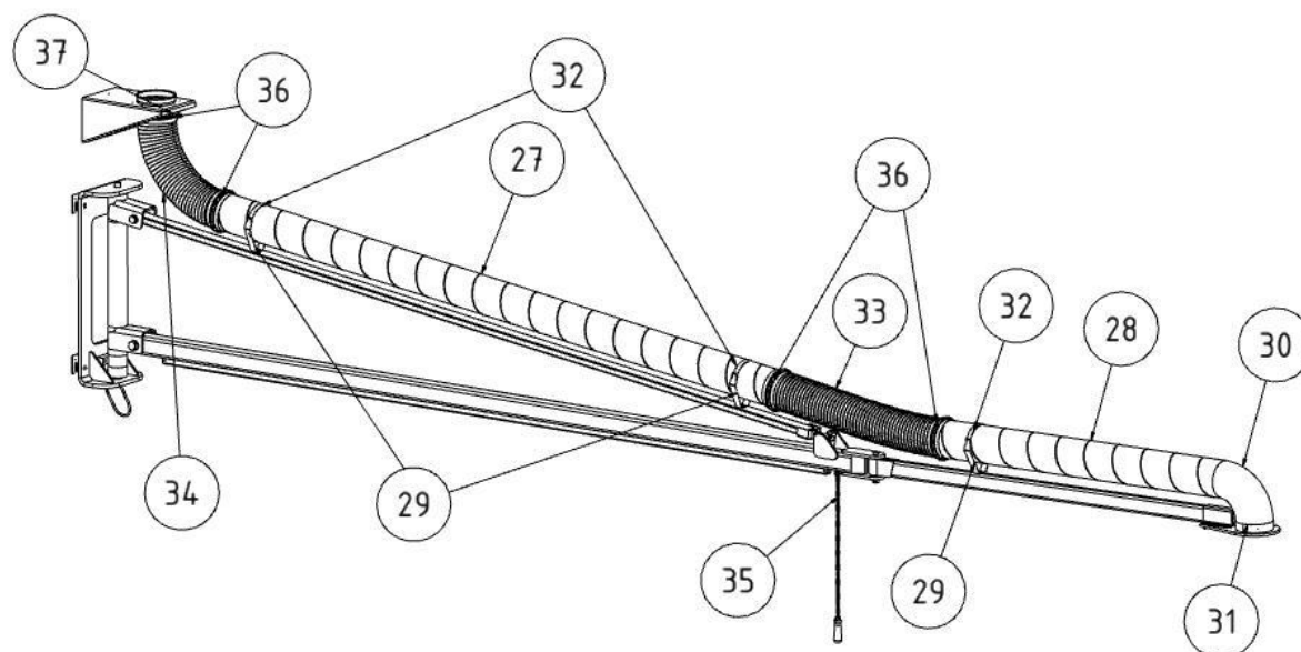
Fig. 124: Montar a conduta espiralada
