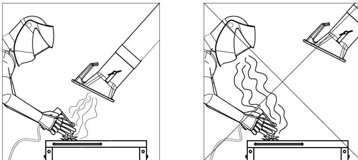
Sl. 263: Nameščanje odsesovalnega pokrova
