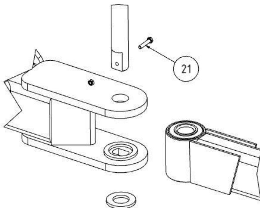
Рис. 209: Соедините консоли друг с другом
