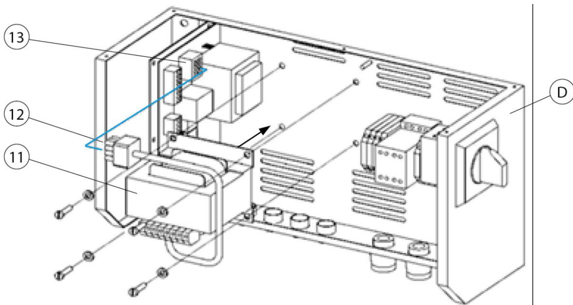
Fig 106: Control-Box - Reequipar transformador
