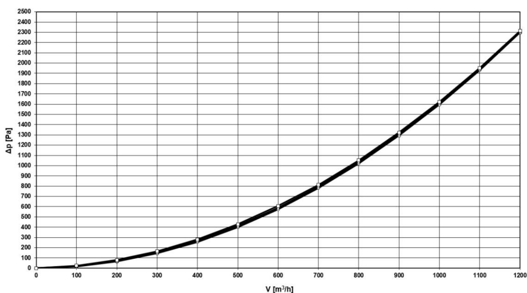
Obr. 176: Graf tlakové ztráty
