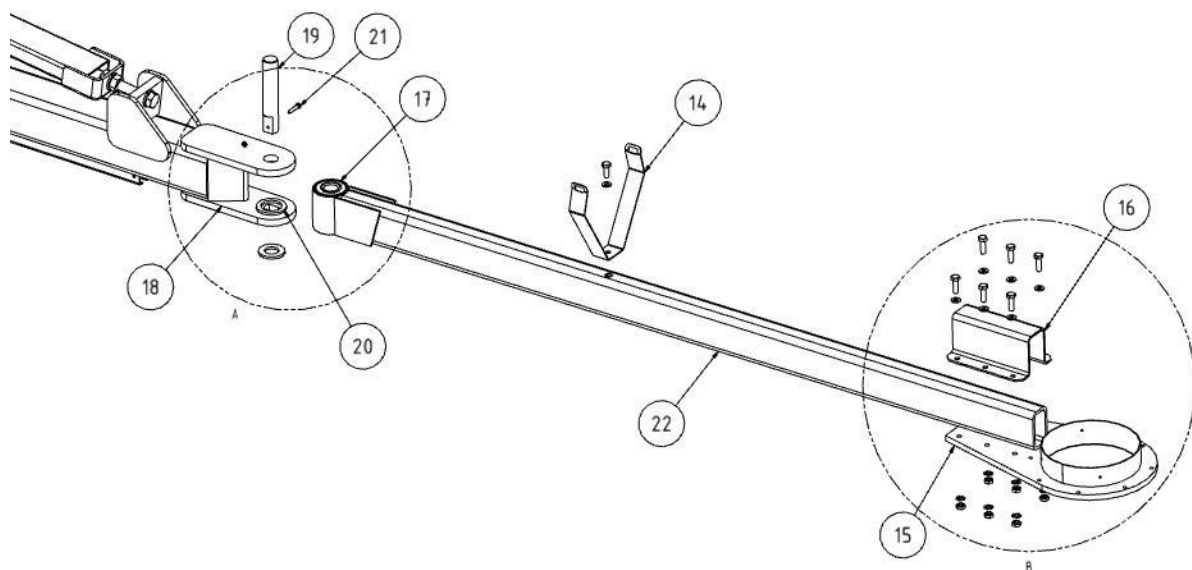
Fig. 97: Brazo pluma parte 2
