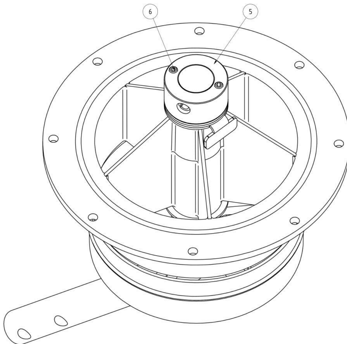
Rys. 189: Hamulec
