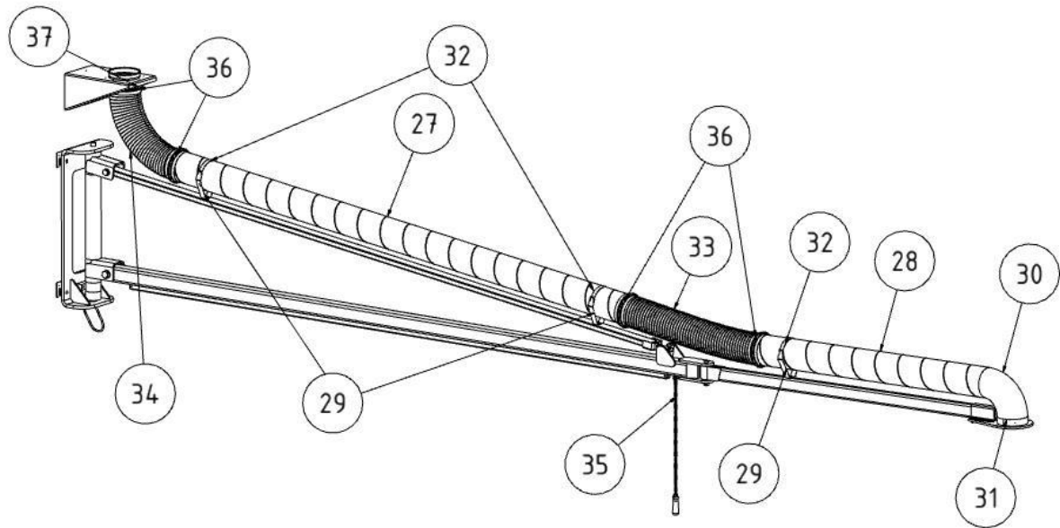
Afb. 80: Spiraalbuis monteren
