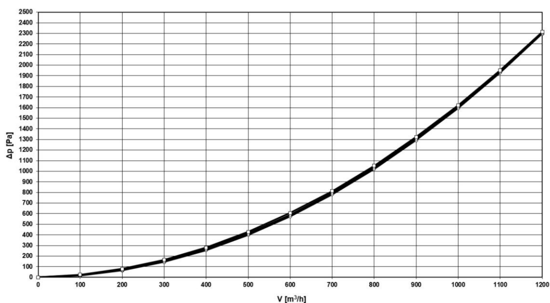
Rys. 198: Wykres strat ciśnienia
