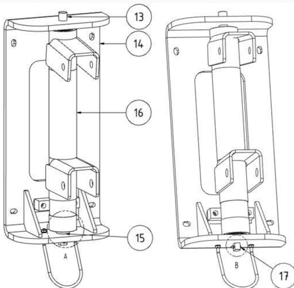
Fig. 50 : support de la potence
