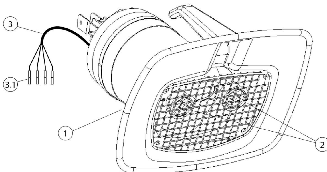
Rys. 195: Okap odciągowy z oświetleniem
