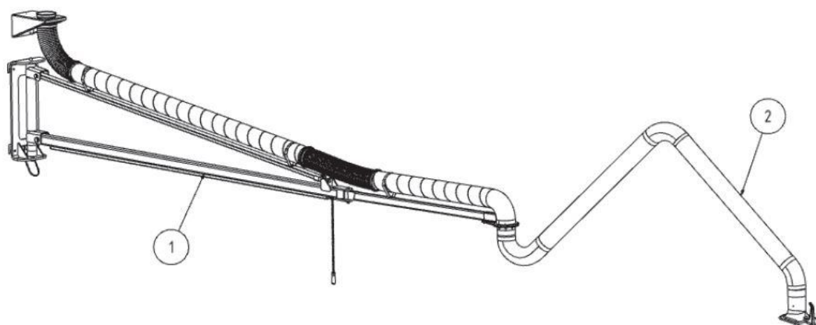
Rys. 179: Ramię wyciągnika z ramieniem odciągowym
