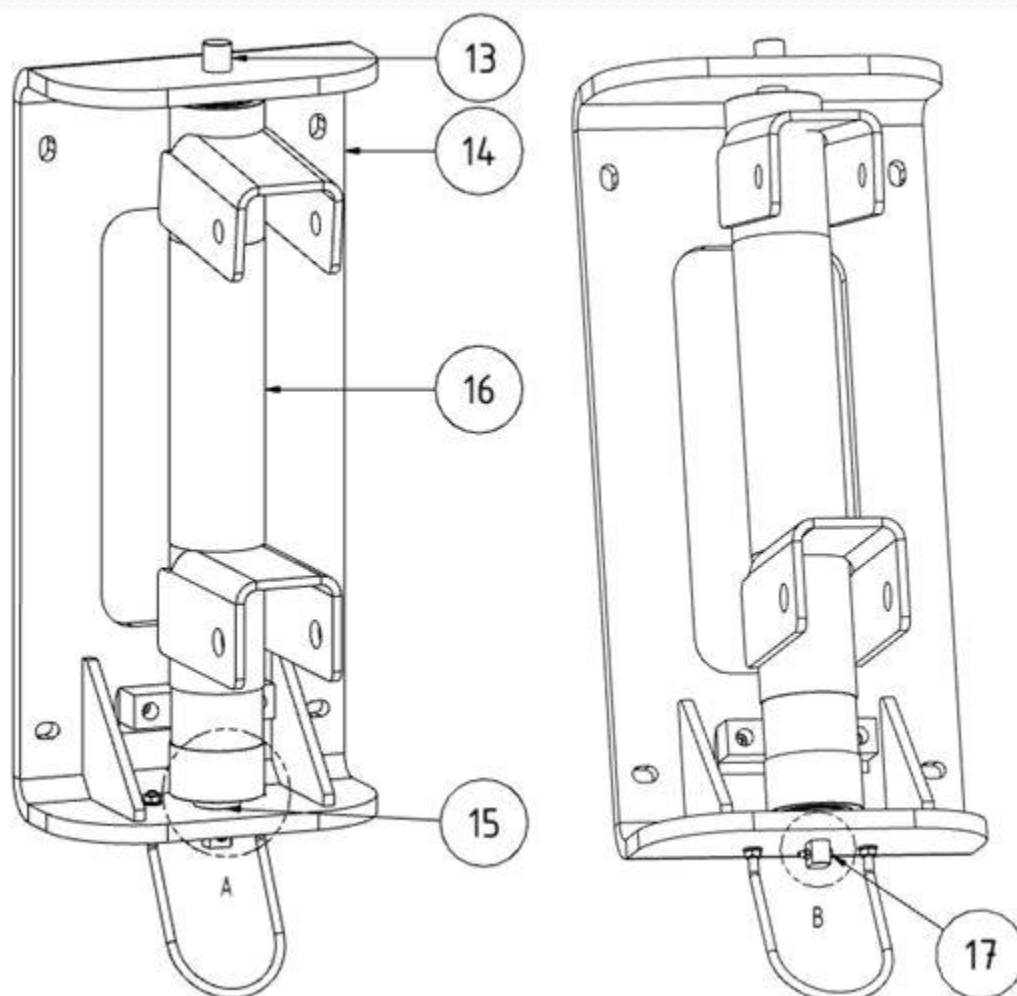
Rys. 182: Uchwyt ramienia wysięgnika
