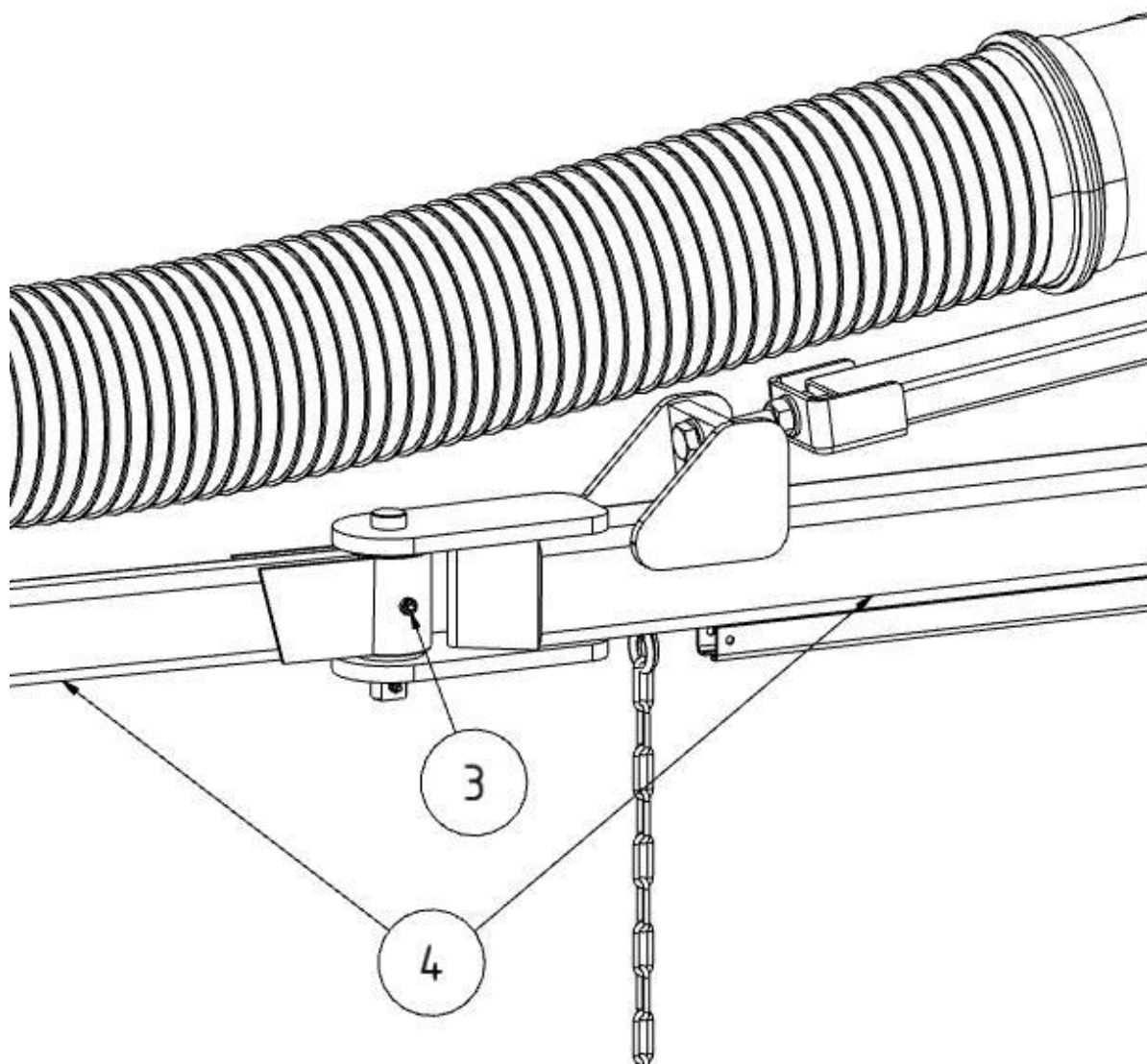
Obr. 170: Brzdíčka
