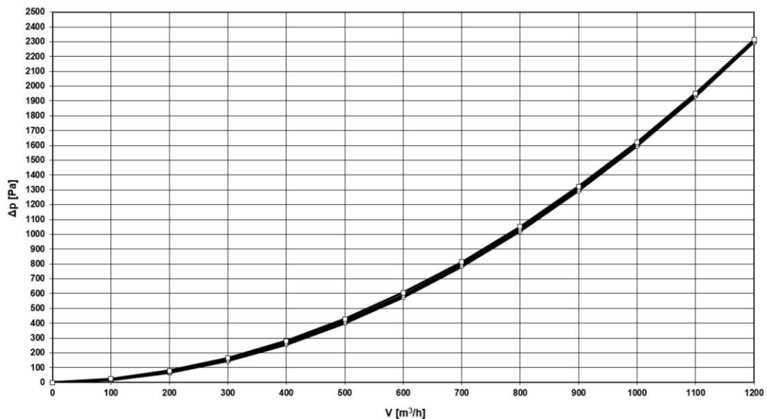
Abb. 22: Druckverlustdiagramm
