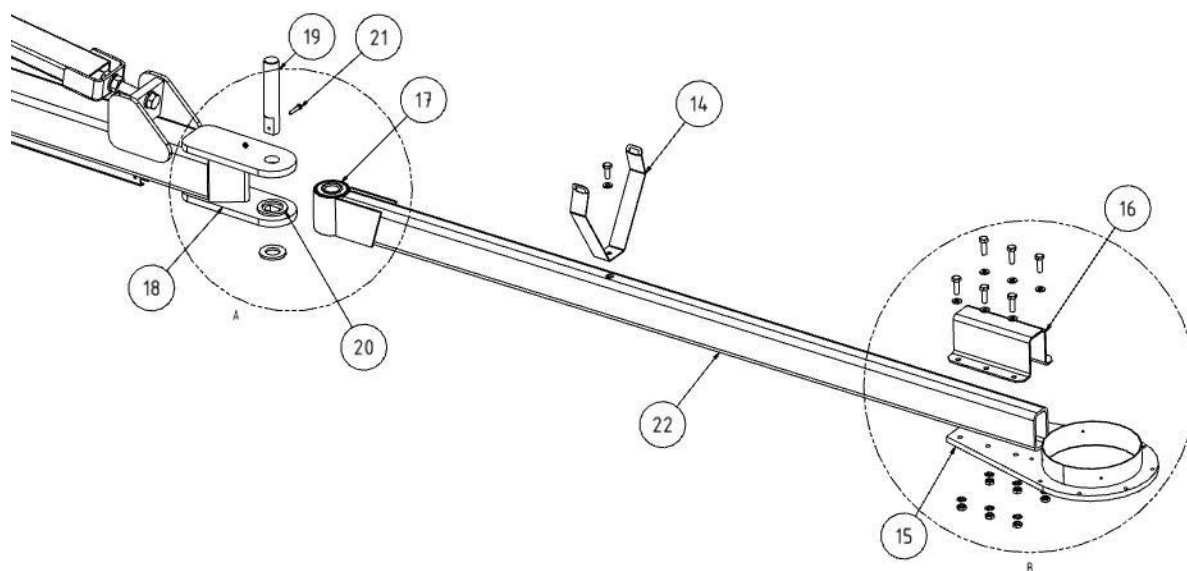
Рис. 207: Поворотная консоль, часть 2
