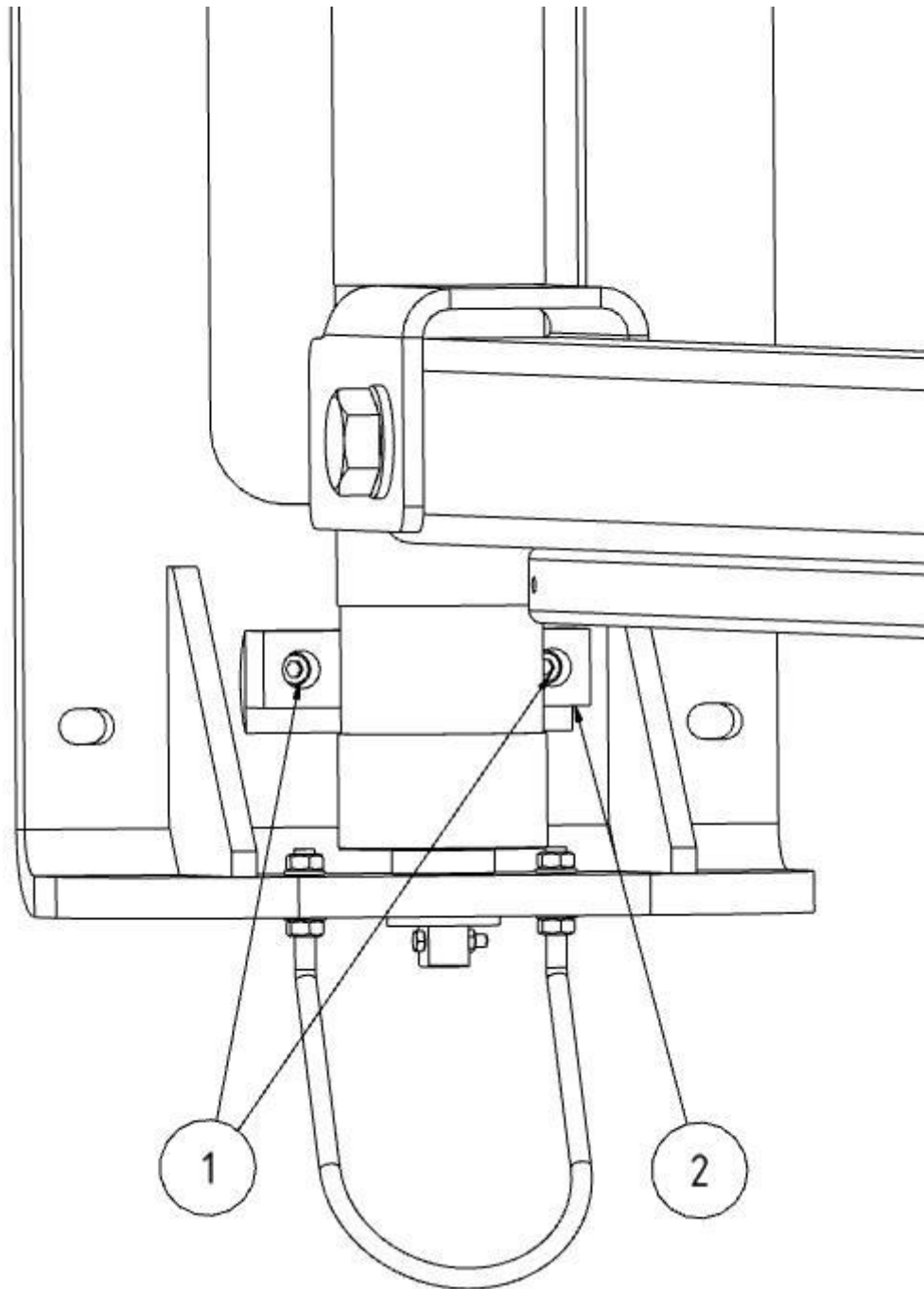
Afb. 81: Rem
