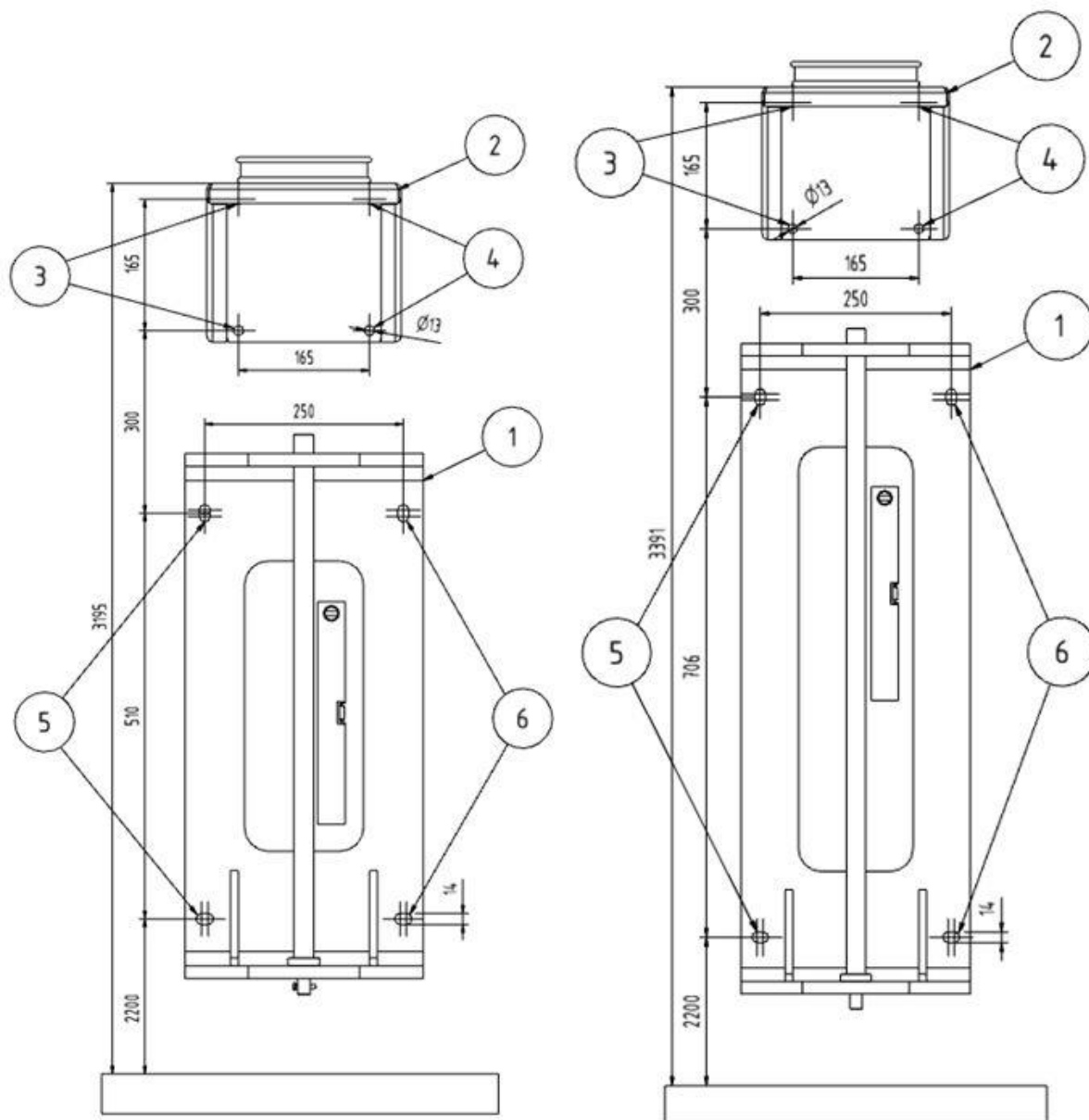
Afb. 71: Wandconsole
