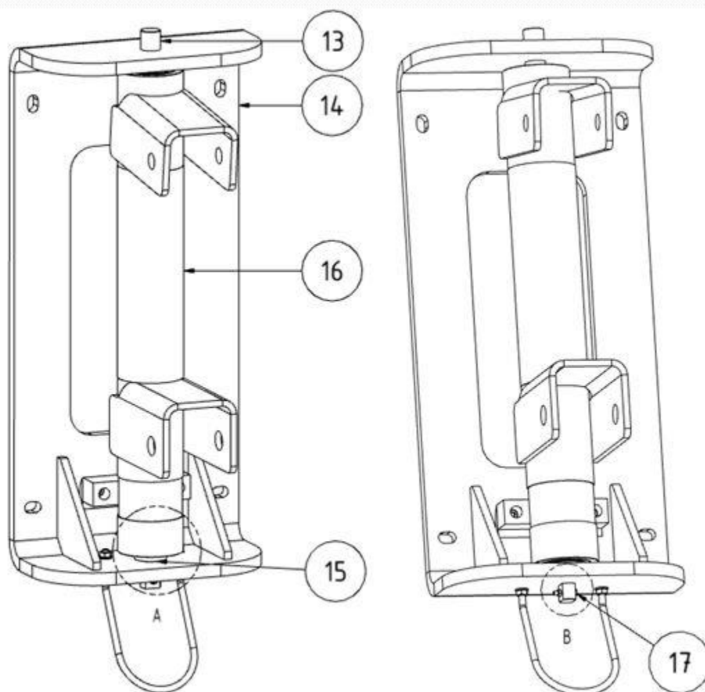
Obr. 160: Držák výkyvné konzoly
