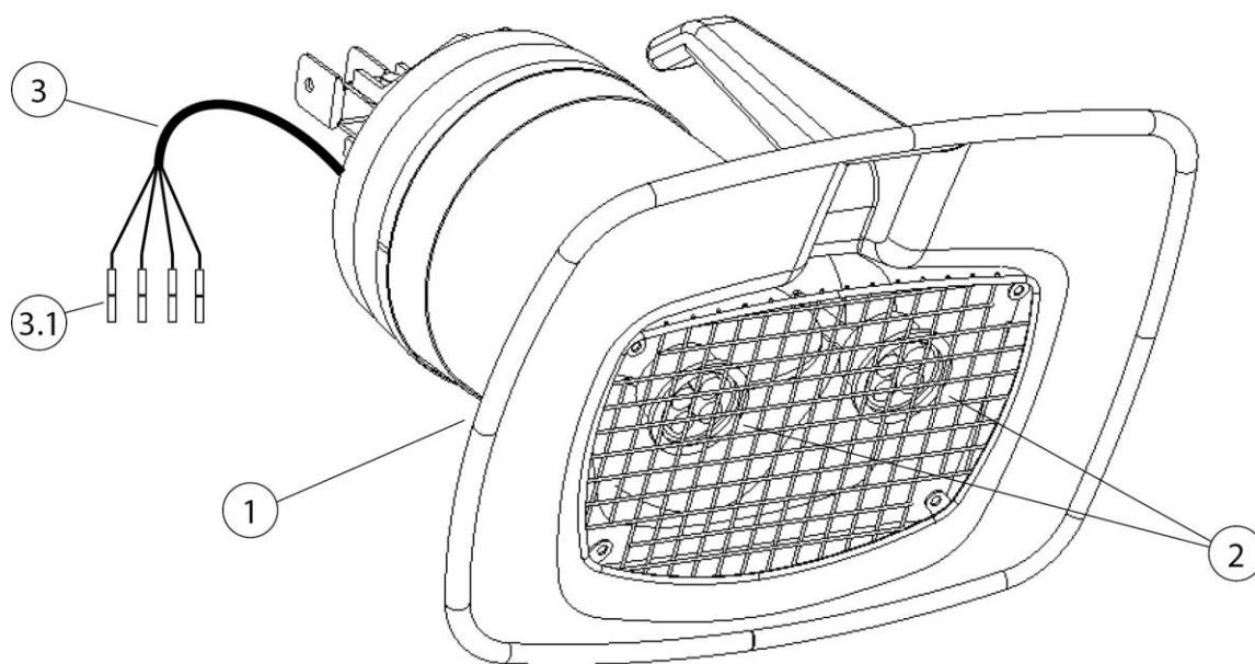
Рис. 217: Вытяжной колпак с подсветкой
