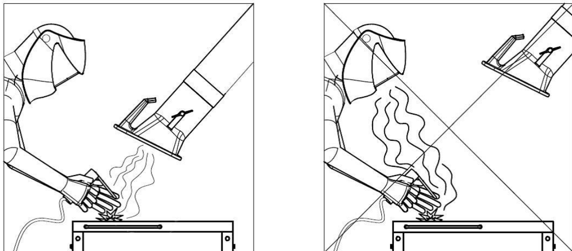
241. ábra: Az elszívóbura pozicionálása
