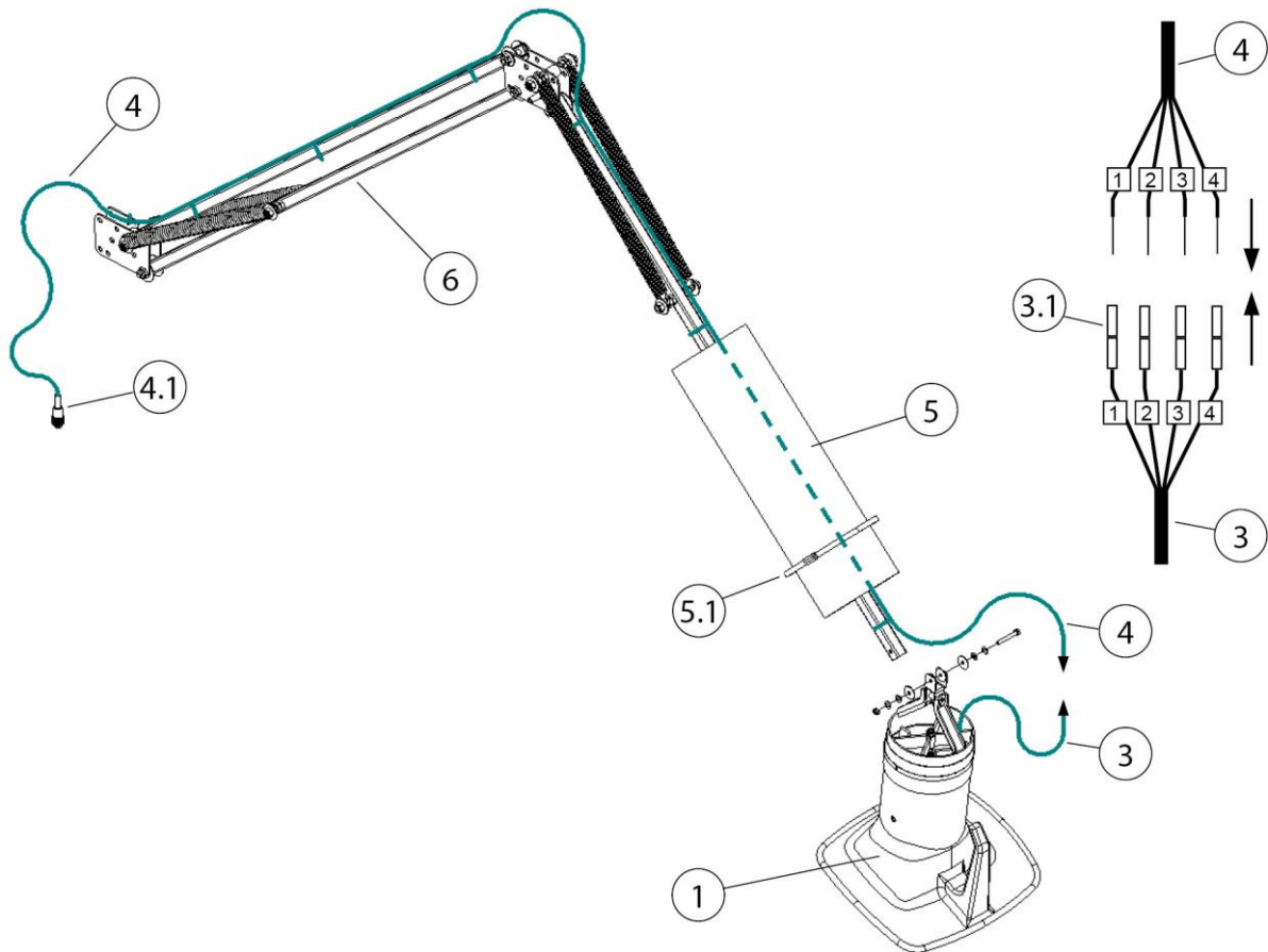
Abb. 20: Kabelverlegung - Absaugarm 2-4 Meter
