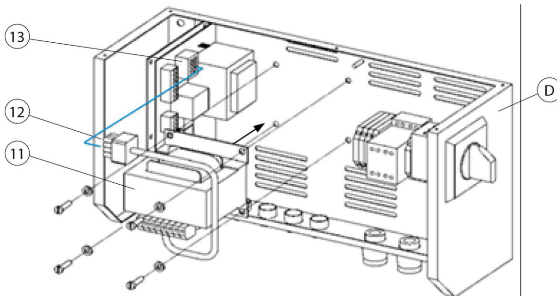
Obr. 172: Řídící skříň - dodatečný transformátor
