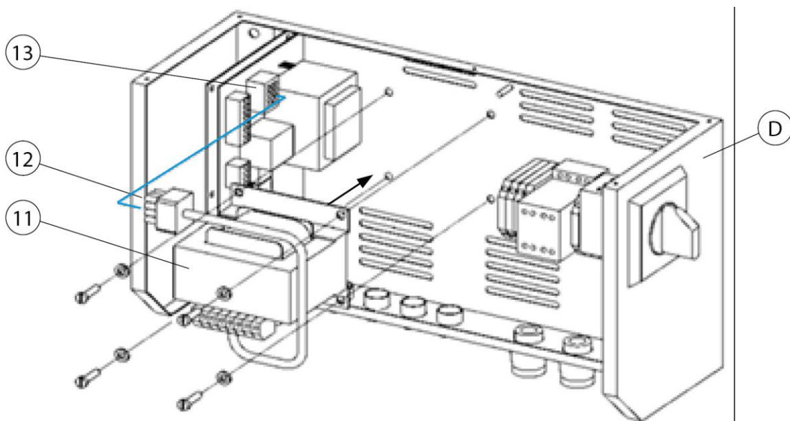
Afb. 84: Control-Box – transformator achteraf uitrusten
