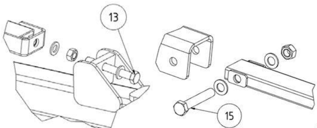
Fig. 96: Brazo pluma
