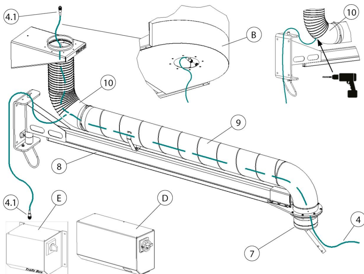
Fig 105: Tendido de cable – Brazos de aspiración con pescante para grúa
