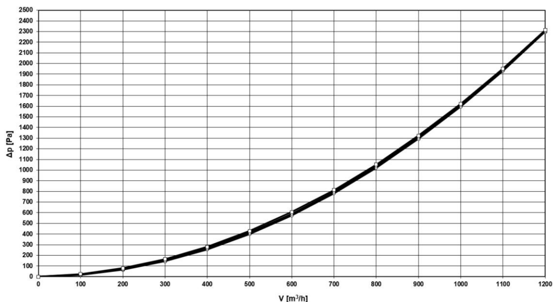
242. ábra: Nyomásvesztési diagram
