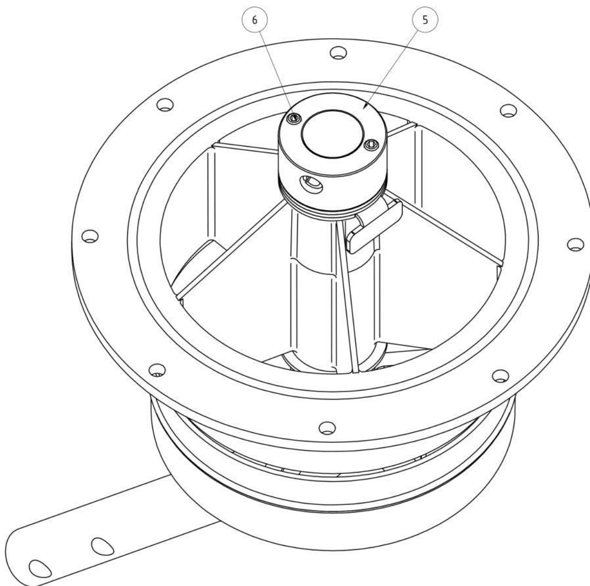
Sl. 255: Zavora
