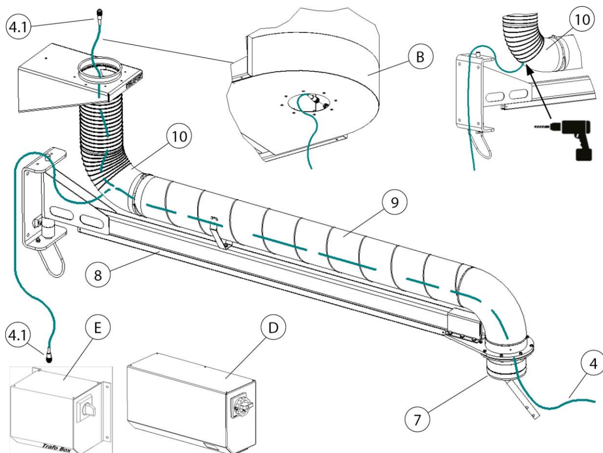
Sl. 259: Polaganje kabla – sesalna roka s krakom žerjava
