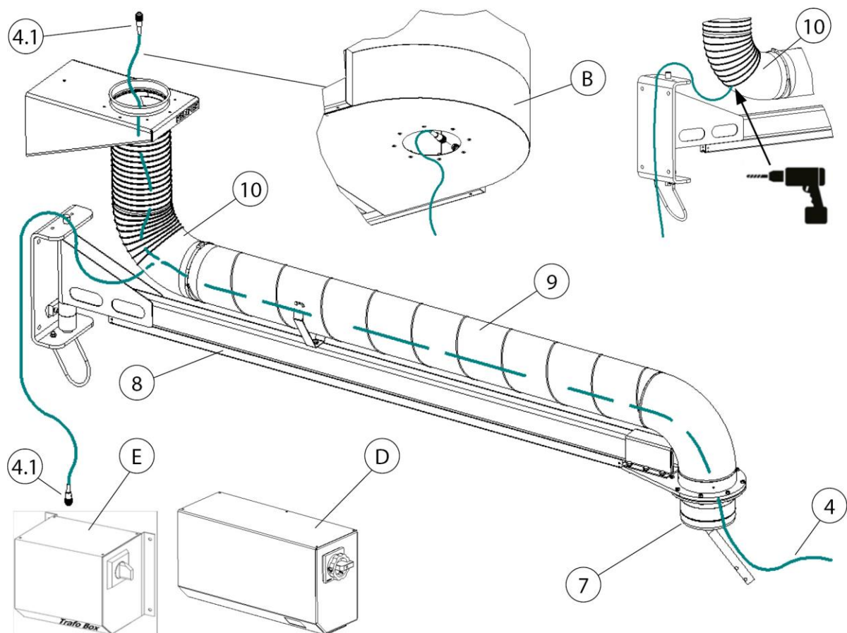
Fig. 61 : Pose des câbles – bras d'aspiration avec potence
