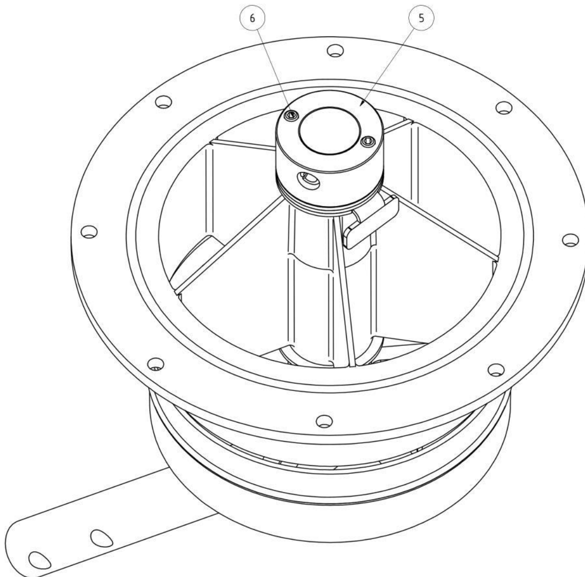
Fig. 101: Freno
