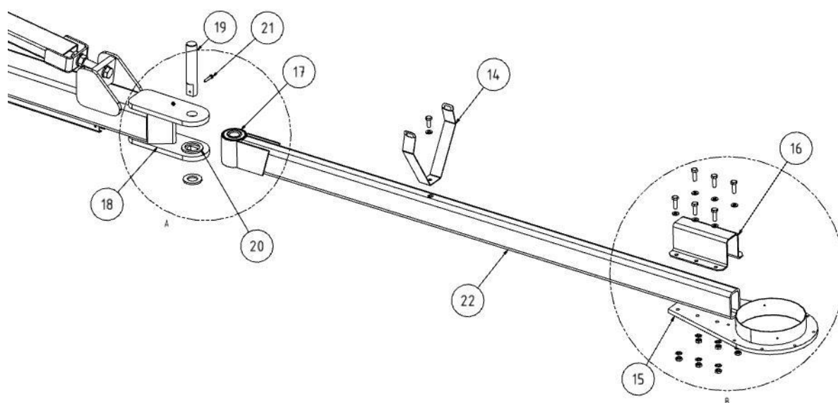
Fig. 141: Braccio a sbalzo Parte 2
