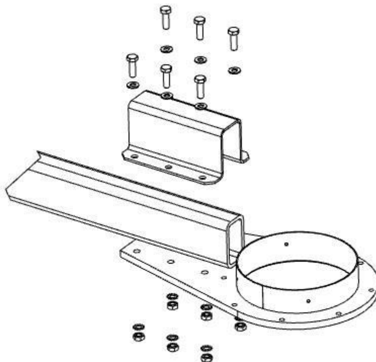
Рис. 208: Монтаж держателя вытяжного рукава
