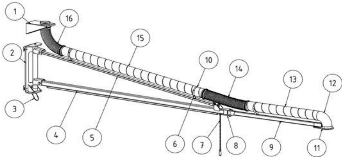
Abb. 2: Auslegerarm
