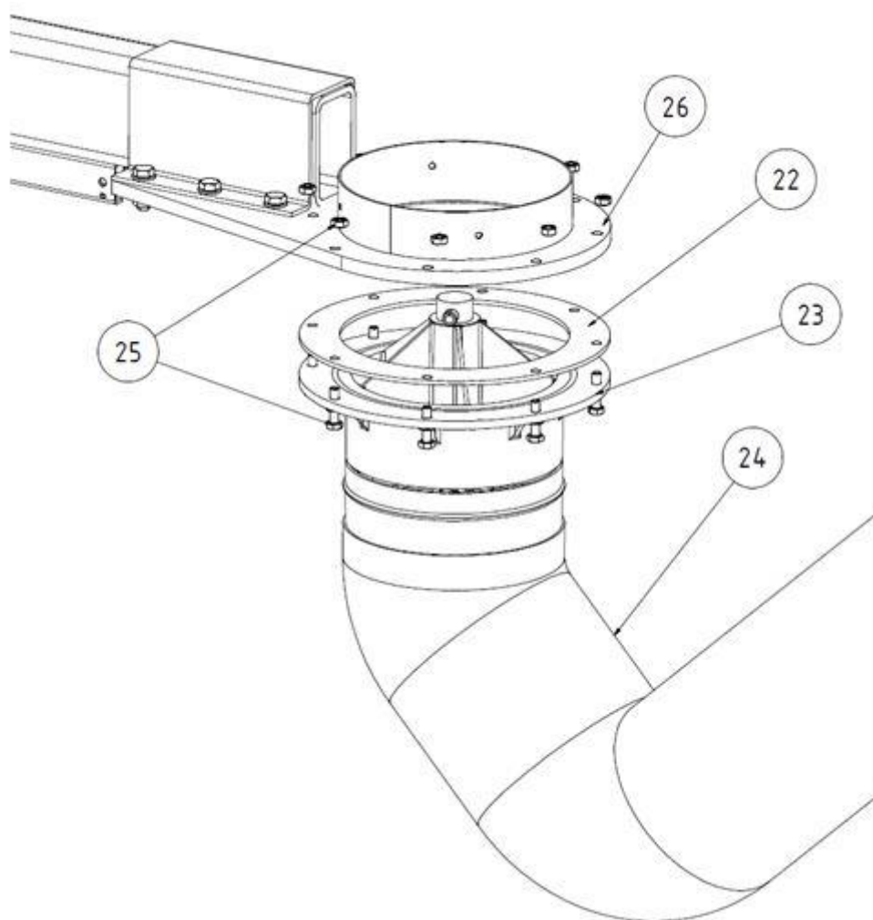
Obr. 166: Odsávací rameno s prodlužovacím ramenem
