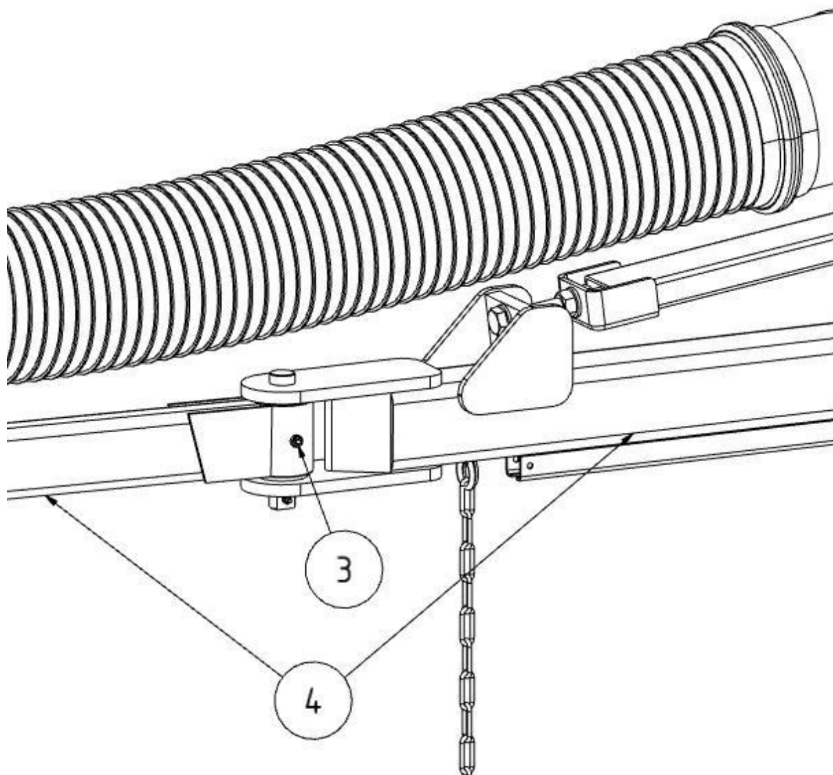
Sl. 258: Zavora
