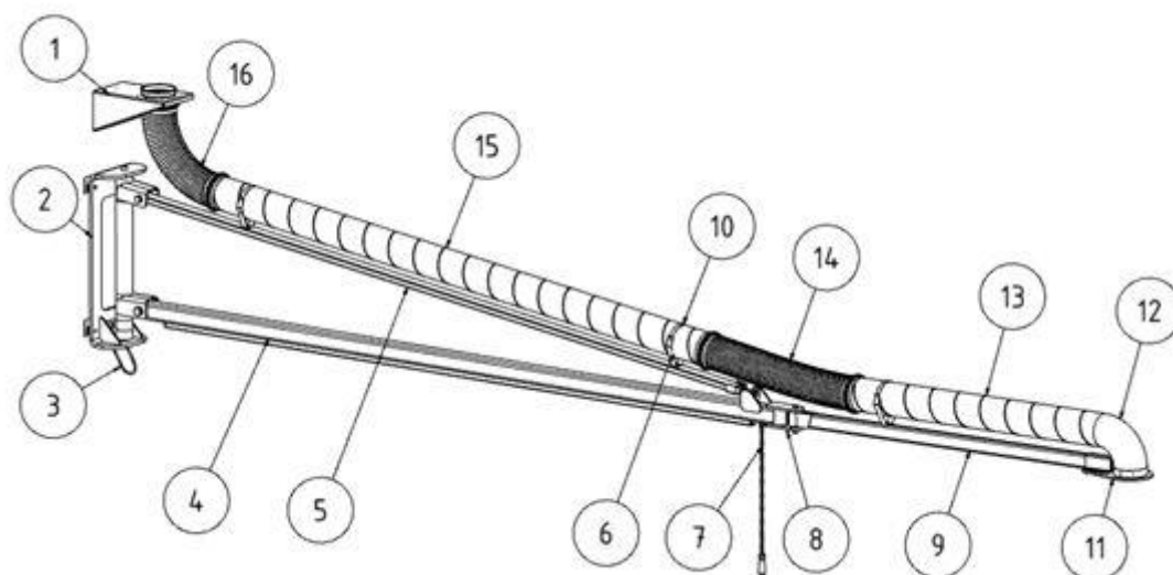
Fig. 136: Posizioni sul prodotto
