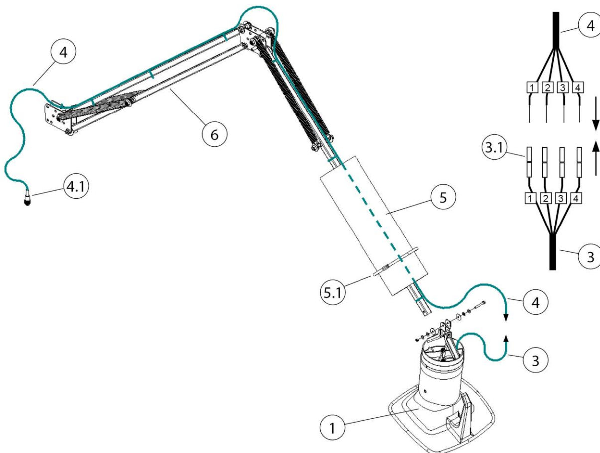
Sl. 262: Polaganje kabla – sesalna roka 2–4 metre
