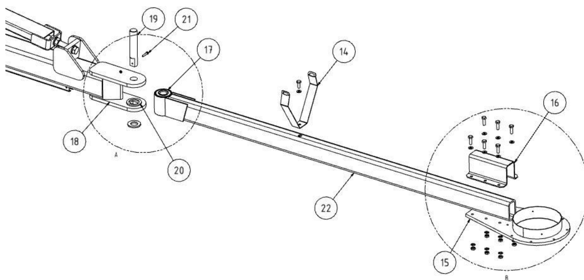
Fig. 119: Braço da lança 2.ª parte
