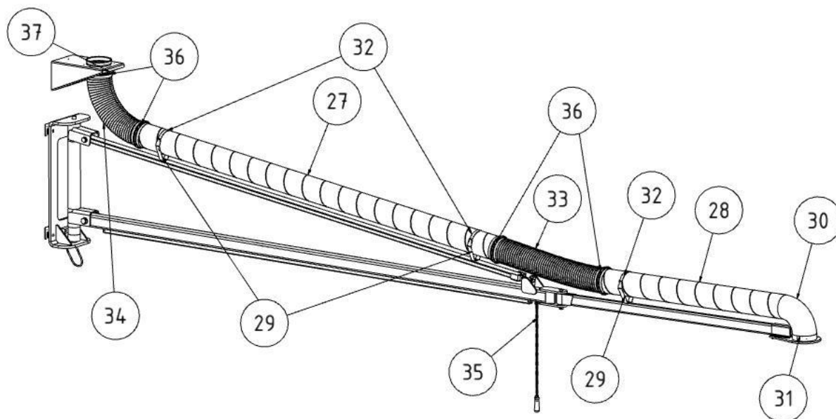
Rys. 190: Montaż rury zwijanej felcowanej
