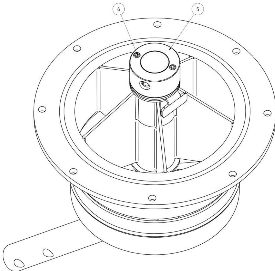
Рис. 211: Тормоз
