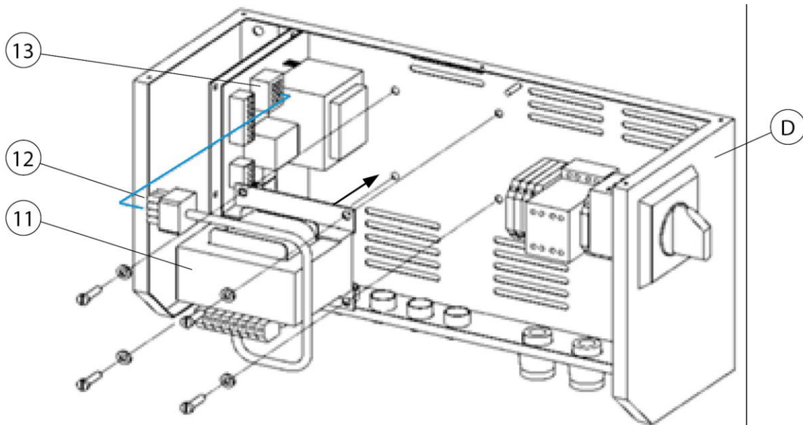
Sl. 260: Nadzorna omarica – dodatna vgradnja transformatorja
