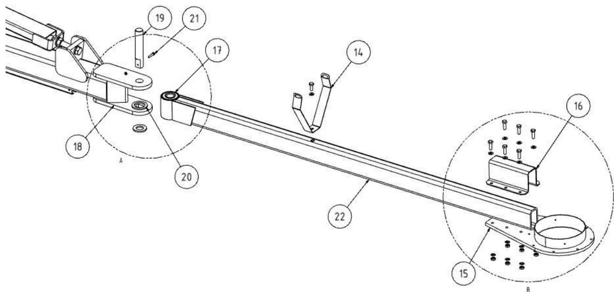
Fig. 53 : potence, partie 2
