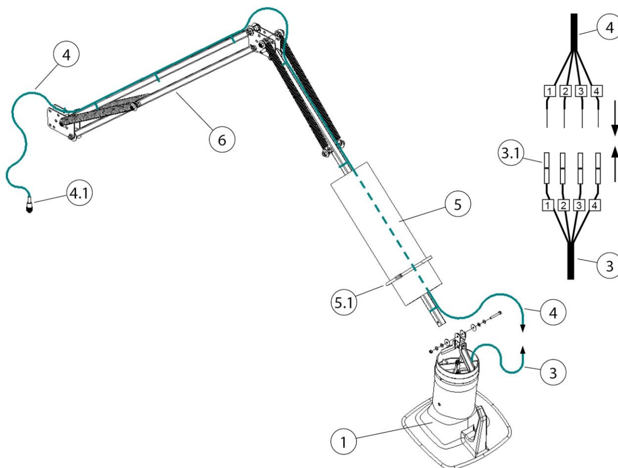
Rys. 196: Układanie kabla – ramię odciągowe 2-4 metrów
