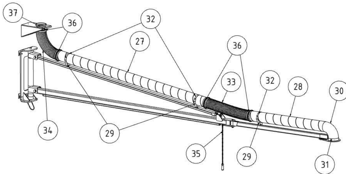
Sl. 256: Namestitev zvite gibke cevi
