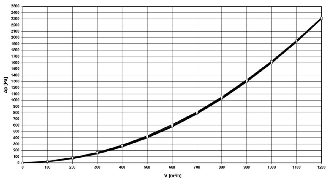
Sl. 264: Diagram izgube tlaka
