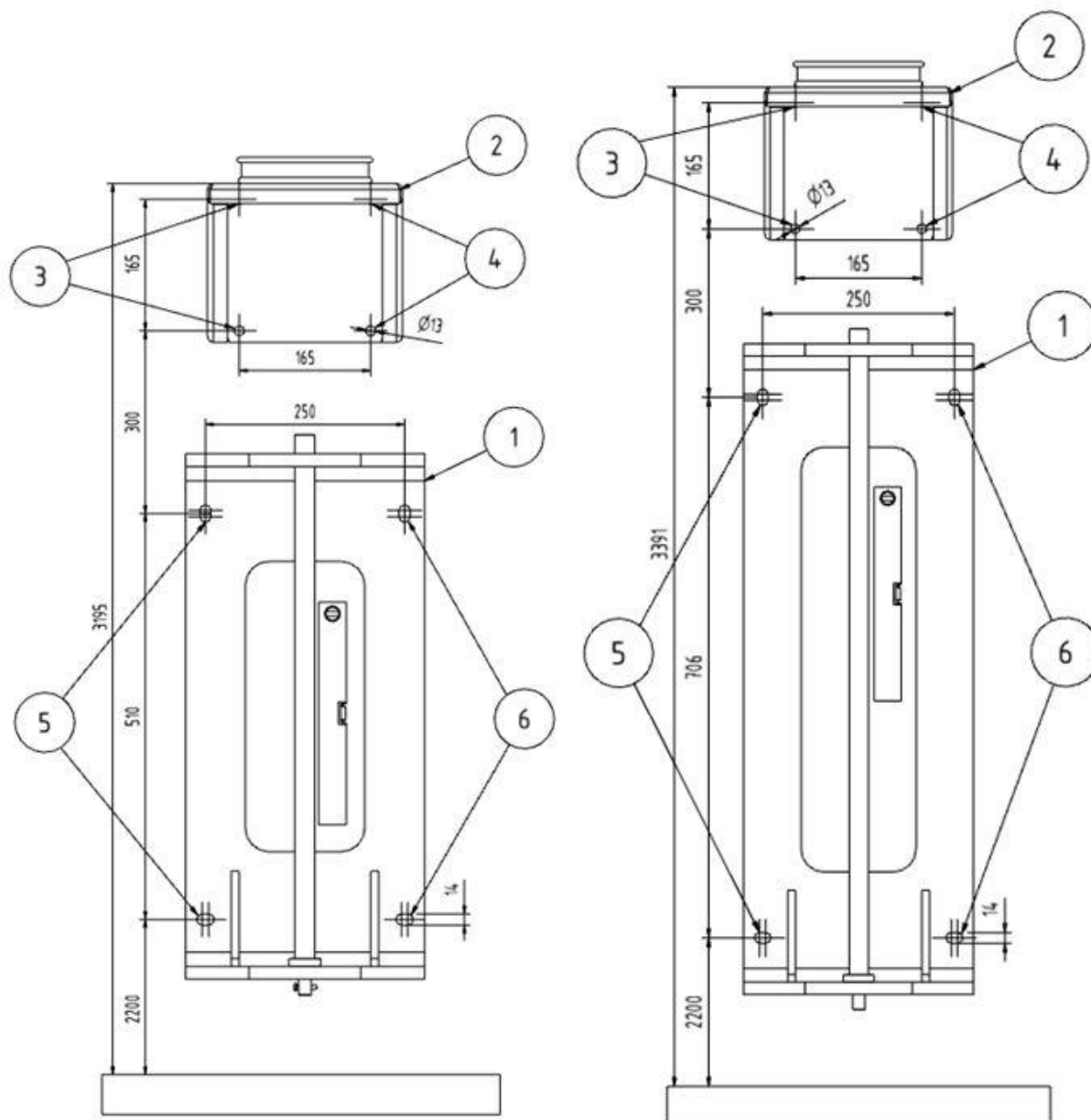
225. ábra: Fali tartó
