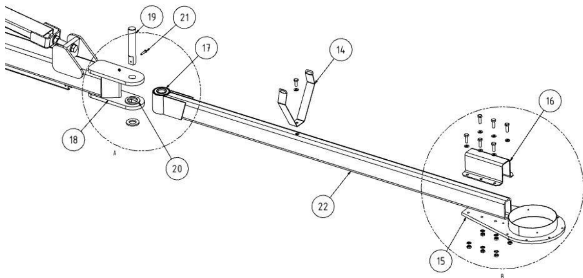
Afb. 75: Giekarm, deel 2
