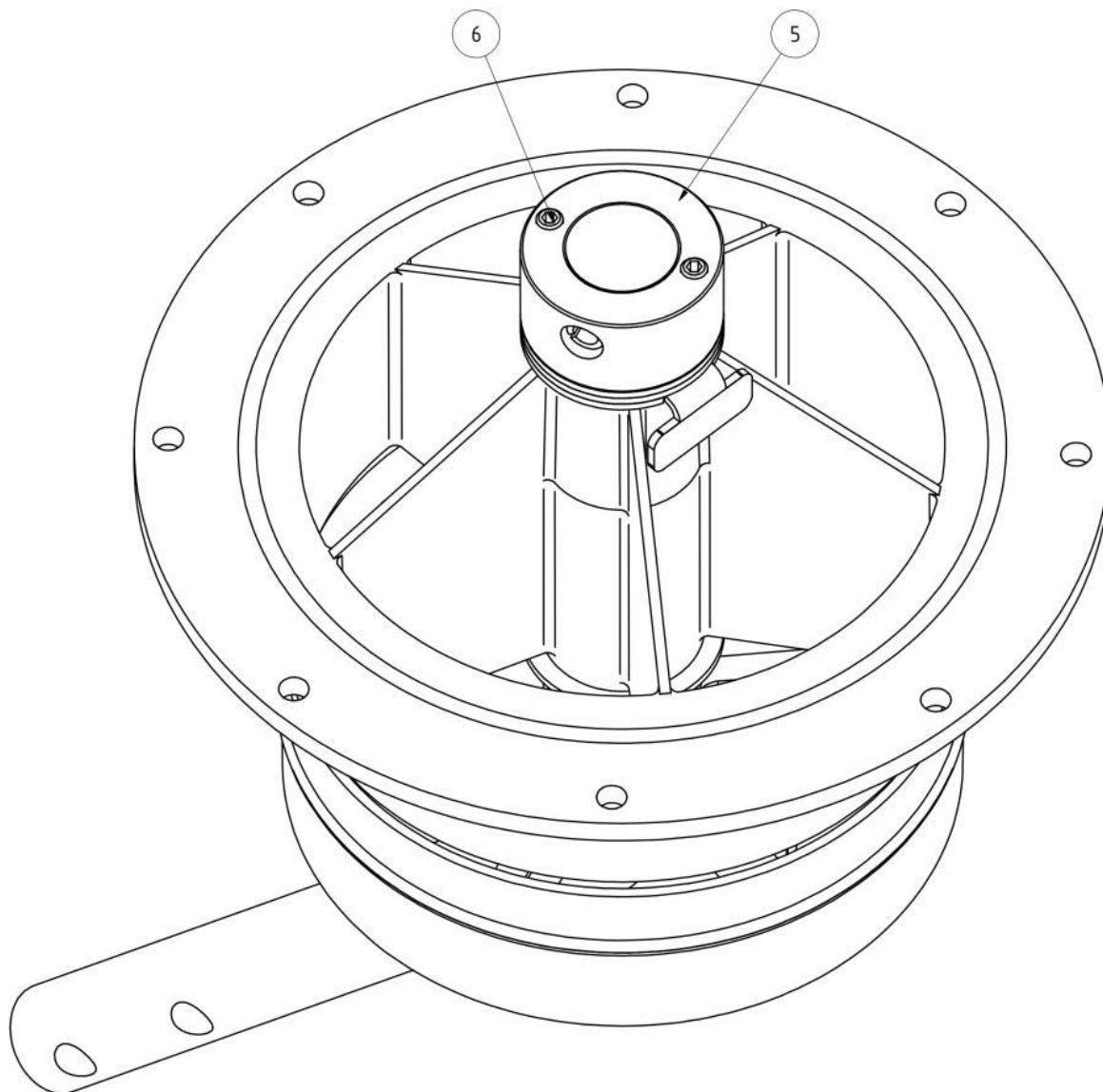
Fig. 57 : Frein
