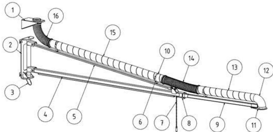
Fig. 46 : potence
