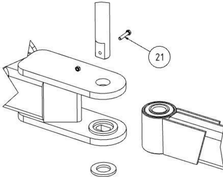
Fig. 99: Unir los brazos pluma entre sí
