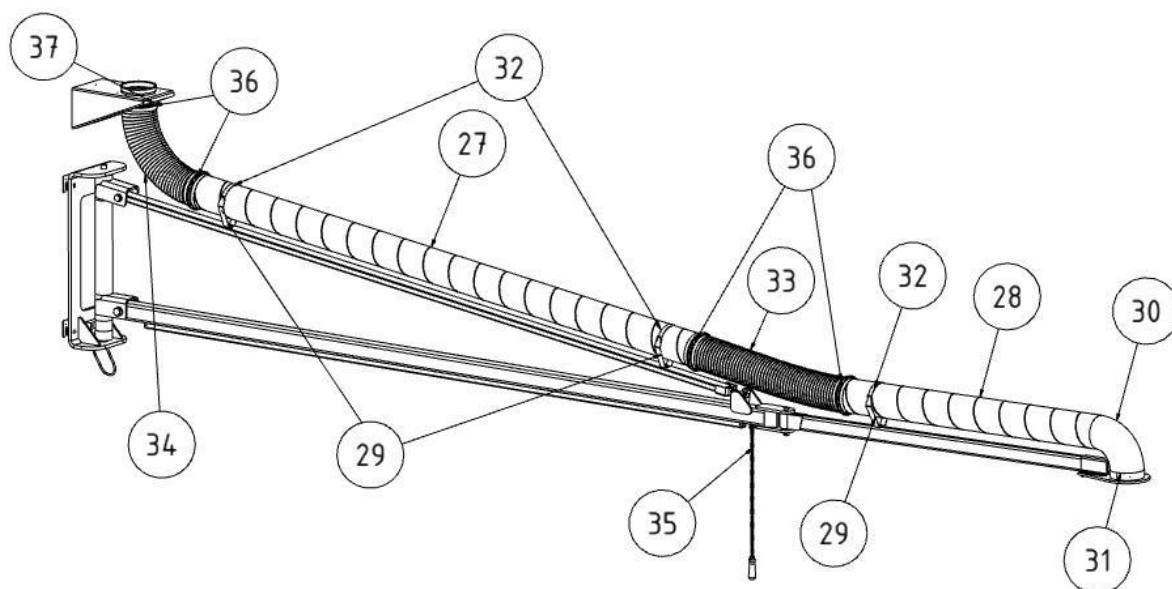
Рис. 212: Монтаж угловой фальцованной трубы
