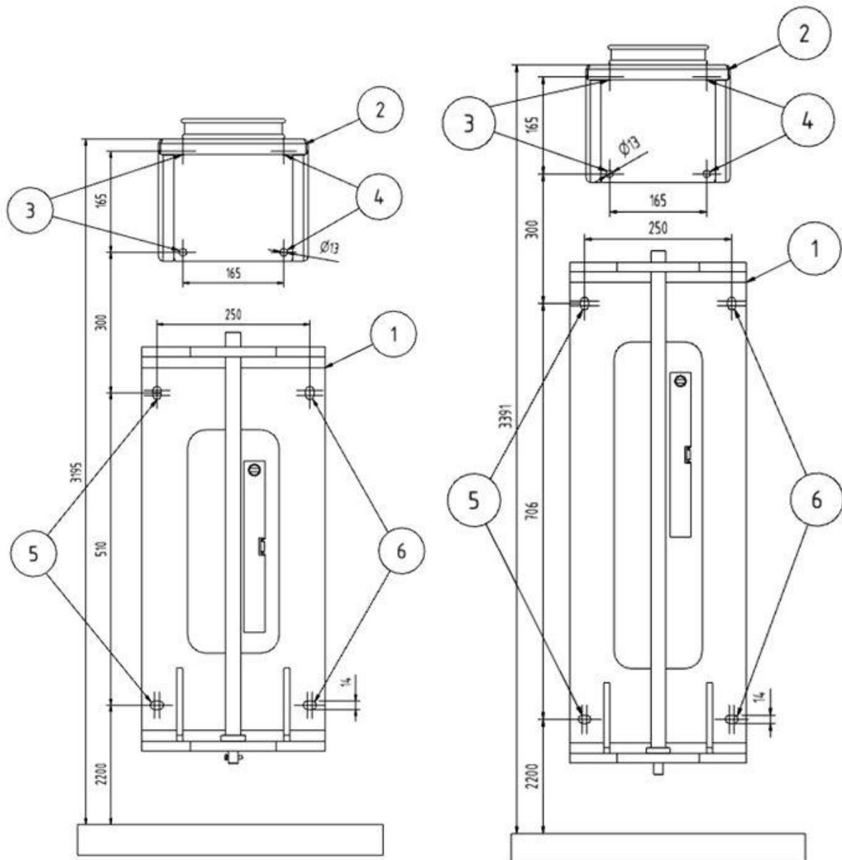
Fig. 93: Soporte de pared
