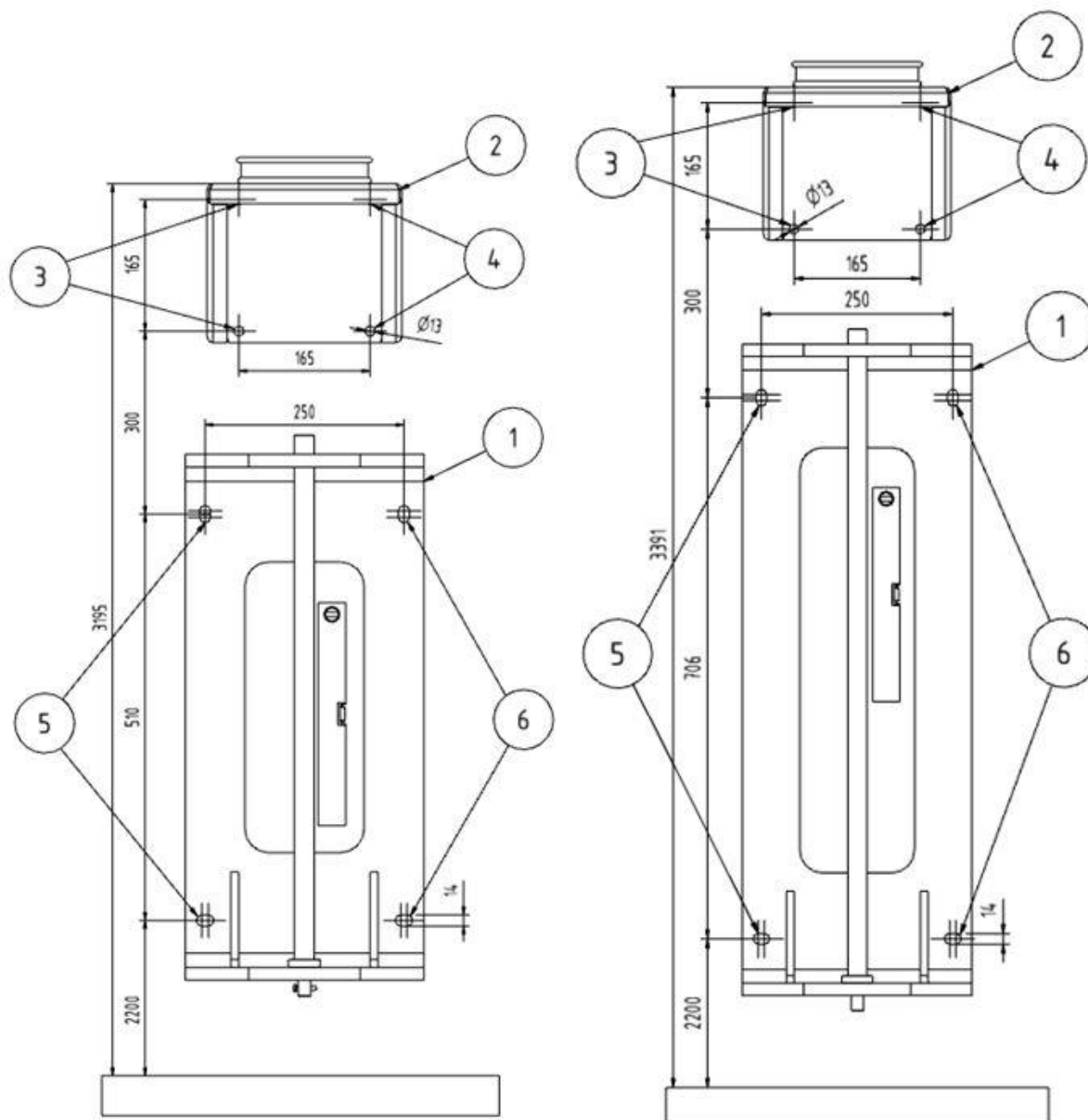
Obr. 159: Nástěnný držák
