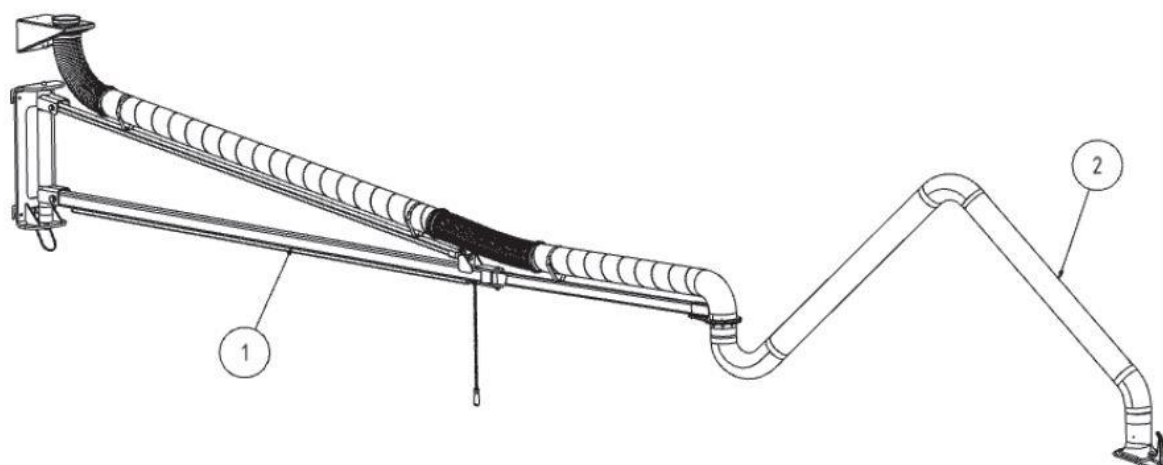
Sl. 245: Roka konzole z sesalno roko
