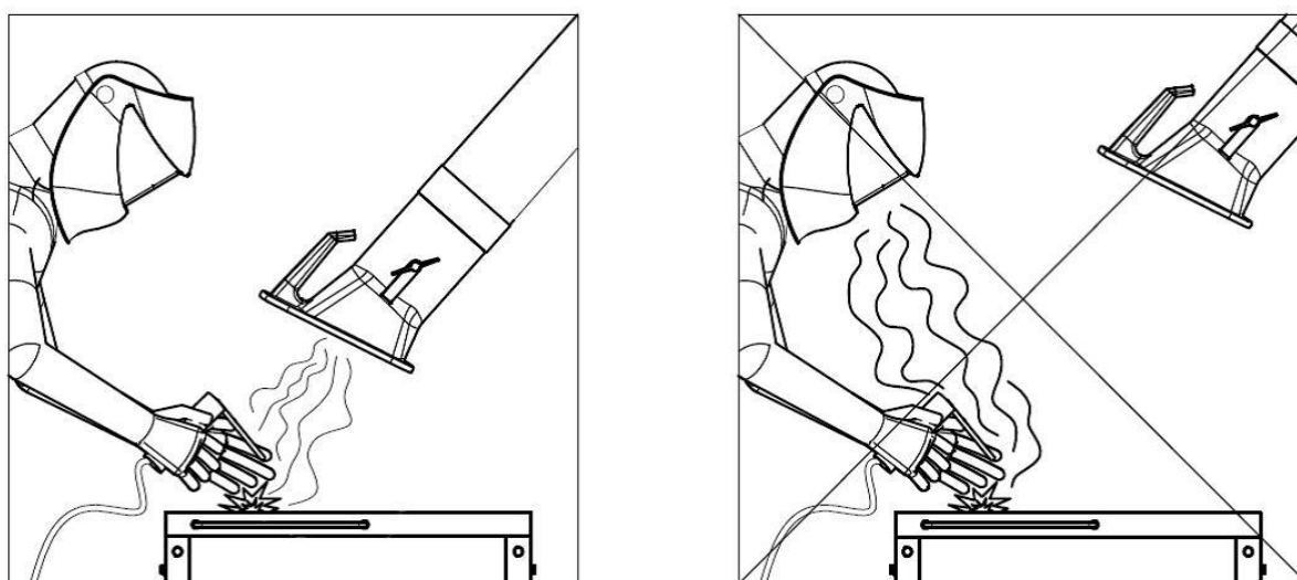
Fig. 65 : positionnement de la hotte d'aspiration
