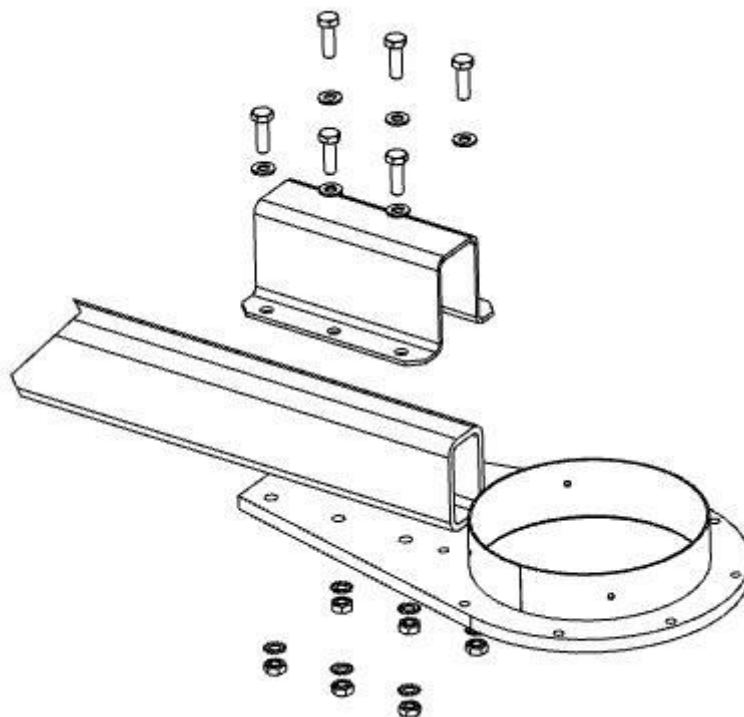
Fig. 120: Montar o suporte do braço de aspiração
