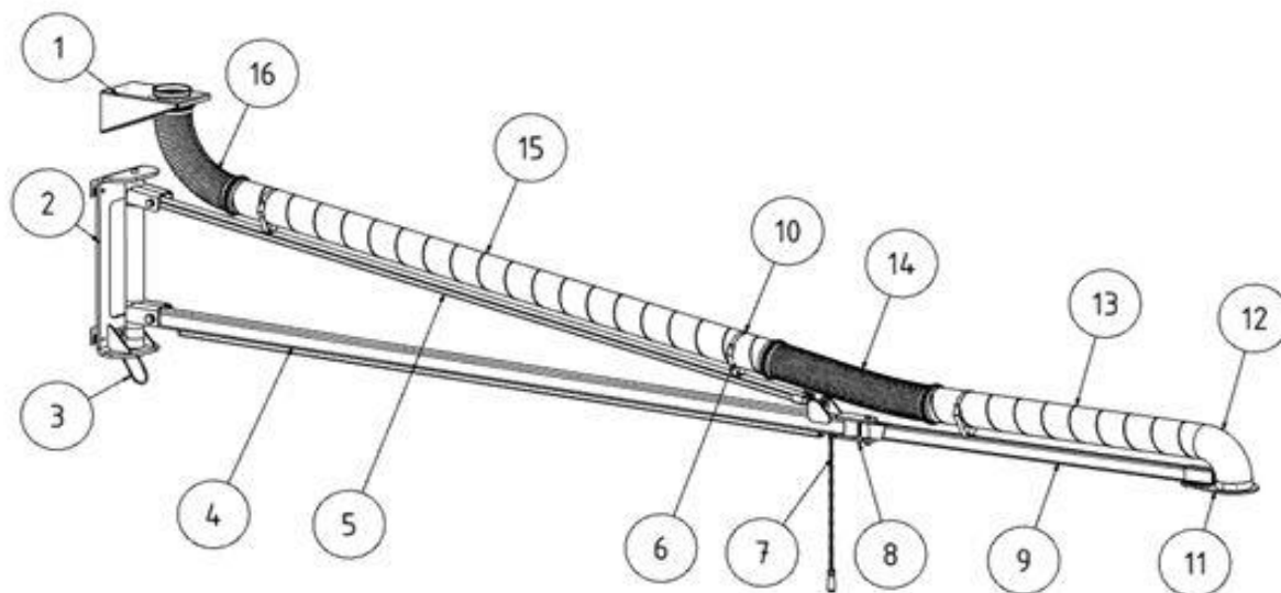
Fig. 90: Brazo pluma
