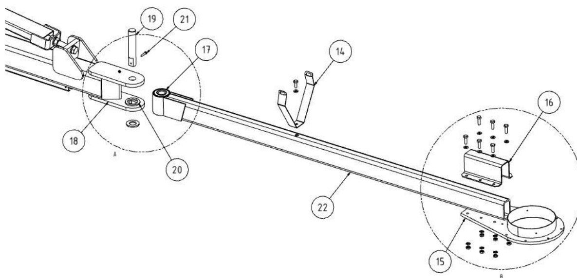
Obr. 163: Výkyvná konzola část 2
