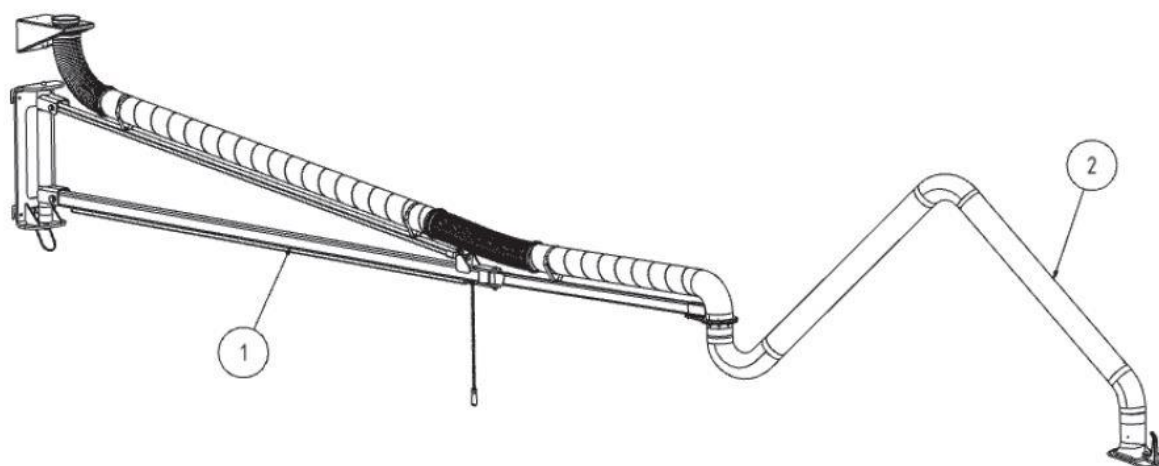
Рис. 199: Вытяжной рукав с поворотной консолью
