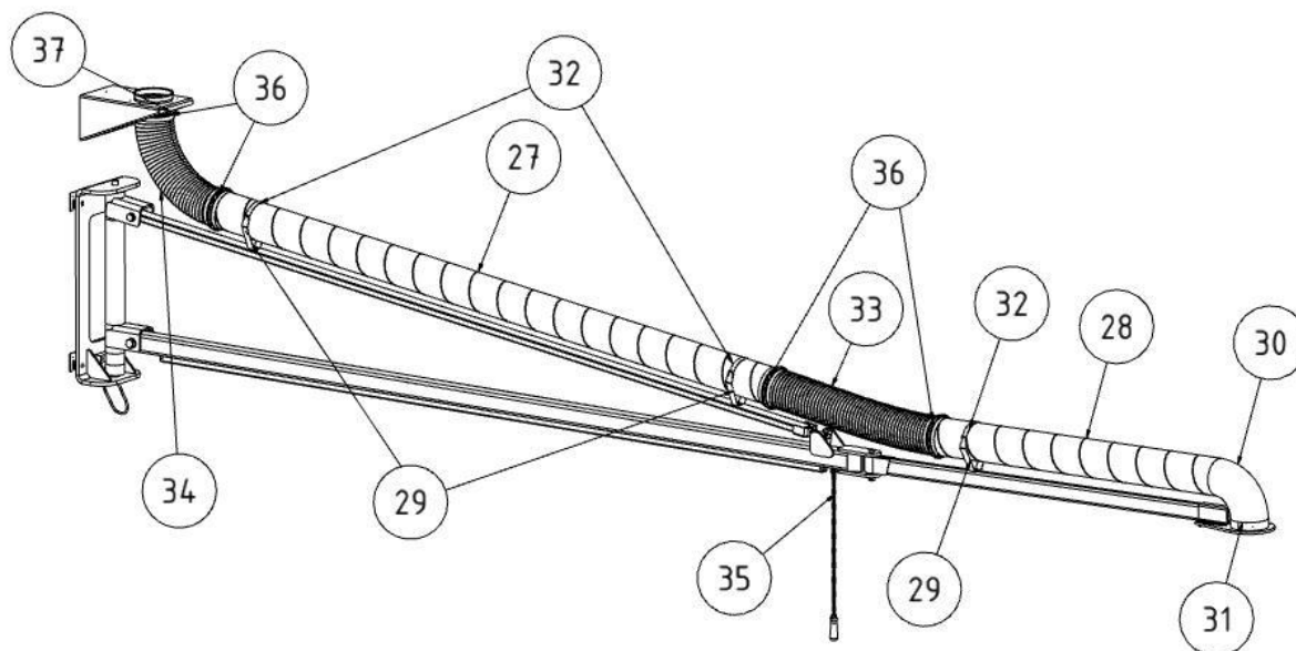
Fig. 146: Montaggio condotto a spirale
