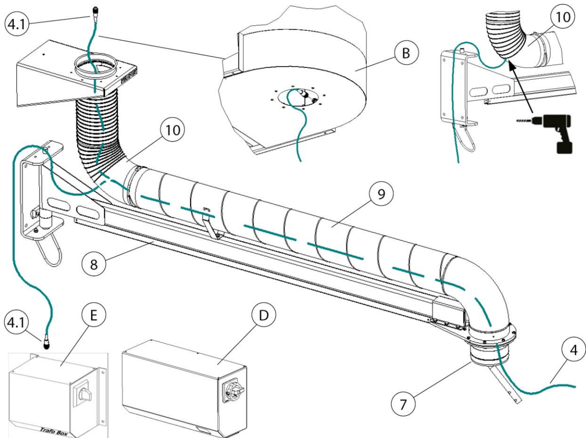
237. ábra: Kábelfektetés – Szívókarok darus hosszabbítóval
