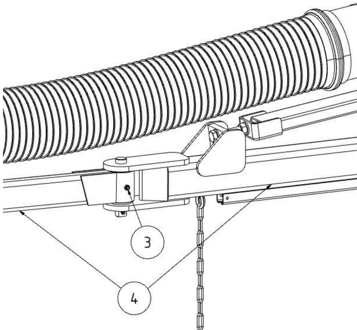
Fig. 38: Brake
