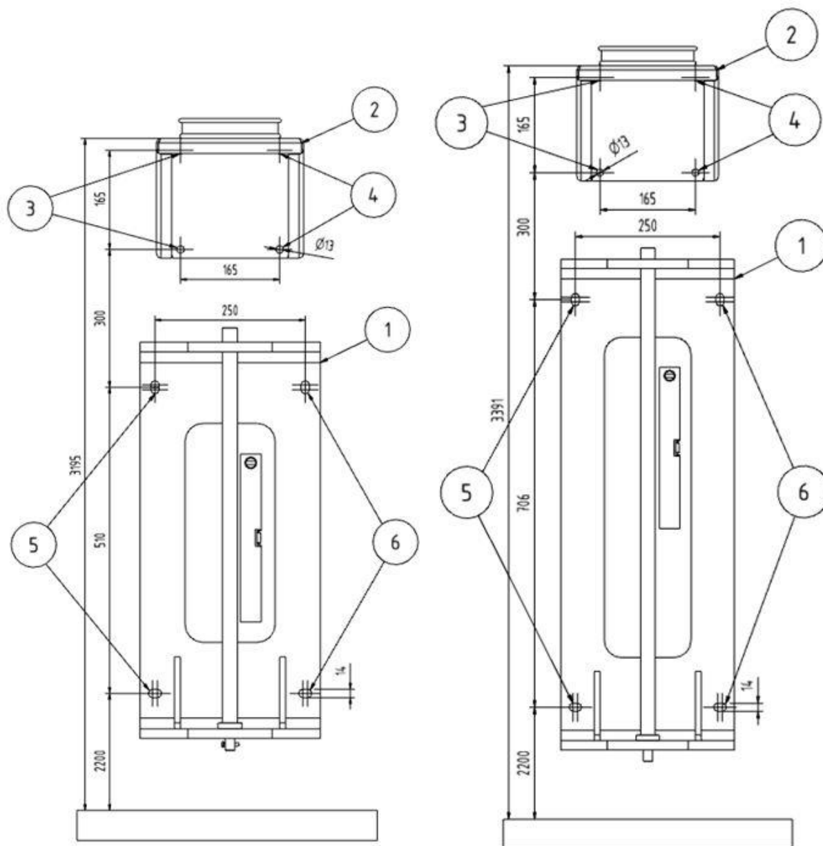
Rys. 181: uchwyt ścienny
