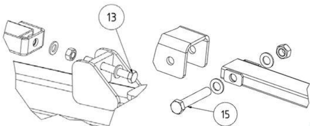
Sl. 250: Roka konzole
