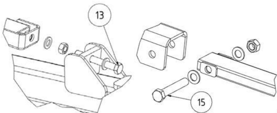
Fig. 118: Braço da lança
