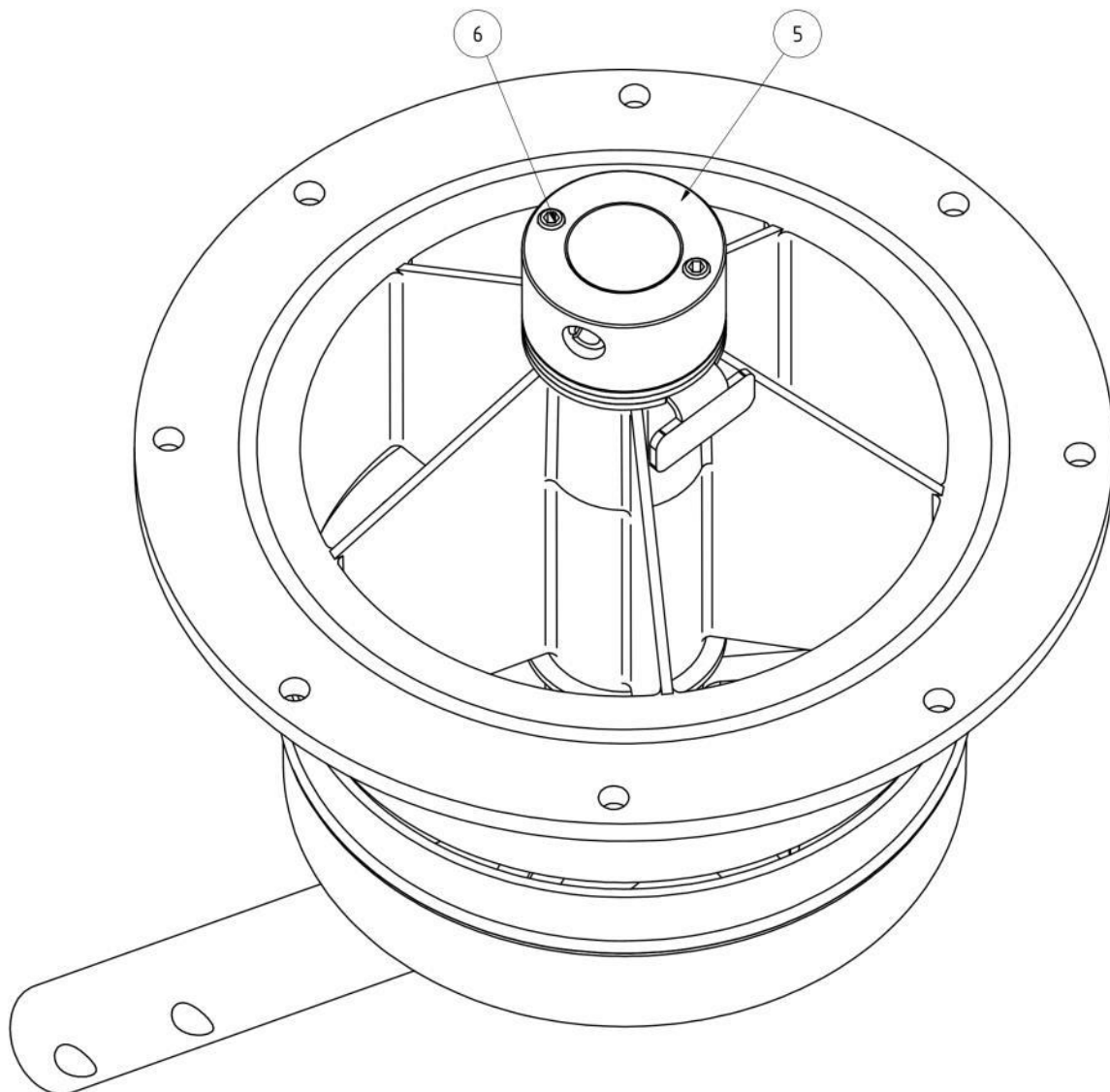
Afb. 79: Rem
