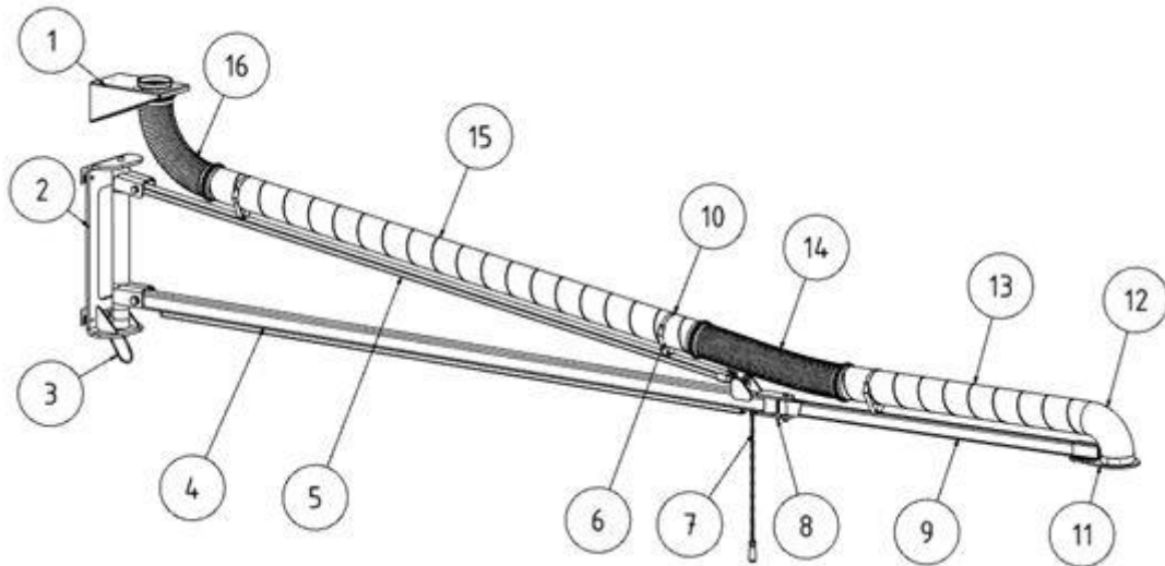
Fig. 48 : positions sur le produit
