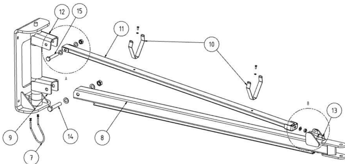
Рис. 205: Поворотная консоль, часть 1
