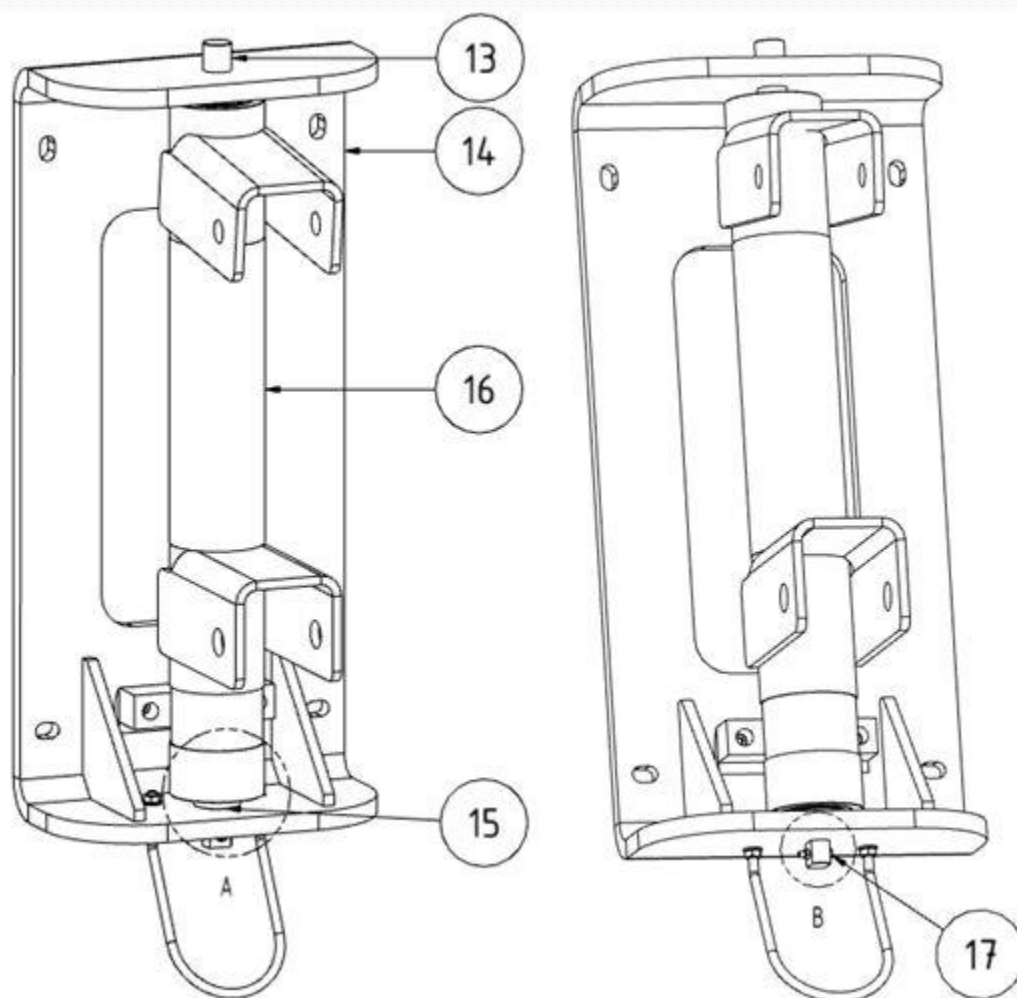
Fig. 138: Supporto braccio a sbalzo
