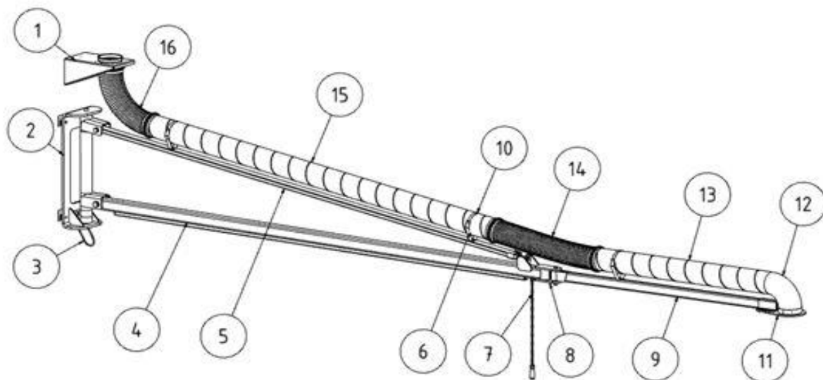
Fig. 134: Braccio a sbalzo
