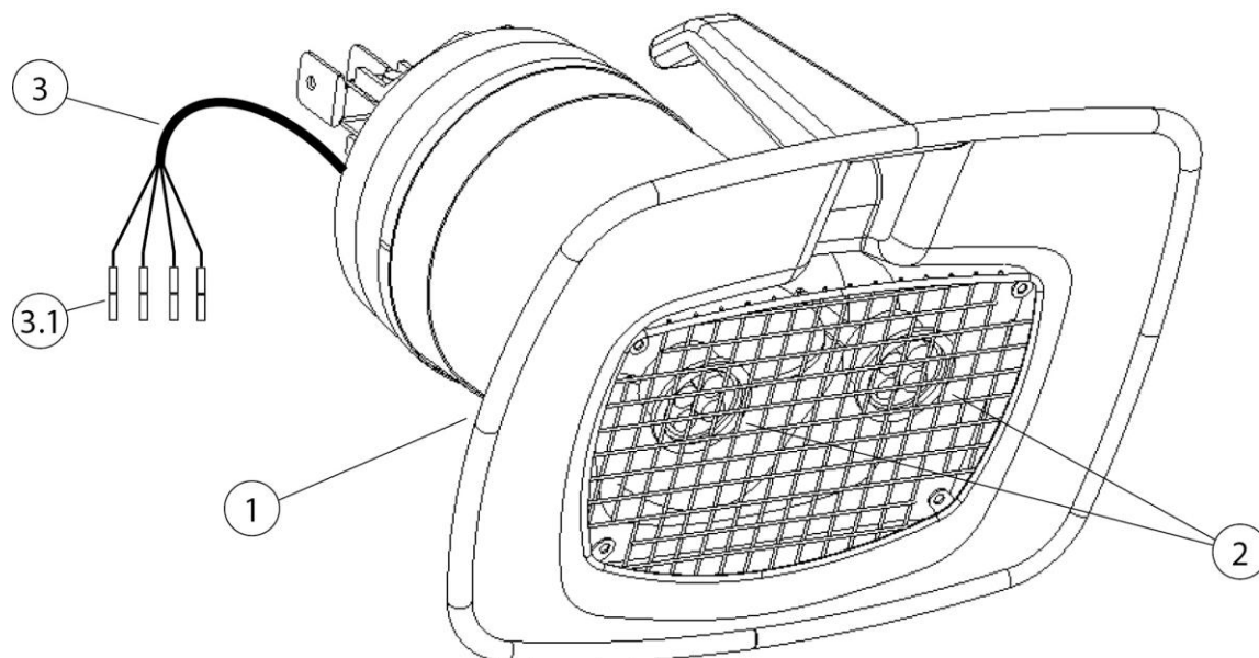
Sl. 261: Odsesovalni pokrov z osvetlitvijo
