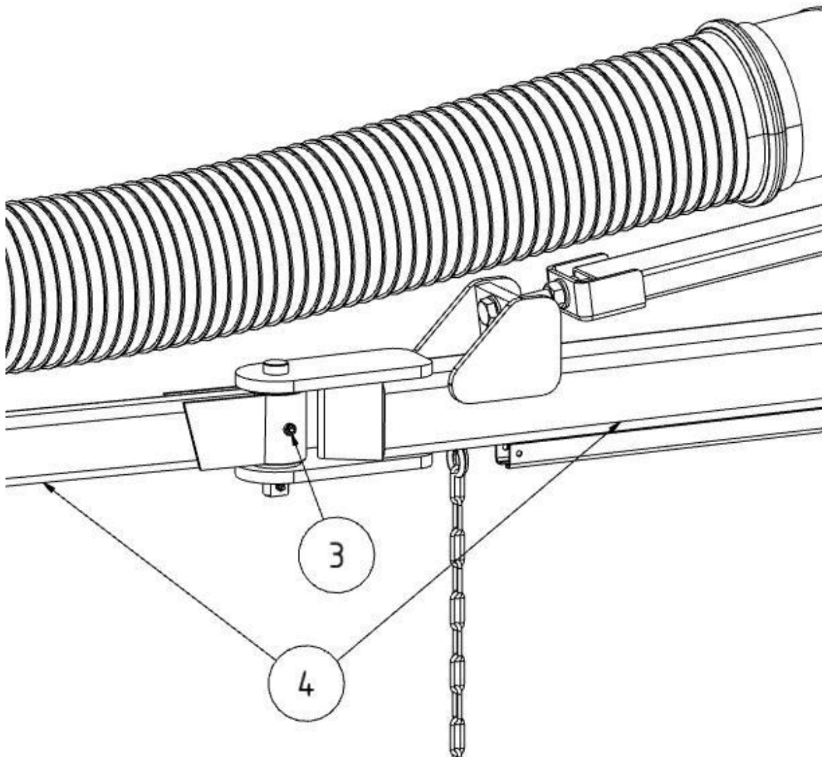
Afb. 82: Rem
