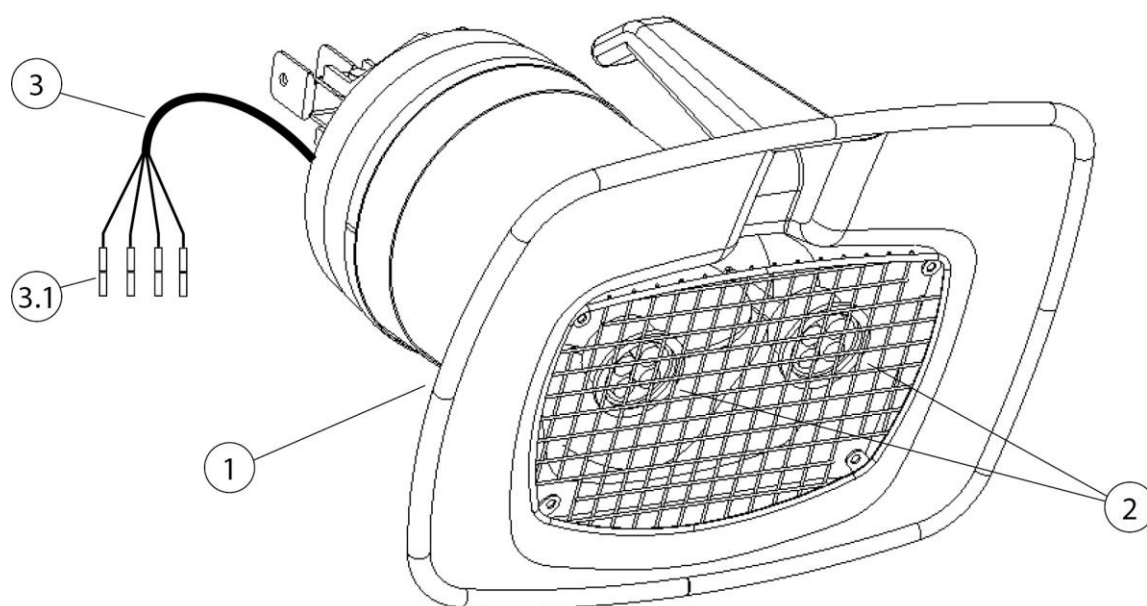
Fig. 151: cappa di aspirazione illuminata
