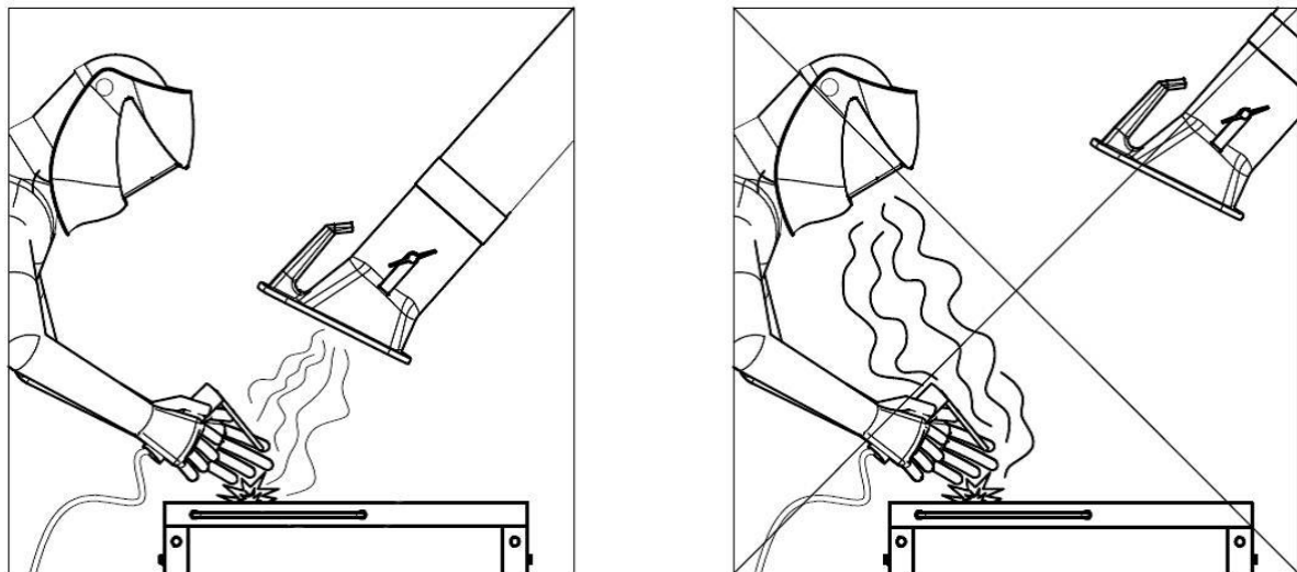
Fig. 153: Posizionamento della cappa di aspirazione
