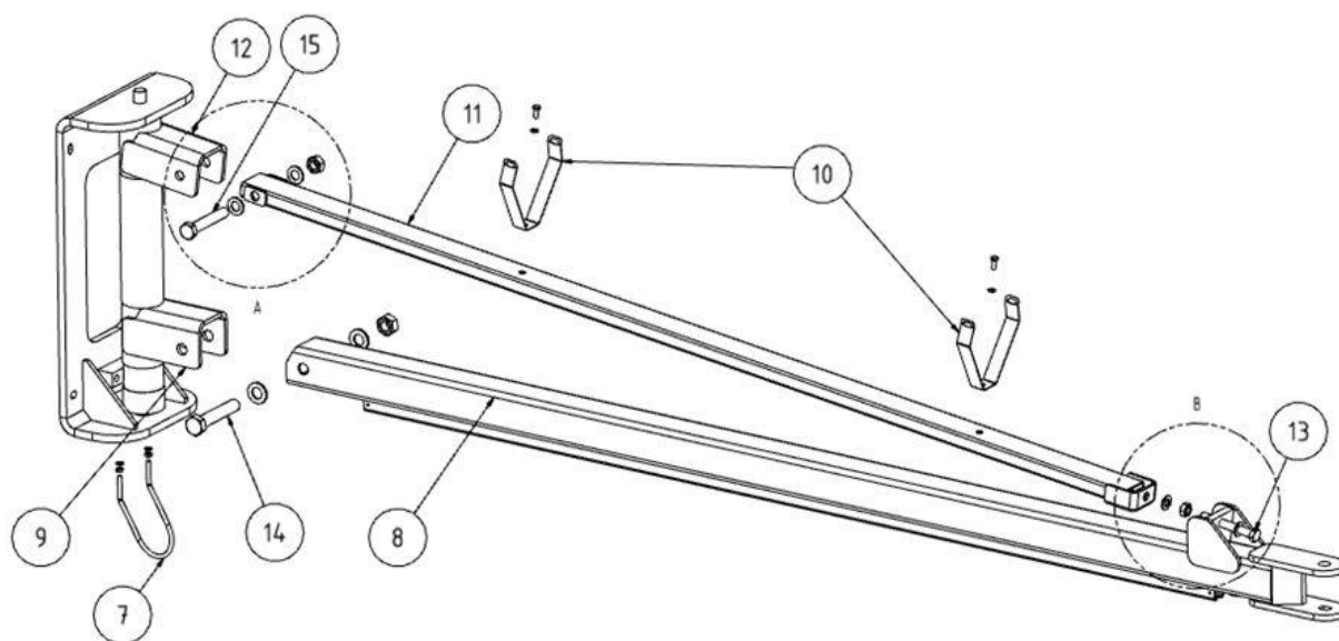
227. ábra: Hosszabbítókar 1. része
