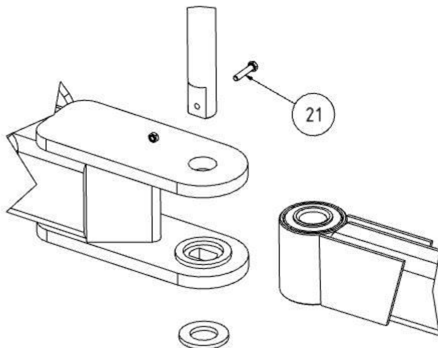
Rys. 187: Łączenie ramion wyciągnika
