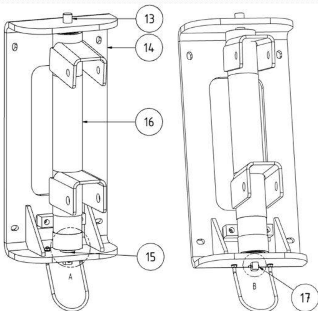
Sl. 248: Držalo roke konzole
