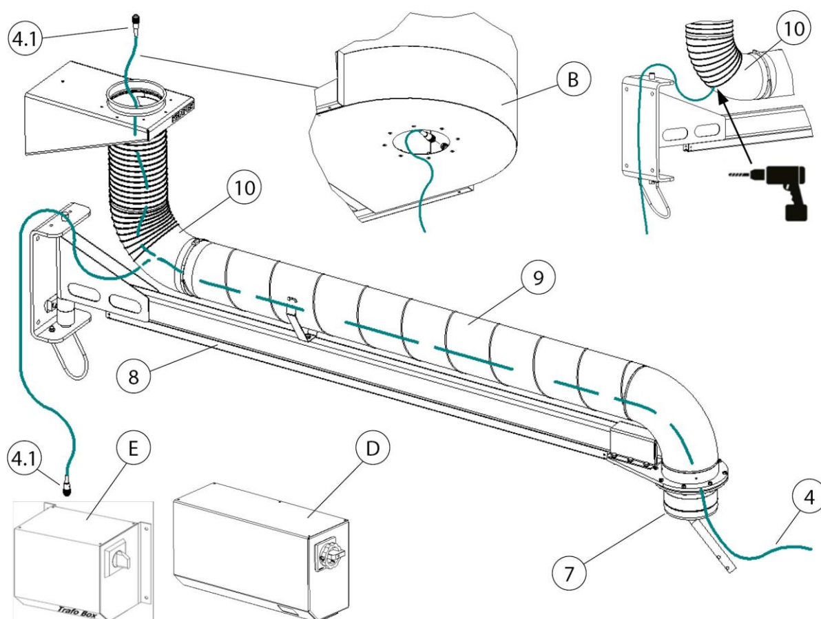
Obr. 171: Pokládka kabelů – odsávací ramena s jeřábovou konzolou
