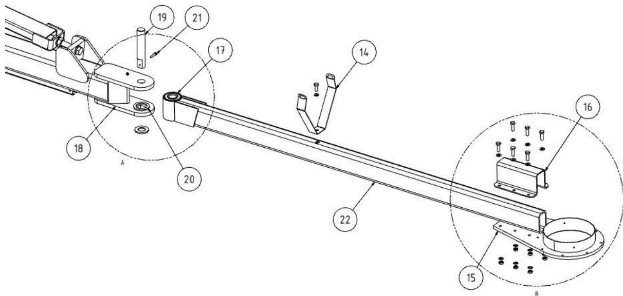
229. ábra: Hosszabbítókar 2. része
