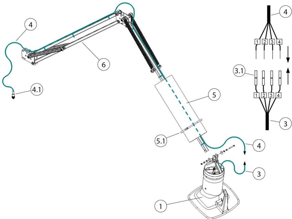
Afb. 86: Kabel leggen – afzuigarm 2-4 meter
