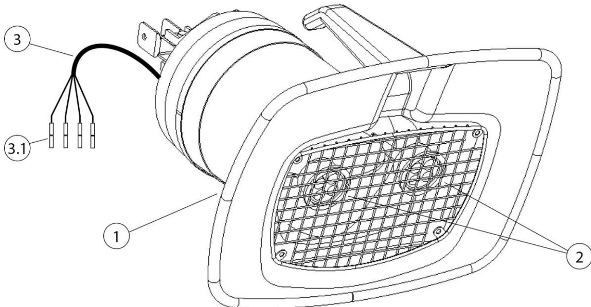
Fig. 63 : Hotte d'aspiration avec éclairage
