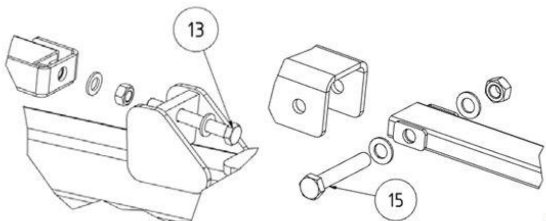
Obr. 162: Výkyvná konzola
