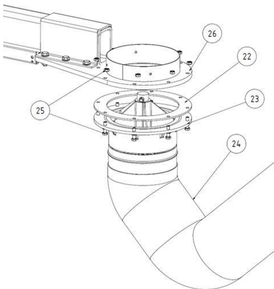
Fig. 56 : bras d'aspiration sur potence
