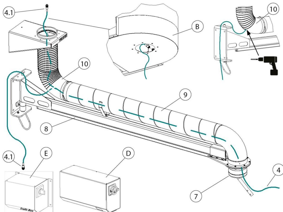
Fig. 149: Posa cavi - Bracci di aspirazione con braccio di gru
