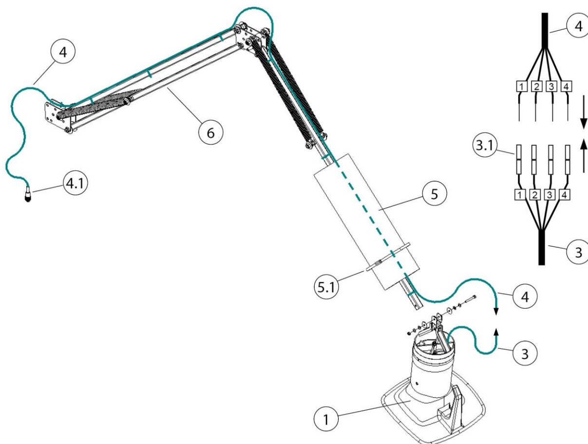
Fig. 64 : Pose des câbles - bras d'aspiration 2-4 mètres
