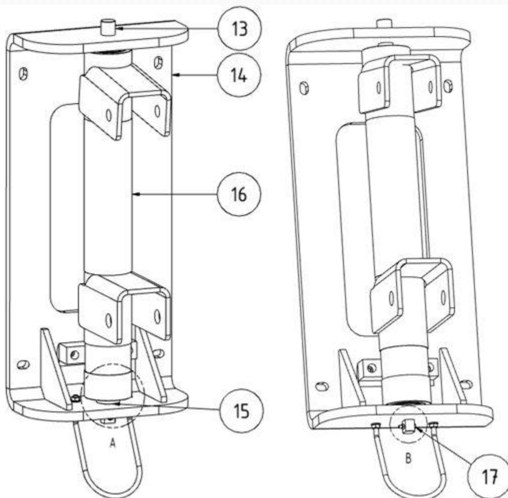
Abb. 6: Halterung Auslegerarm
