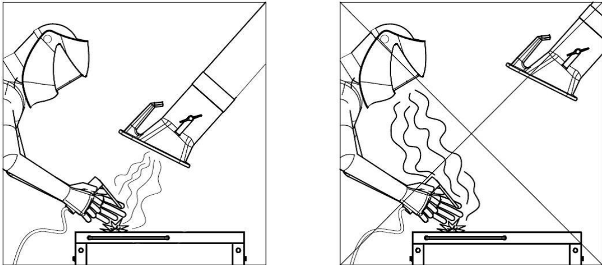
Abb. 21: Positionierung der Absaughaube
