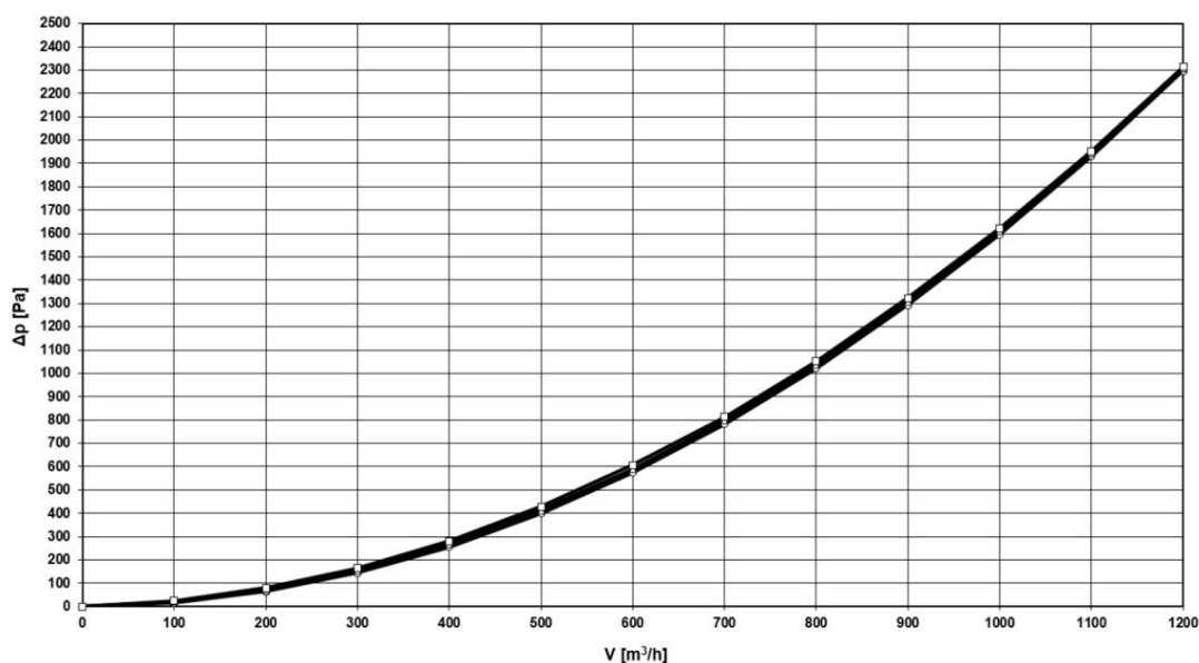
Рис. 220: Диаграмма падения давления
