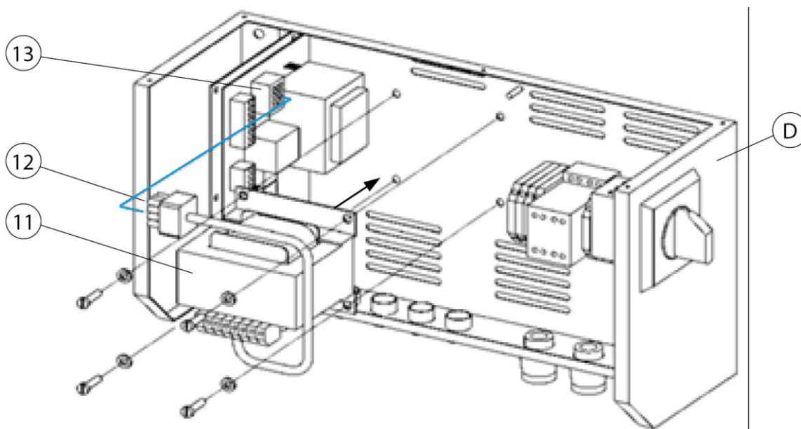
Fig. 150: installazione a posteriori scatola di controllo trasformatore
