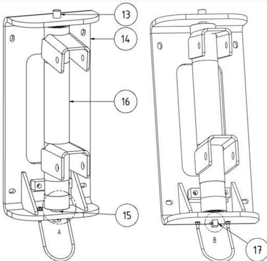
Afb. 72: Houder giekarm
