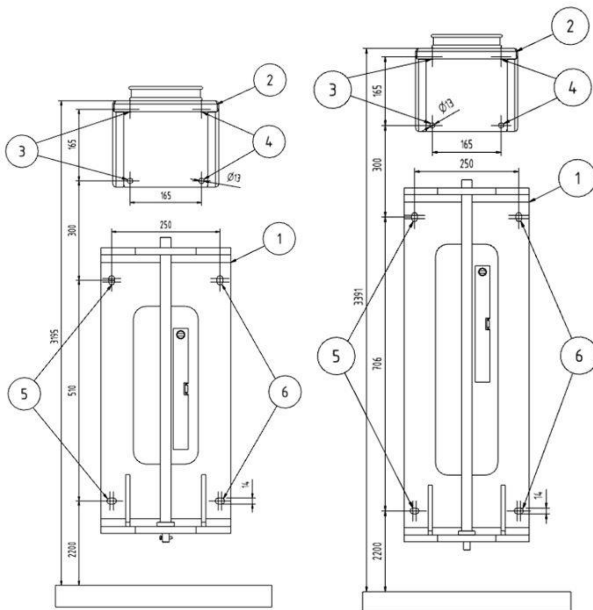
Sl. 247: Stensko držalo
