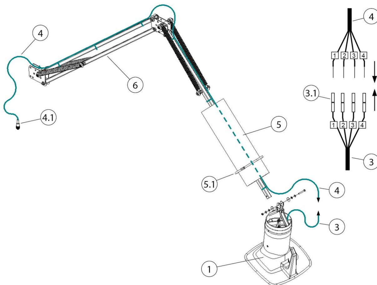
Рис. 218: Прокладка кабеля – вытяжной рукав 2 - 4 метра
