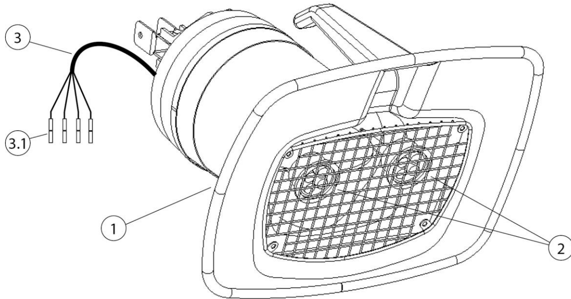
Abb. 19: Absaughaube mit Beleuchtung
