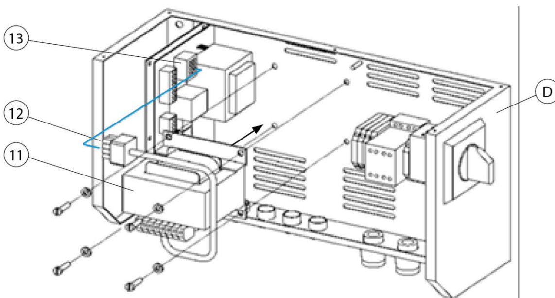
Rys. 194: Doposażenie panelu sterowniczego w transformator
