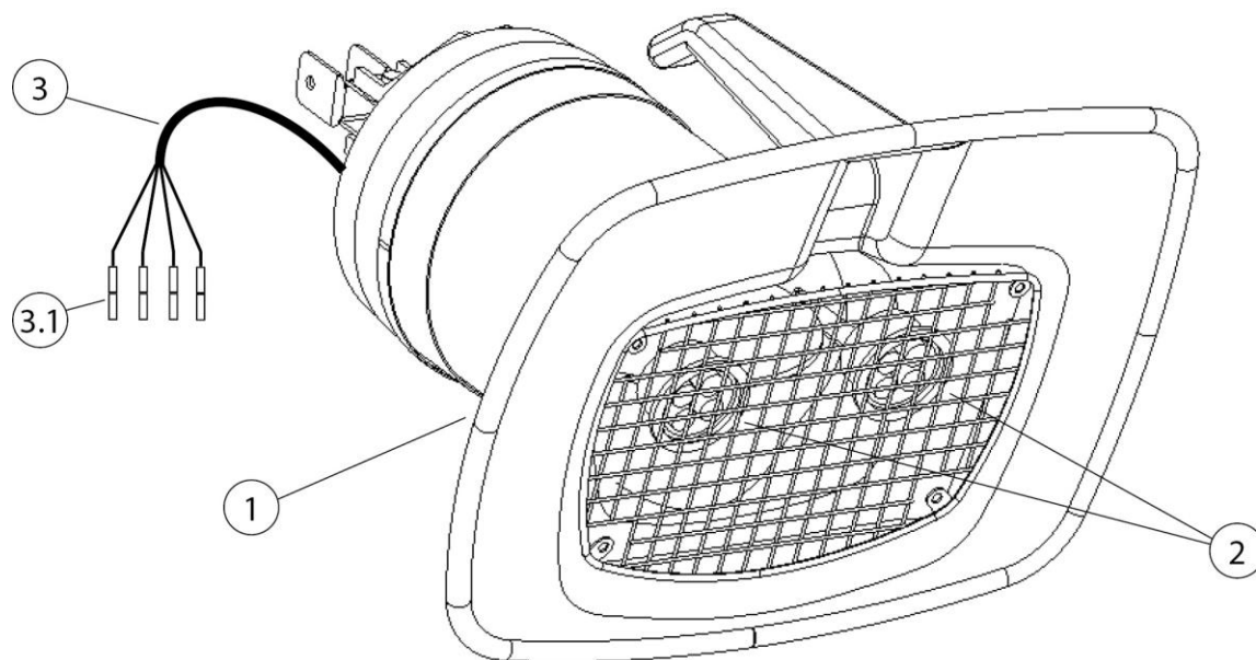
Fig 107: Campana de aspiración con iluminación
