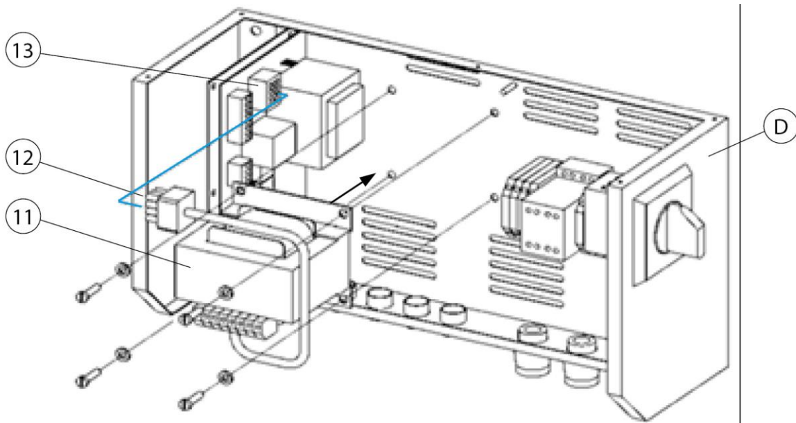
238. ábra: Vezérlődoboz - Transzformátor utólagos felszerelése
