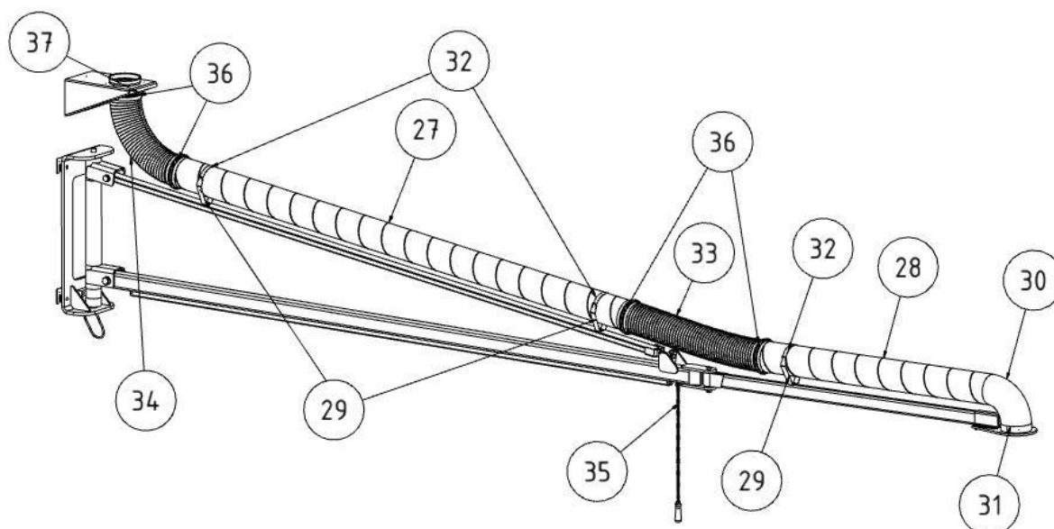
Fig. 102: Montar el tubo espiral
