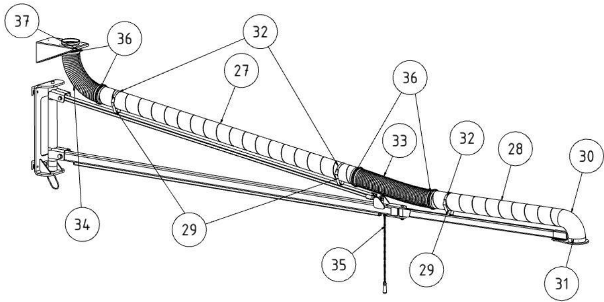
234. ábra: A spirálkorcolt cső felszerelése
