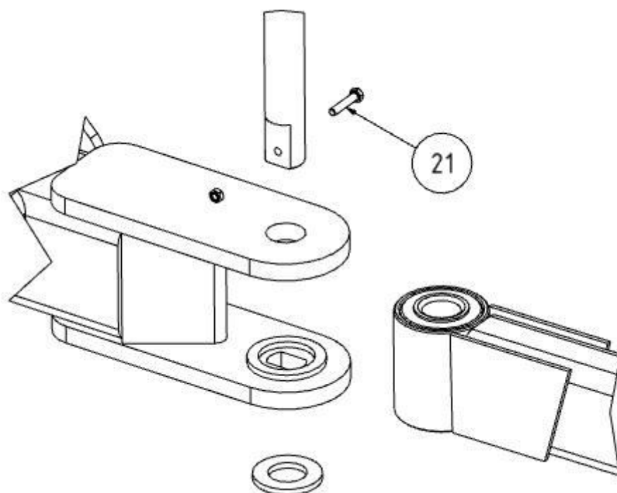
Obr. 165: Spojení výkyvné konzoly a prodlužovacího ramene
