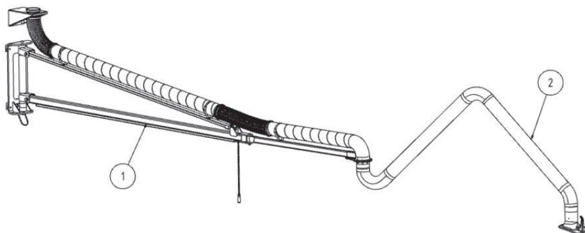
Fig. 45 : bras d'aspiration avec potence pivotante
