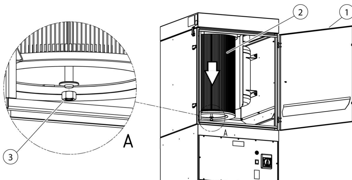
Afb. 8: Filter vervangen
