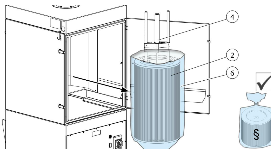
Afb. 10: Filterpatroon verwijderen
