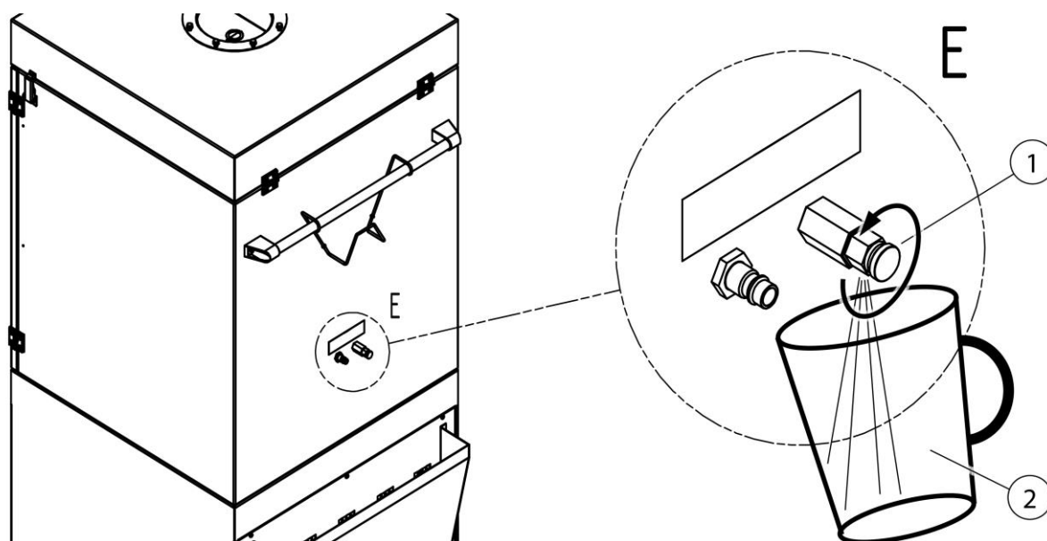
Afb. 7: Condensaat aftappen
