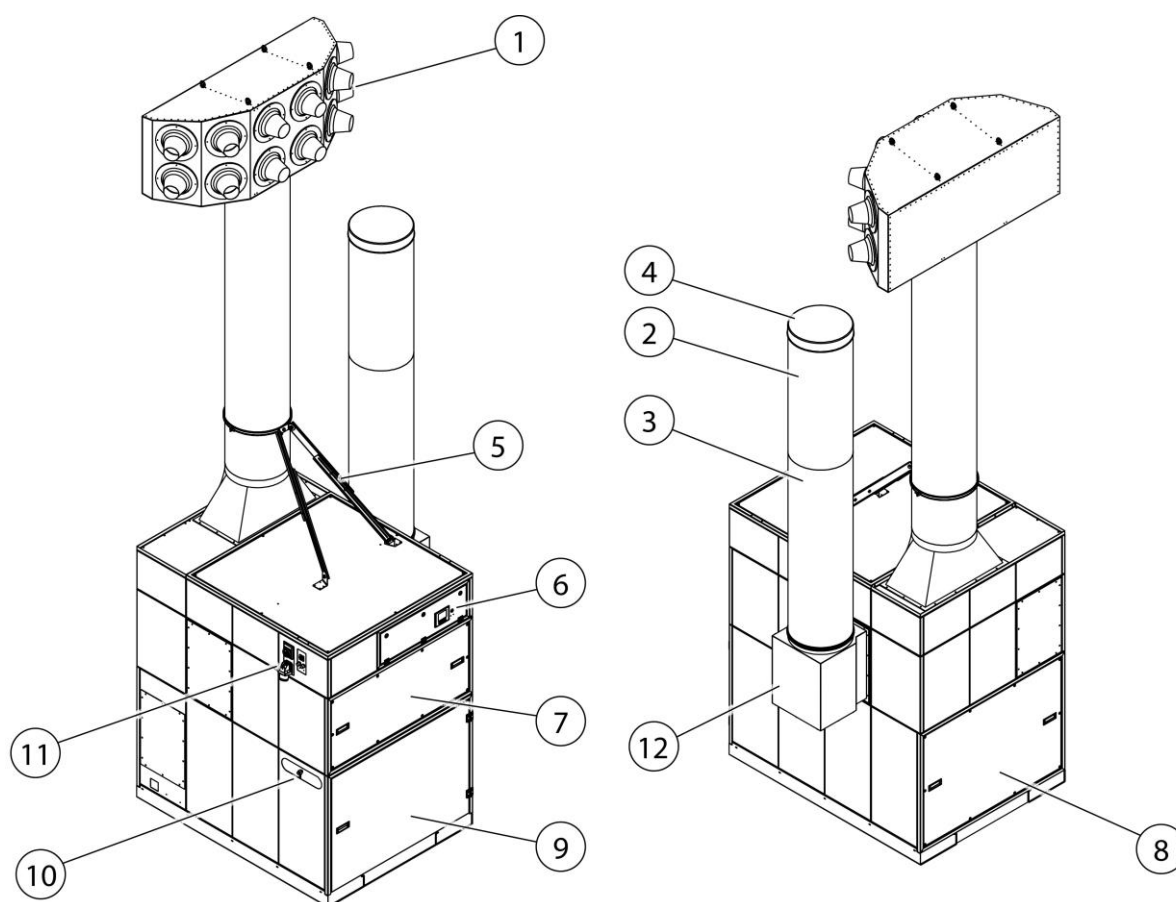
Obr. 5: Popis funkce – 998800462
