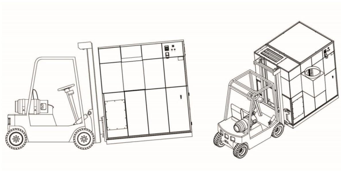
Obr. 8: Přeprava výrobku
