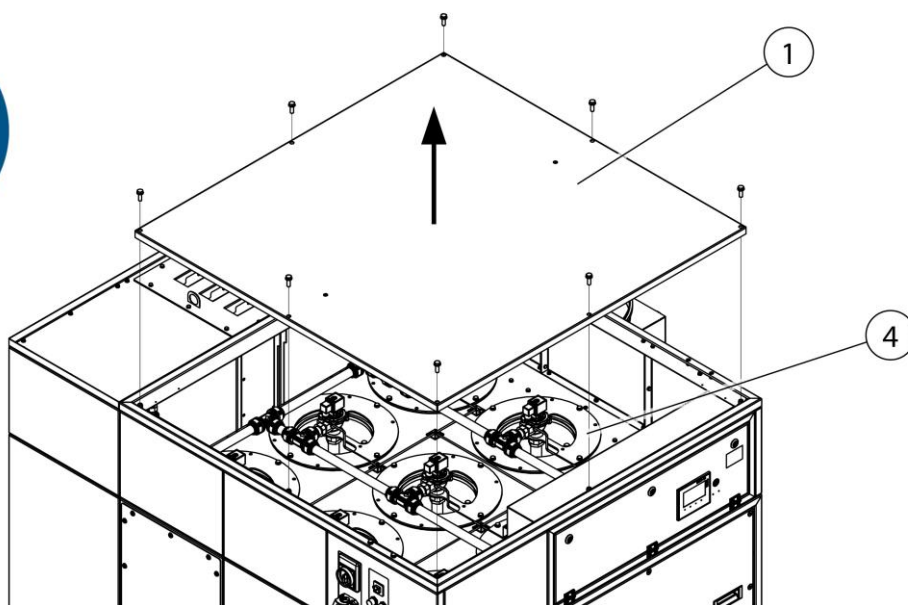
Obr. 42: Výměna filtru – demontáž filtračního plechu
