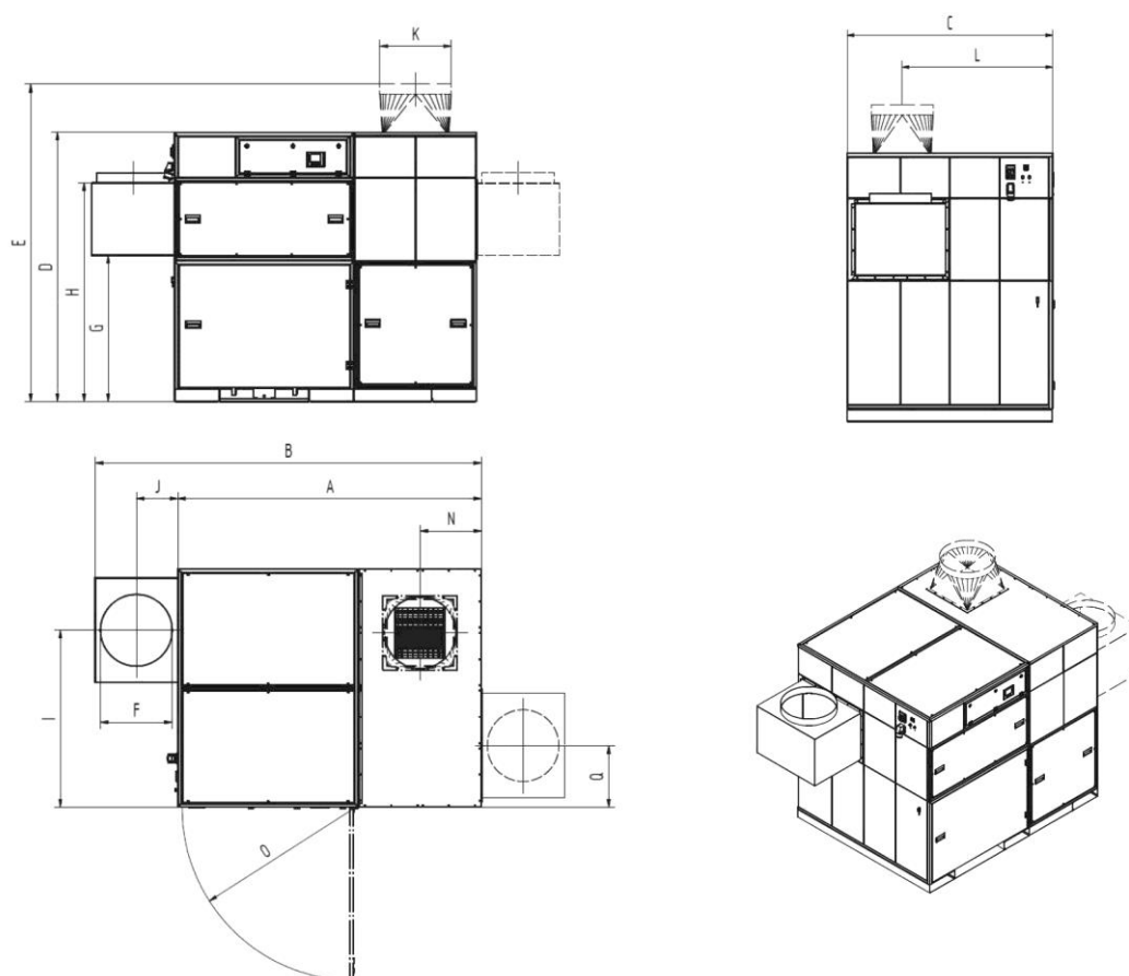
Obr. 56: Rozměrový výkres 998701370 (998800414, 998800463)
