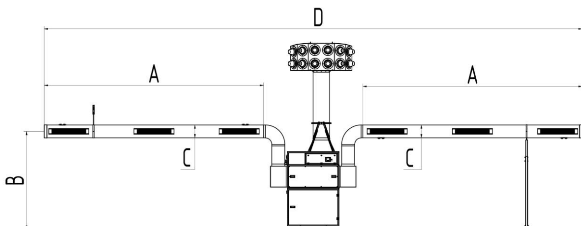
Obr. 58: Rozměrový výkres – 998800401
