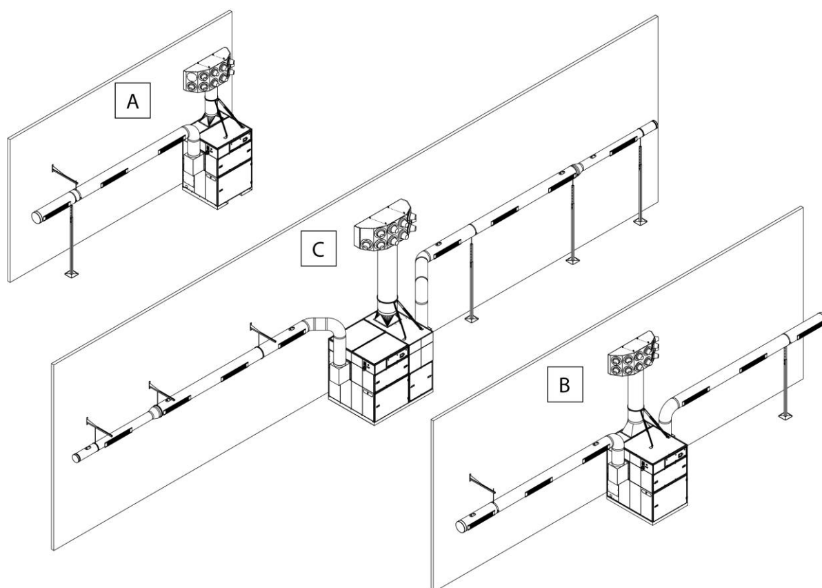
Obr. 11: Montáž – přehled variant produktů
