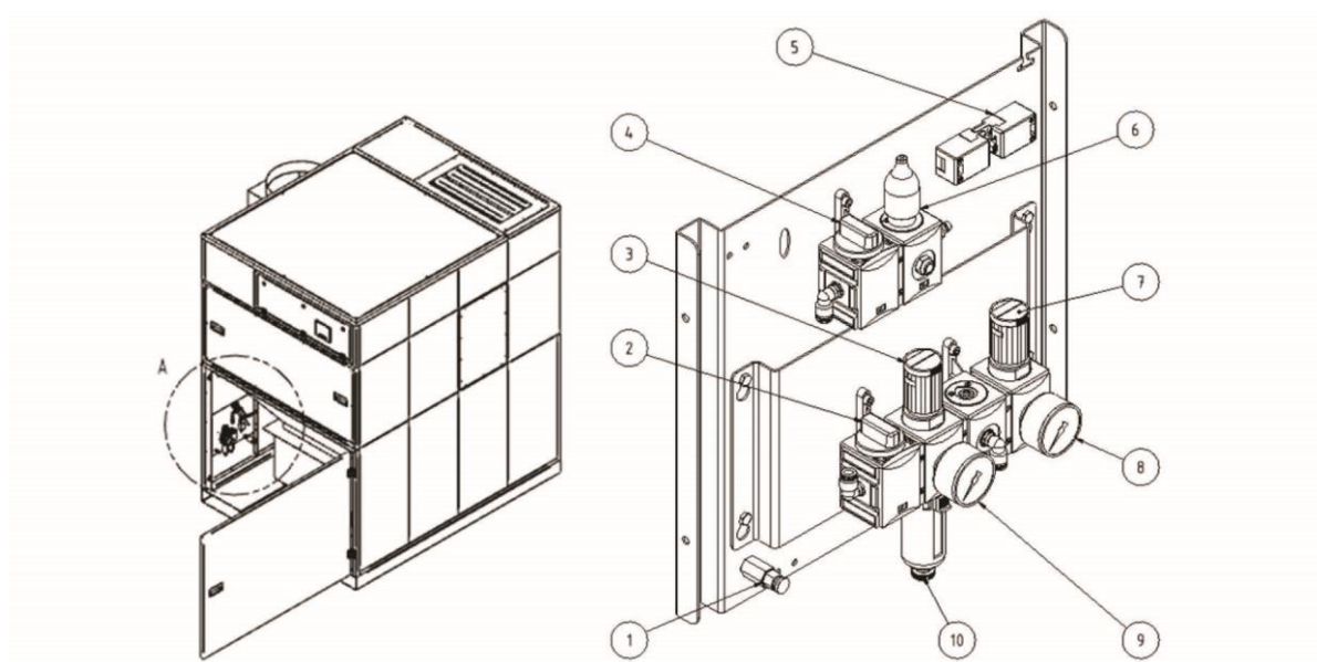
Obr. 10: Pneumatická jednotka
