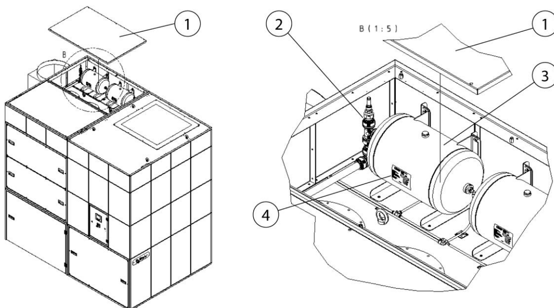
Obr. 74: Přístup k zásobníku stlačeného vzduchu a pojistnému ventilu
