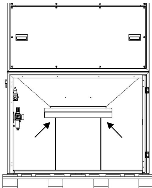
Obr. 19: Nadzvednutí filtrační jednotky vysoko zdvižným vozíkem
