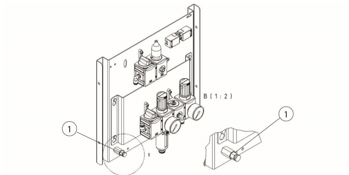
Obr. 70: Vypouštěcí ventil kondenzátu zásobníku stlačeného vzduchu
