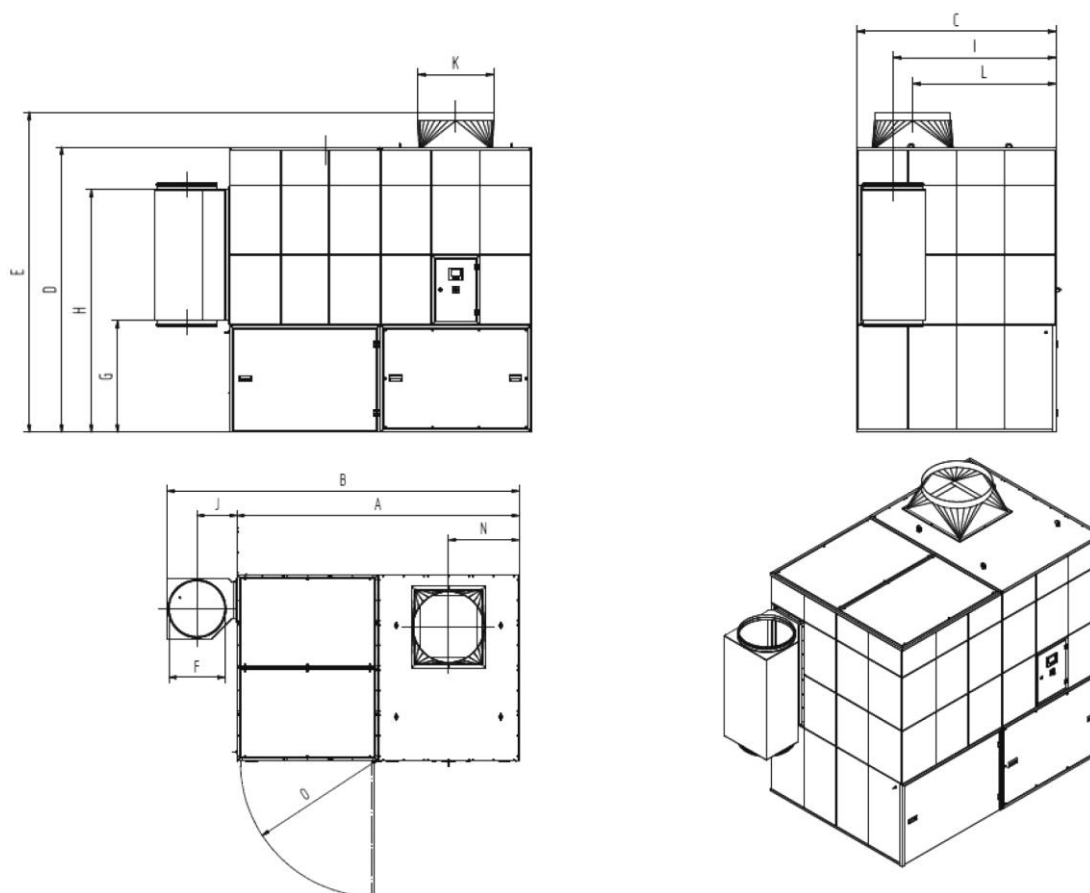
Obr. 75: Rozměrový výkres 34110
