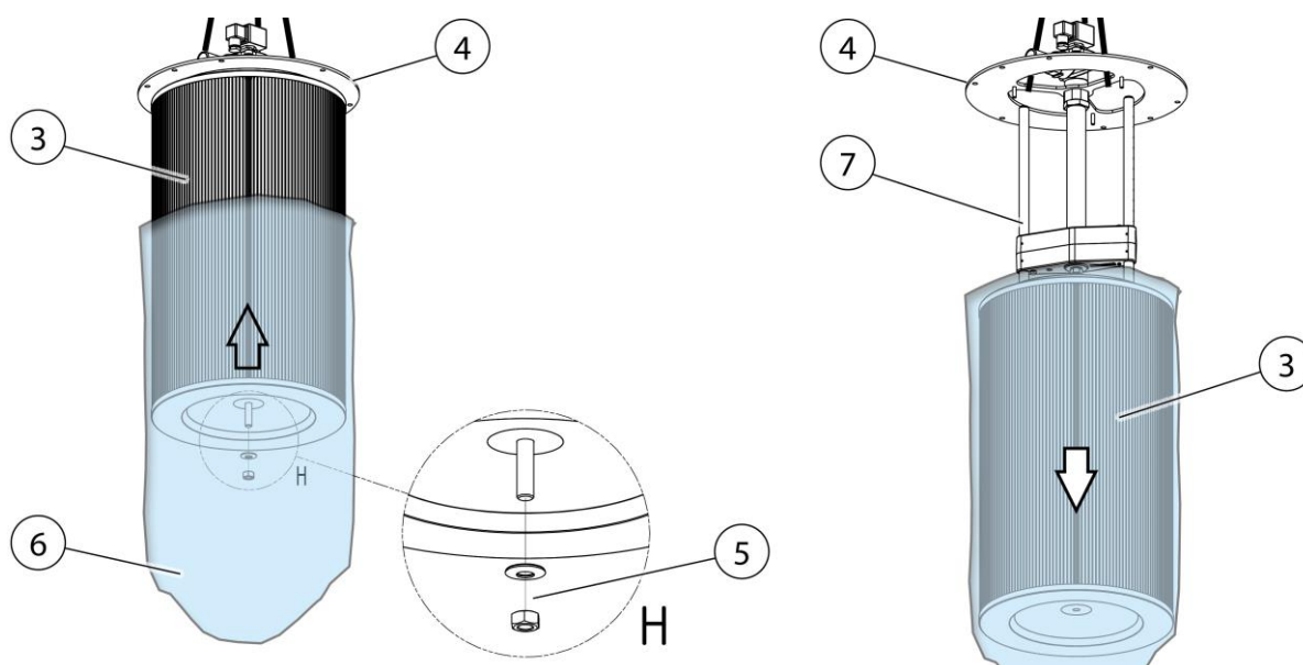
Obr. 68: Výměna filtru – demontáž filtrační patrony
