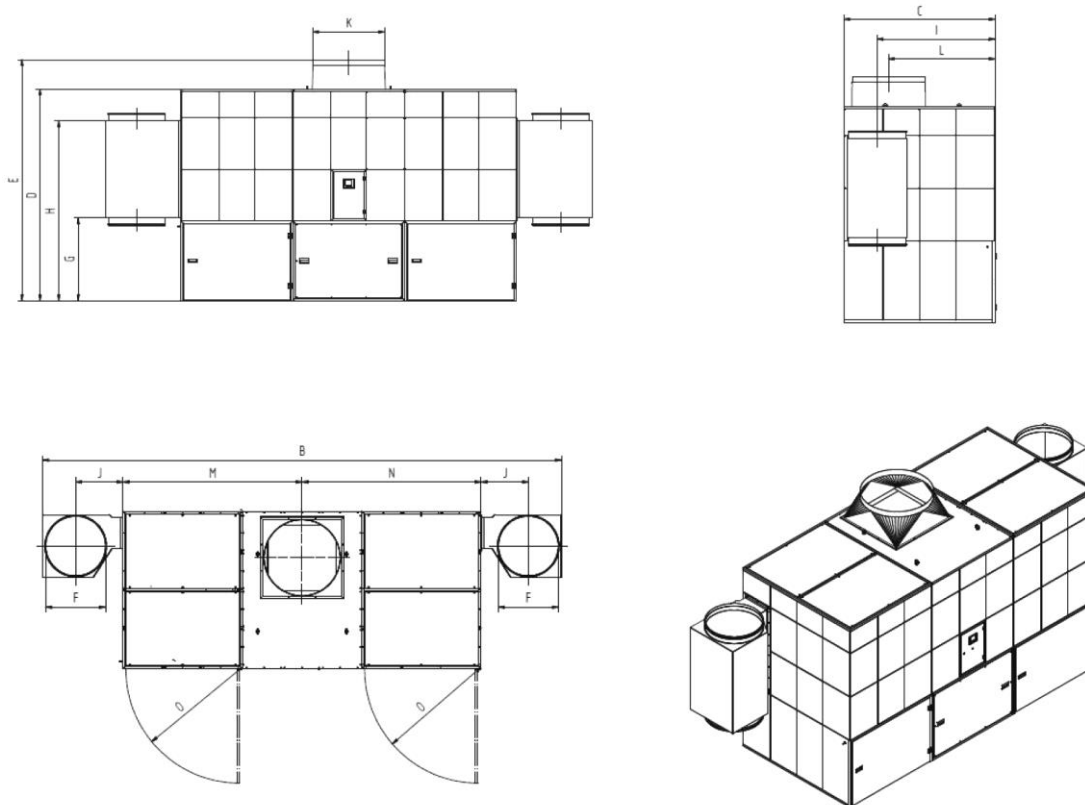
Obr. 78: Rozměrový výkres 34180
