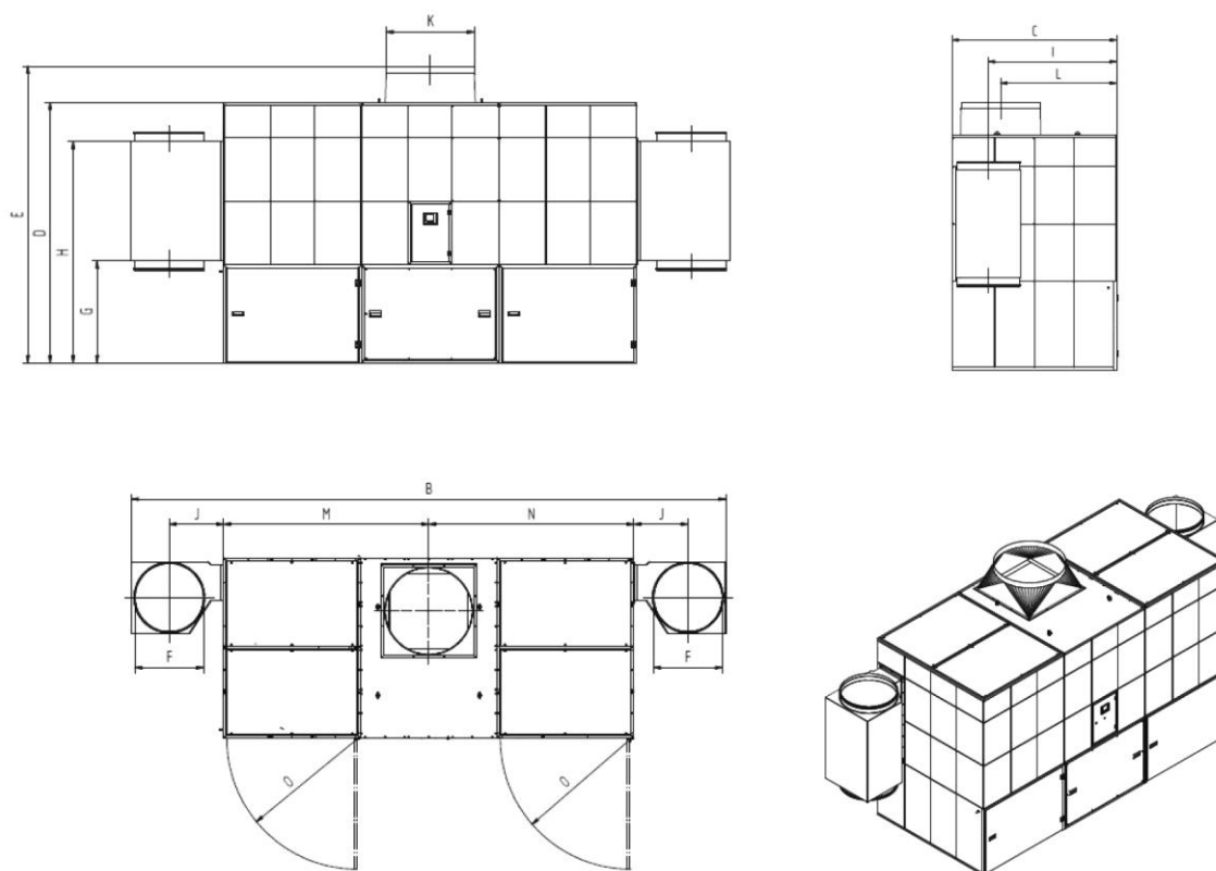
Obr. 79: Rozměrový výkres 34200 + 34220
