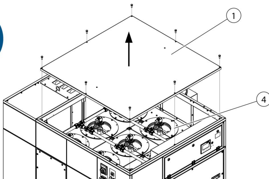
Obr. 64: Výměna filtru – demontáž filtračního plechu
