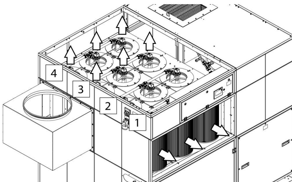
Obr. 61: Výměna filtru
