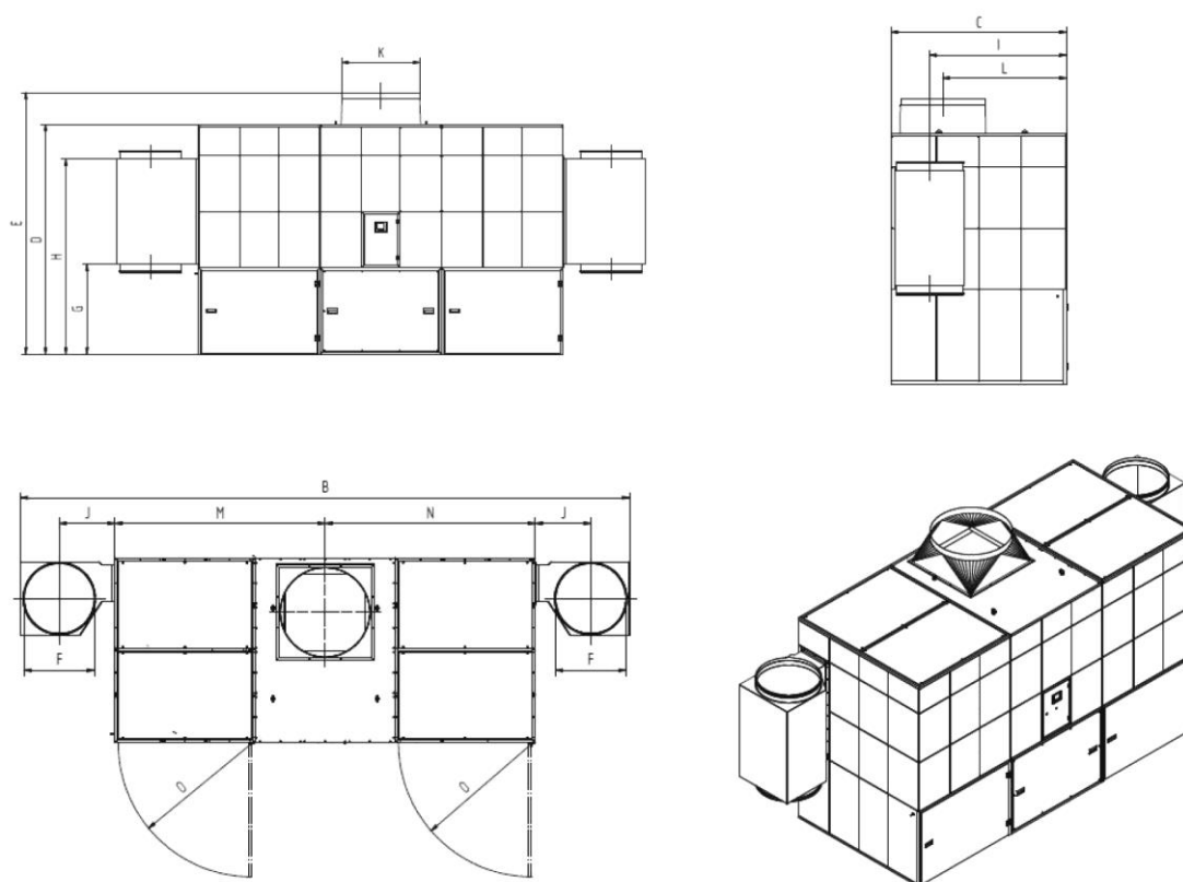
Obr. 77: Rozměrový výkres 34160
