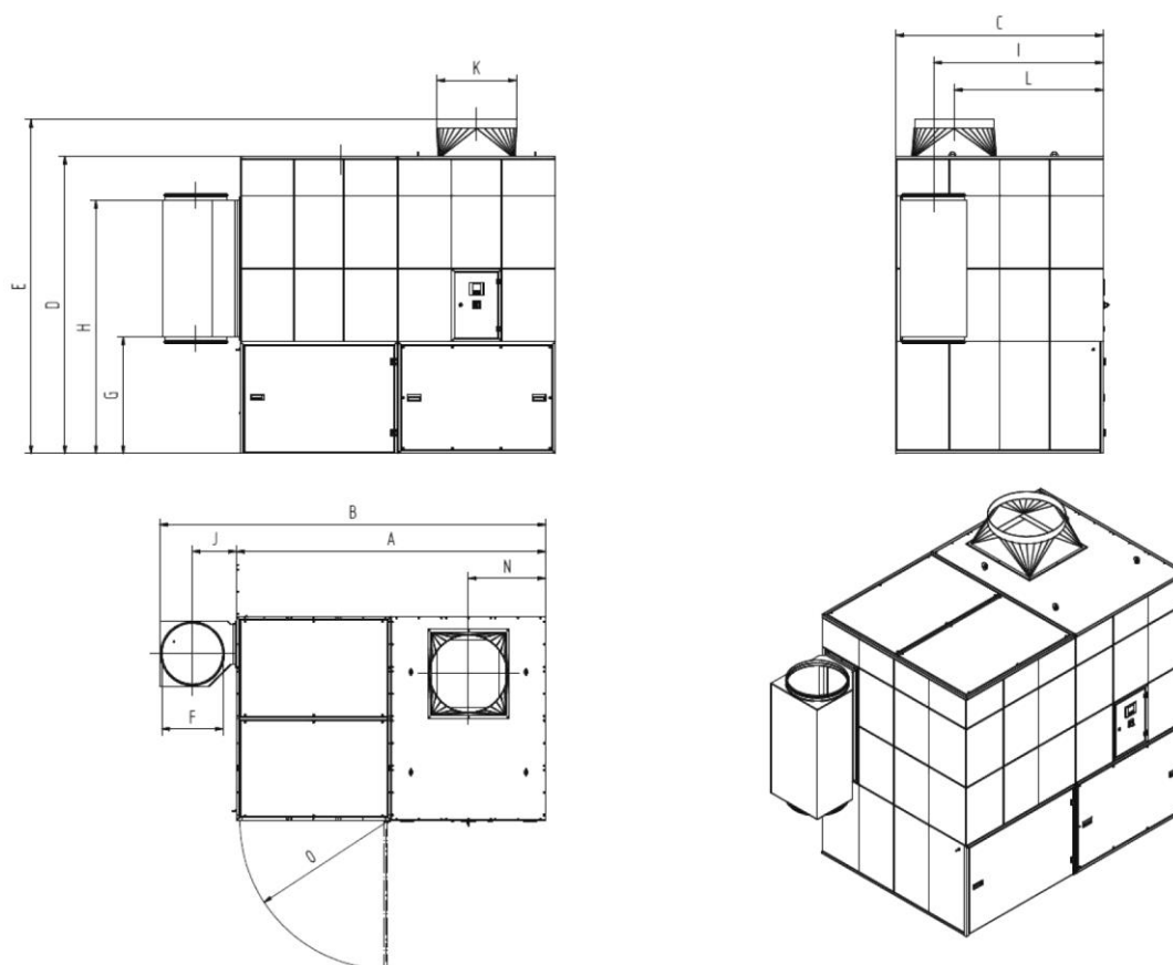
Obr. 76: Rozměrový výkres 34130
