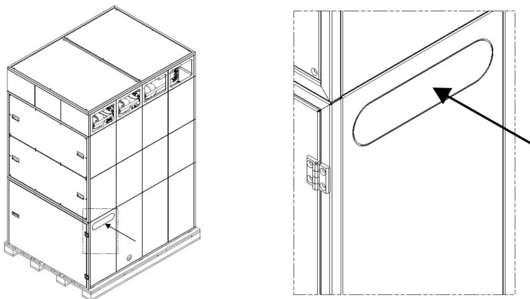
Obr. 13: Děrovaný plech
