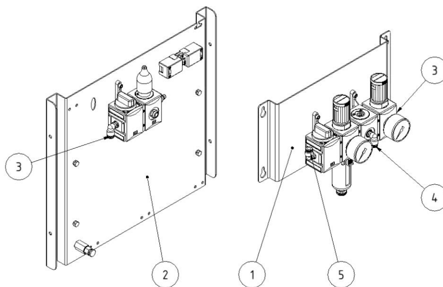
Obr. 31: Pneumatická jednotka
