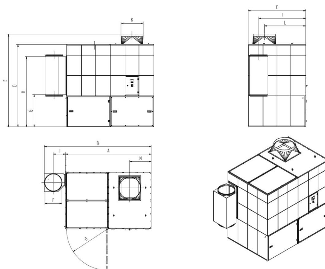
Rys. 76: Karta wymiarowa 34130
