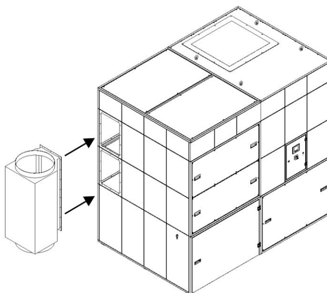
Rys. 26: Montaż skrzynki przyłączeniowej od strony odciagu
