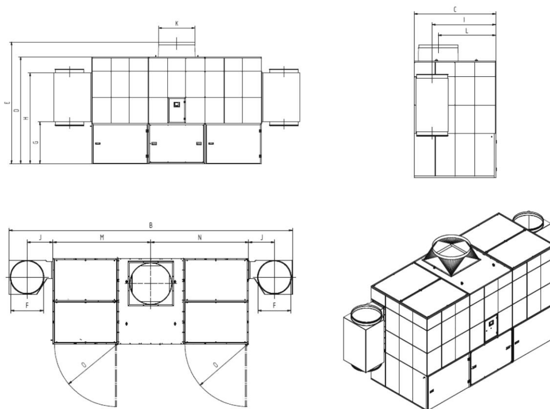
Rys. 77: Karta wymiarowa 34160
