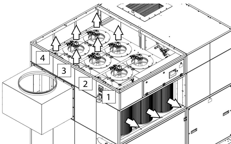
Rys. 61: Wymiana filtra
