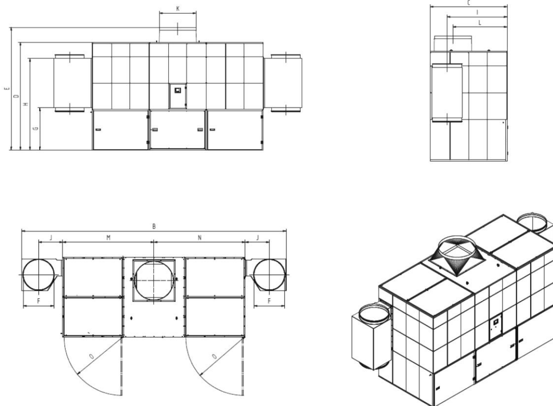
Rys. 78: Karta wymiarowa 34180
