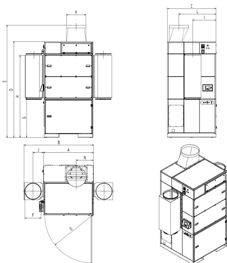
Obr. 62: Rozměrový výkres 3475
