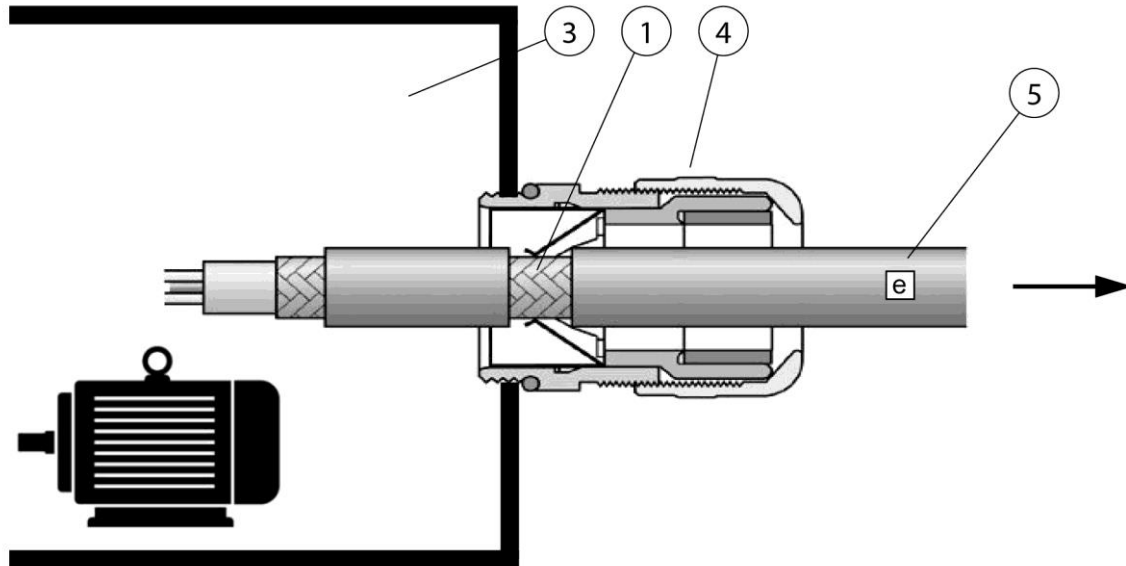
Abb. 19: Motorkabel-Abschirmung anschließen
