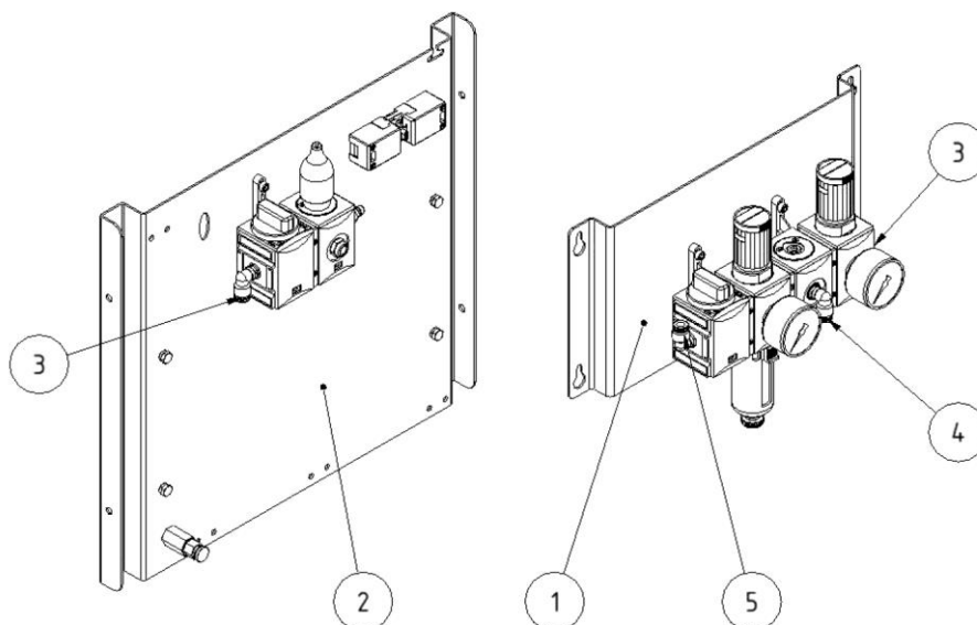
Abb. 13: Drucklufteinheit (Outdoor-Version)
