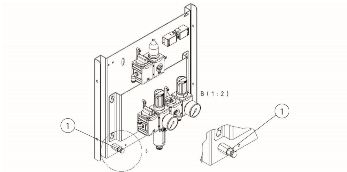
Abb. 52: Kondensatablassventil Druckluftbehälter
