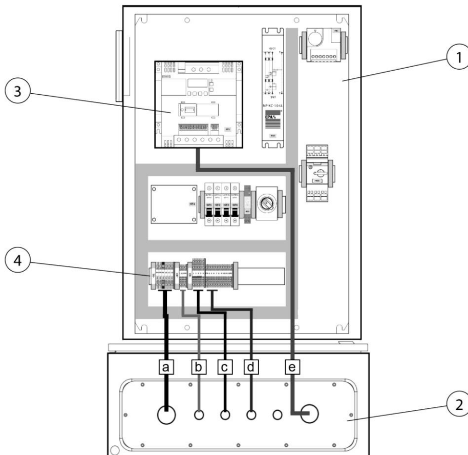
Abb. 16: Schalterschrank Absaugleistungsregelung
