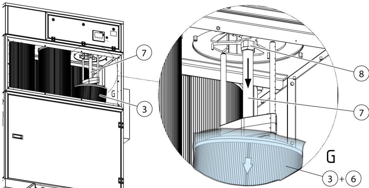
Abb. 45: Rotationsdüse demontieren
