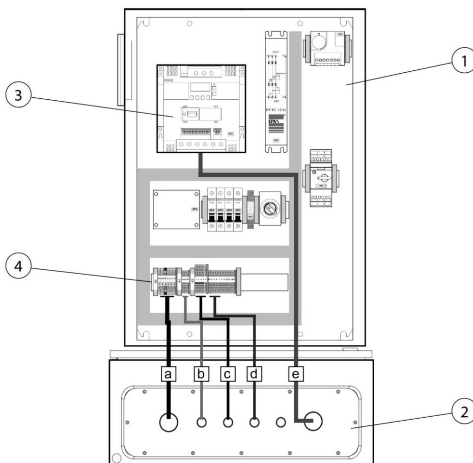
Fig. 16 : armoire de commande régulation de la puissance d'aspiration
