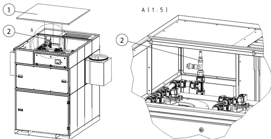
Fig. 57 : accès à la vanne de sécurité d'air comprimé
