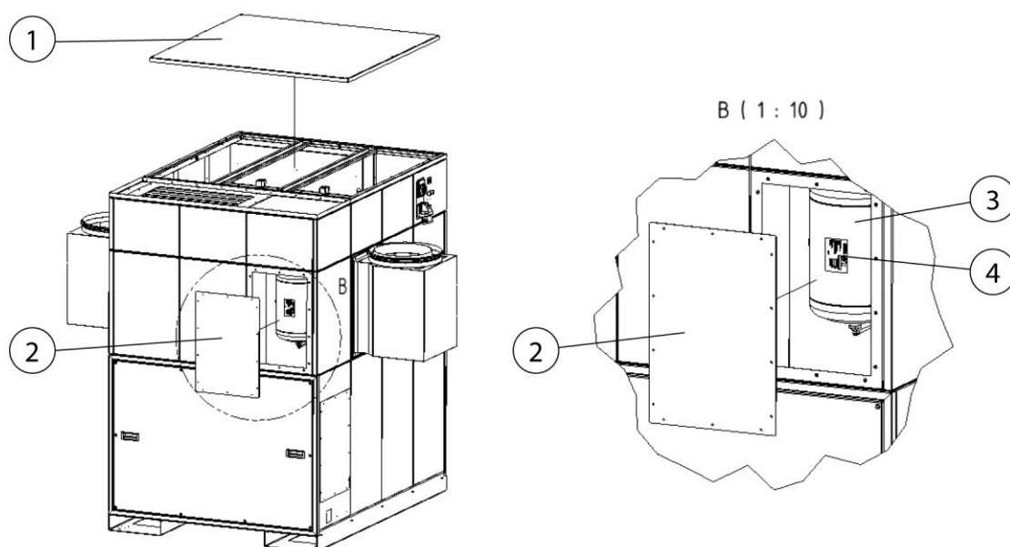
Fig. 56 : accès au réservoir d'air comprimé
