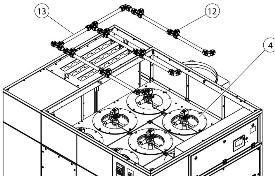
Fig. 48 : Remplacement du filtre – Démontage de la tuyauterie d'air comprimé
