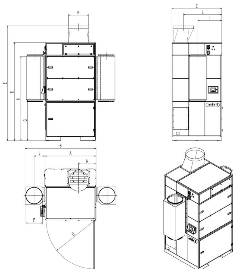
Fig. 62 : Fiche dimensionnelle 3475
