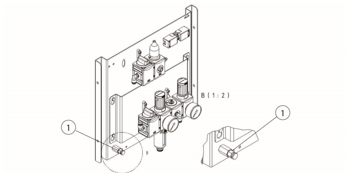
Fig. 52 : soupape de vidange des condensats réservoir d'air comprimé
