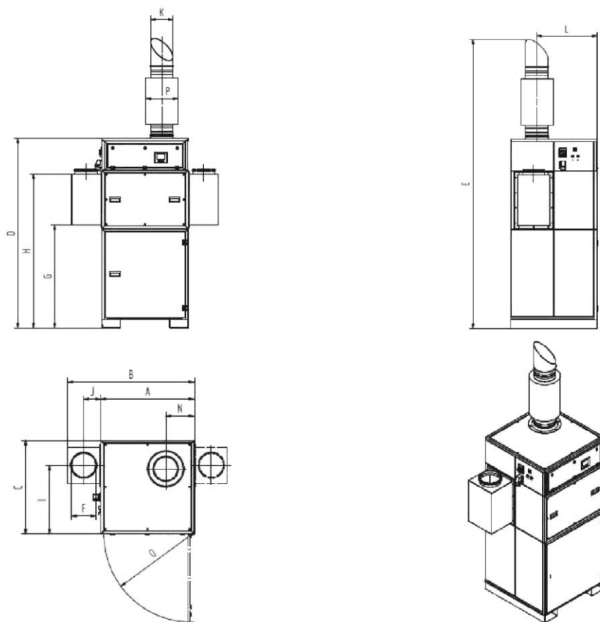
Fig. 58 : Fiche dimensionnelle 3420
