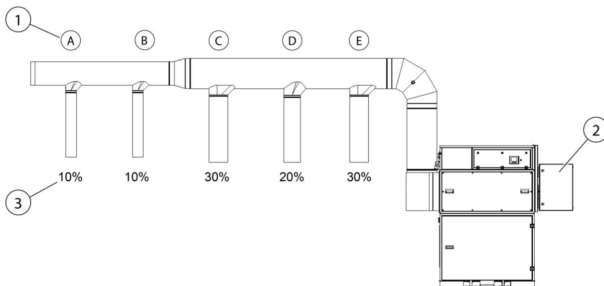
Fig. 36 : réglage de la régulation de la puissance d'aspiration
