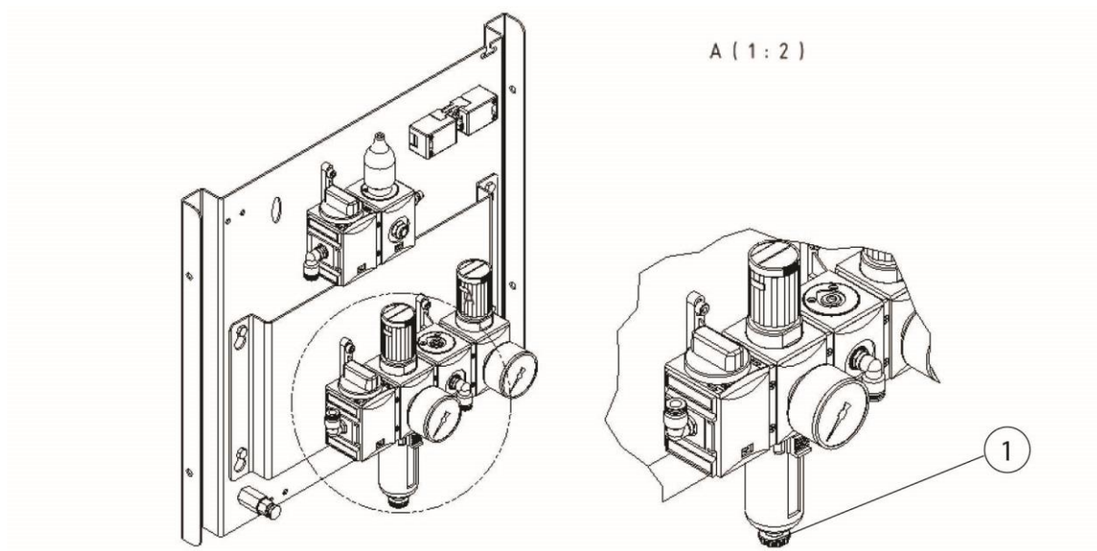
Fig. 53 : soupape de vidange des condensats unité de maintenance d'air comprimé
