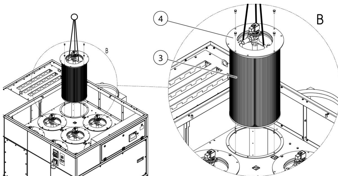
Fig. 49 : Remplacement du filtre – Démontage du porte-filtre
