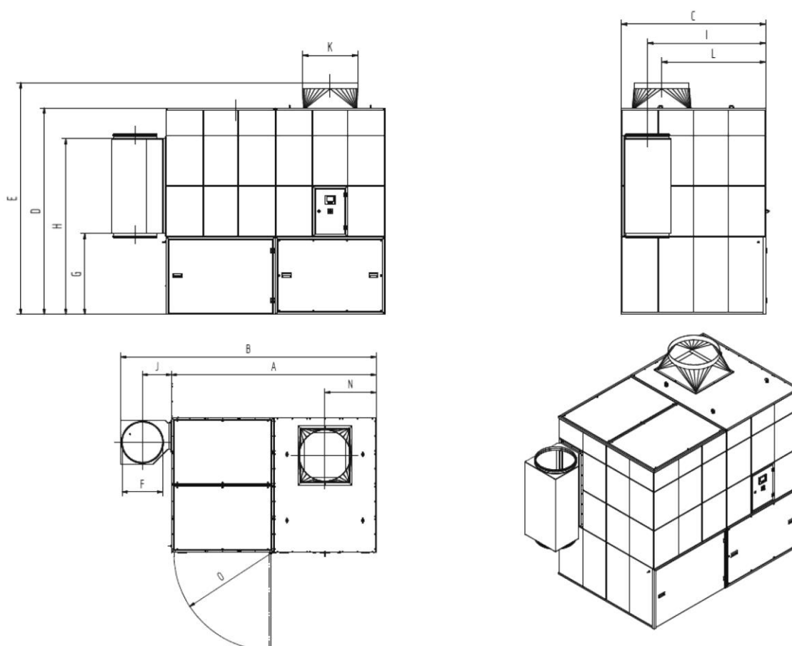
286. ábra: Méretlap - 328528 + 328529 + 3211029
