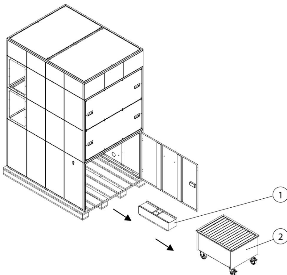
Sl. 305: Odstranitev zbiralnika za prah in dvižne naprave
