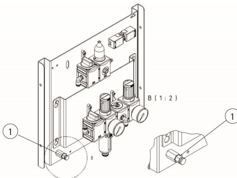
Rys. 136: Zawór spustowy skroplin zbiornika sprężonego powietrza
