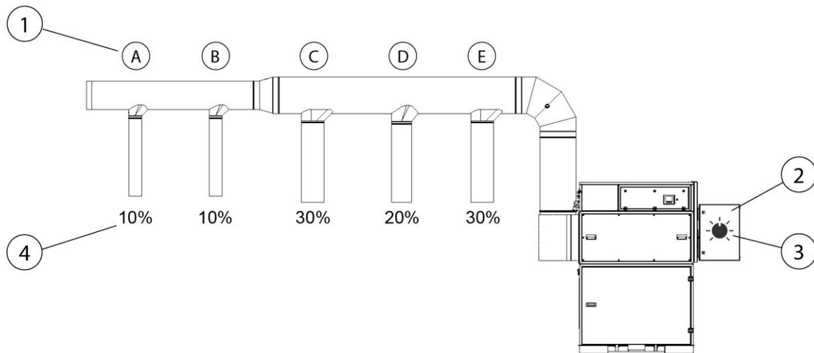
271. ábra: Az elszívási teljesítmény-szabályozó beállítása
