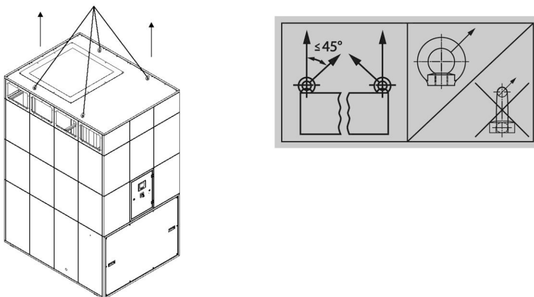
Рис. 155: Подъем вентилятора в сборе краном
