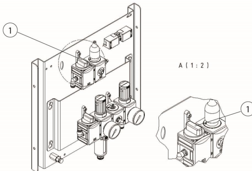
272. ábra: Porgyűjtő tartály pneumatikus szelepe
