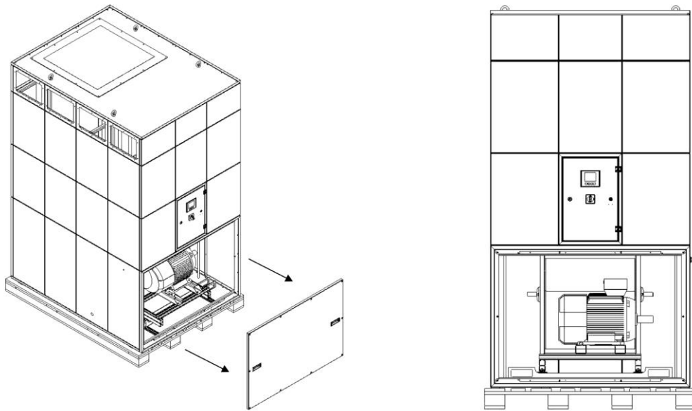
226. ábra: Ventilátorrész és karbantartási ajtó kinyitása
