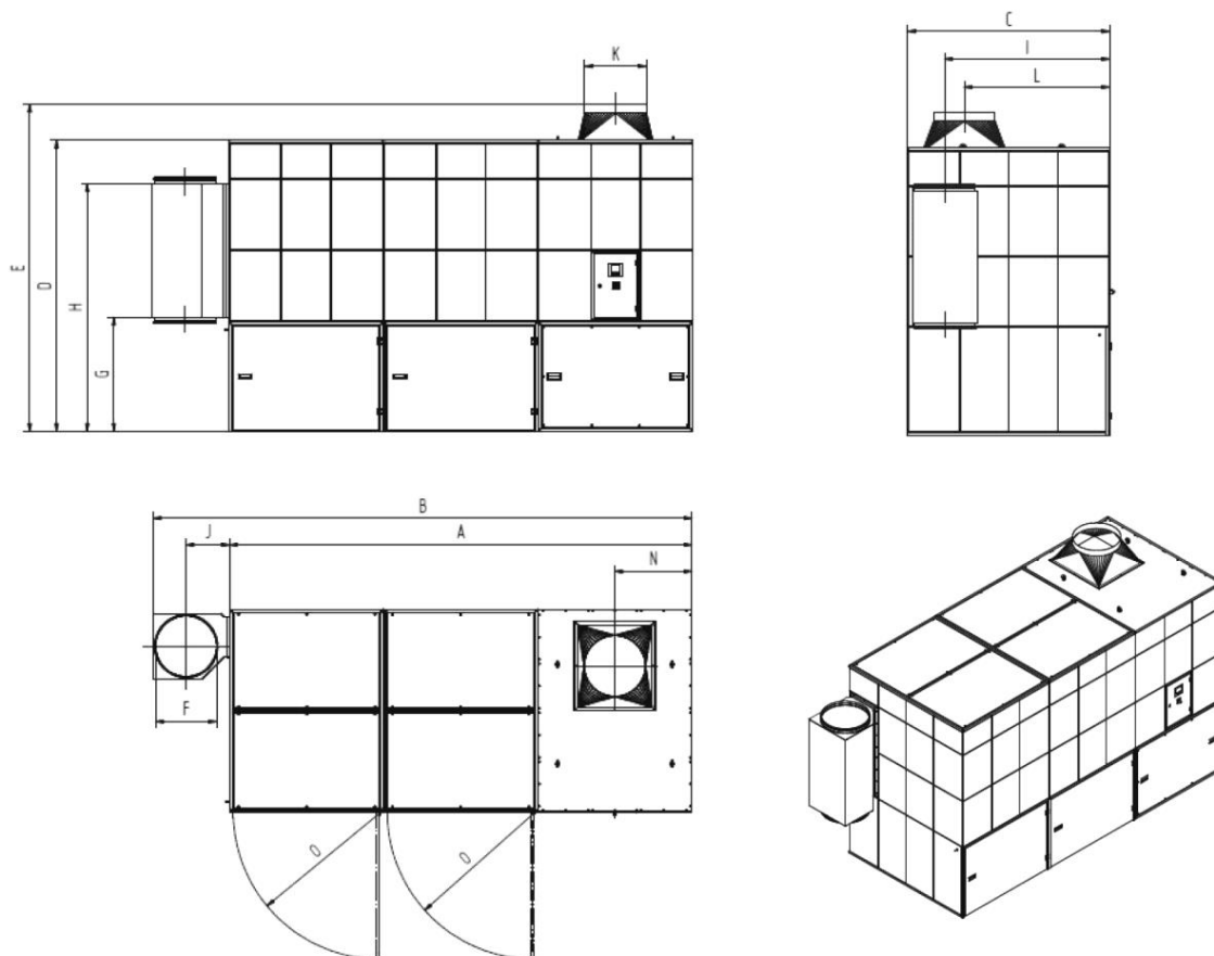
Рис. 215: Габаритный чертеж 32110211 + 32110212 + 32130211 + 32130212 + 32130213
