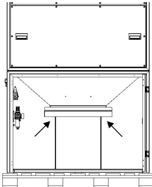
Рис. 164: Подъем фильтровального блока вилочным погрузчиком
