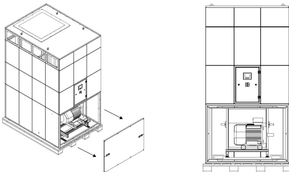
Rys. 82: Otworzyć drzwiczki serwisowe w module wentylatora
