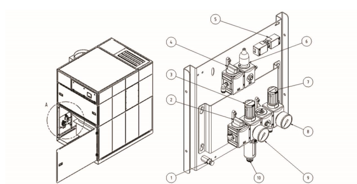
244. ábra: Sűrített levegős egység
