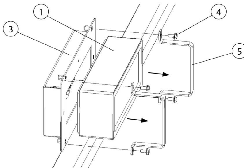
Рис. 204: Замена защитного фильтра
