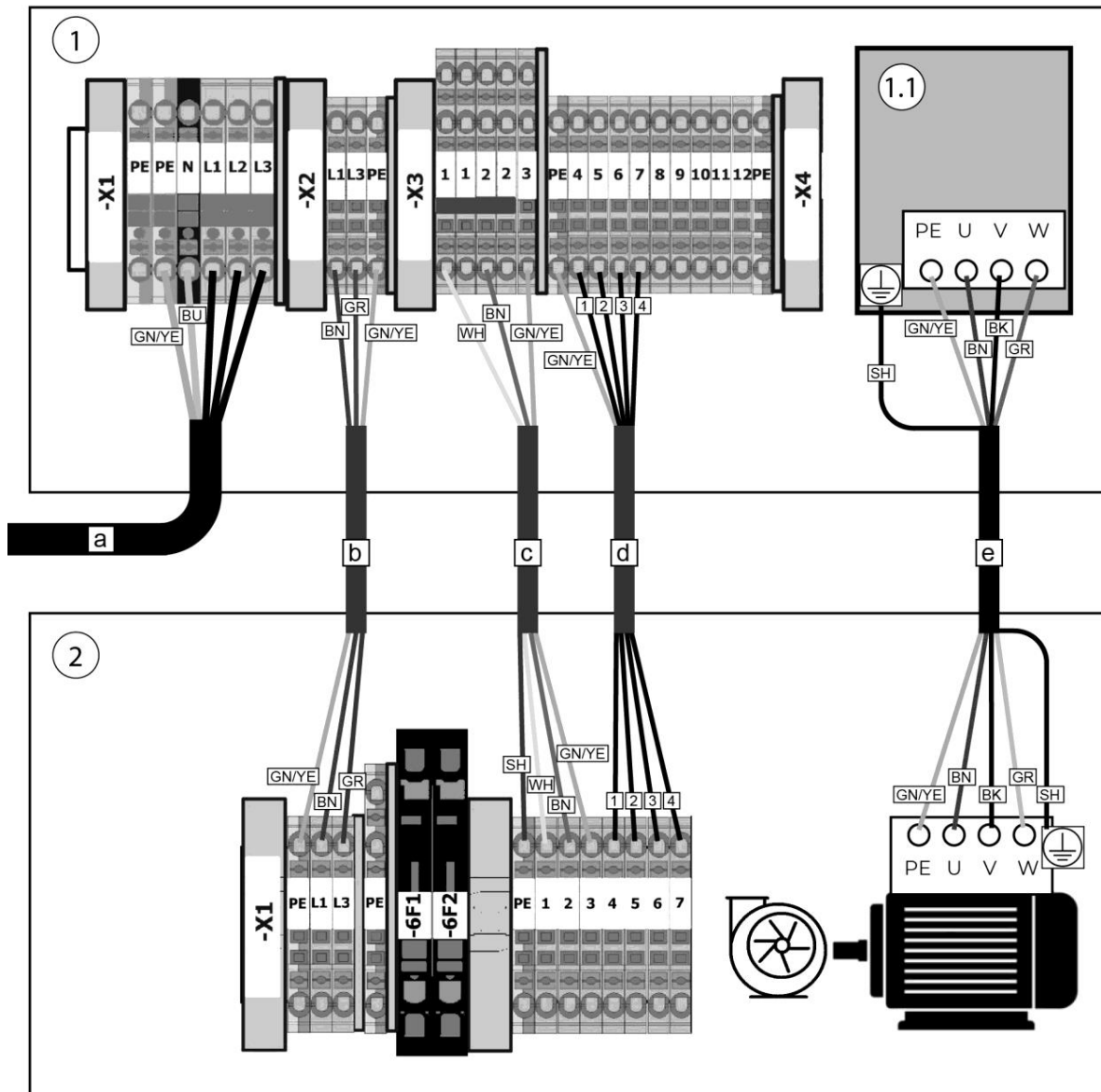
Sl. 324: diagram ožičenja upravljanja zmogljivosti odsesavanja z izdelkom
