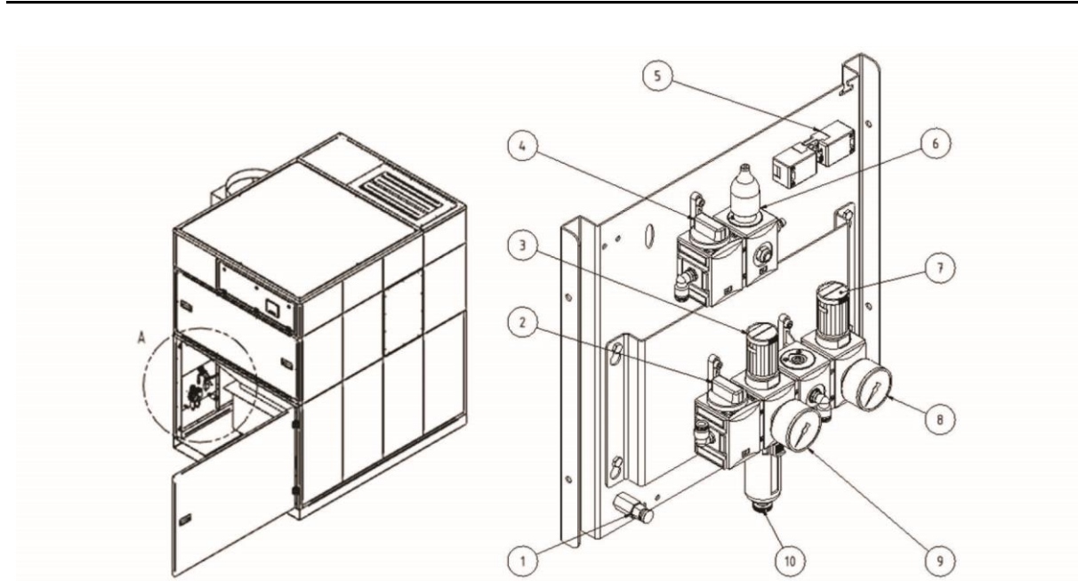
Rys. 100: Jednostka sprężonego powietrza
