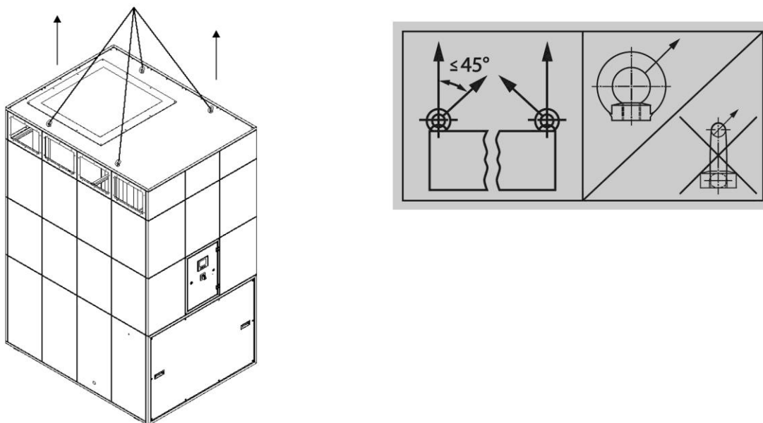
Obr. 11: Nadzvednutí jednotky ventilátoru jeřábem
