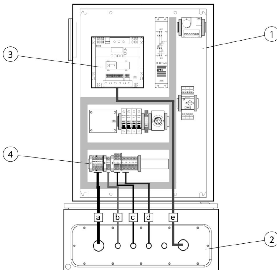
Рис. 179: Распределительный шкаф регулирования мощности вытяжки
