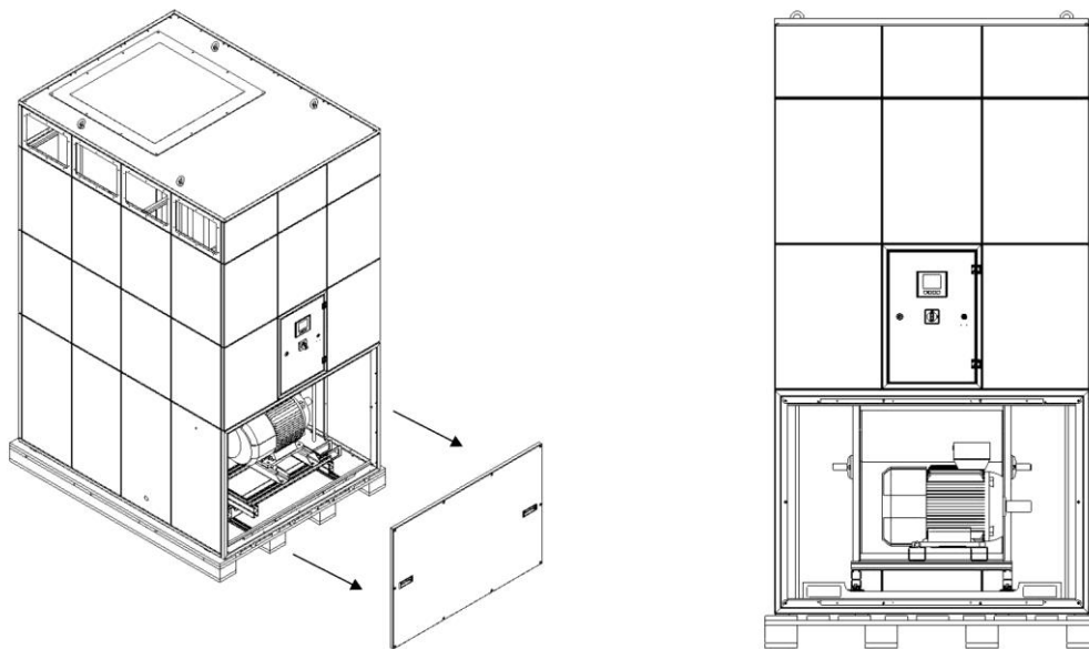
Sl. 298: Odpiranje servisnih vrat ventilatorskega dela
