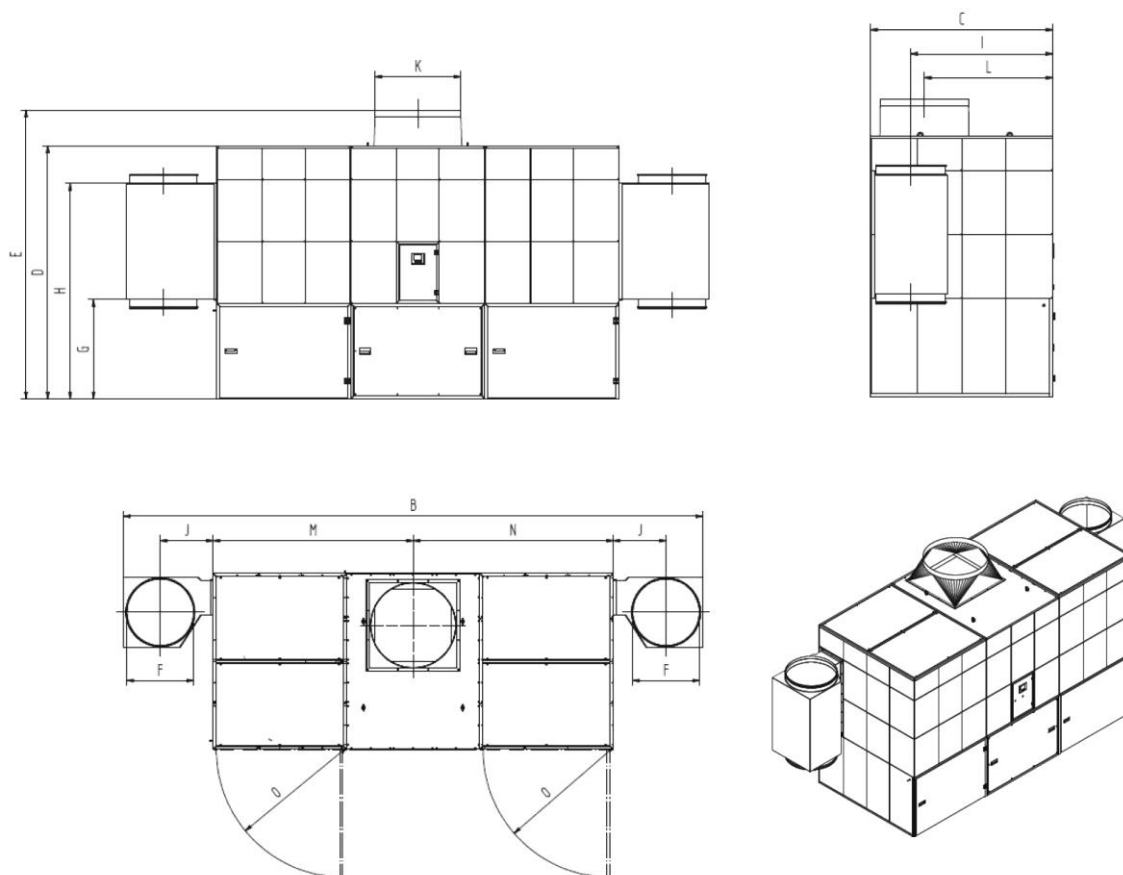
Obr. 72: Rozměrový výkres 32160213 + 32160214 + 32180216 + 32180218
