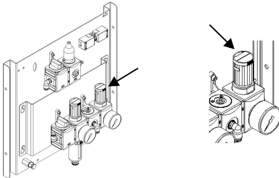
Рис. 175: Регулировка давления грузоподъемного приспособления/ пылесборник.
