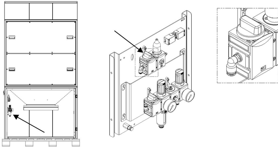
231. ábra: Porgyűjtő tartály lesüllyesztő szelepe
