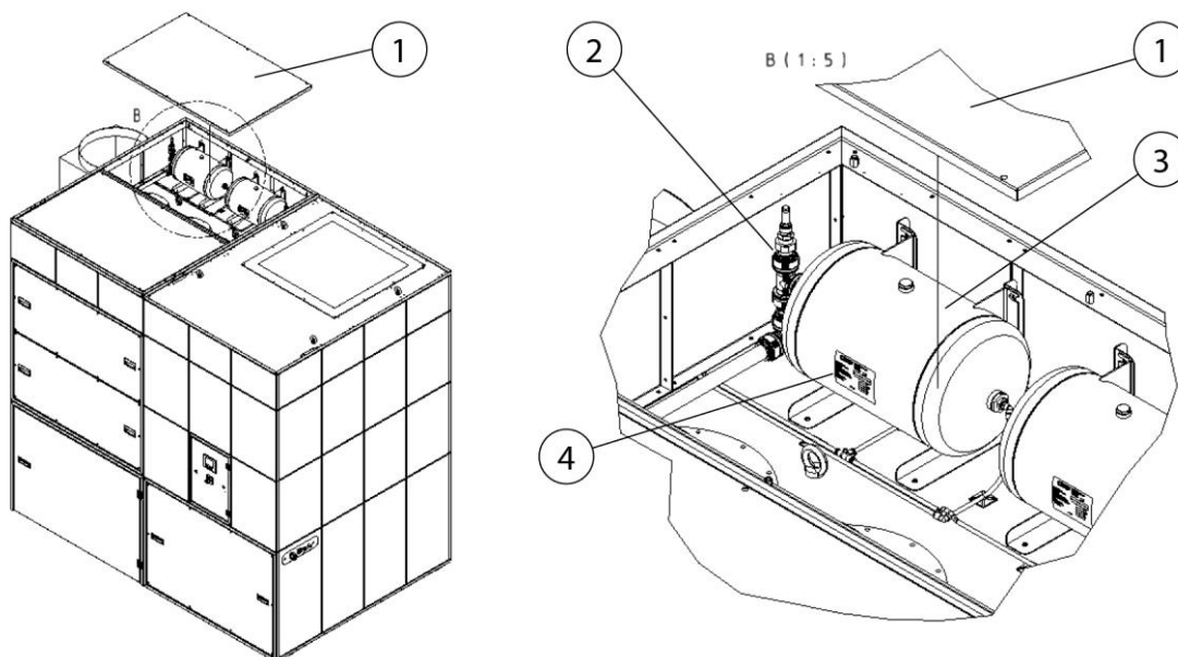
Obr. 68: Přístup k zásobníku stlačeného vzduchu a pojistnému ventilu
