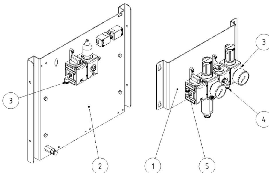
Obr. 32: Pneumatická jednotka
