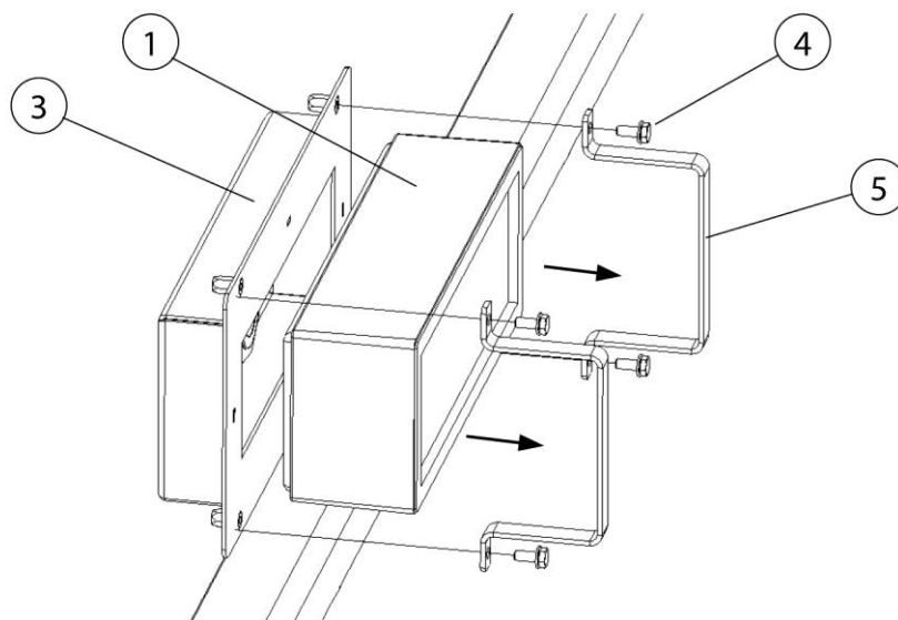
276. ábra: Biztonsági szűrő cseréje
