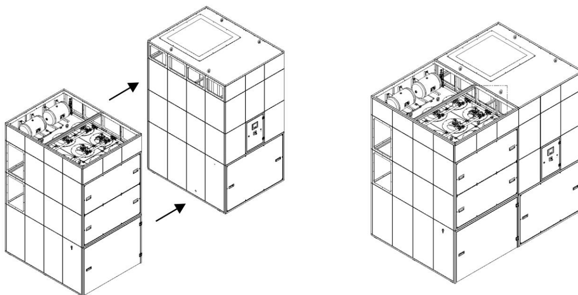
Rys. 93: Połączyć wentylator z filtrem
