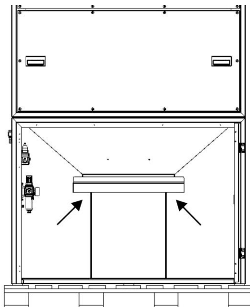
Sl. 308: Dvigovanje filtrskega dela z viličarjem
