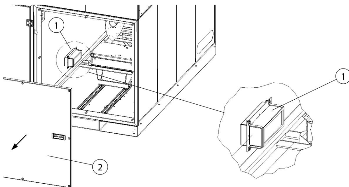
Рис. 203: Доступ к защитному фильтру
