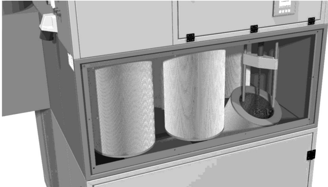
Obr. 63: Výměna filtrů – vyjmutí filtračních patron
