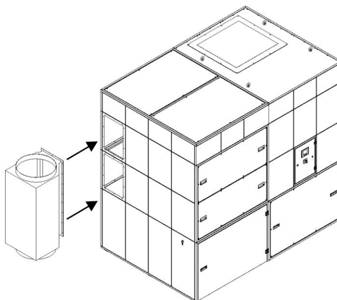
Rys. 99: Montaż skrzynki przyłączeniowej od strony odciągu
