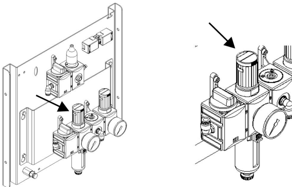
246. ábra: Üzemi nyomás beállítása
