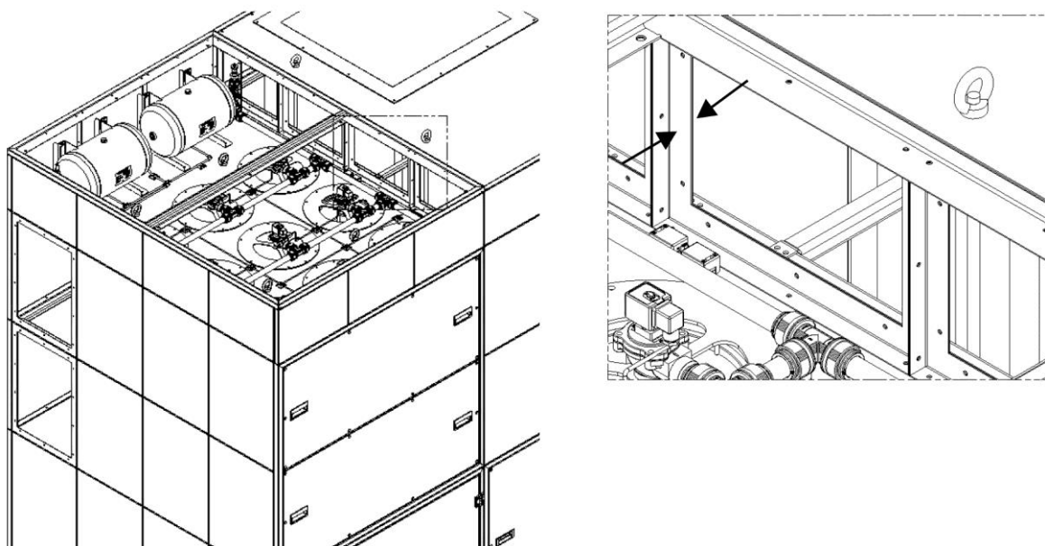
Rys. 94: Połączyć wentylator z filtrem
