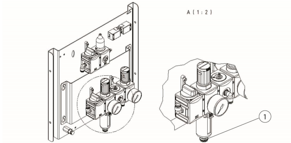
Rys. 137: Zawór spustowy skroplin jednostki uzdatniania sprężonego powietrza
