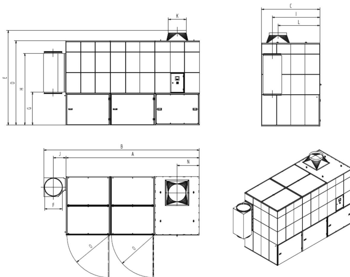
287. ábra: Méretlap - 32110211 + 32110212 + 32130211 + 32130212 + 32130213
