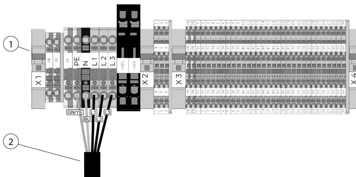
Рис. 177: Рейка с присоединительными зажимами в распределительном шкафу изделия
