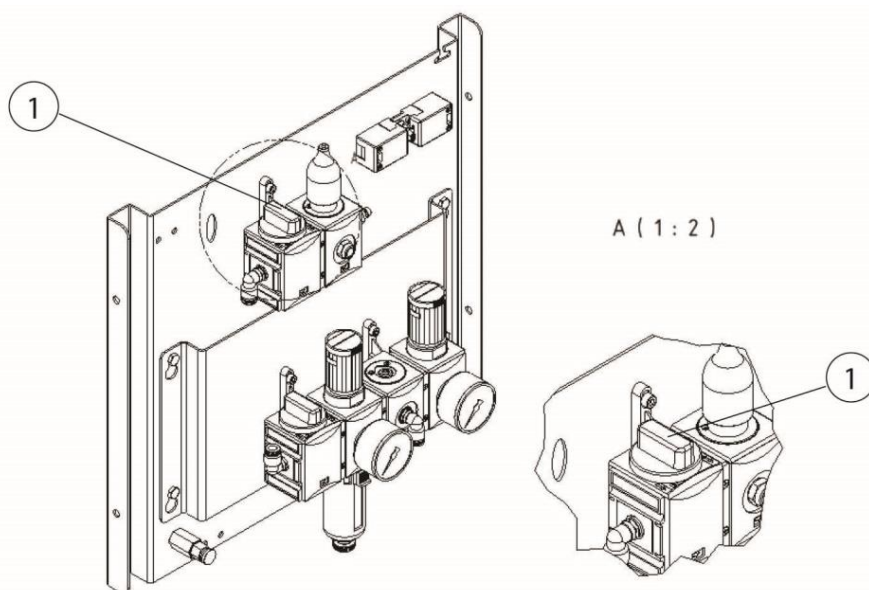
Sl. 344: Ventil stisnjenega zraka zbiralnika za prah
