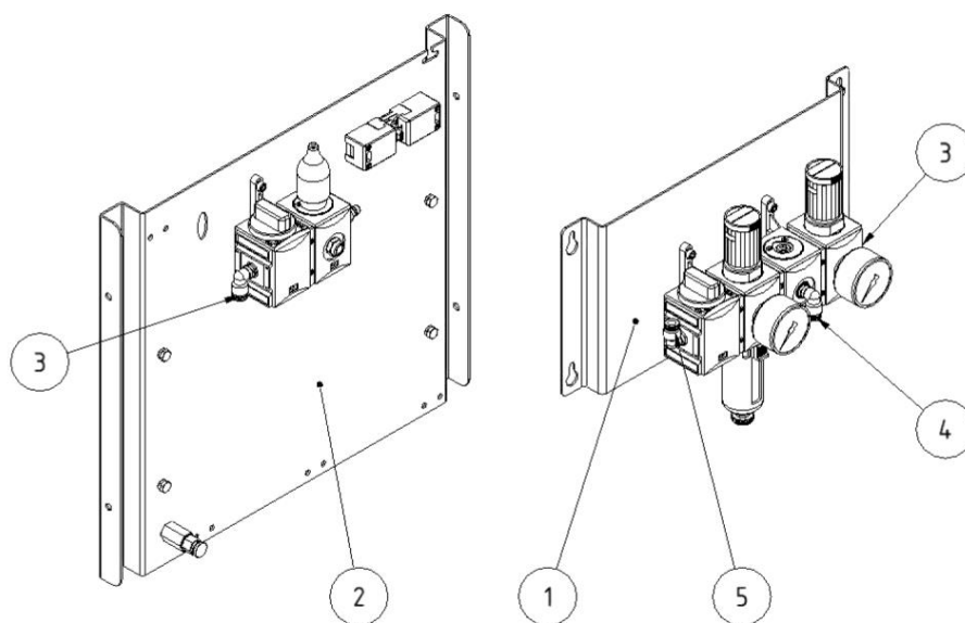
Рис. 176: Узел пневмосистемы
