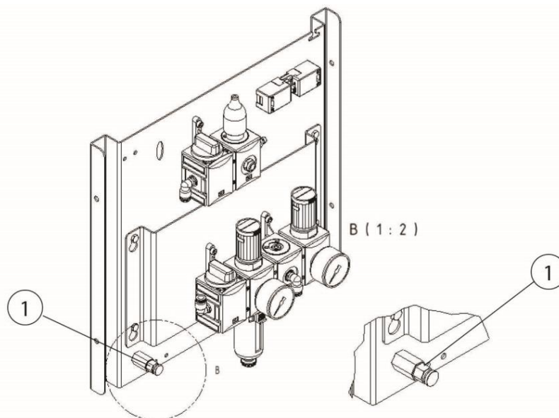
Рис. 208: Вентиль слива конденсата из ресивера
