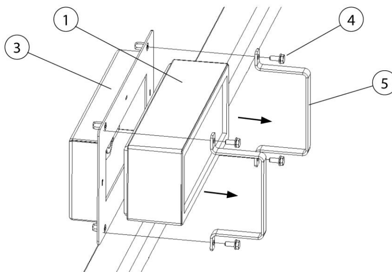
Obr. 60: Výměna bezpečnostního filtru
