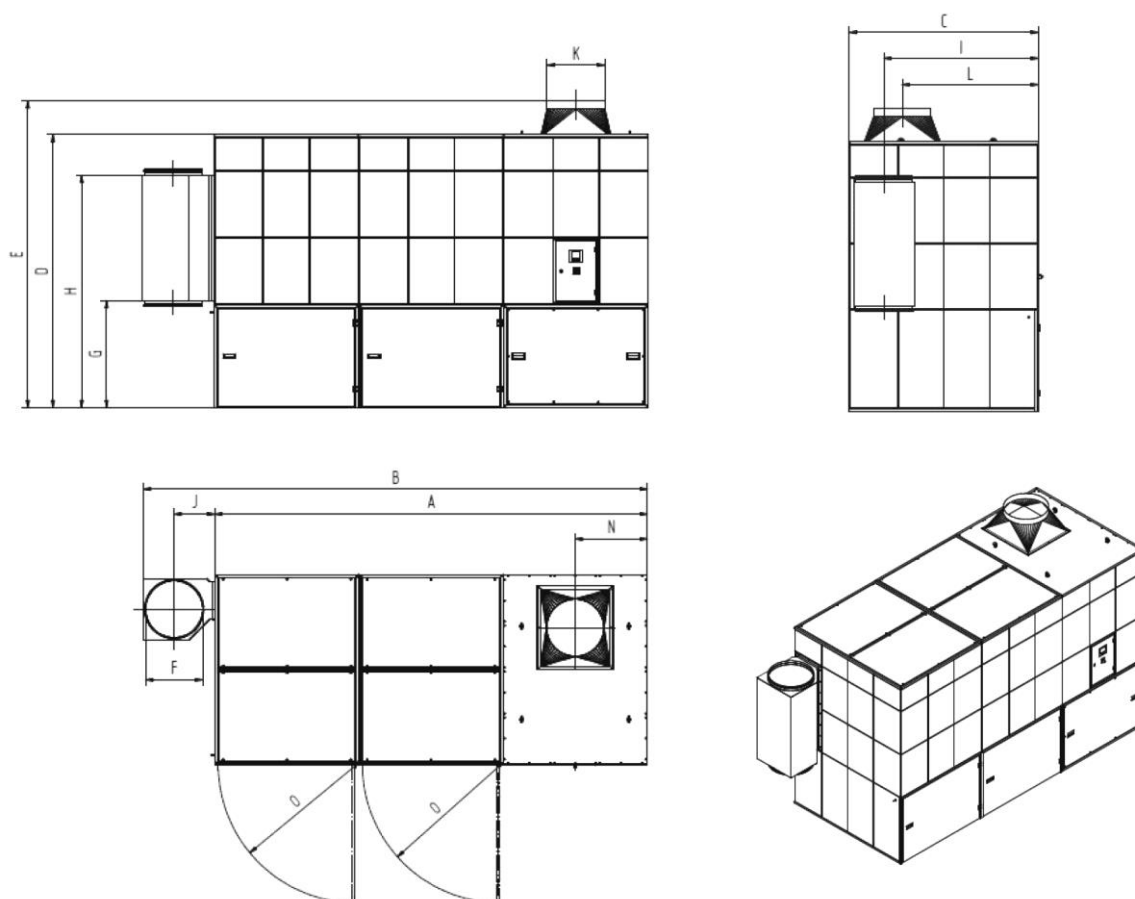
Obr. 71: Rozměrový výkres 32110211 + 32110212 + 32130211 + 32130212 + 32130213
