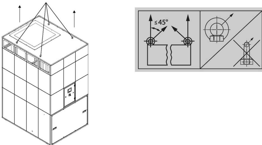
Sl. 299: Dvig ventilatorskega dela z žerjavom
