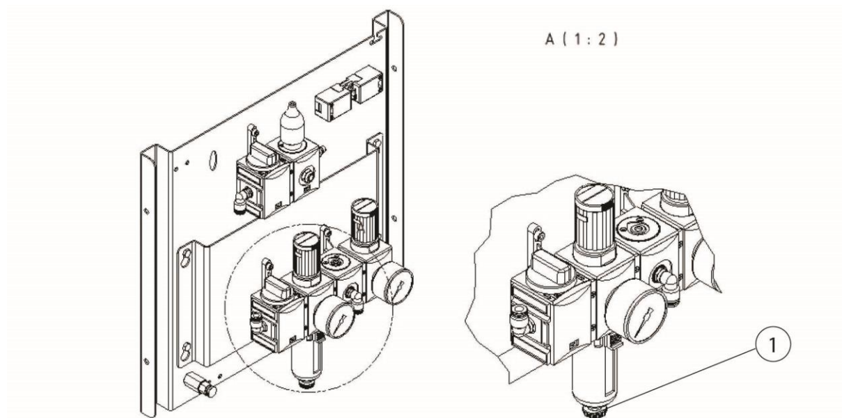
Obr. 65: Vypouštěcí ventil kondenzátu jednotky pro úpravu stlačeného vzduchu
