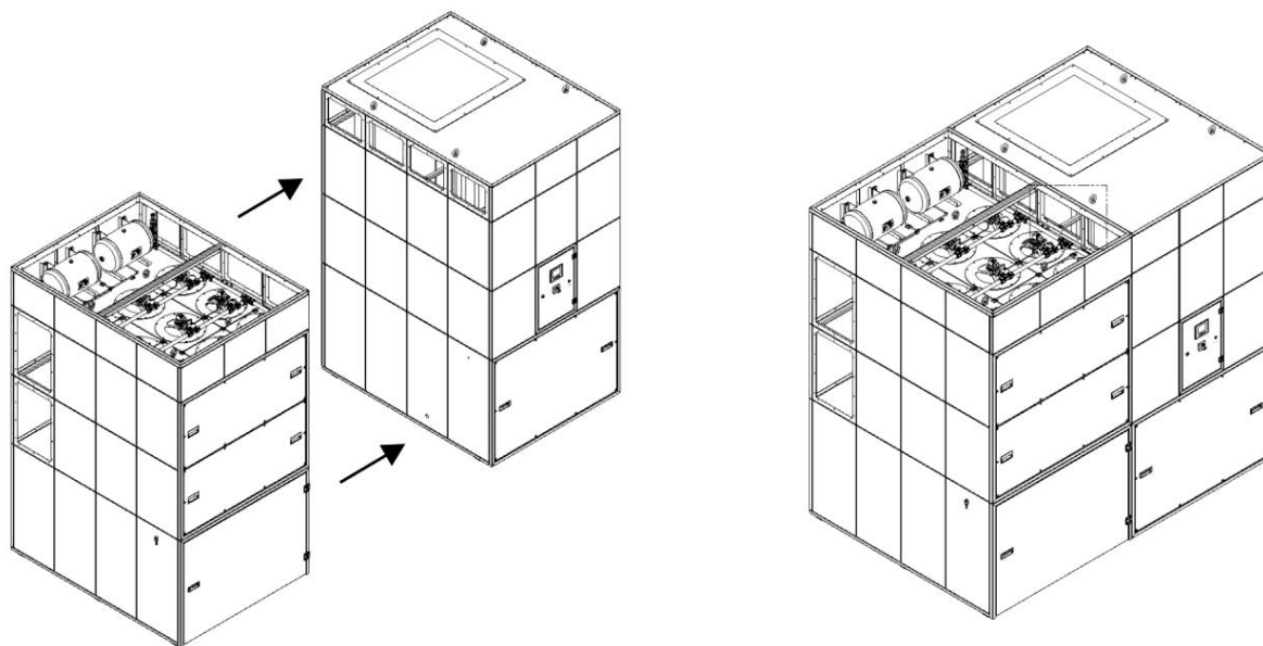
Рис. 165: Соединение фильтра в сборе с вентилятором в сборе
