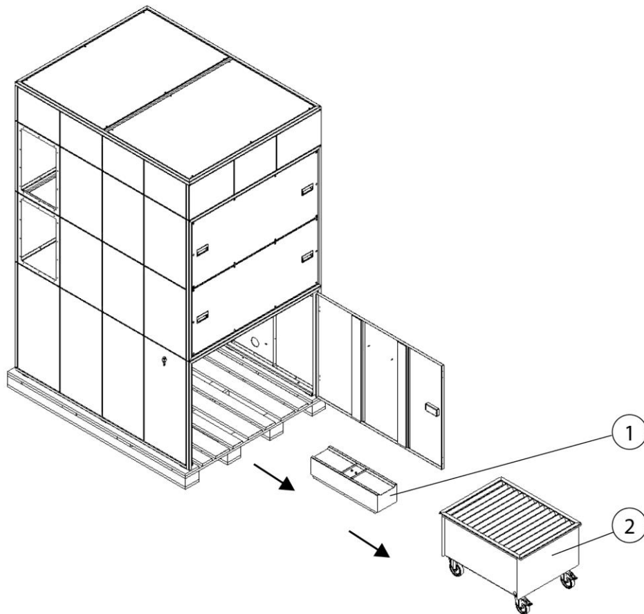
233. ábra: A porgyűjtő tartály és az emelőberendezés eltávolítása
