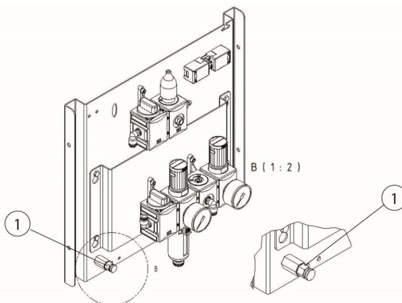
Obr. 64: Vypouštěcí ventil kondenzátu zásobníku stlačeného vzduchu
