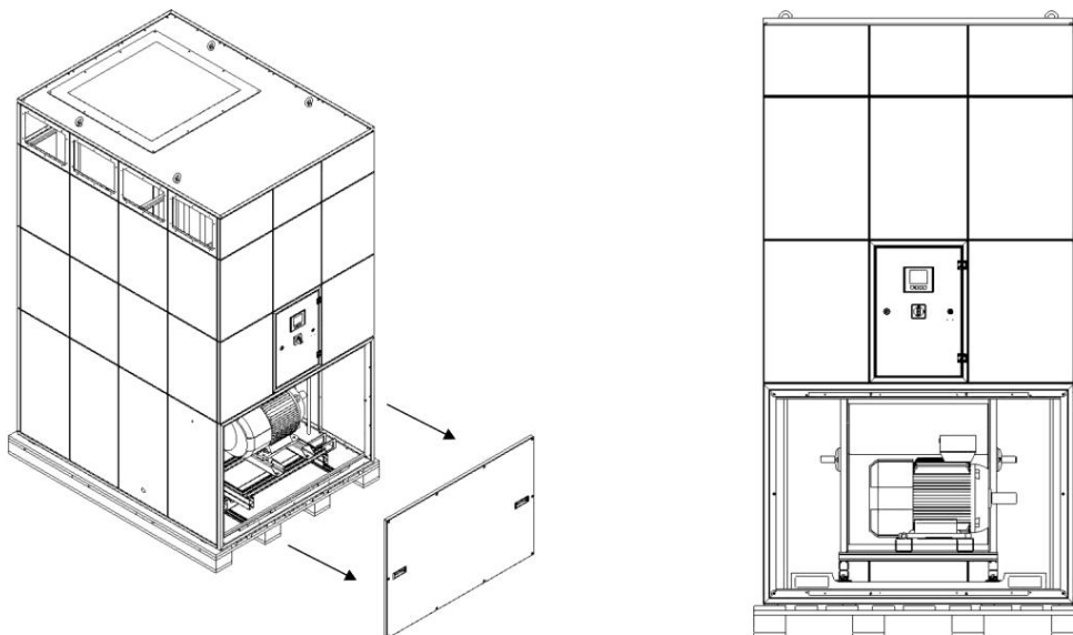
Рис. 154: Открыть дверь для техобслуживания вентилятора
