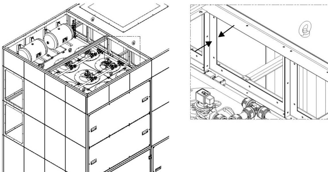
Рис. 166: Соединение вентилятора с фильтром
