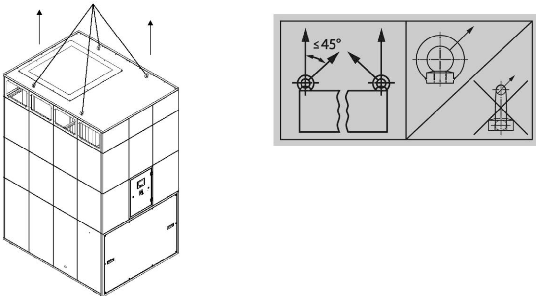
227. ábra: Ventilátorrész megemlése daruval
