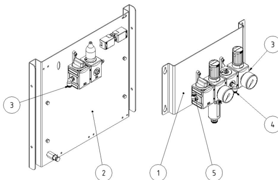
Sl. 320: Enota s stisnjenim zrakom
