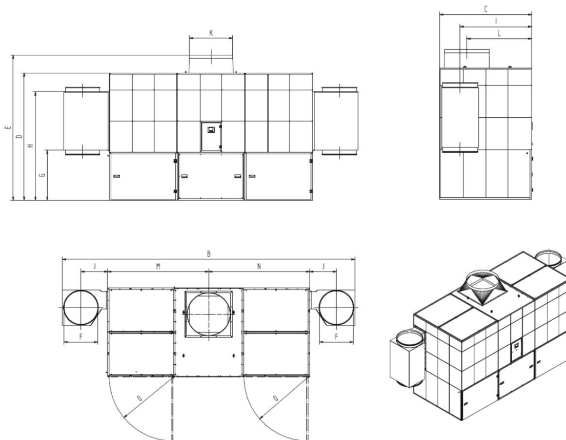
Рис. 216: Габаритный чертеж 32160213 + 32160214 + 32180216 + 32180218
