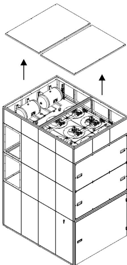
Rys. 90: Zdejmowanie pokrywy blaszanej
