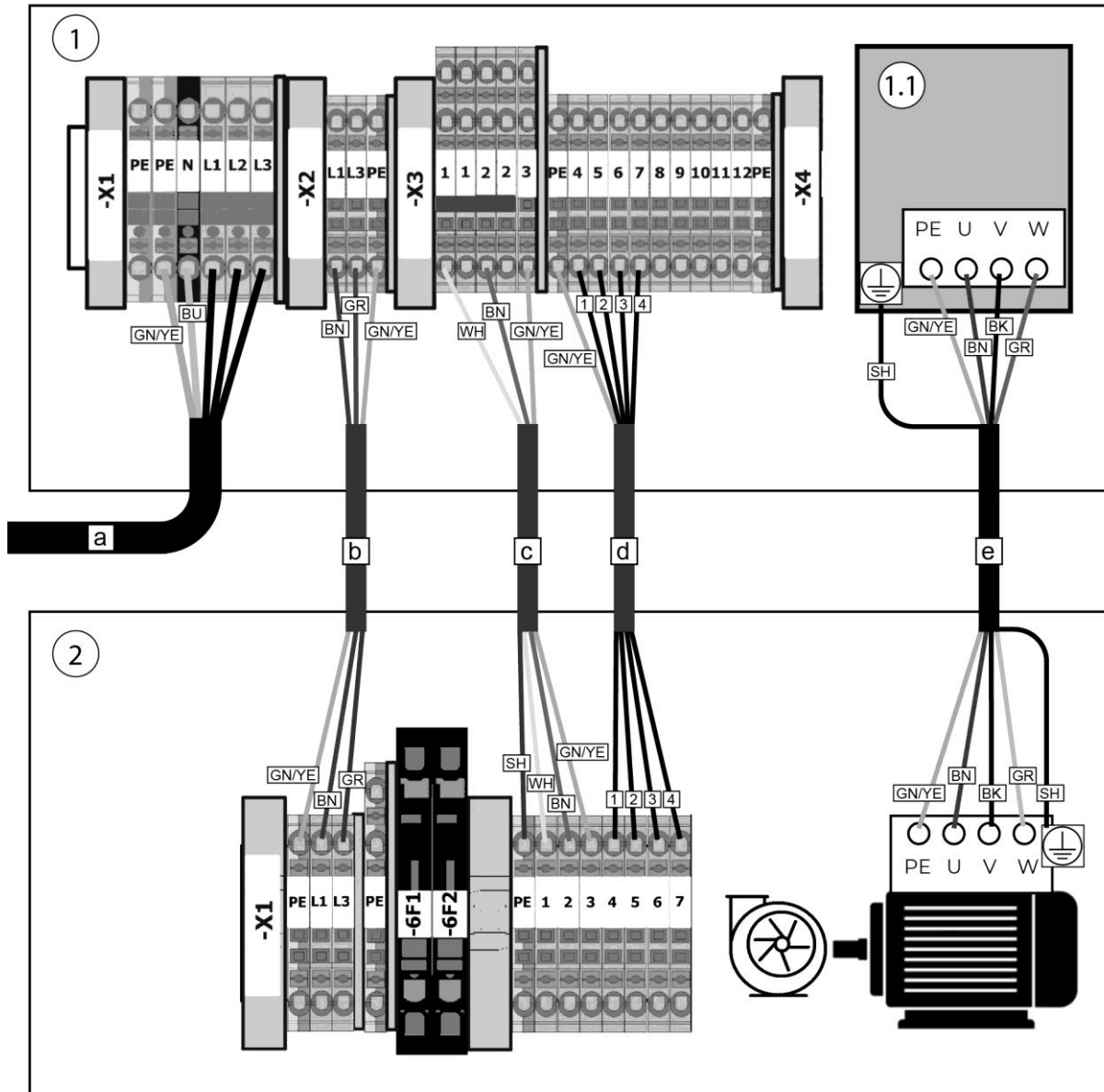
Obr. 36: Schéma elektrického zapojení regulace odsávacího výkonu s výrobkem
