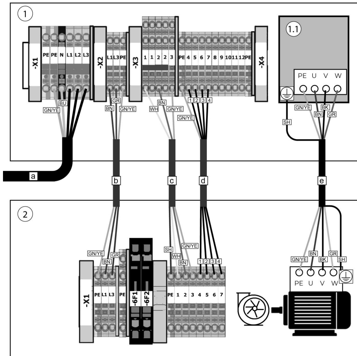
252. ábra: Huzalozási terv - elszívási teljesítmény-szabályozó és termék
