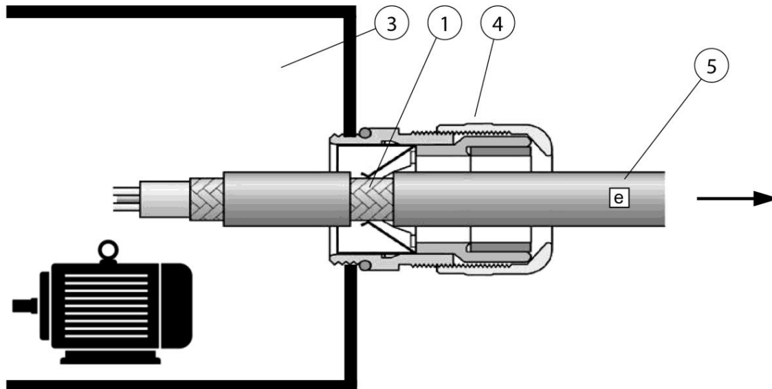
Sl. 326: Priključitev zaslona motornega kabla
