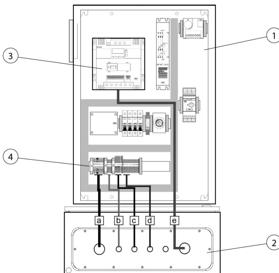
Sl. 323: Nadzorna omarica upravljanja zmogljivosti odsesavanja
