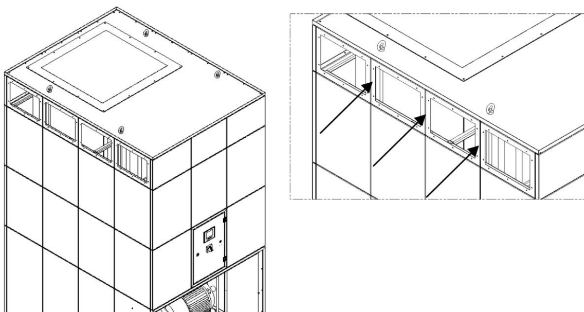
Sl. 301: Dovod čistega zraka
