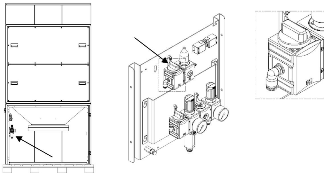
Obr. 15: Ventil pro snižování sběrné nádoby na prach
