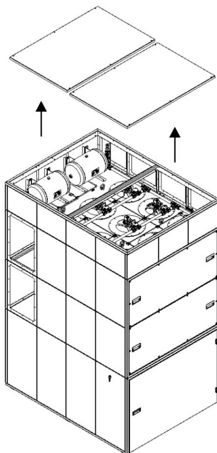
Рис. 162: Демонтаж крышки
