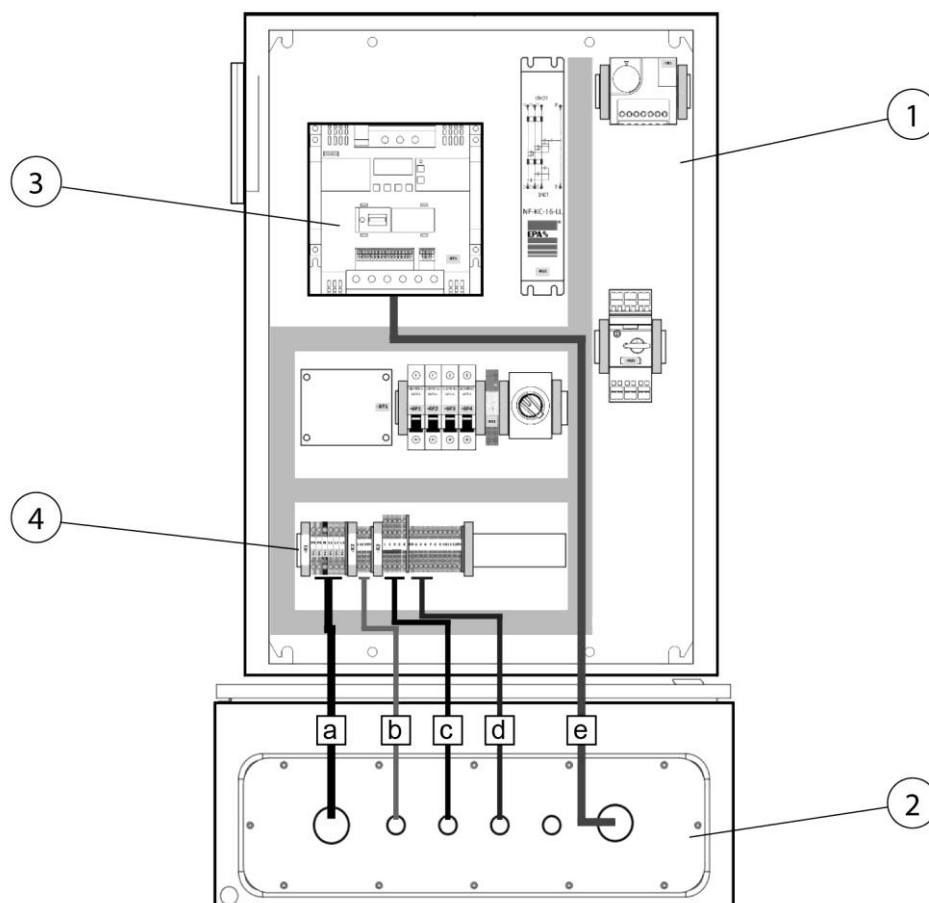
Rys. 107: Szafa rozdzielcza, układ regulacji mocy ssącej
