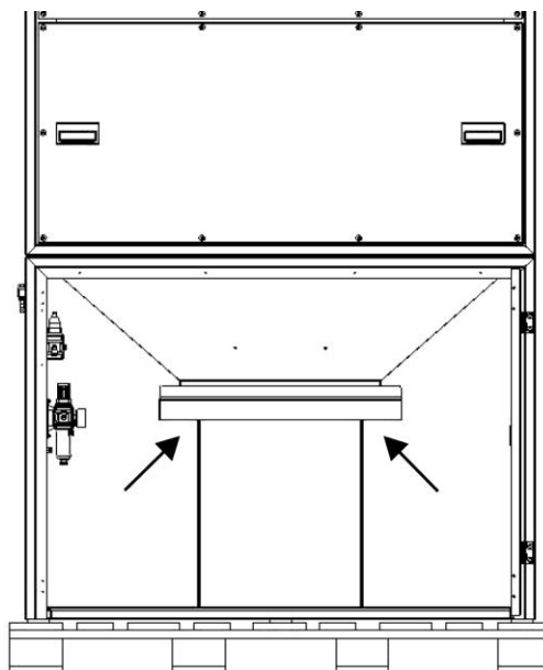
Rys. 92: Podnoszenie modułu filtra za pomocą wózka widłowego
