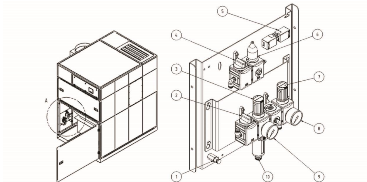
Obr. 28: Pneumatická jednotka
