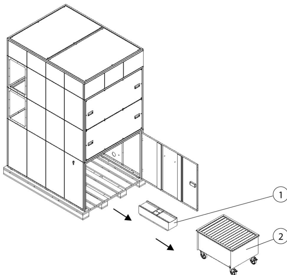
Рис. 161: Извлечение пылесборника и подъемника
