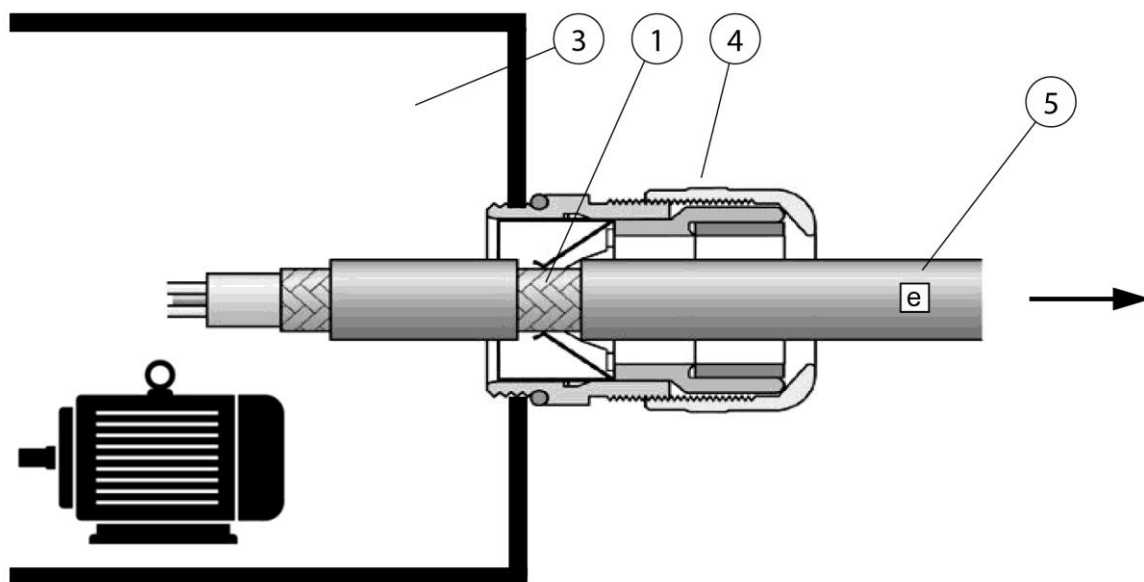
Obr. 38: Připojení stínění kabelu motoru
