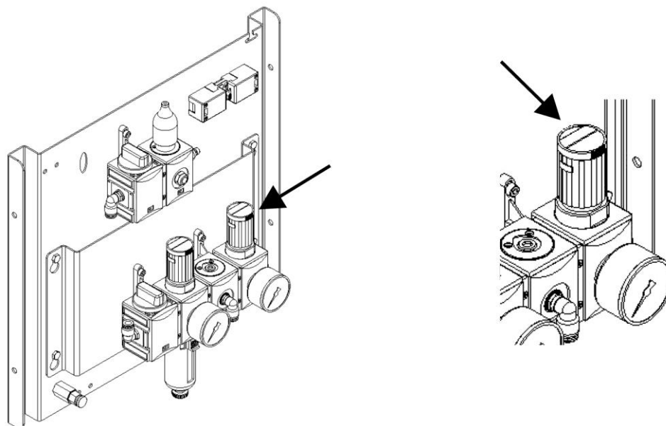
Sl. 319: Nastavitev tlaka dvizhne naprave/zbiralnika za prah
