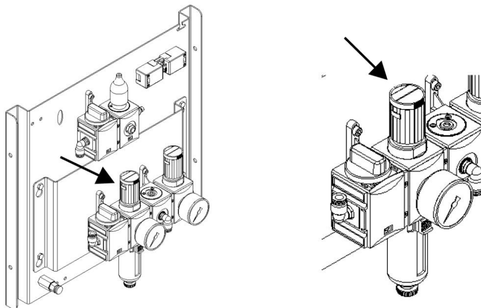
Sl. 318: Nastavitev delovnega tlaka
