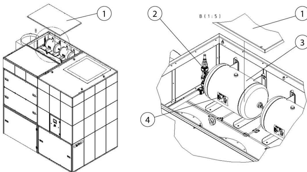
Рис. 212: Доступ к ресиверу сжатого воздуха и предохранительному клапану
