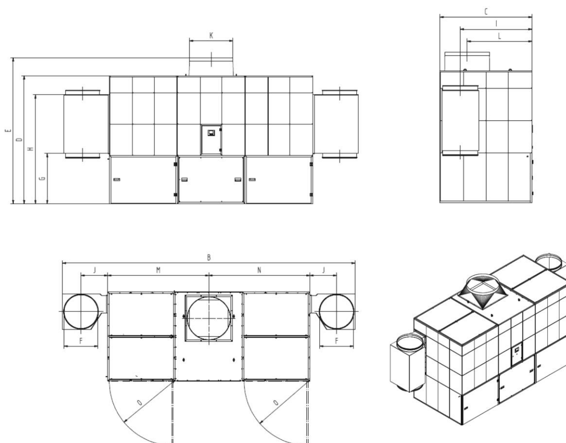
Rys. 144: Karta wymiarów 32160213 + 32160214 + 32180216 + 32180218
