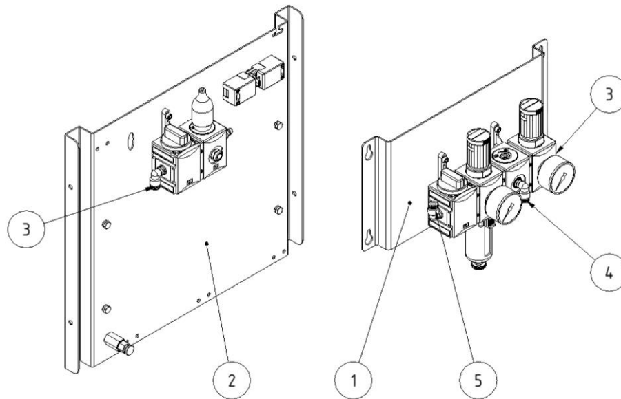
248. ábra: Sűrített levegős egység
