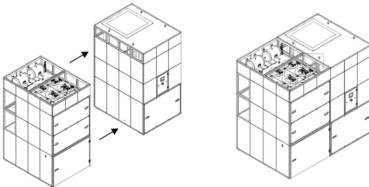
Obr. 21: Spojení filtrační jednotky s jednotkou ventilátoru
