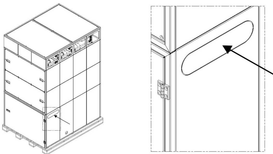
Рис. 158: Панель продольного отверстия
