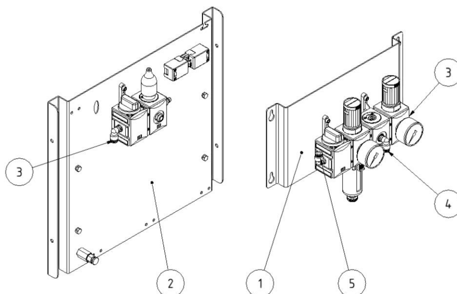
Rys. 104: Jednostka sprężonego powietrza
