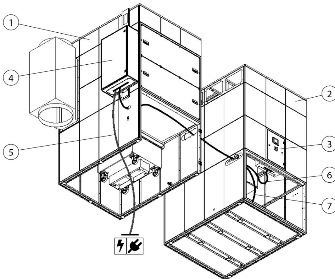
Sl. 322: Primer: Položitev kabla za upravljanje zmogljivosti odsesavanja
