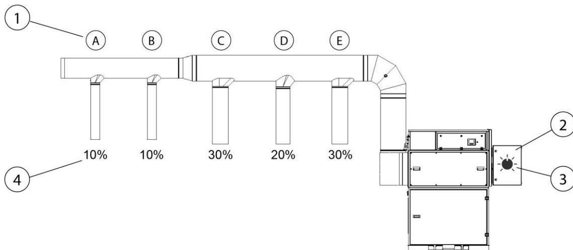
Sl. 343: Nastavitev upravljanja zmogljivosti odsesavanja
