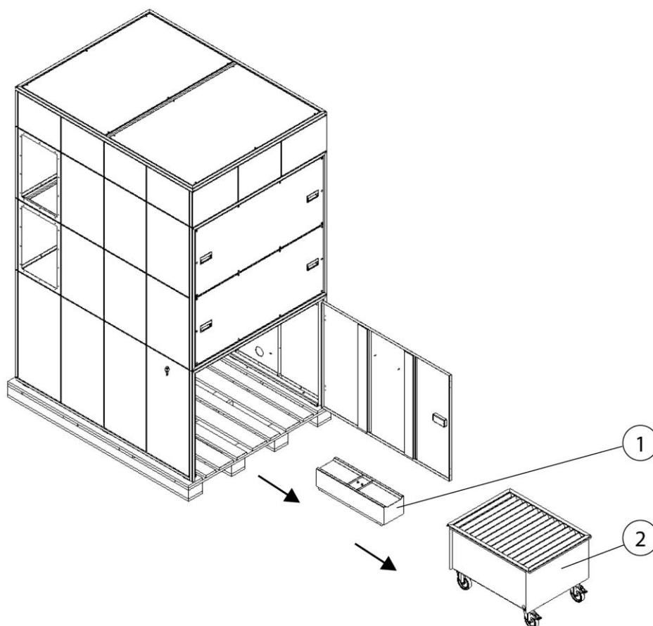
Obr. 17: Vyjmutí sběrné nádoby na prach a zvedacího zařízení
