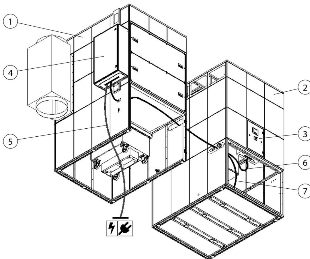
Rys. 106: Przykład: Przebieg przewodu układu regulacji mocy ssącej
