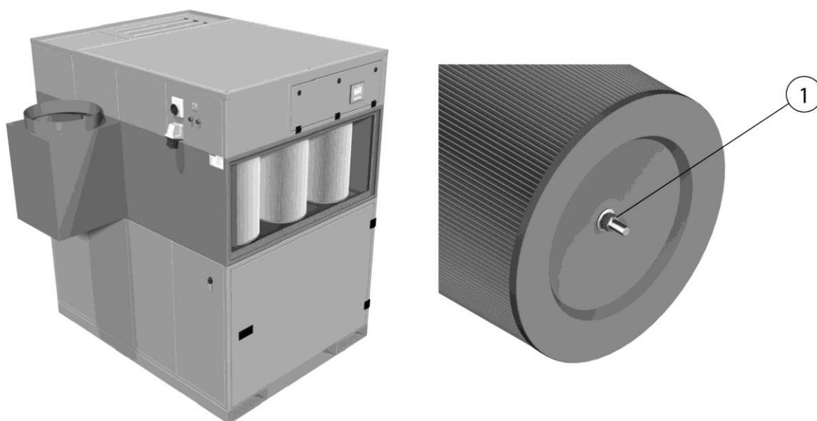
Obr. 61: Výměna filtru – servisní kryt
