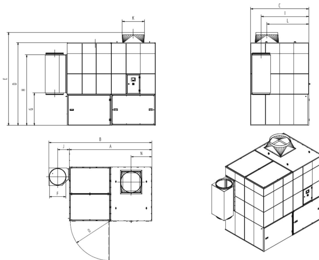
Рис. 214: Габаритный чертеж 328528 + 328529 + 3211029
