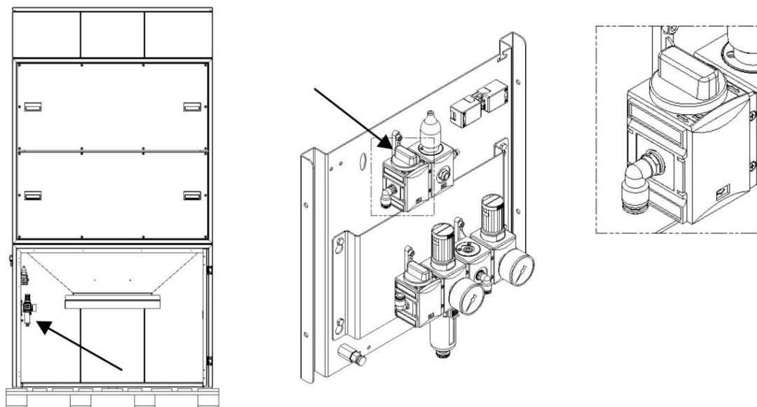
Рис. 159: Клапан опускания пылесборника
