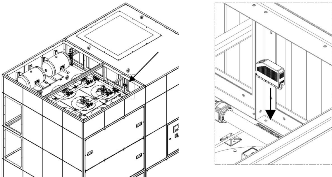
239. ábra: Zöld színű csatlakozódugó felszerelése
