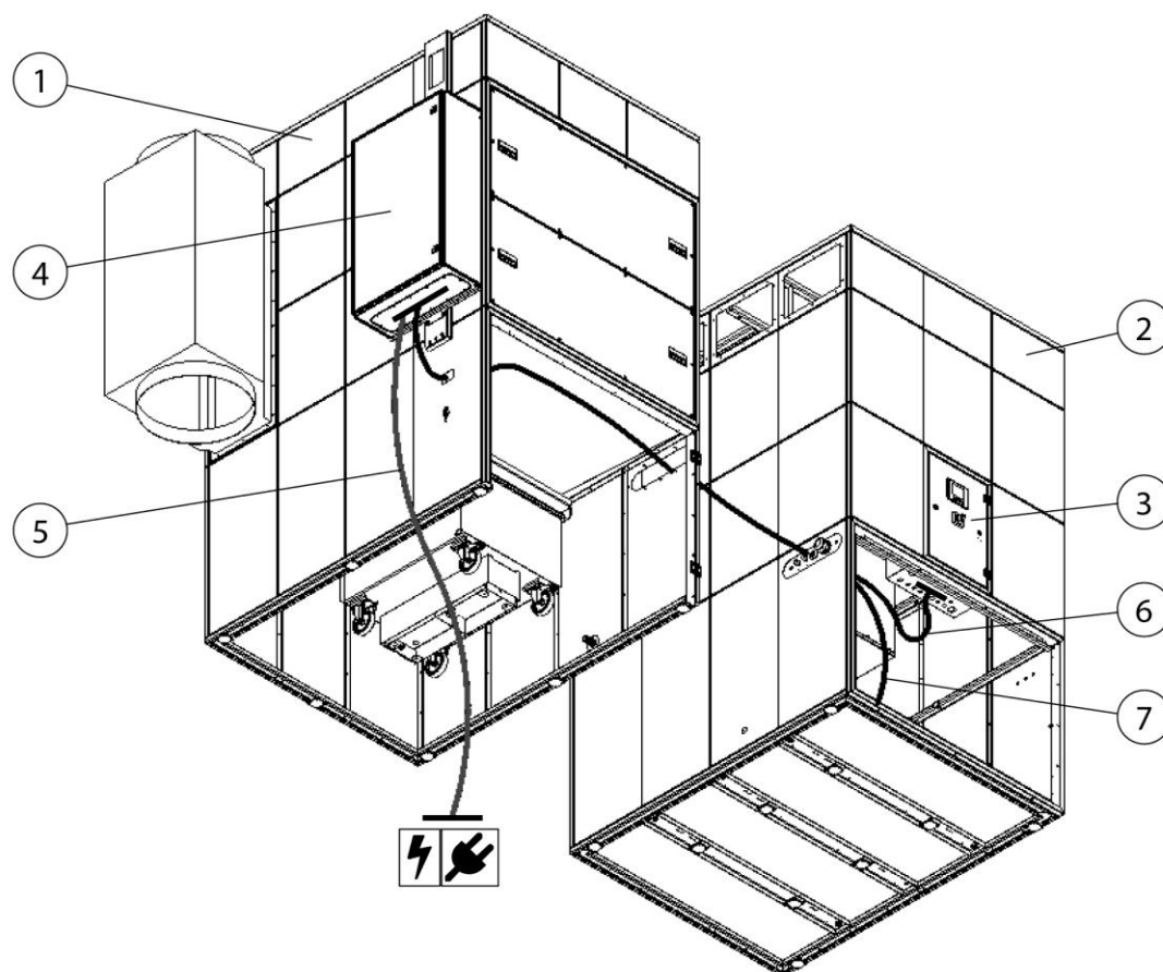
Рис. 178: Пример: прокладка кабеля, вариант с регулированием мощности ВЫТЯЖКИ
