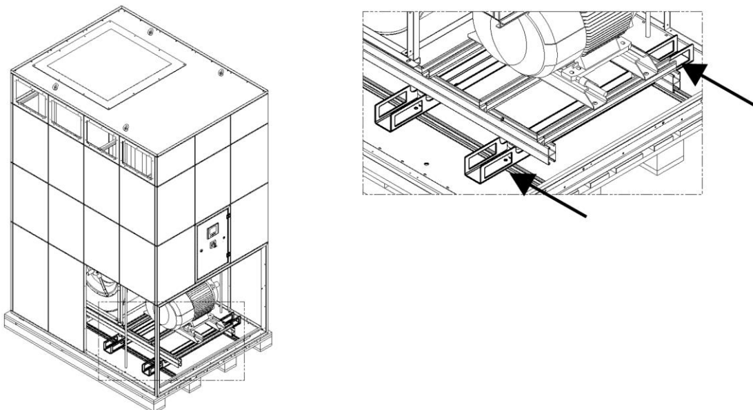
Sl. 300: Dvigovanje ventilatorskega dela z viličarjem
