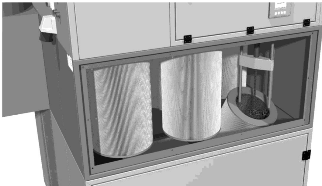
Rys. 135: Wymiana filtra- wymiana wkładu filtra
