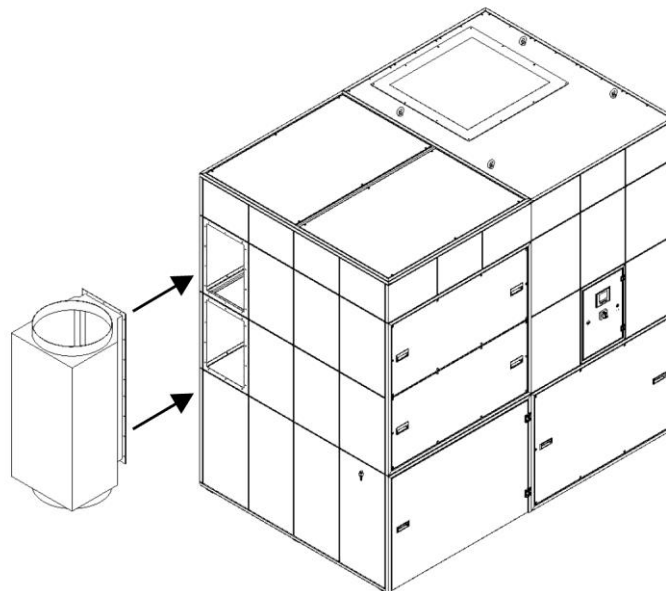
243. ábra: Szívóoldali csatlakozódoboz felszerelése
