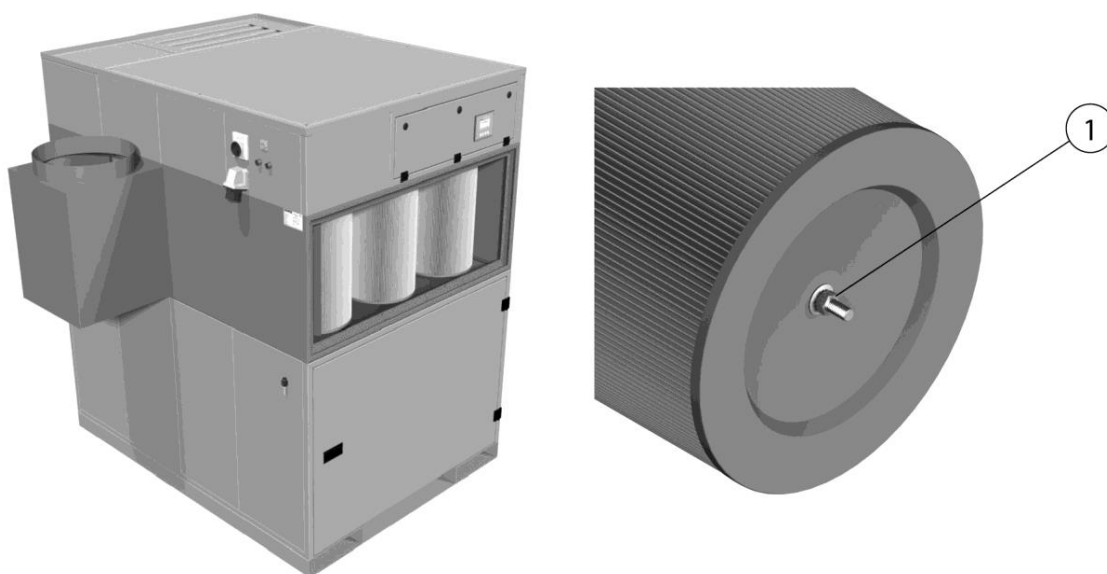
Рис. 205: Замена фильтра– крышка для технического обслуживания
