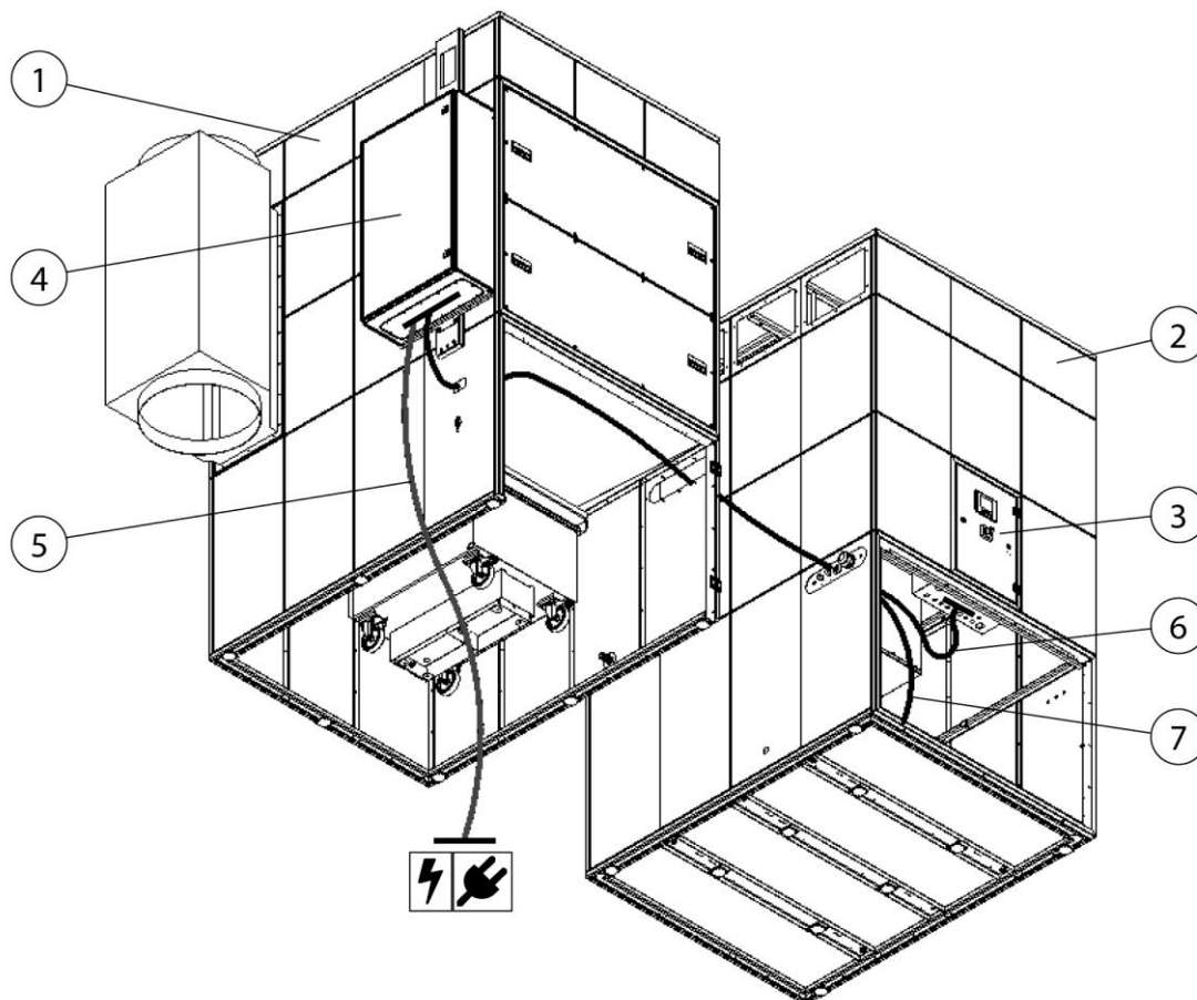
250. ábra: Példa: Az elszívási teljesítmény-szabályozó kábelének fektetése
