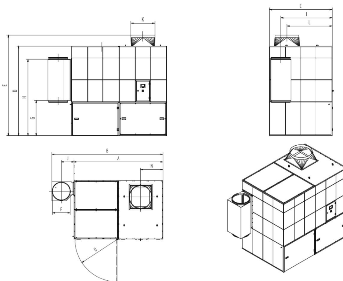
Obr. 70: Rozměrový výkres 328528 + 328529 + 3211029
