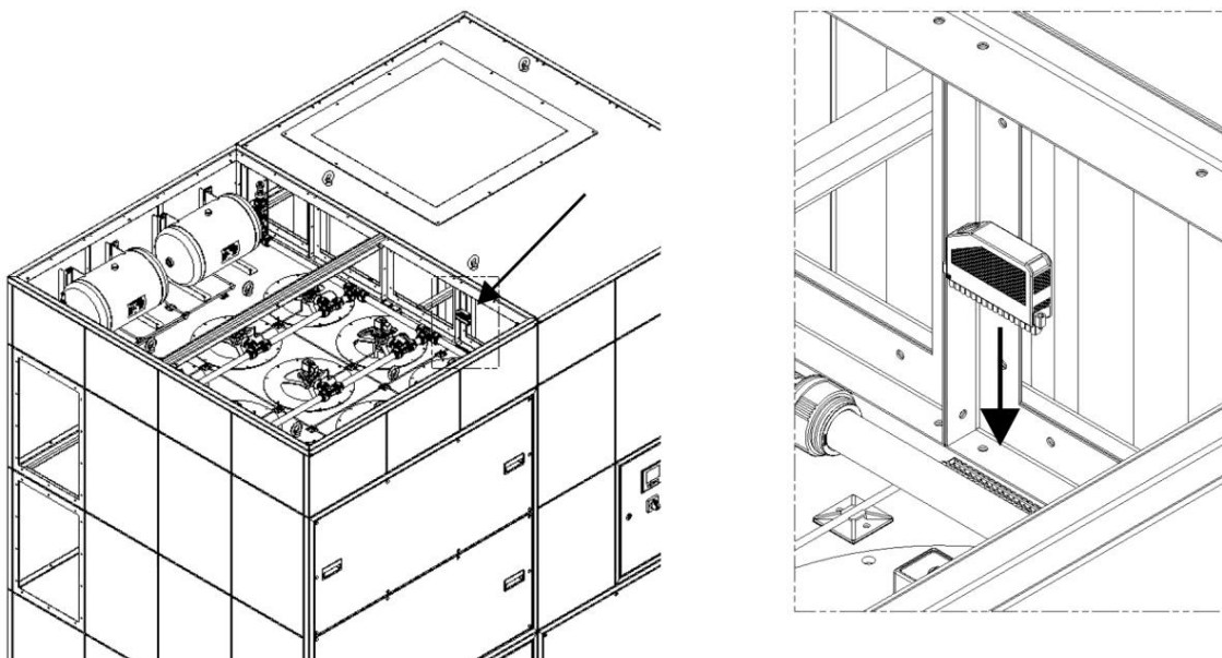
Рис. 167: Монтаж зеленого штекера
