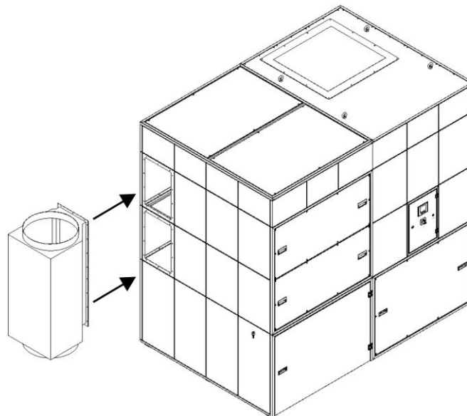
Рис. 171: Монтаж соединительной коробки на стороне всасывания
