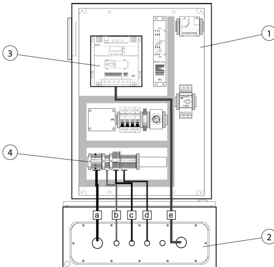
Obr. 35: Skříňový rozvaděč regulace odsávacího výkonu
