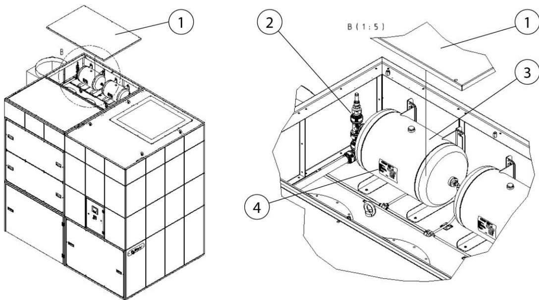
284. ábra: Hozzáférés a sűrítettlevegő-tartályhoz + biztonsági szelephez
