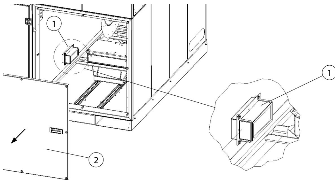
275. ábra: Hozzáférés a biztonsági szűrőhöz
