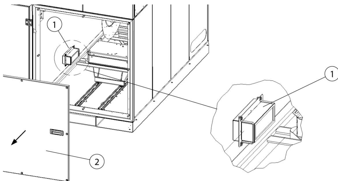
Sl. 347: Dostop do varnostnega filtra
