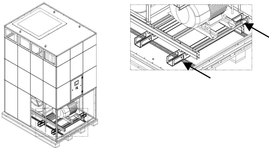
Рис. 156: Подъем вентилятора вилочным погрузчиком
