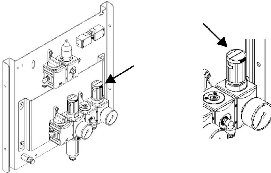
Rys. 103: Ustawianie ciśnienia podnośnika / zbiorczego pojemnika na pył
