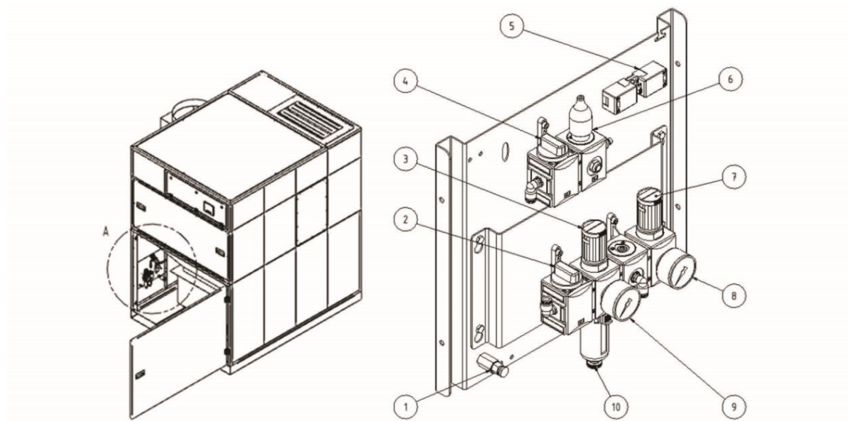
Рис. 172: Узел пневмосистемы
