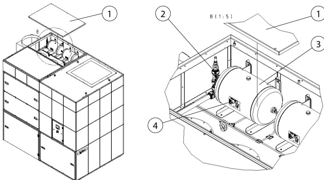
Sl. 356: Dostop do posode s stisnjnim zrakom in varnostnega ventila
