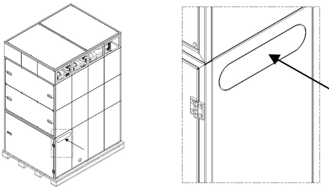
Sl. 302: Plošča z režo
