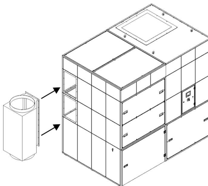
Obr. 27: Montáž přípojovací skříňe na straně sání
