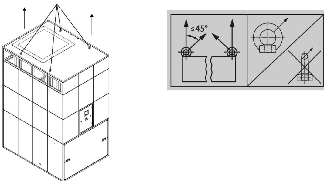
Рис. 163: Подъем вентилятора краном
