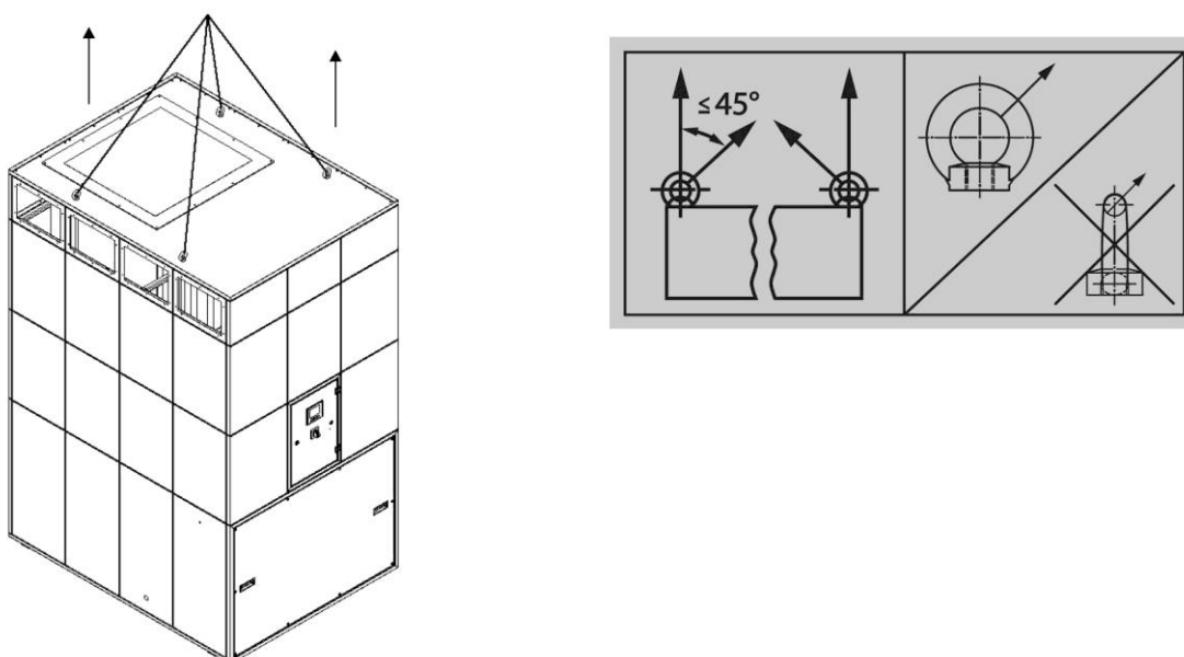
Rys. 83: Podnoszenie modułu wentylatora za pomocą dźwigu
