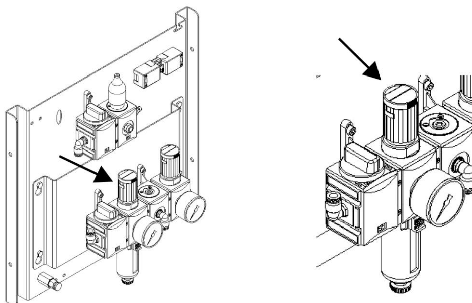
Rys. 102: Ustawienie ciśnienia roboczego
