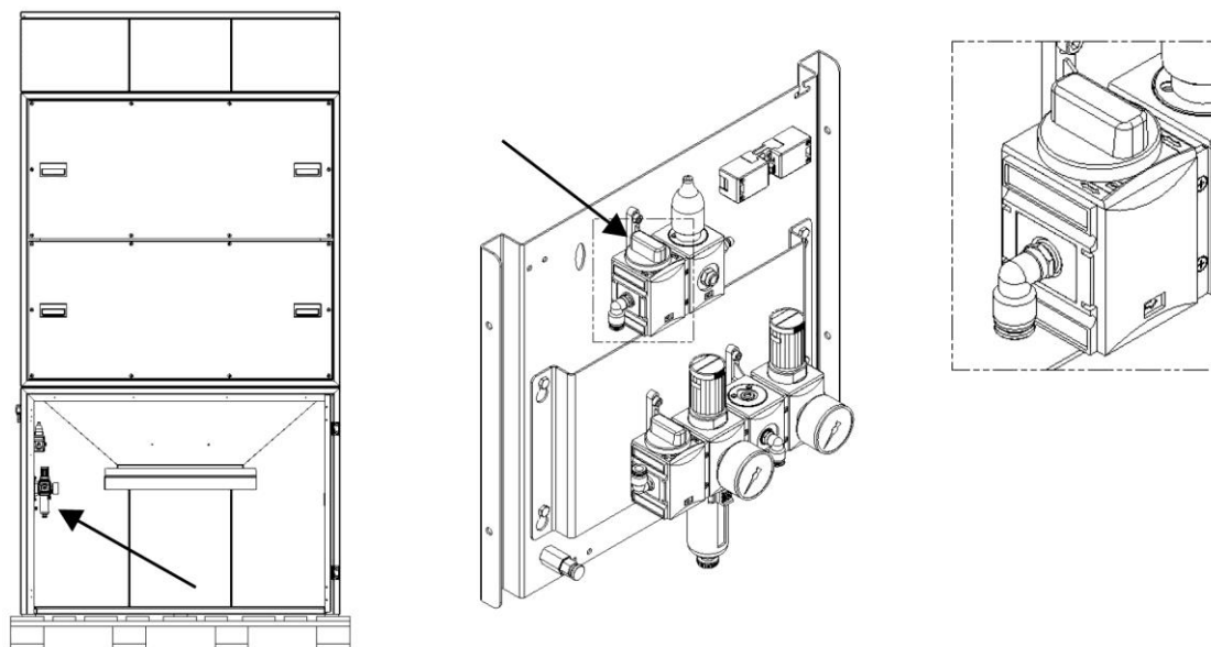
Sl. 303: Spustni ventil zbiralnika za prah
