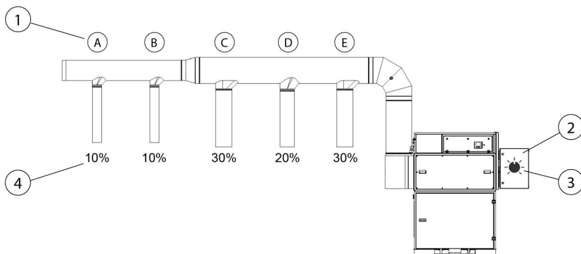
Рис. 199: Регулировка производительности вытяжки
