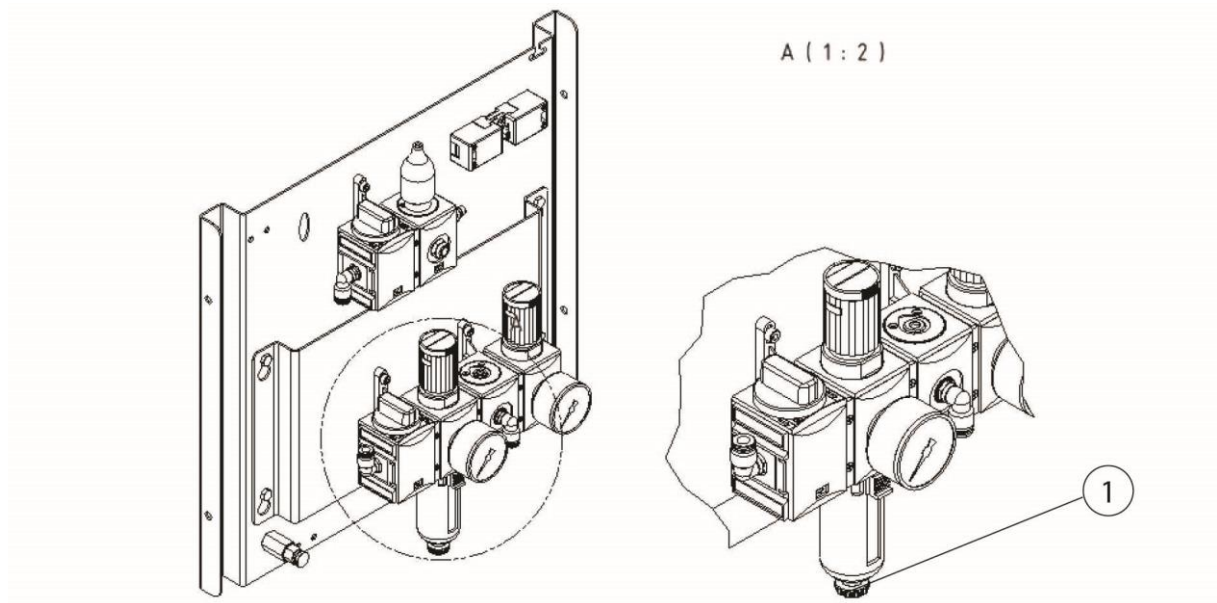
281. ábra: A sűrített levegős karbantartó egység kondenzvíz leeresztőszelepe
