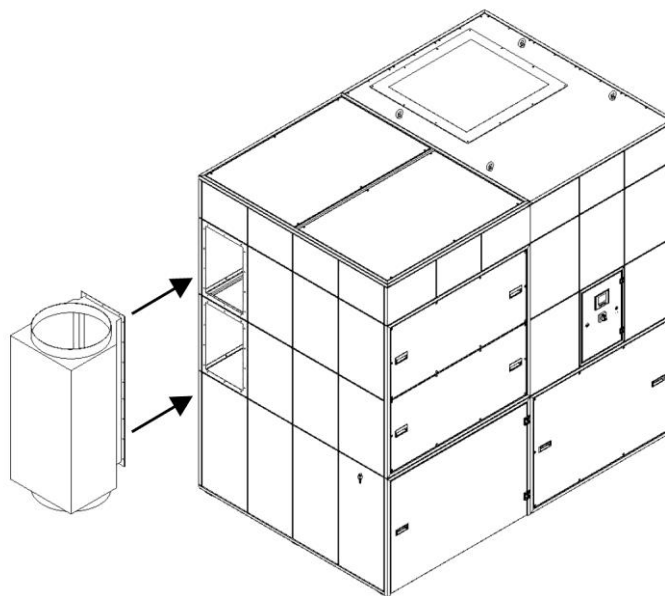
Sl. 315: Montaža priključne omarice na sesalni strani
