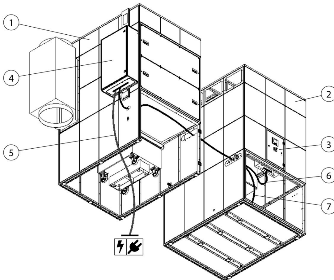
Obr. 34: Příklad: Pokládání kabelů regulace odsávacího výkonu
