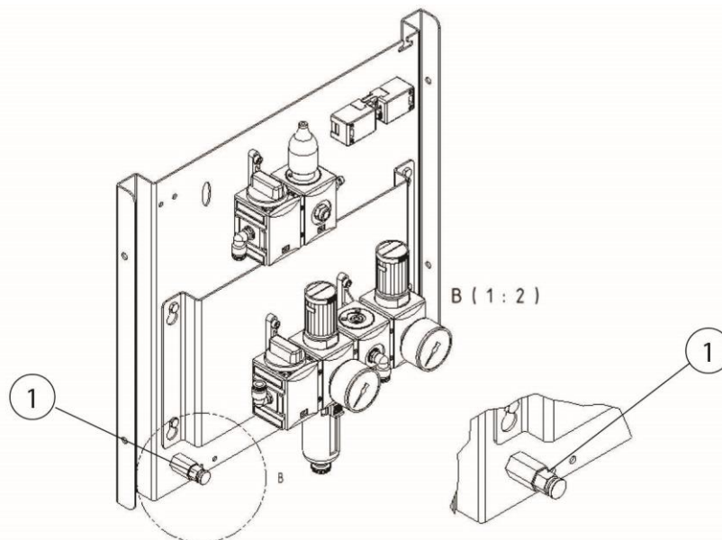
280. ábra: Sűrítettlevegő-tartály kondenzvíz leeresztőszelepe
