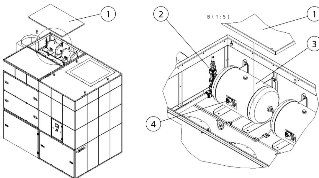
Rys. 140: Dostęp do zbiornika sprężonego powietrza + zawór bezpieczeństwa
