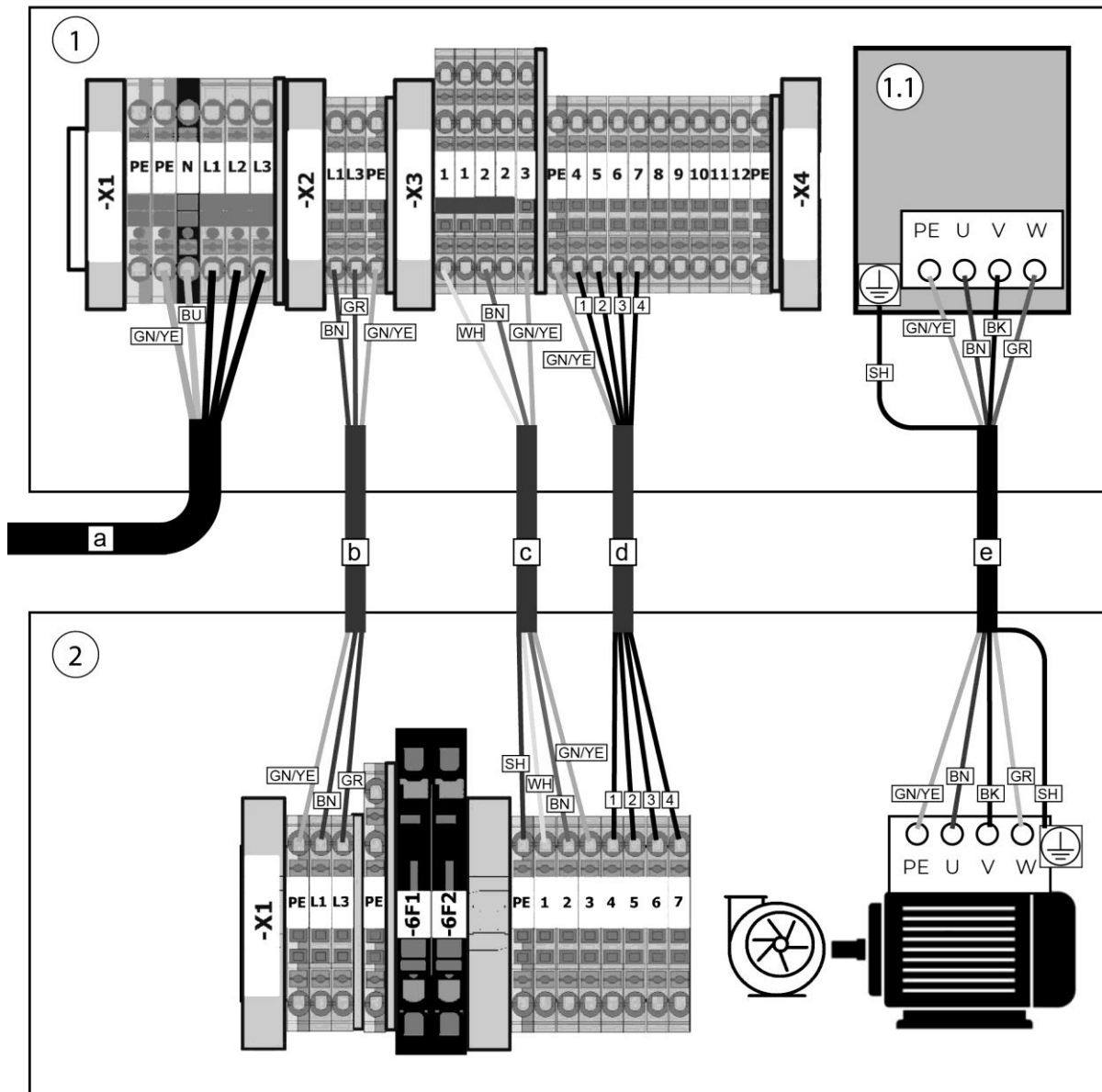
Rys. 108: Schemat połączenia układu regulacji mocy ssącej z produktem
