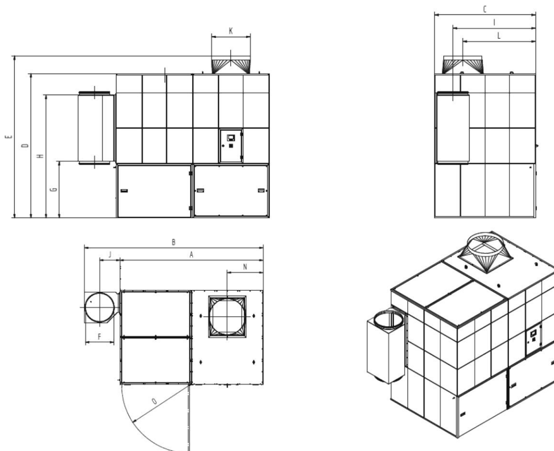
Sl. 358: List z merami 328528 + 328529 + 3211029
