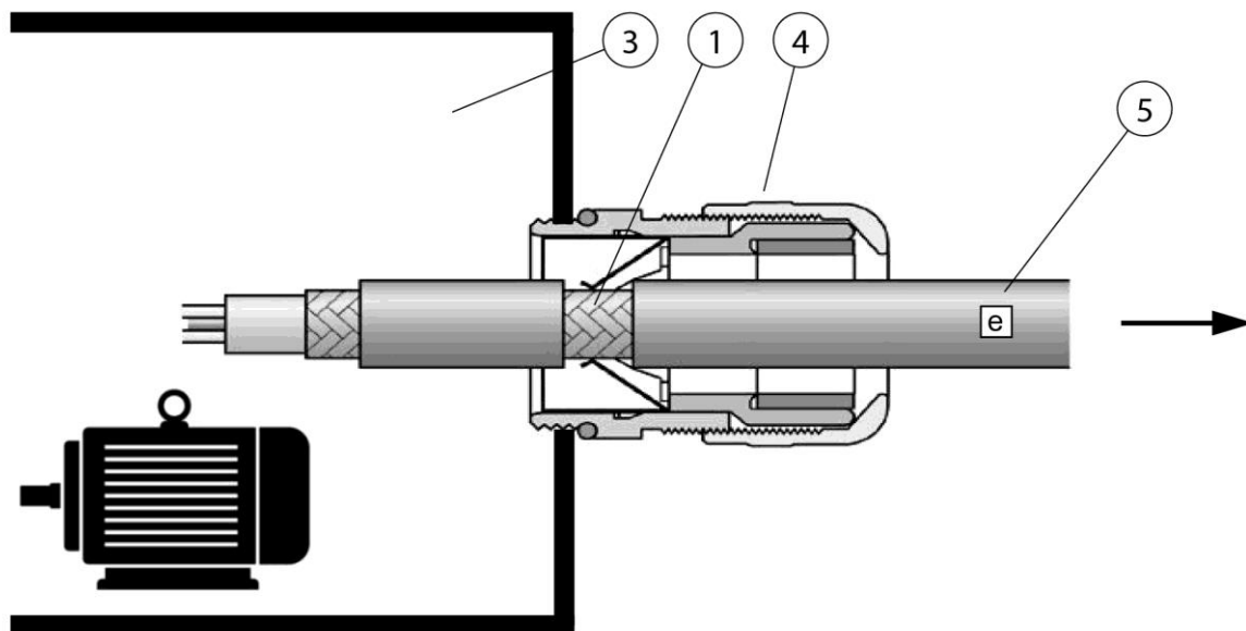
254. ábra: A motorkábel árnyékolásának csatlakoztatása
