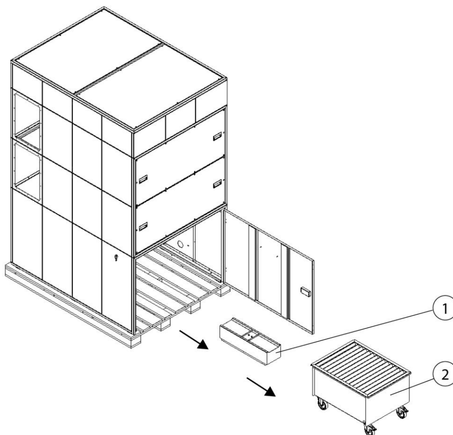
Rys. 89: Usunąć pojemnik zbiorczy pyłu i podnośnika
