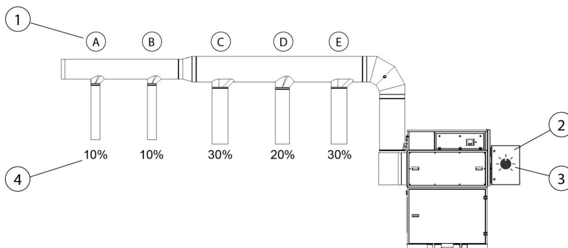
Obr. 55: Nastavení regulace odsávacího výkonu
