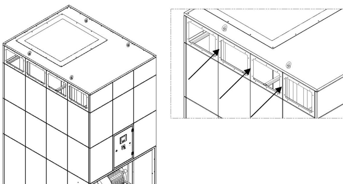
Rys. 85: Przelot czystego powietrza
