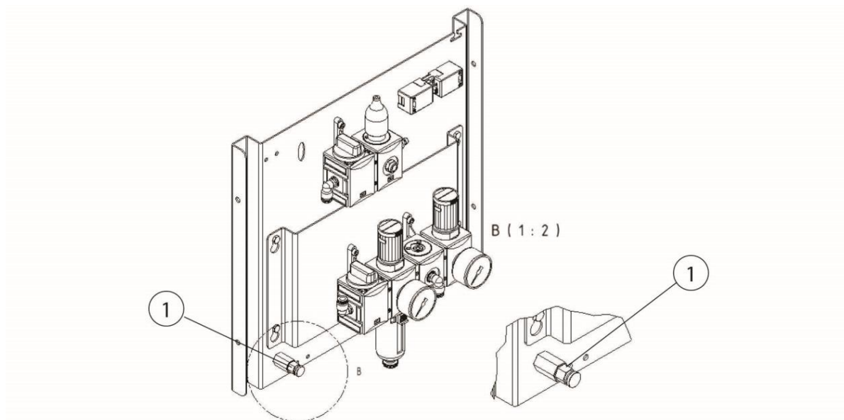
Sl. 352: Ventil izpusta kondenzata iz posode stisnjenega zraka
