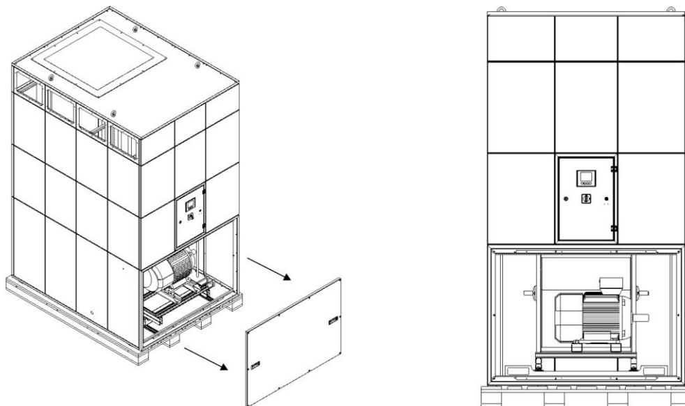
Obr. 10: Otevření servisních dvířek jednotky ventilátoru
