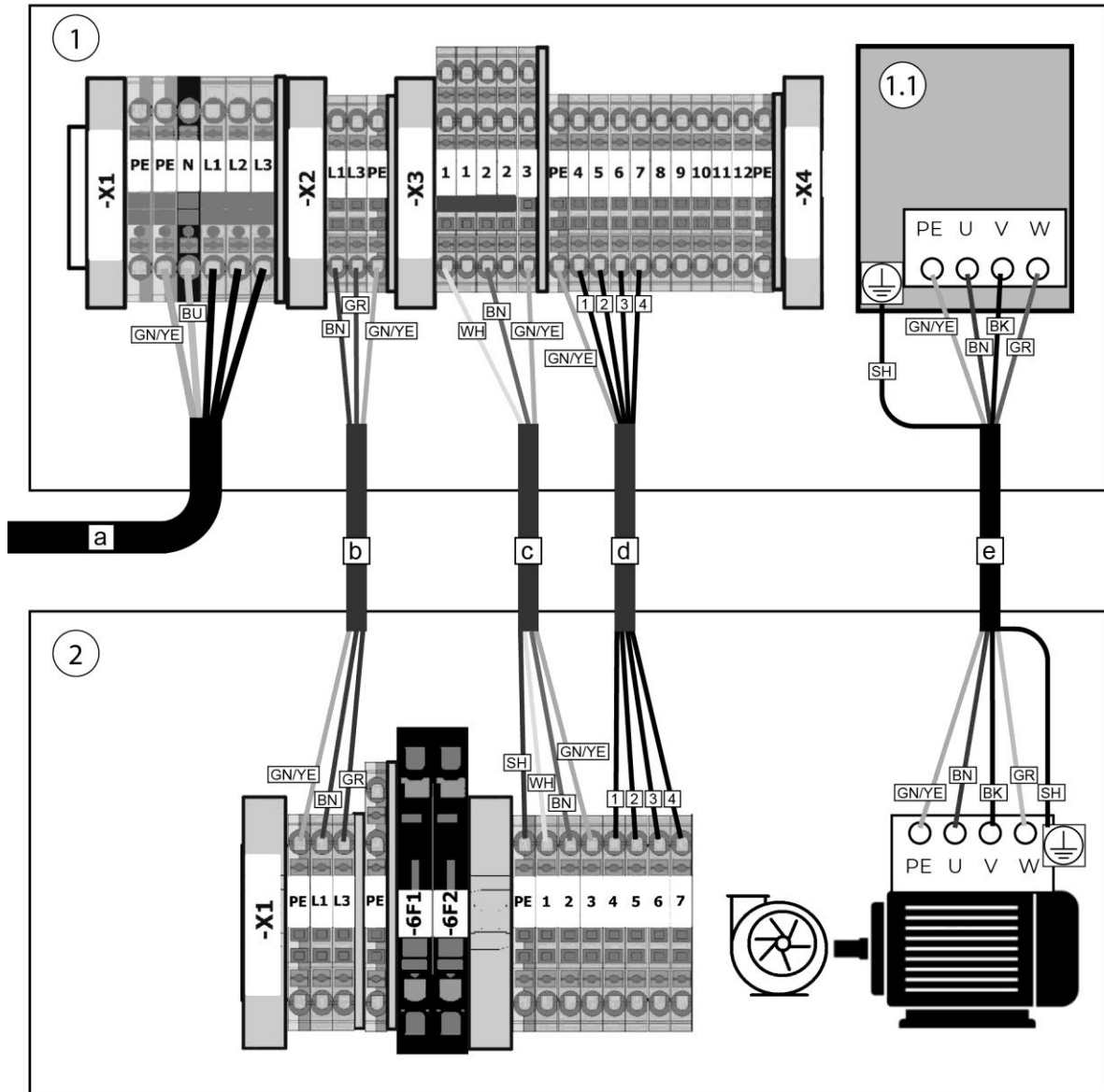
Рис. 180: Схема соединения системы регулирования мощности вытяжки с изделием
