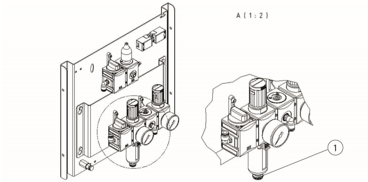
Sl. 353: Ventil odtoka kondenzata vzdrževalne enote s stisnjenim zrakom
