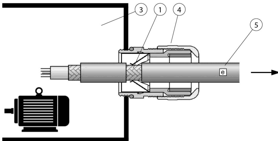
Рис. 182: Присоединение экранирующей плетки кабеля двигателя
