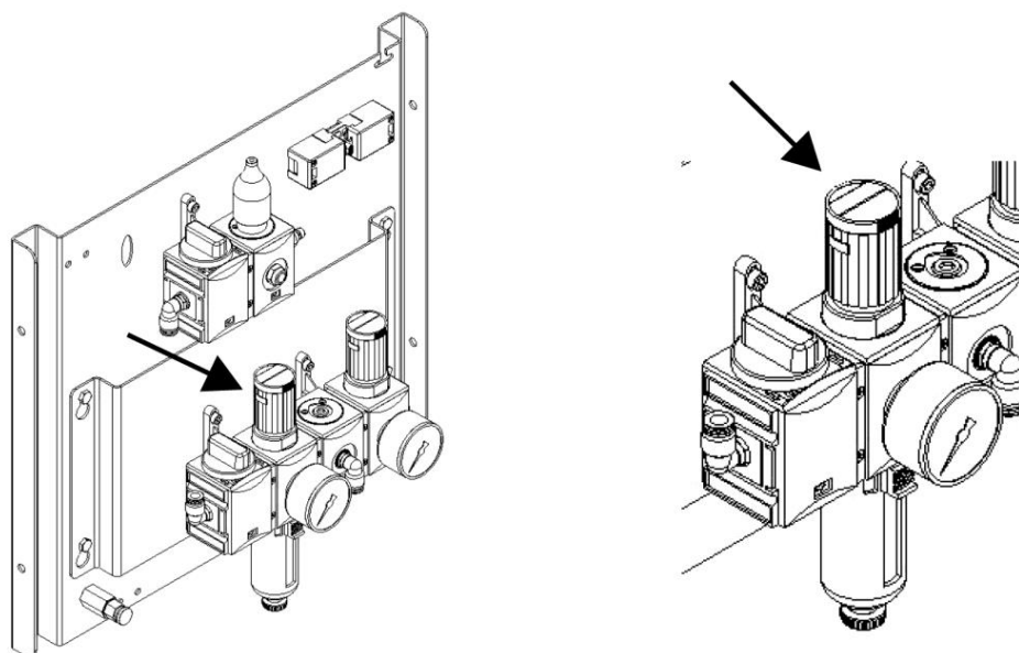
Рис. 174: Регулировка рабочего давления
