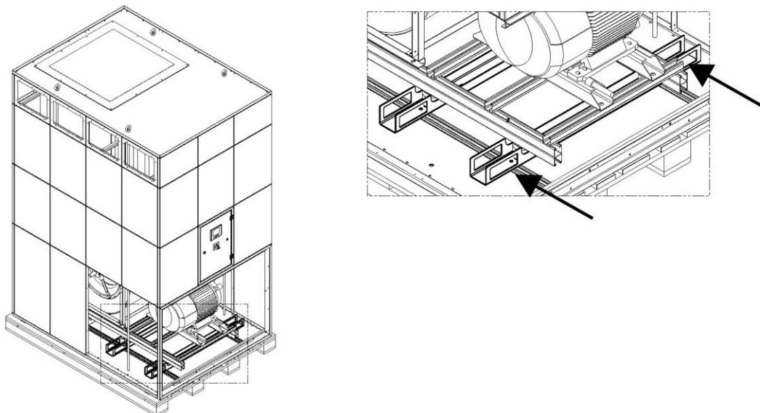
228. ábra: Ventilátorrész megemelése villás targoncával
