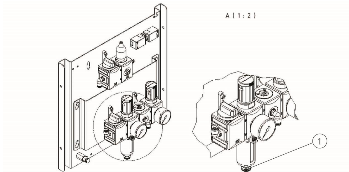
Рис. 209: Вентиль слива конденсата узла подготовки воздуха
