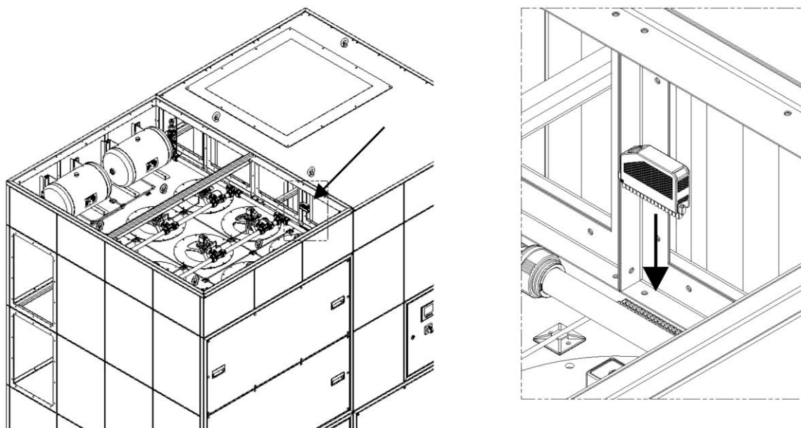
Rys. 95: Montaż zielonej wtyczki
