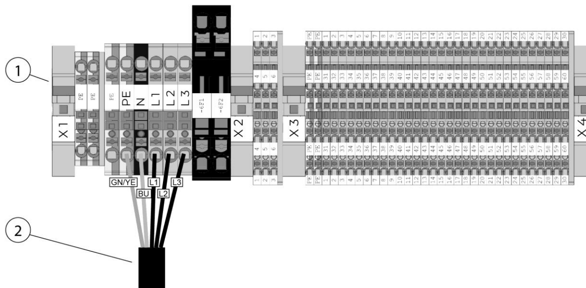
Obr. 33: Připojovací svorkovnice ve skříňovém rozvaděči výrobku
