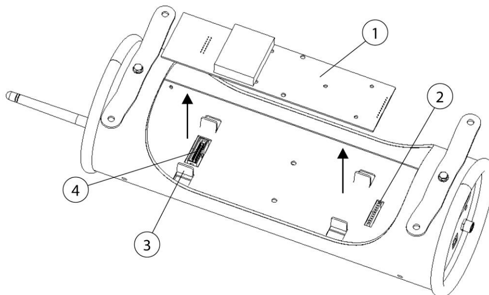
Rys. 116: Wymiana płytki czujników
