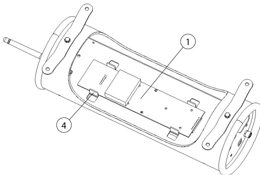
Rys. 115: Płytkę czujników
