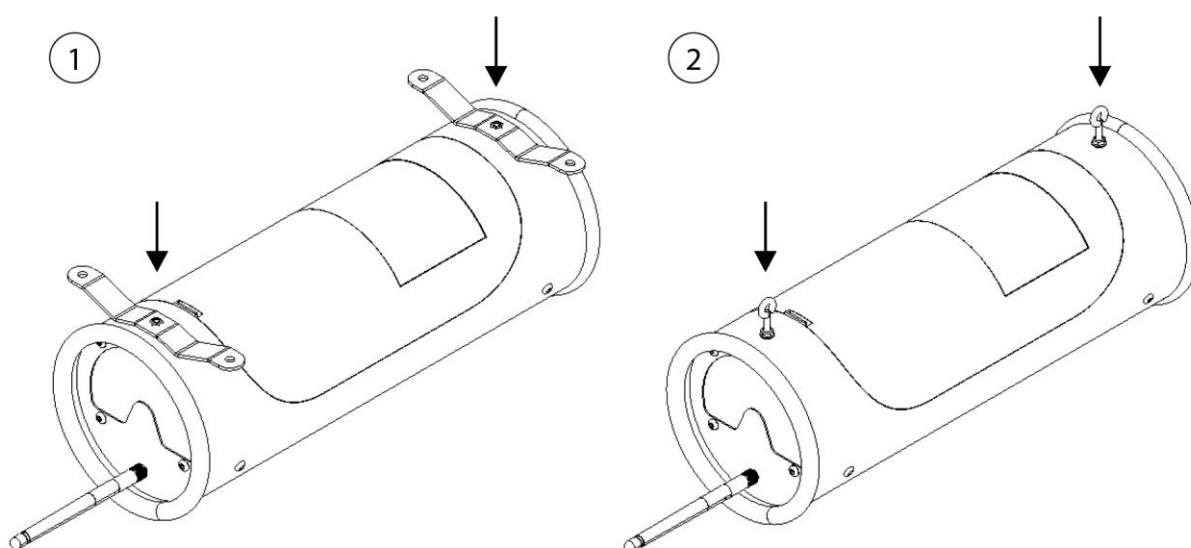
137. ábra: Szerelési változatok
