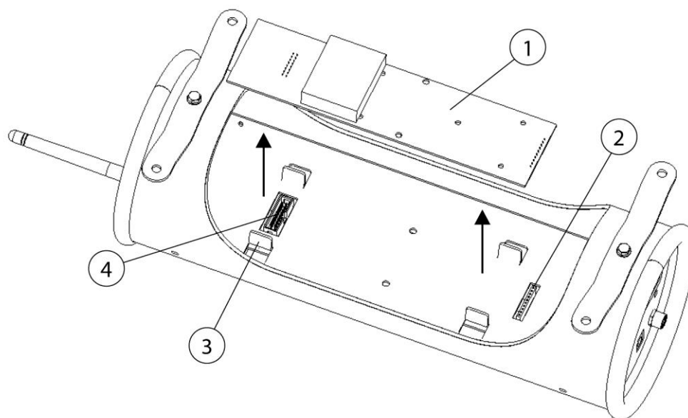
Sl. 155: Menjava tipalne plošče
