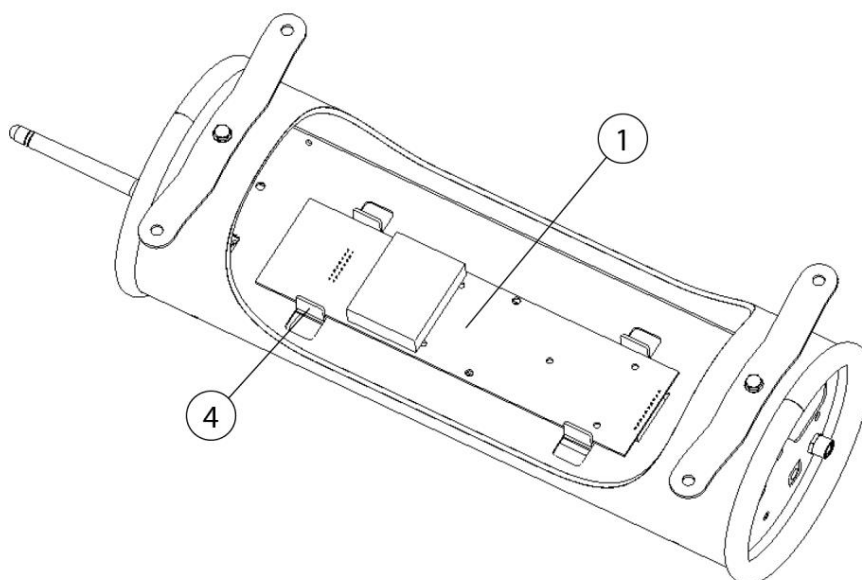
Fig. 76: Placa do sensor
