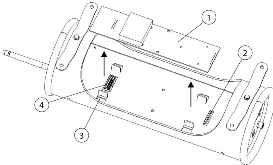
Abb. 12: Sensorplatine wechseln
