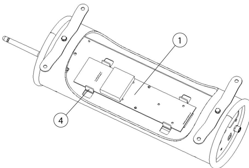
Obr. 102: Deska senzorů
