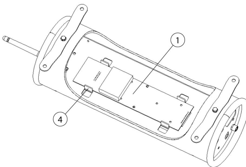
Fig. 89: Scheda del sensore
