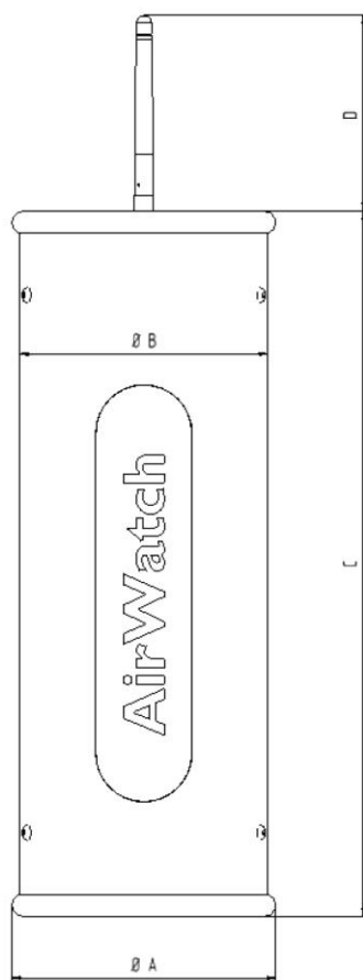
Fig. 91: Disegno quotato
