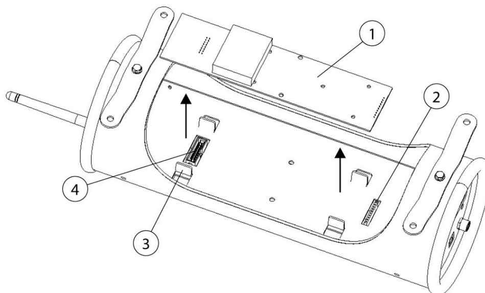
Afb. 51: Sensorprintplaat vervangen
