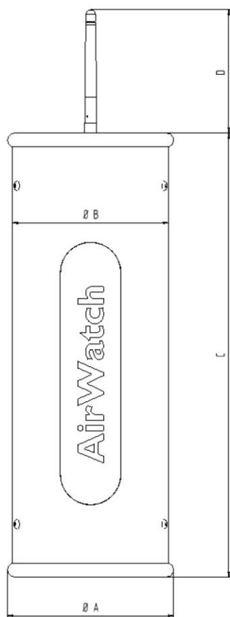
Fig. 78: Folha de dimensões
