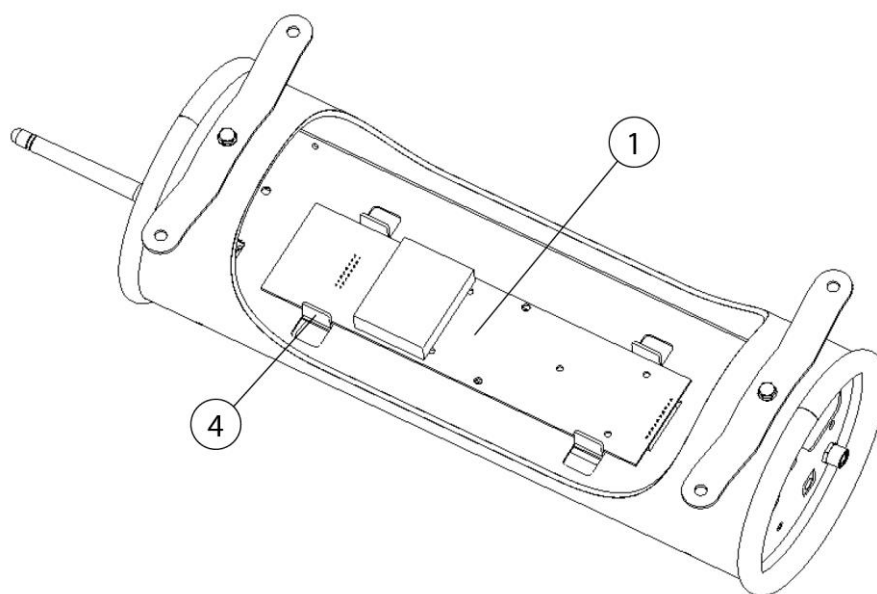
141. ábra: Érzékelőkártya
