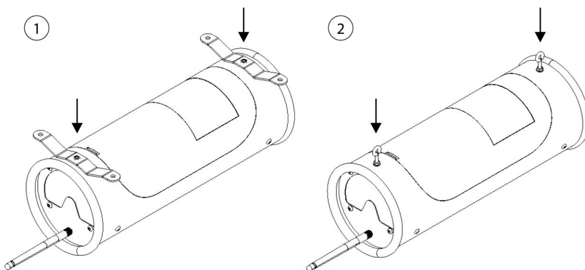
Rys. 111: Warianty montażu
