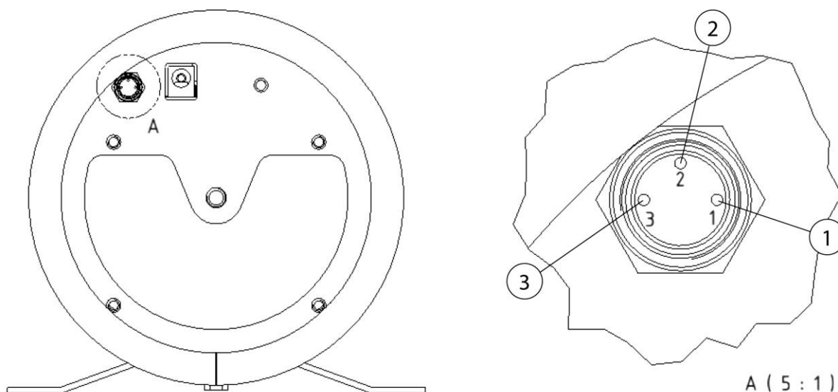
140. ábra: M8 csatlakozóaljzat PIN-kiosztása
