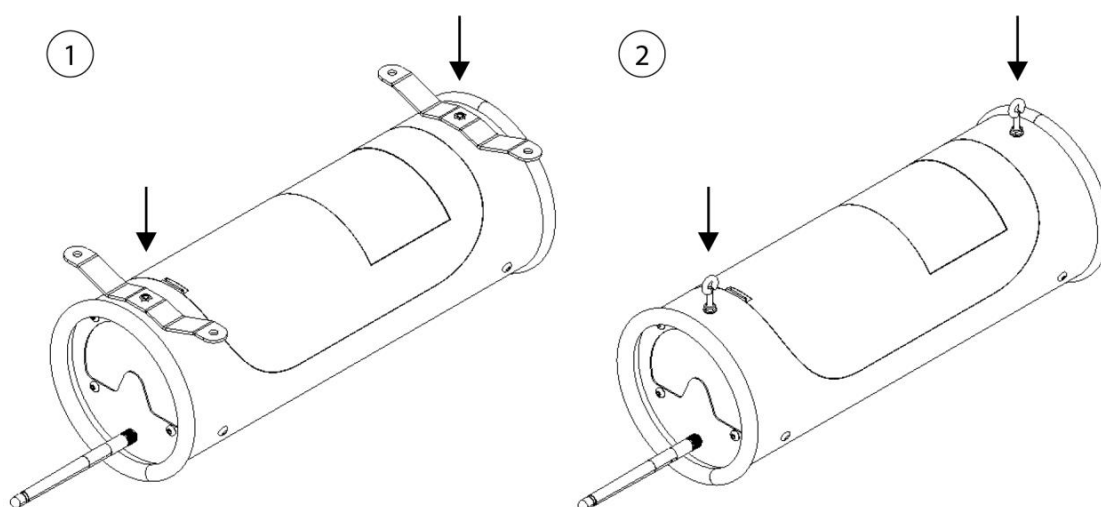
Afb. 46: Montage-varianten
