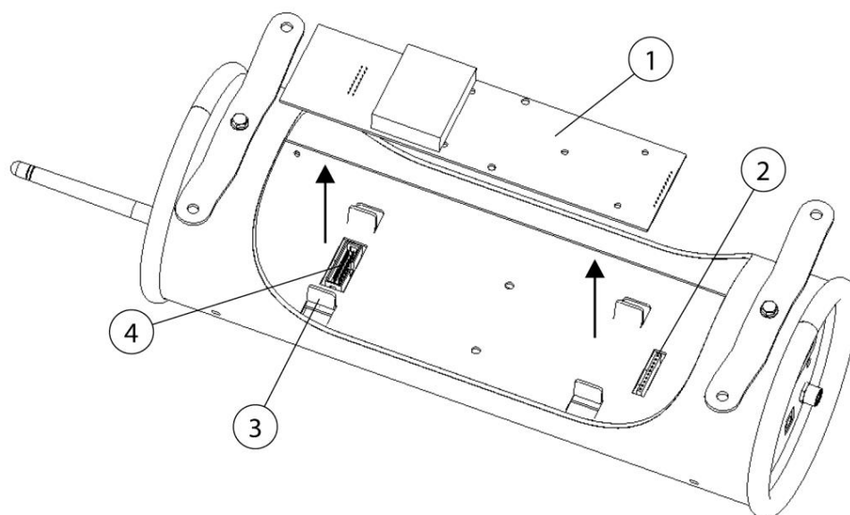
Fig. 77: Substituir a placa do sensor
